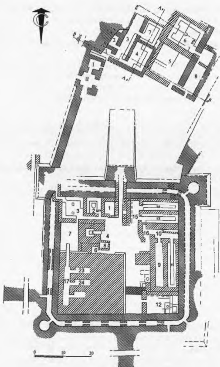
Актепа Юнусабад. План. VII—VIII вв.
