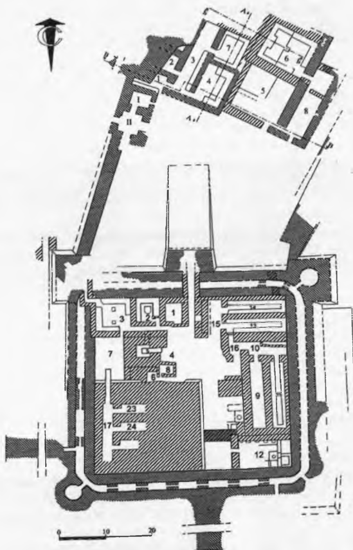
Юнусобод Оқтепаси. Тарҳ. Эрамизнинг VII—VIII асрлари.
