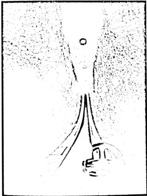
Мирзо Улуғбек расадхонаси. Самарқанд.
