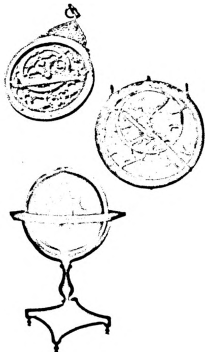
Қадимги астрономик асбоблар.
