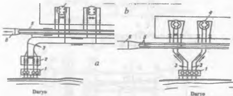
1.5-rasm. Issiqlik elektr stansiyalar (IES) ni suv bilan ta'minlash tizimi nasos stansiyalar chizmasi:
