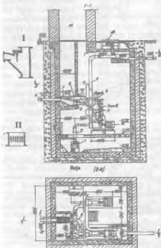
4.6 - r a s m . ToshTYMI tipidagi eksperimental nasos stansiyasi
