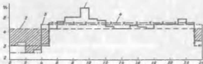
2.1-rasm. Suv iste'moli va nasos stansiyasining bir tekisda hamda pog'onali uzatishining birlashtirilgan grafiqi
