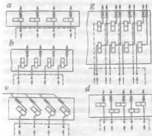
3.7-rasm. Gorizontal markazdan qochma nasosli agregatlarning joylashishi.
