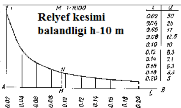
3.4-rasm. Nishablik masshtabi grafigi
