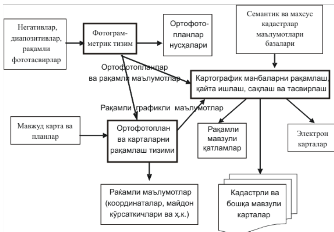
20.1-rasm. Yer resurslari xaritasini yaratishning blok-chizmasi
