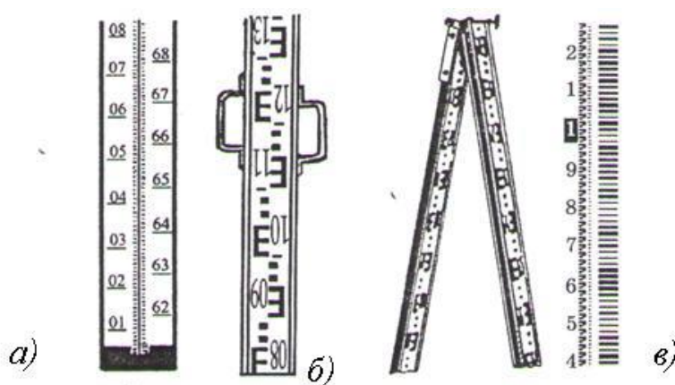
6.9-rasm. Nivelirlash reykalari
