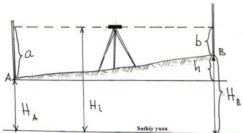
6.11-rasm. O`rtadan nivelirlash
