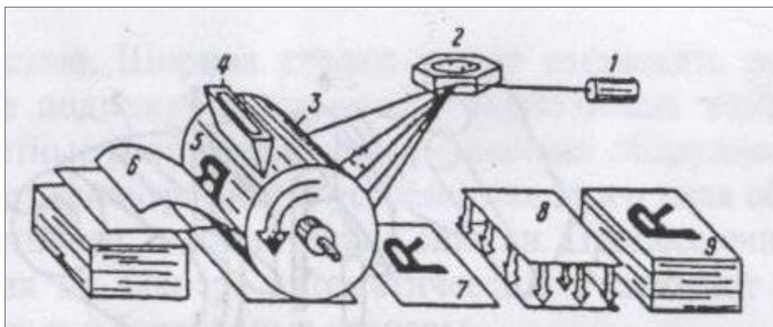
22.13-rasm. Elektronografik (lazyer) printyerlarning ishlash chizmasi.
