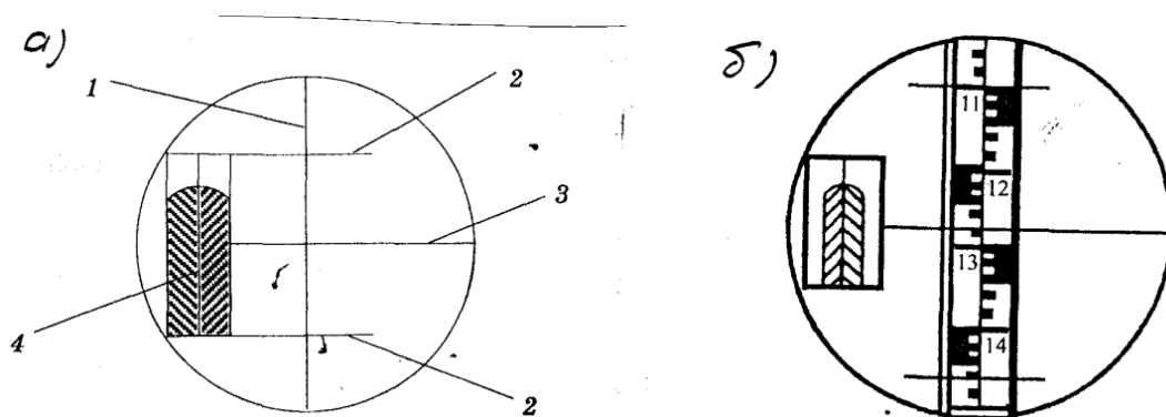
6.7-rasm. 1-vertikal ip; 2-dalnomer iplari; 3- o'rta ip; 4- silindrik adilak pufakchasining uchlari ,bir-biriga to'g'ri keltirilgan (kontakt) holati; 6) qarash trubasida reyka tasviri
