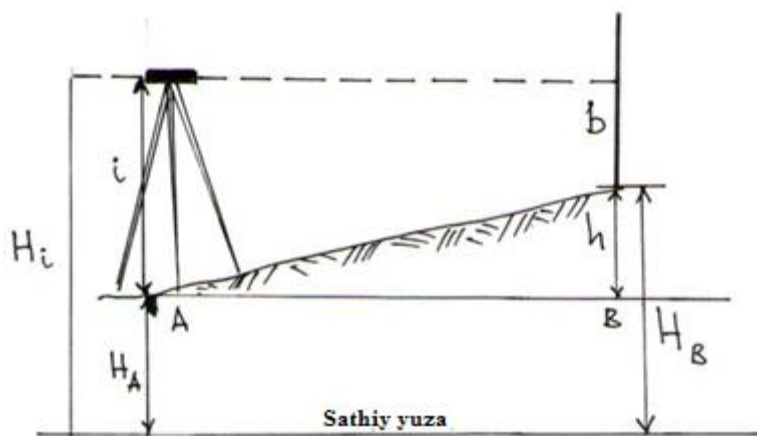
6.10-rasm. Oldinga nivelirlash
