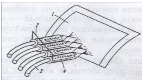
22.14-rasm. Oqimli (struyali) printyerni tuzilishi
