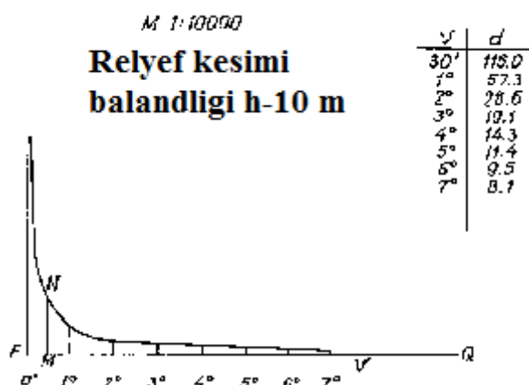
3.3-rasm. Quyilish mashtabi grafigi
