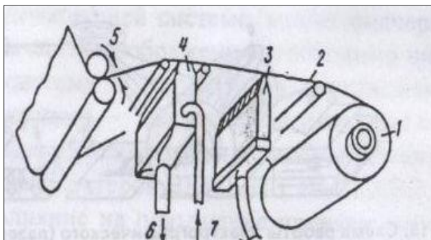
22.12-rasm. Elektrostatik bosma uskunaning ishlash chizmasi.
