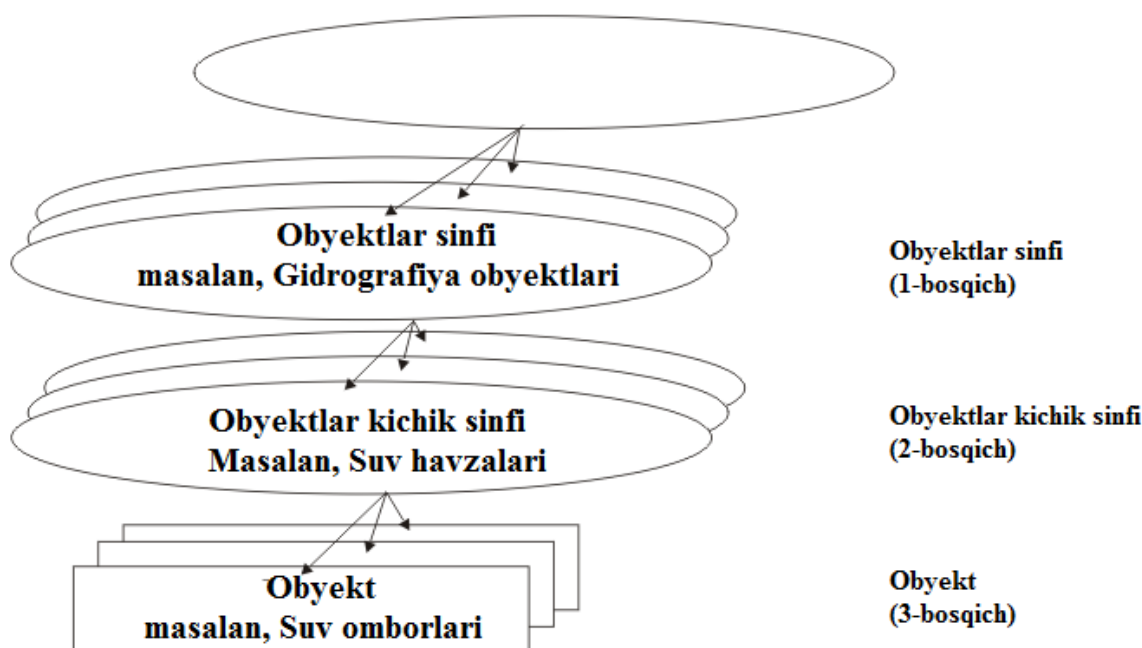
22.17-rasm. Ma'lumotlar bazasi iyerarxik modelida tasvirlash
