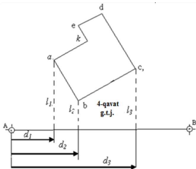
6.2-rasm. Perpendikulyar usul
