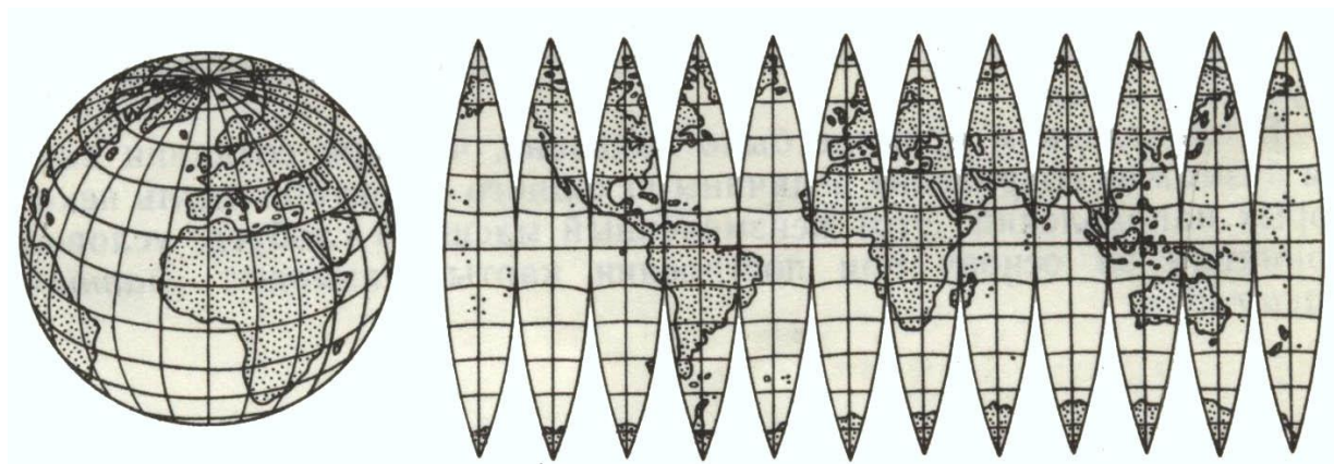
8.2-rasm. Meridianlar bo'yicha zonalarga (tilimlarga) bo'lingan globus yuzasi. Yerning egri yuzasini tekislikda uzilishsiz tasvirlab bo'lmasligini tasdiqlovchi sxema
