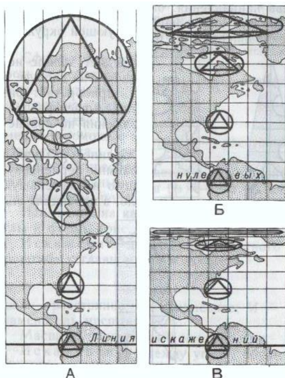
8.4-rasm. Slindrik proyeksiyalarda tuzilgan xaritalardagi xatoliklar ellipsi
