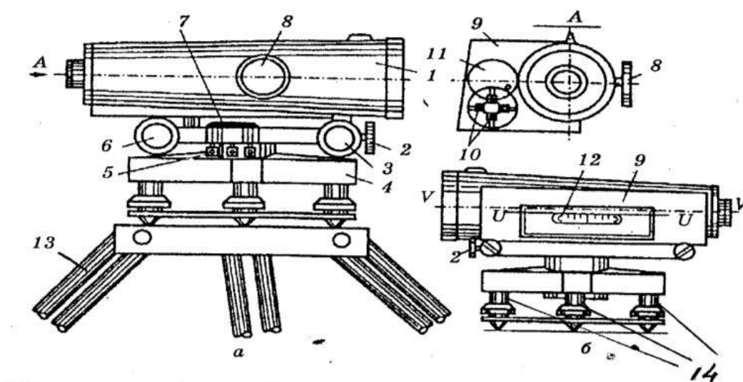
6.6-rasm. H3 niveliri tuzilishi
