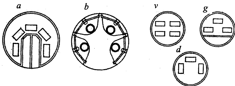
3.9-rasm. Doira shaklidagi mashinalar binosida agregatlarning joylashishi
