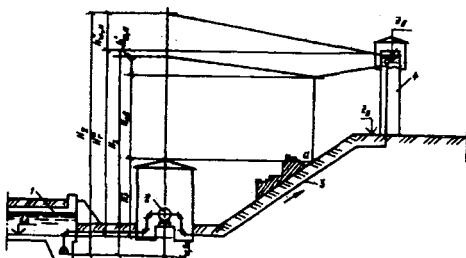
2.4-rasm. Rezervuardan suvni kontrezervuarli tizimga uzatishning balandlik sxemasi
