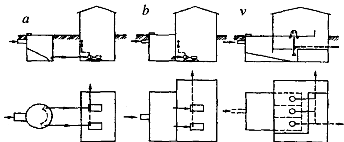
4.3-rasm. Loyqa va cho'kmalarni haydash nasos stansiyalarining sxemalari
