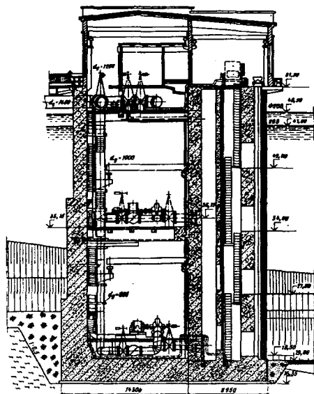
3.22-rasm. Tog'-kon kombinatini suv ta'minoti aylanma tizimidagi sirkulyatsiya nasos stansiyasi
