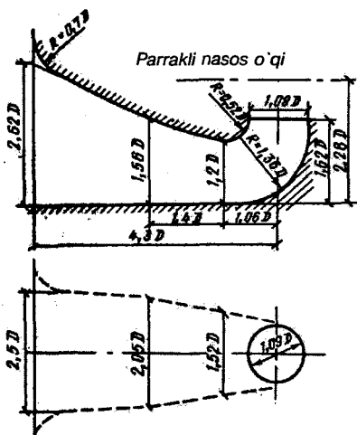
3.5-rasm. O'qli nasosdagi qayrilgan so'rish quvuri
