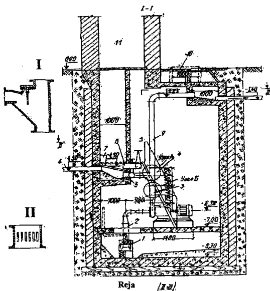
4 . 6 - r a s m . Tosh TYMI tipidagi eksperimental nasos stansiyasi
