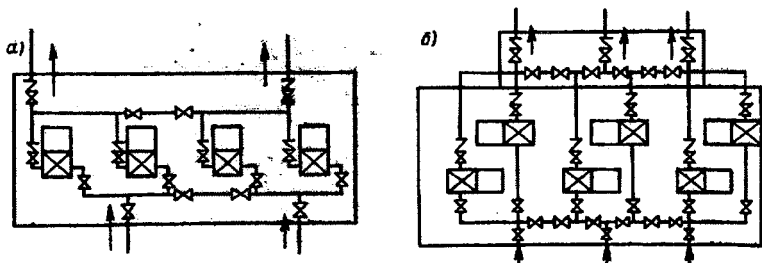
3.4-rasm. Soʻrish va siquv quvurlaridagi kollektorli ulanishlar
