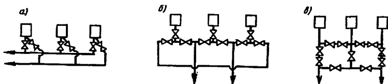
3.6-rasm. Siquv quvurlarini seksiyalar ichi kommunikativlari
