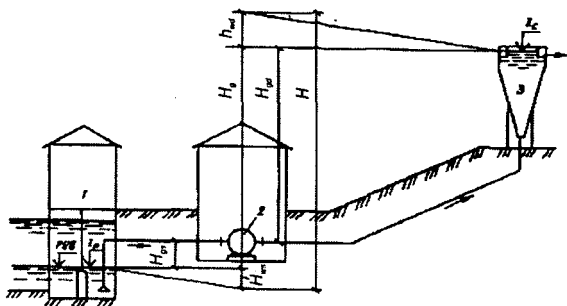
2.2 — rasm. Suvni tozalash inshootlariga suv uzatish balandligi sxemasi 1-suv qabul qiluvchi qirg'oq qudug'i; 2-nasos; 3-aralashtirgich; RUV-suvning hisobiy sathi.
