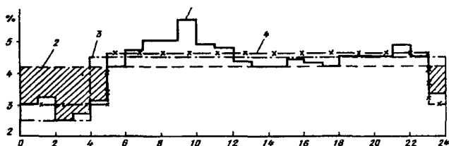
2.1-rasm. Suv iste'moli va nasos stansiyasining bir tekisda hamda pog'onali uzatishining birlashtirilgan grafigi
