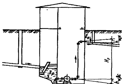
4.4-rasm. Oqova suvni chuqurlashgan kollektordan yuqoriga uzatish sxemasi
