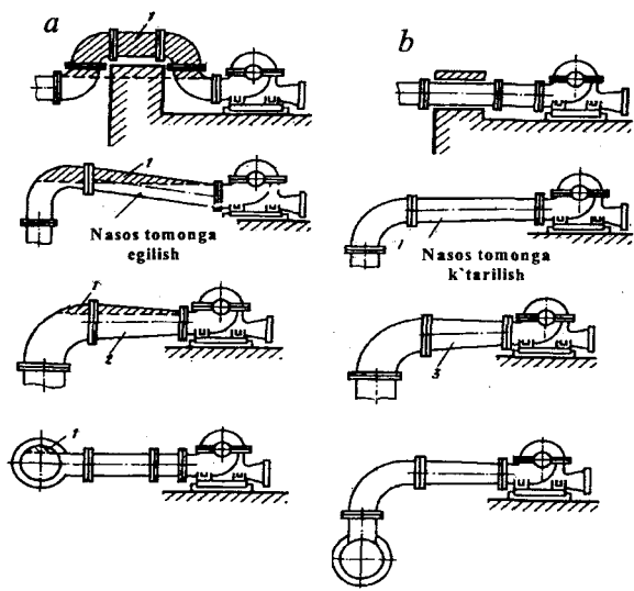
3.1-rasm. So'rish quvurlarini to'g'ri (a) va noto'g'ri (b) joylashishi
