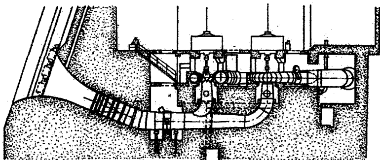
3.8-rasm. Kashi-el-Jirba (Sudan)dagi 1-ko'taruv nasos stansiyasi
