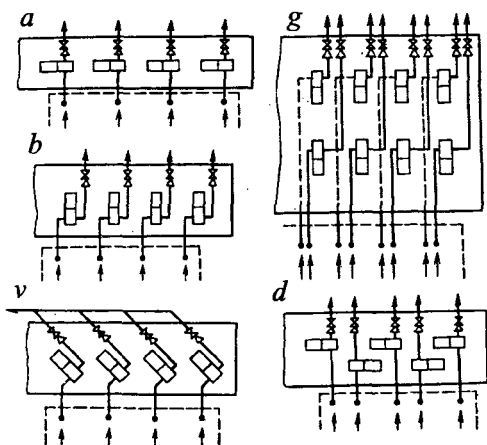
3.7-rasm. Gorizontaal markazdan qochma nasosli agregatlarning joylashishi.
