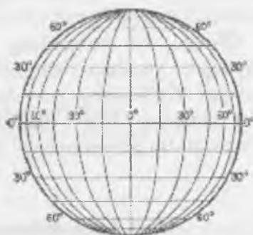
31-rasm. Ko'ndalang ortografik proyeksiya
