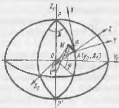
1-rasm. Geosentrik va toposentrik fazoviy koordinatalar tizimlari
