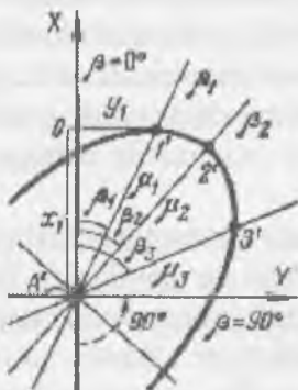
8-rasm. Xatoliklar ellipsi elementlari
