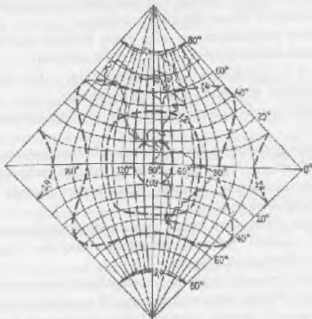
68-rasm. Adams proyeksiyasida r izokollalari
