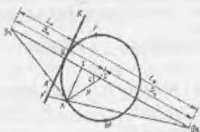
28-rasm. Negativ va pozitiv tasvirli perspektiv proyeksiyalarni hosil qilish sxemasi
