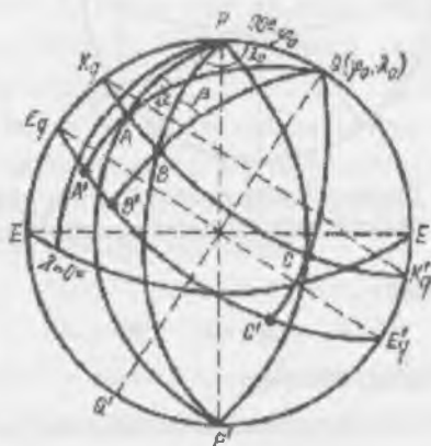
21-rasm. Berilgan uchta nuqta ho'yicha (A, B, C) qutb koordinatalarini hisoblash chizmasi
