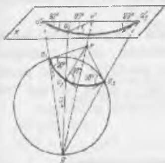
30-rasm. Stereografik proyeksiyaning asosiy xossasini isbotlash sxemasi
