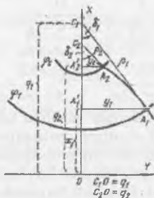
50-rasm. Yarim konusli proyeksiyalarning koordinatalari tizimi
