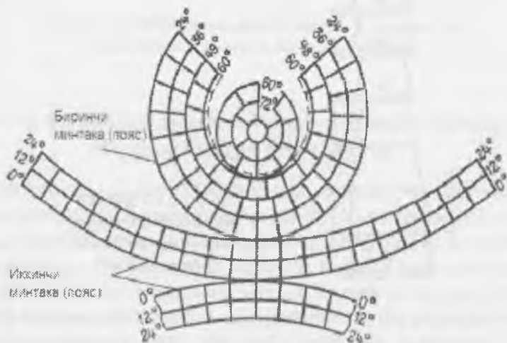
61-rasm. 1:2 500 000 masshtabli kartada zonalarining joylashish sxemasi.
