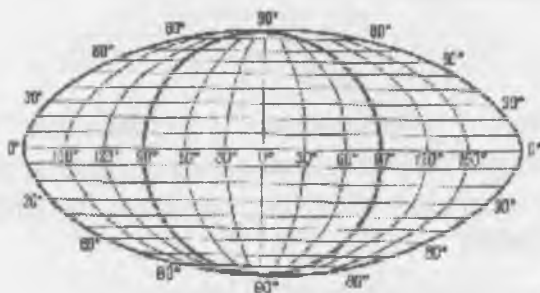
44-rasm. Qutbi nuqta bo'lgan teng maydonli elliptik pseudosilindrik proyeksiya
