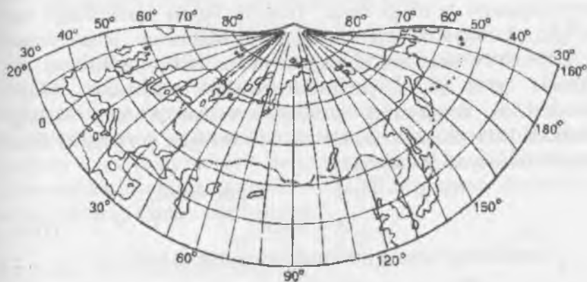
48-rasm. Ko'rinishi o'zgartirilgan Bonn proyeksiyasi
