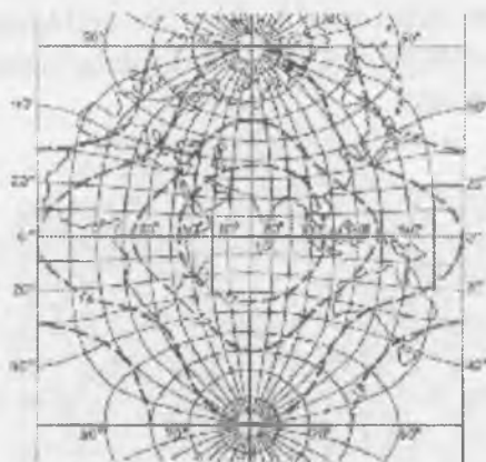
66-rasm. Gyuy proyeksiyasida p izokolalari
