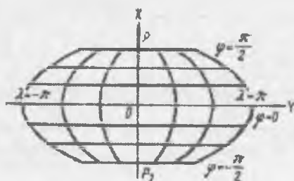
42-rasm. Psevdosilindrik proyeksiyalar koordinatalari tizimi
