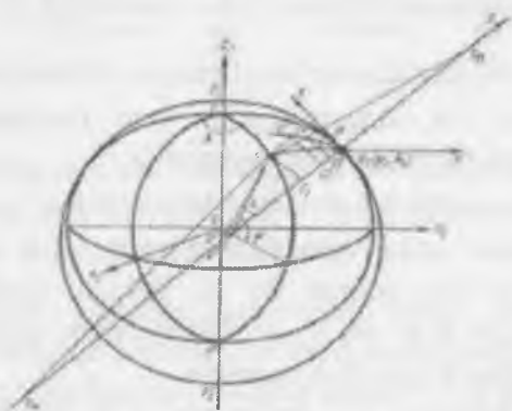
11-rasm. Sferada ellipsoidni perspektiv tasvirlash
