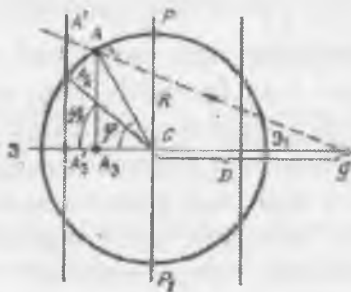
40-rasm. Normal perspektiv-silindrik proyeksiyani hosil qilish
