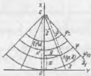
22-rasm. Normal konusli proyeksiyada koordinatalar tizimi
