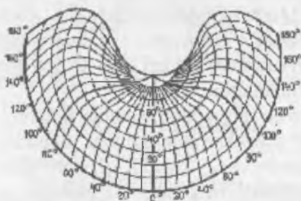
16-rasm. Psevdokonusli proyeksiya
