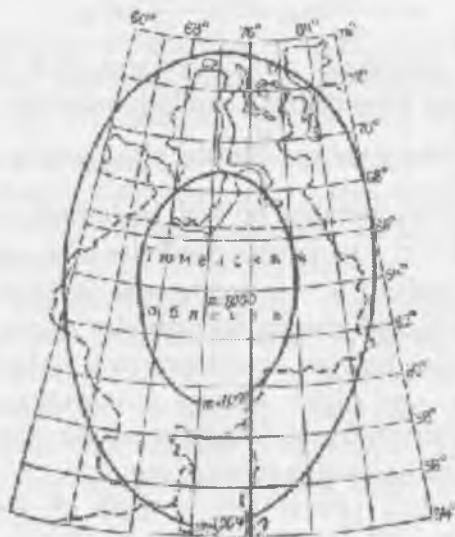
65-rasm. Qatorlardan foydalanish yo'li bilan hosil qilingan Tyumen viloyati kartasi proyeksiyasi.
