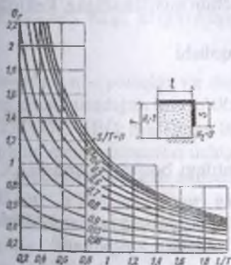
3.12-rasm. Ichki fragment uchun keltirilgan sarf Q ni aniqlash grafigi ( H_1 va H_2 – fragment chegaralaridagi bosim).
