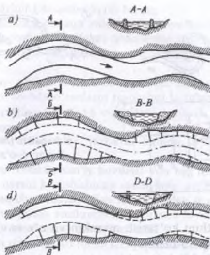
7.14-rasm. O'zanni toraytirish sxemalari:
