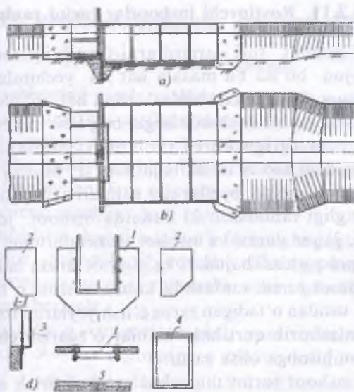
5.24-rasm. Yig'ma konstruksiyali ochiq temir-betonli rostlagich:
