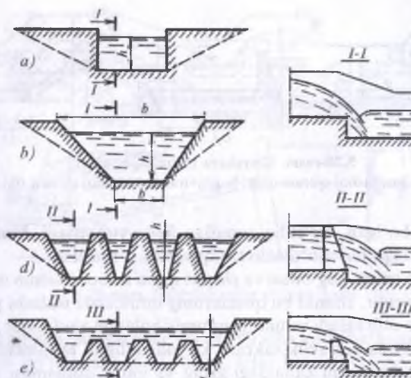
5.27-rasm. Sharshara kirish qismi sxemalari: a—to'g'ri burchakli; b—trapetsiya; c—tirqishli; d—tepasimon
