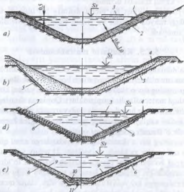
5.3 - rasm. Kanal qoplamalari sxemasi: a - gruntli (loyli ekran bilan); b - polimerli (sintetik plyonka bilan); d - to'kilgan toshli yoki tosh yotqizilgan; e - ko'ndalang va bo'ylama chok o'rnatilgan beton va temir-betonli; 1, 4, 9 - himoya qatlami mos ravishda qalinligi 0,2 m li shag'aldan, beton plitadan, 2 - loyli ekran; 3 - muz; 5 - simmetrik plyonka; 6 - graviy qumli to'shama; 7 - qalinligi 0,1...0,3 m li to'kilgan tosh; 8 - bir qatorli to'shama tosh; 10 - o'lchami 8x8 sm li yog'och to'sin; 11 - drenaj.
