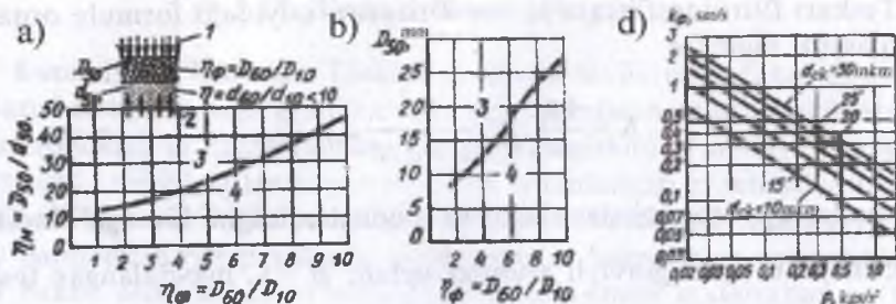
3.31-rasm. Teskari filtrlarni tanlash grafiklari:
