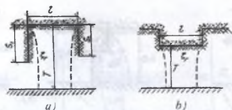
3.20-rasm. Gorizontalar fragmentlar sxemalari.
