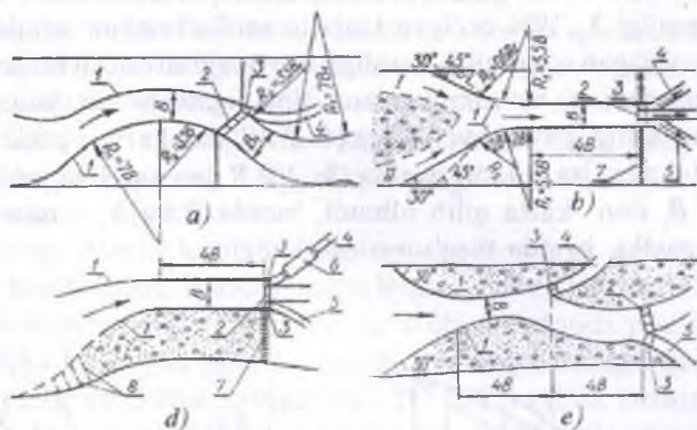
7.11-rasm. To'g'onli suv olishda daryo o'zanlarini rostlash sxemalari:
