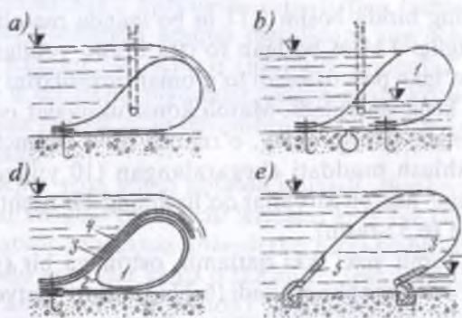
6.32-rasm. Matoli zatvorlar konstruktiv sxemalari: 1-havo; 2-ichki qobiq; 3-ushlab turuvchi qobiq; 4- himoyalovchi qobiq; 5-metall tasma.
