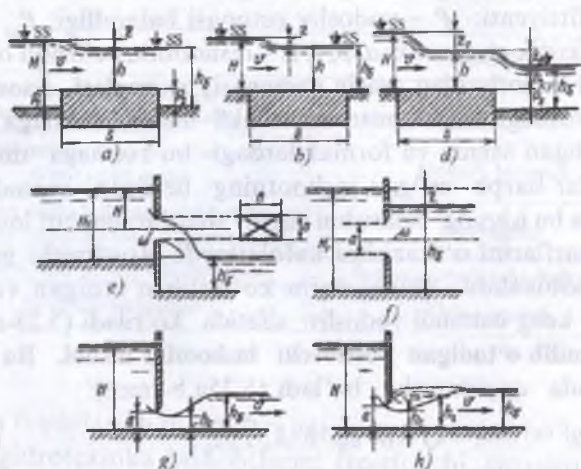
5.25-rasm. Ochiq rostlovchi inshootlar gidravlik hisobi sxemalari: a – ko'tarilgan keng ostonali vodosliv; b – tubda joylashgan oqim ko'milib o'tadigan keng ostonali vodosliv;
