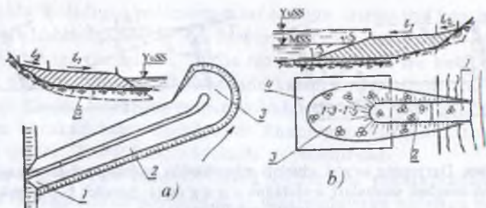
7.29-rasm. Poluzapruda turlari va ularning asosiy elementlari: a- kotlovanga monolit mustahkamlangan mahalliy gruntli poluzapruda; b- har xil materiallardan terilgan, tubi va qiyaliklariga egiluvchan qilib mustahkamlangan proluzaprudalar; 1- o'zak, 2- tana; 3- bosh; 4- tubdagi to'shama; 5- kotlovan.
