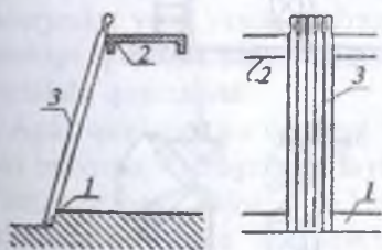
6.8-rasm. Yog'och spitsalar: 1-flyutbetga o'yilgan chuqurcha; 2-xizmat ko'prigi; 3-spitsalar.
