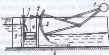
6.47-rasm. Muvozanatlashtiruvchi po'kak-posangili segmentli zatvor-avtomat sxemasi:
