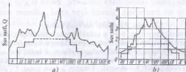
7.31- rasm. To'g'onsiz suv olish qo'llanishi shartlari: a – daryoning gidrografi va suv iste'moli grafigi; b – daryo va kanalning suv sathi o'zgarish grafiqlari.
