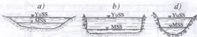
7.6-rasm. Daryoning tekis va o'rta uchastkalari ko'ndalang kesimlari: a-qirg'oqlari va zamini yuviladigan; b-qirg'oqlari yuviladigan; d-qirg'oqlari va zamini yuvilmaydigan.
