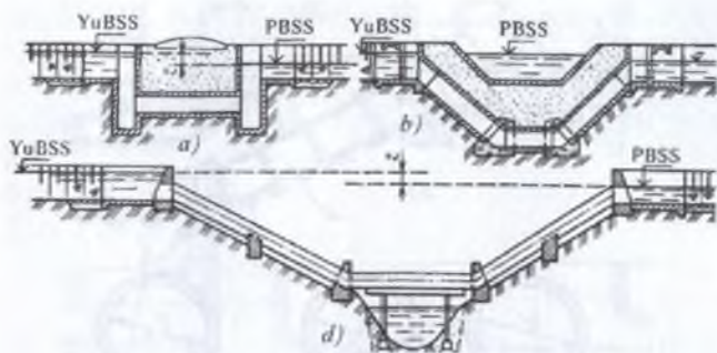
5.41- rasm. Dyukerlarning asosiy konstruktiv sxemalari: a–yopiq, quduqli; b–yopiq, egri chiziqli, d–ochiq, soy bilan kesishgan joyda oʻrnatilgan.
