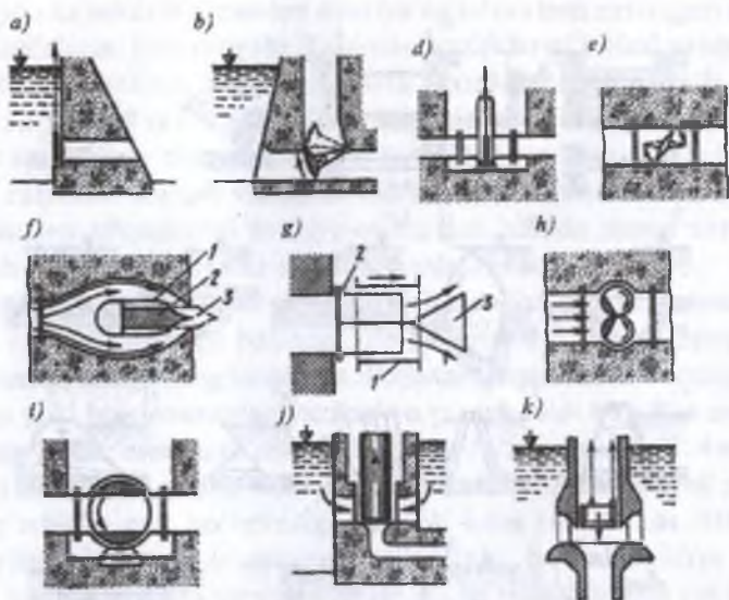
6.2-rasm. Chuqur joylashgan asosiy zatvorning turlari.
