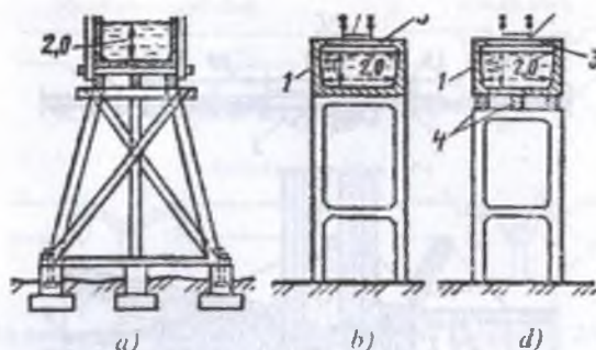
5-48-rasm. Estakadadagi novlar: a-yog'ochli; b,d -temir-betonli; 1-nov; 2-piyodalar uchun ko'prikl; 3-to'sinlar; 4-ko'tarib turuvchi to'sin.
