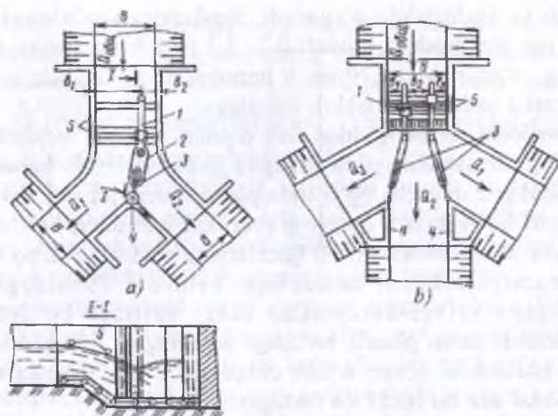
6.51-rasm. Yassi proporsional suv bo'lgichlar sxemalari:
