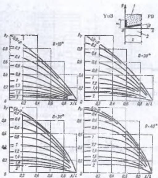
3.47-rasm. V turdagi tutashgan yon devor fragmenti sxemasi va tutashgan devor bo'ylab keltirilgan bosim h , ning x o'qiga nisbatan uning turli qiyalik burchaklari \theta da va shpora S li uzunliklarida aniqlash grafiklari: 1 – gruntli to'g'on; 2 – suv tashlash inshooti.
