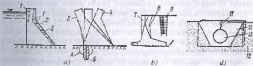
4.11-rasm. Ekspluatatsiya davrining harorat kuchlanishi va deformatsiyalari: a—to'g'onlardagi yoriqlar va to'g'onlar siljishi; b -tirgak devorning gruntga «yotishi»; d quvurli yig'ma rostlagichlar diafragmasidagi yoriqlar; 1-ochilgan choklar; 2-boshlang'ich hisobiy kesim; 3-choklar ochilishi inobatga olingan hisobiy kesim; 4,5-to'g'onning qish va yoz faslidagi holati; 6-sementli devor; 7-tirgak devor; 8-shuning o'zi yoz oylari old tomon isiganda; 9-devor «yotganda» passiv bosim; 10-quvur rostlagich diafragmasi; 11-yoriq; 12-muzlagan grunt; 13-quvurli rostlagich ostidagi teshik.
