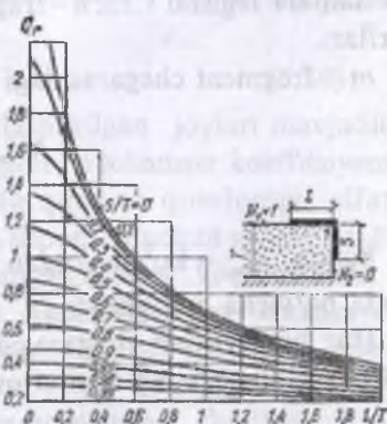
3.13-rasm. Tashqi fragment uchun keltirilgan sarf Q ni aniqlash grafigi.
