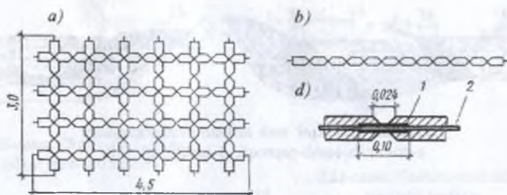
7.24-rasm. Egiluvchan temir-betonli panjaralar:
