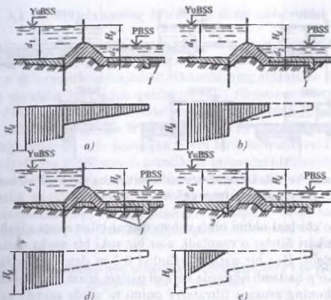
3.26-rasm. Inshoot yer osti konturida drenajlarni joylashtirish sxemalari:
