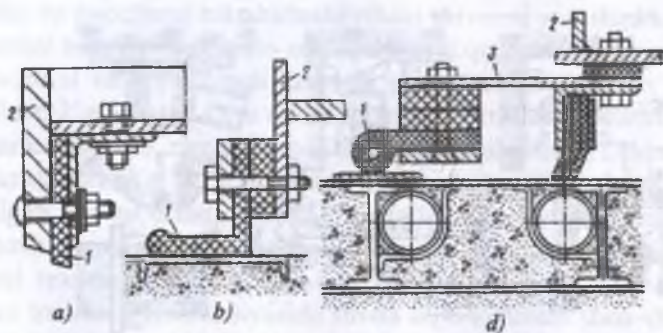
6.24-rasm. Segmentli zatvorlar zichlagichlari sxemalari: a–tubdagi; b,d–yon tomondagi; 1–zichlaydigan rezina elementi; 2–qoplama; 3–egiluvchan metall list.
