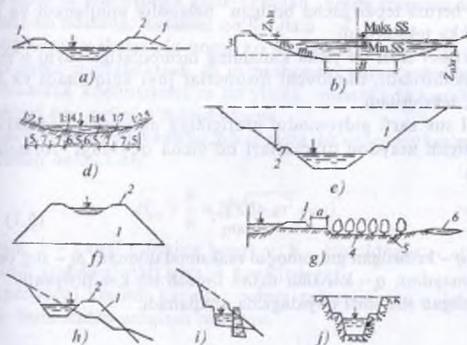
5.1-rasm. Kanallarining ko'ndalang kesimlari: a-yarim qazima-yarim ko'tarmali trapetseidal; b-polygonal; d-parabolik; e- chuqur qazimali; f-ko'tarmali; g-yo'l va rezerv joylashtirilgan; h,i-qiya tog' yon bag'irli; j-qoyali gruntlarda. 1-ko'tarma; 2-berma; 3-qoplama chegarasi; 4- daraxt ekilgan rezerv; 5-suv olib ketuvchi ariq; 6- inspektorlik yo'li.
