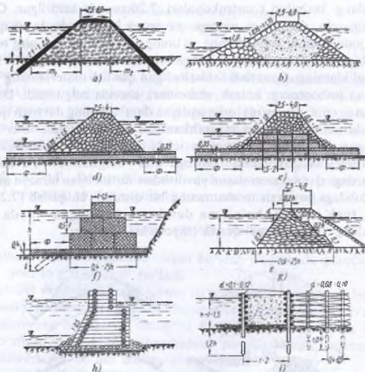
7.26-rasm. Oqimni yo'naltiruvchi dambalar ko'ndalang kesimlari konstruksiyalari: a-zarralari o'zaro birikkan gruntlardan qiyaliklari va tepasini mustahkamlash bilan; b-o'zaro birikmagan tosh tashlash bilan; d-yoyilgan shox-shabba to'shama tosh tashlash bilan; e-to'shama toshli; f-gabionli, g-qorishmasiz terilgan tosh; h-yog'och qutisimon; i-ikki qatorli chetan devorli traversa bilan.
