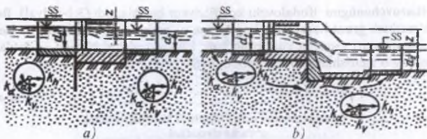
3.3-rasm. Suv dimlovchi inshootlardagi yuza va filtratsiya oqimlari sxemalari: a – bir jinsli-izotrop, gruntli zaminlarda yuza oqimlar; b – bir jinsli-anizotrop, gruntli zaminlarda yuza va filtratsiya oqimlari.
