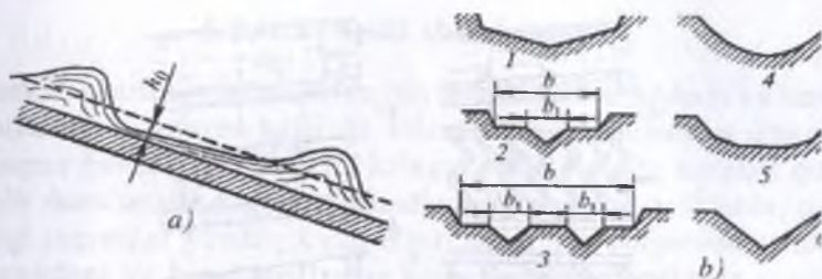
5.34-rasm. Tezoqardagi bo'ylama to'liqlar va to'liqqa qarshi ko'ndalang kesimlar: a - bo'ylama to'liqlar hosil bo'lish sxemasi; b - nov ko'ndalang kesimlari; 1 - yon tomonlari qiyalik koeffitsiyentlari o'zgaruvchan trapetsiya; 2 - tubida uchburchak qir qilgan kesimli trapetsiya; 3 - tubida ikkita uchburchak qir qilgan kesimli; 4 - parabolik; 5 - poligonal; 6 - uchburchakli.
