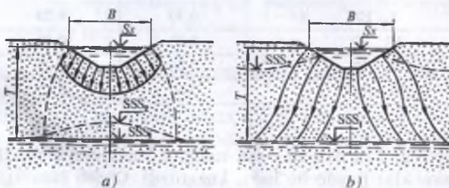
5.2-rasm. Kanallardagi filtratsiya suvlari sxemasi. a - erkin; b - erkin bo'lmagan.
