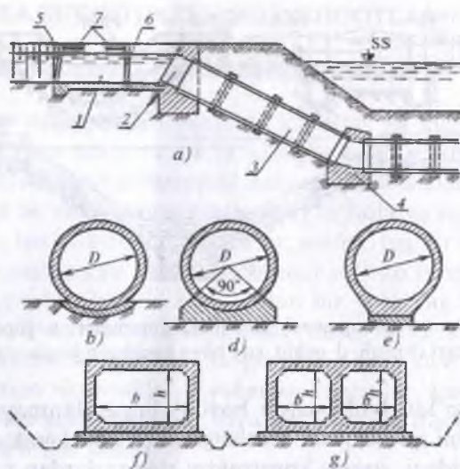
5.42-rasm. Kanal tagidan o'tkazilgan dyuker konstruksiyasi: a—bo'ylama qirg'iq; b,d,e—doiraviy quvurlar; f,g—mos ravishda bir va ko'p ko'zli quvurlar; 1—kirish qismi; 2—kirish kallagi; 3—bosimli quvur; 4—ankerli tayanch; 5—panjara; 6—zatvor; 7—xizmat ko'p rigi.
