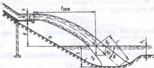
5.40-rasm. Konsolli sharshara gidravlik hisobi sxemasi.
