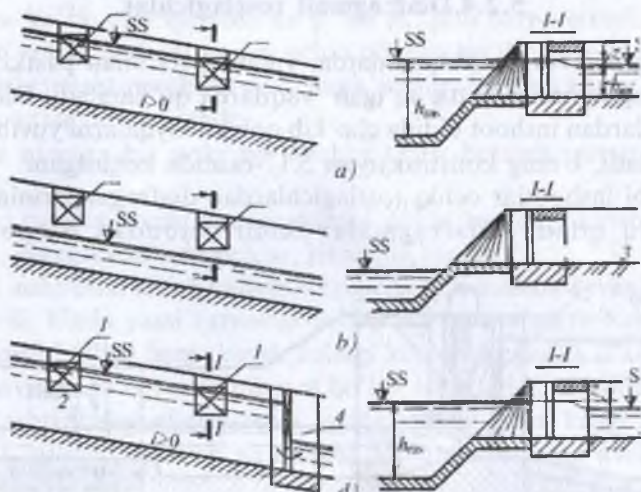
5.18- rasm. Dimlovchi inshoot o'rnatilganda kanalning ishlash rejimi:
