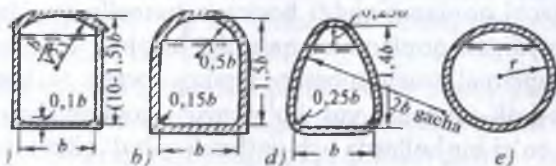
5.54-rasm. Bosimsiz tunnel ko'ndalang kesimlari: a-to'g'ri burchakli gumbazli; b-to'g'ri burchakli radial gumbazli; d-pastki tomonga kengiyadigan; e-doiraviy.
