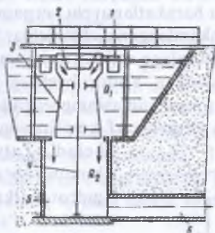
6.49-rasm. Suv bilan o'zaro ta'sir etuvchi zatvor-avtomat sxemasi:
