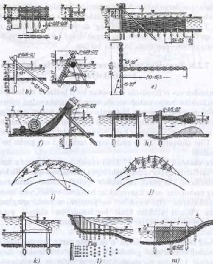
7.30-rasm. Tanasidan suv o'tkazuvchi inshootlar turlari va konstruksiyalari: a) tirgaksiz bir qatorli chetan devor; b) tirgaklari orasidagi masofa 1,5...2,5 m li bir qatorli chetan devor; d) senoyali chetan devorli shit, 1,5...2 m masofada o'rnatilgan; e) T-shakldagi I.A.Shadrin chetan devor tizimi; d-to'rt oyoqda o'rnatilgan og'ir fashina yuklangan supurgisimon shitlar; g) qoziqlarga ilingan fashinali shitlar; h,i,j) bo'ylama va ko'ndalang shox-shabbali inshootlar; k) qoziqlarga o'rnatilgan taxtali devorli inshootlar; l) qoziqli poluzaprudalar; m) qoziqlarga o'rnatilgan simdan to'qilgan statsionar inshoot; 1- yuk; 2- sim chiviqli arqon; 3- og'ir fashina; 4- qirg'oqni mustahkamlash.
