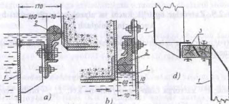
6.18-rasm. Chuqur va ikki qatorli joylashgan zatvor zichlagichlari turlari: 1– zatvor qoplamasi; 2–profil rezina; 3–yog'och bruslar.
