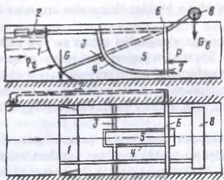
6.46-rasm. Suv bilan o'zaro ta'sir etuvchi korrektorli segmentli zatvor-avtomat sxemasi: 1-zatvor; 2-galercya; 3-tayanch to'sini; 4-korrektor kamerasi; 5-korrektor; 6-zatvor o'qi; 7-quyilish joyi; 8-muvozanat yuki.
