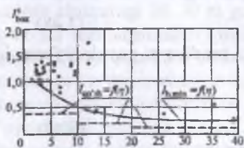
3.28-rasm. J_{buz}^s = f(\eta) . bog'lanish grafigi.
