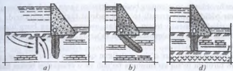
3.32-rasm. Kimyoviy suffoziyani bartaraf etish tadbirlari sxemalari:
