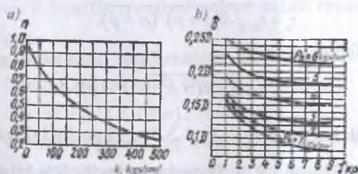
5.58-rasm. Bosimli tunnel qoplamasi qalinligini dastlabki aniqlash grafigi.
