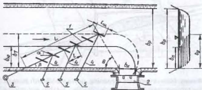
7.9-rasm. To'g'onsiz suv olishda oqimni yo'naltiruvchi tizimini joylashtirish:
