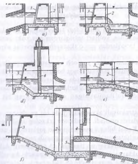
5.43-rasm. Dyuker kirish va chiqish qismlarining konstruksiyalari: b,d,e,f – kirish qismi; a–chiqish qismi; 1 – spitsalar; 2–shandorlar uchun paz; 3–panjara; 4–zatvor; 5–chuqur joylashgan zatvor; 6–tezoqar; 7–dyuker.
