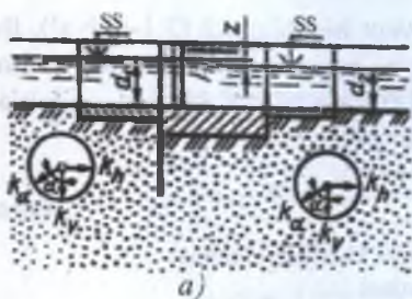
3.3-rasm. Suv dimlovchi inshe oqimlari sxemalari: a – bir jinsli-izotrop b – bir jinsli-anizotrop, gruntli zamin
