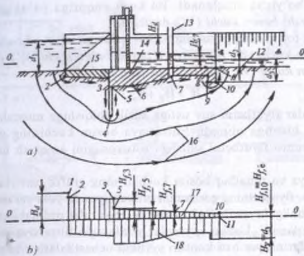
3.24 - rasm. Suv dimlovchi inshoot yer osti konturiga filtratsiya oqimi kuchi ta'siri sxemasi: a -- suv dimlovchi inshoot kesimi; b -- flyutbet gorizontaal proyeksiyasidagi bosim epyuralari; 1 - 11-flyutbet yer osti chiziqlari bo'yicha filtratsiya oqimining aylanib o'tishi; 12 - risberma; 13 - pezometr; 14 - suv urilma; 15 - ponur; 16 - grunt suvlarining tok chiziqlari; 17, 18 - flyutbet gorizontaal proektsiyasidagi muallaq va filtratsiyaga qarshi bosimi epyuralari.
