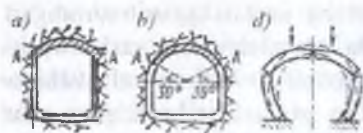
5.57-rasm. Bosimsiz tunnelning qoplamasini hisobiy sxemasi.
