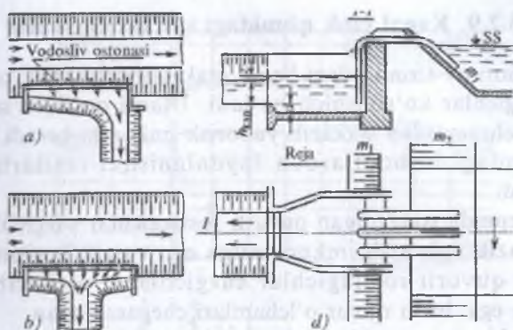
5.23-rasm. Avariya holatidagi suv tashlagichlari: a,b – yon tomonli va polygonal vodoslivli; d – sifonli.
