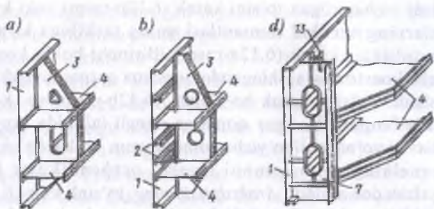
6.13-rasm. Yassi zatvor oraliq tuzilmasi elementlari: (ko'rinish 6.12-rasmga qarang).
