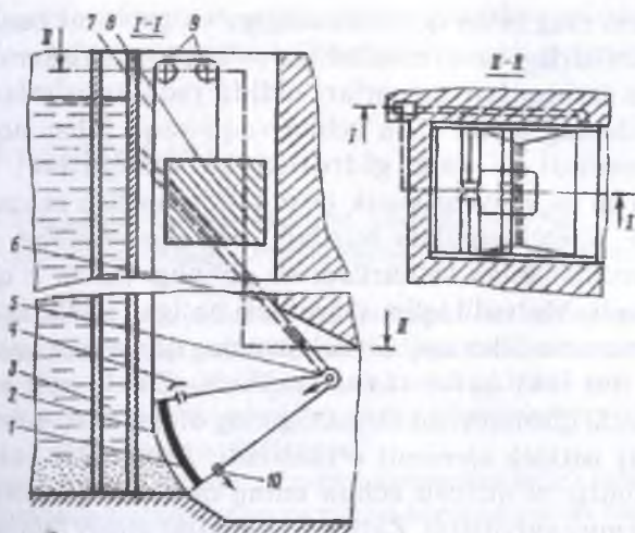
6.52-rasm. Muvozanatlashgan sektorli zatvor-avtomat sxemasi:
