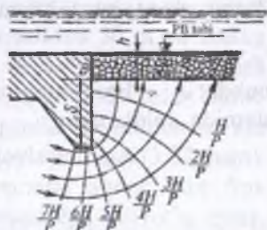
3.29-rasm. Bo'rtib chiqish hisobi sxemasi.
