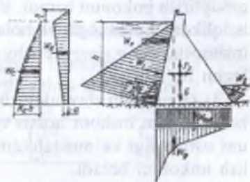
4.1-rasm. To'g'onga ta'sir etuvchi kuchlar sxemasi.
