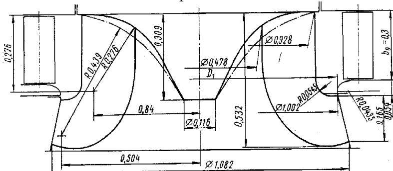
3-rasm. RO75/702 gidroturbinaning ishchi g'ildiragini suv o'tkazuvchi qismi D_1 ni ulishida
