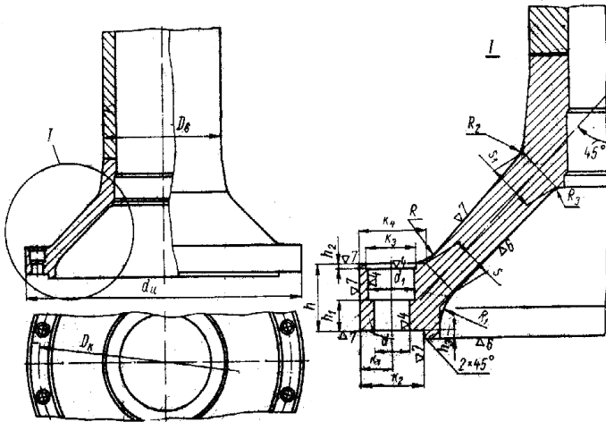
5 – rasm. Ishchi g‘idirak qopqog‘i bilan biriktirilgan buram-kurakli turbinavi
