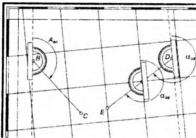
6.7–shaki. Kartadagi yo'nalishning haqiqiy azimuti va direktsion burchagini aniqlash sxemasi
