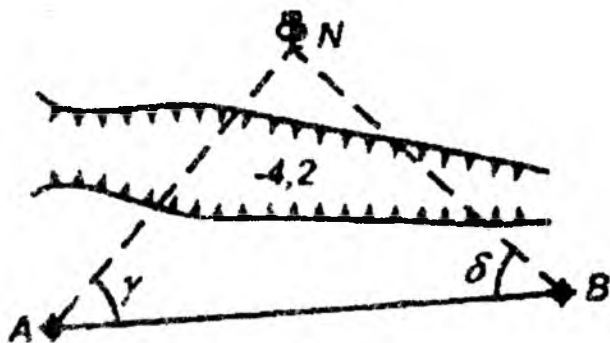
13.7-shakl. Burchakli kesishtirish usulida s'yomka sxemasi
