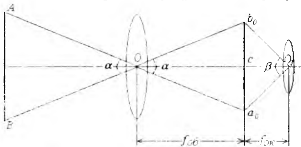
9.9-shakl. Ko'rish trubasining kattalashtirishini aniqlash sxemasi
