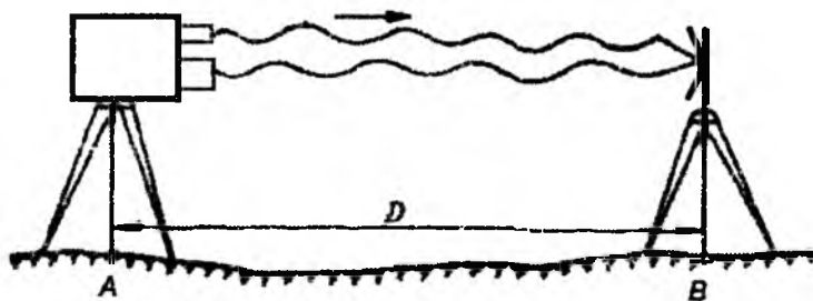
10.13-shakl. Elektron dalnomerlar yordamida masofa o'lchash sxemasi
