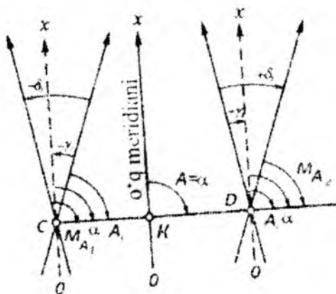
4.3-shakl. Yo'nalish orientirlash burchaklari orasidagi bog'lanish
