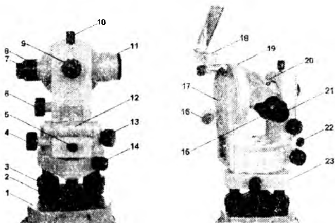
9.3-shakl. 4T30N optik teodolitning tuzilish qismlari
