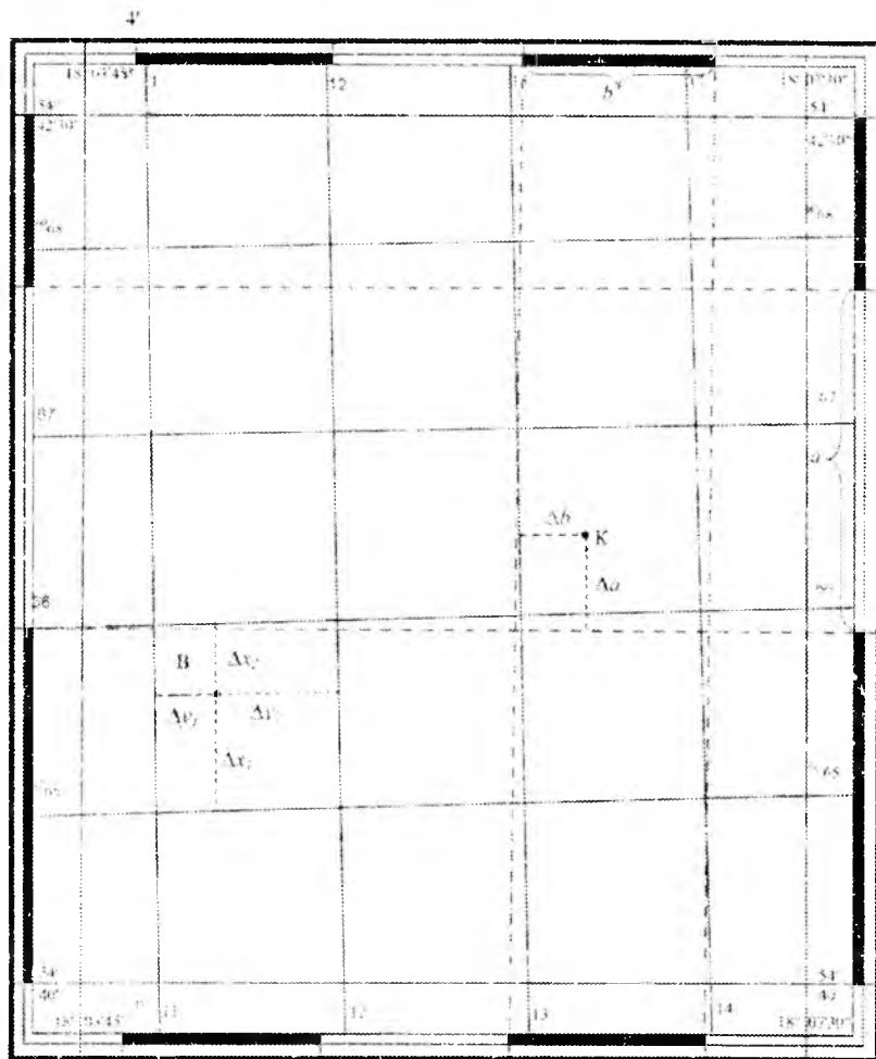
6.2- shakl. Topografik kartalarning matematik elementlari
