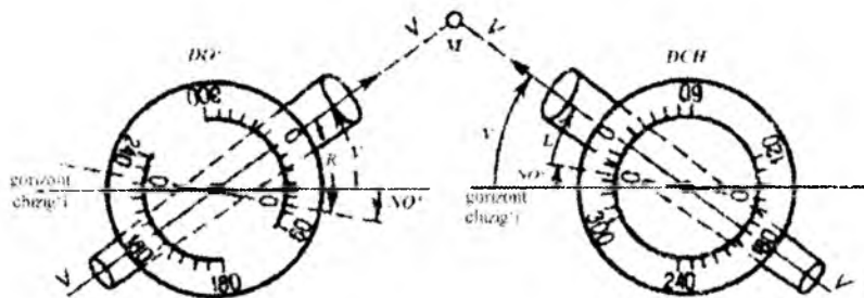
9.5-shakl. Vertikal doirada qiyalik burchagini o'lchash sxemasi ko'rsatilgan.
