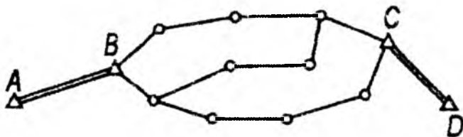
13.9-shakl. Teodolit yo'lini o'tkazish orqali tayanch to'r yaratish sxemasi
