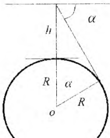
1.2-shakl. Beruniyning yer shari kattaligini aniqlash sxemasi
