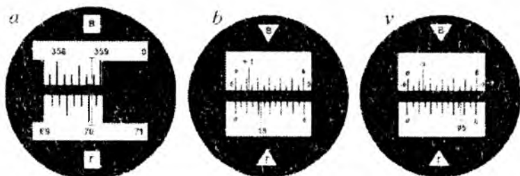
9.4-shakl. Sanoq olish mikroskopining ko'rish maydoni:
