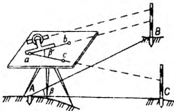
13.6-shakl. Menzula va kiprigel yordamida gorizontal burchakni chizmaga tushirish.
