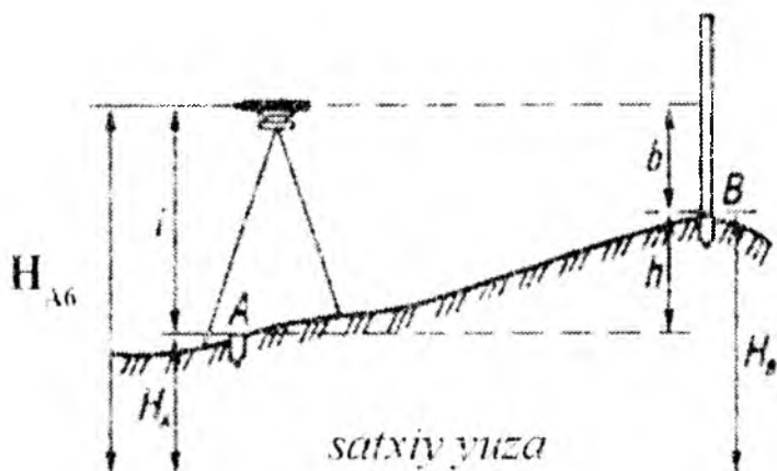
11.1-shakl. Oldinga nivelirlash sxemasi
