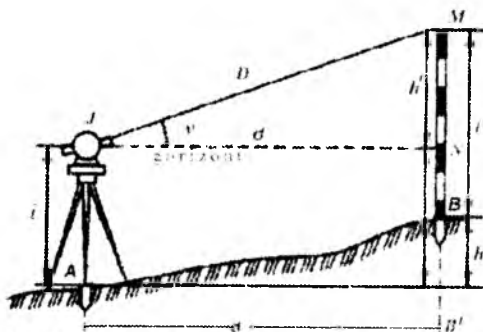
11.16- shakl. Trigonometrik nivelirlash sxemasi
