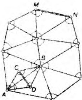
12.1-shakl. Triangulyatsiya to'rining ko'rinishi
