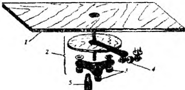
13.7-shakl. Menzula plansheti.
