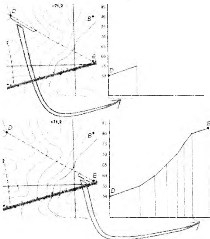
6.10-shakl. Kartada profil tuzish
