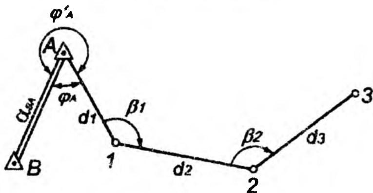
13.3-shakl. Osmu teodolit yo'li
