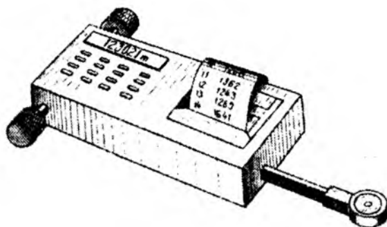
8.4-shakl. PLANIX-7 raqamli planimetrini ko'rinishi
