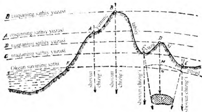
2.1-shakl. Yer sirtidagi nuqtalardan o'tkazilgan sathiy yuzalar va geoid sxemasi
