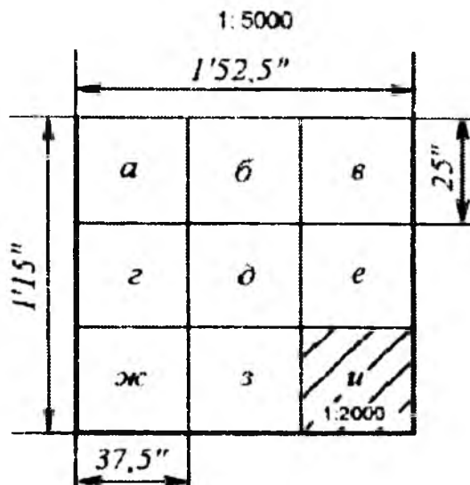
5.7- shakl. 1:5000 masshtabli plandan 1:2000 masshtabdagi plan varaqlarini olish sxemasi
