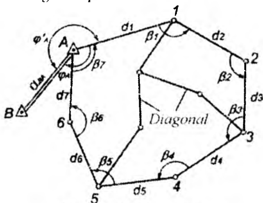
13.2 -shakl. Tutash teodolit yo'li
