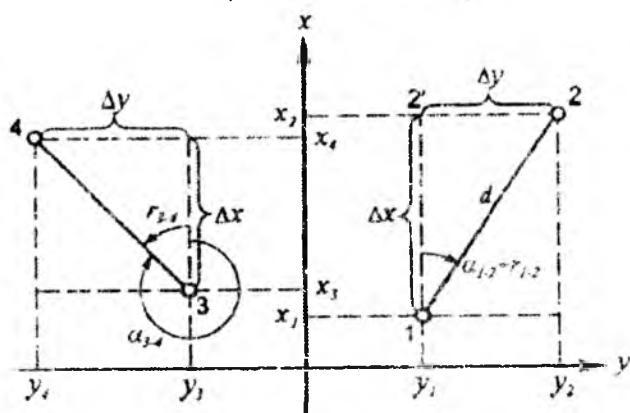
4.6-shakl. To'g'ri va teskari geodezik masalalar.
