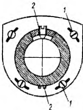
11.13-shakl. Kompesatorli nivelirning okulyarini tozilish sxemasi:
