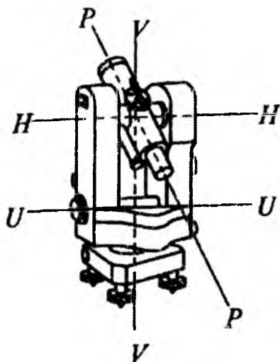
9.13 – shakl. Teodolit geometrik o‘qlarining sxemasi
