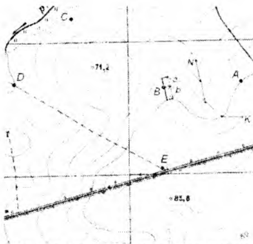
6.9-shakl. Kartadagi nuqtalar o'tmetkalarini gorizontallar yordamida aniqlash
