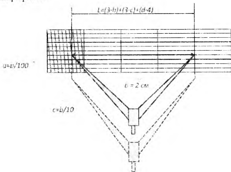
5.2-shakl. Ko'ndalang masshtabda masofa aniqlash
