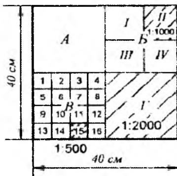
5.8 shakl. 1:5000 masshtabli plandan 1:2000, 1:1000 va 1:500 masshtabdagi plan varaqlarini olish sxemasi
