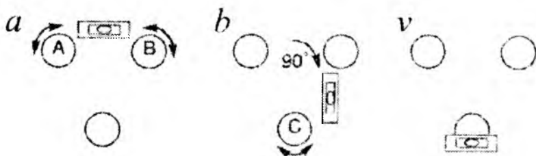
9.14-shakl. Teodolitning silindrik adalaki bilan ishlash sxemasi
