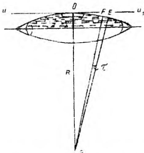
9.11-shakl. Adilak bo'lak qiymatini aniqlash sxemasi
