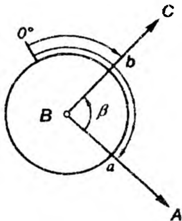
9.17– shakl. Gorizontaal burchakni priyomlar usulida oʻlchash sxemasi
