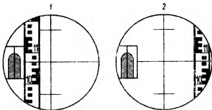
11.11-shakl. Nivelir aylanish o'qiga iplar to'rining gorizontall ipi esa perpendikulyar bo'lish shartini tekshirish sxemasi
