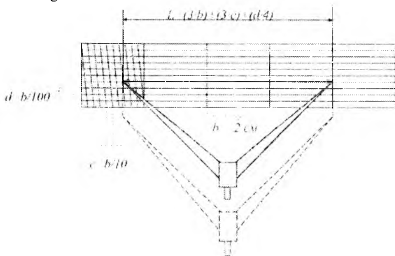
6.4-shakl. Ko'ndalang masshtabda masofa aniqlash
