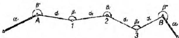
12.2-shakl. Poligonometriya to'rini ko'rinishi
