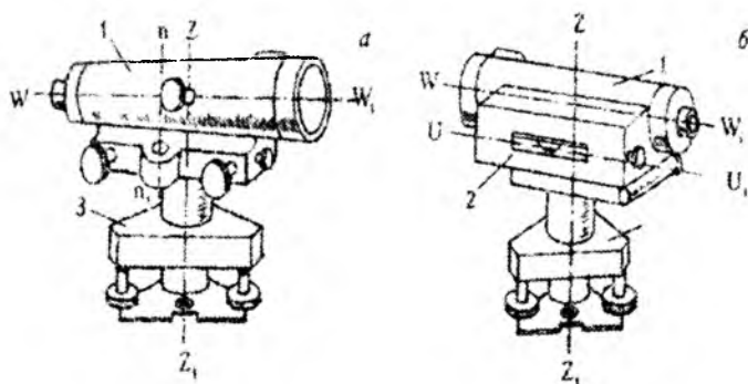
11.9-shakl. Optik nivelirning tuzilishi va geometrik o'qlari:
