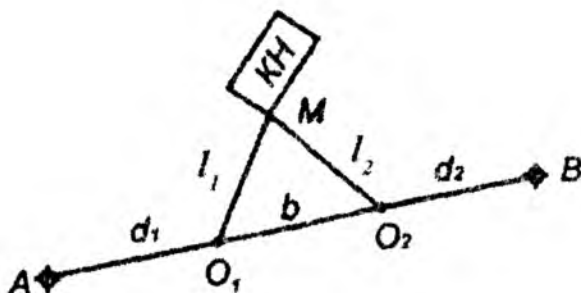
13.6-shakl. Chiziqli kesishtirish usulida s'yomka sxemasi
