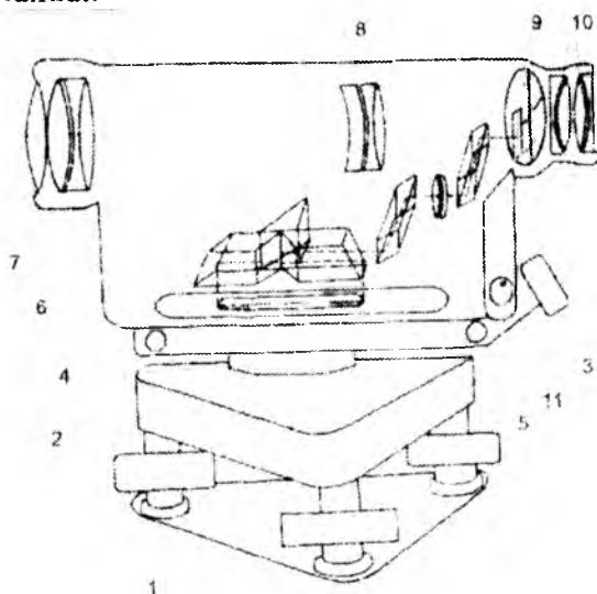
11.5-shakl. H3 nivelirini optik sxemasi:
