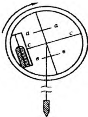
11.10-shakl. Nivelir aylanish o'qiga iplar to'rining vertikal ipi parallel bo'lish shartini tekshirish sxemasi
