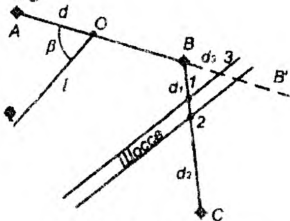
13.8-shakl. Stvor usulida s'yomka sxemasi
