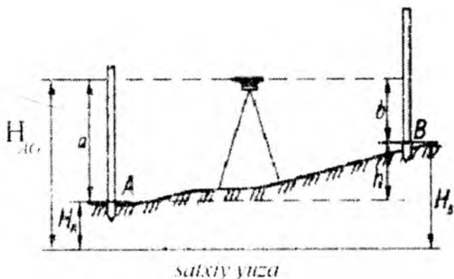
11.2-shakl. O'rtadan nivelirlash sxemasi. sxemasi
