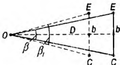
10.7-shakl. O'zgarmas bazisli dalnomer sxemasi
