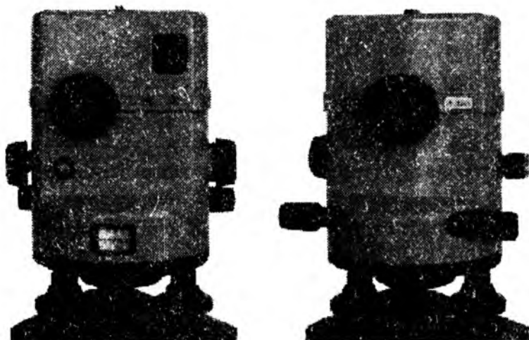
11.7-shakl. Kompensator va limbli 3H3KJ aniq nivelirining ko'rinishi 1 – limb; 2 – yo'naltirish vinti; 3 – kremalera; 4 – vizir
