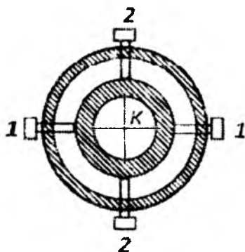
9.7-shakl. Iplar to'r halqasini o'rnatish sxemasi
