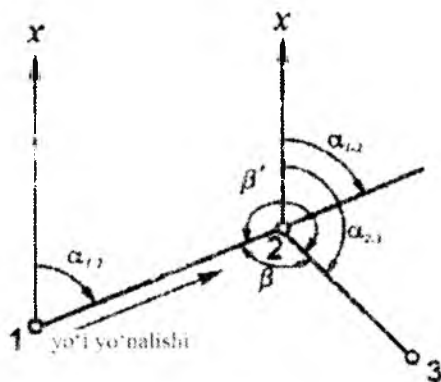
4.5-shakl. Direktsion burchak va gorizontal burchak orasidagi bog'lanish sxemasi
