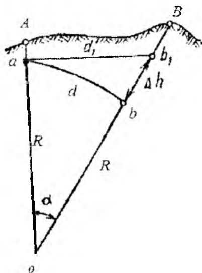
2.5-shakl. Yer sirti egriligini gorizontal va vertikal masofaga ta'siri
