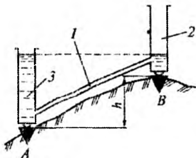
7.18-shakl. Gidrostatik nivelirlash sxemasi:
