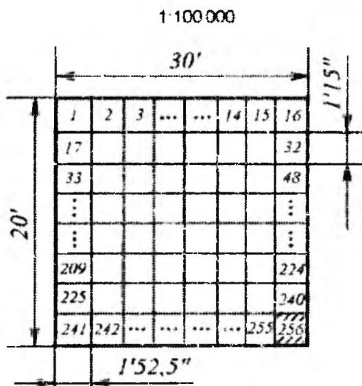
5.6-shakl. 1:100000 masshtabli kartadan 1:5000 masshtabdagi plan varaqlarini olish sxemasi
