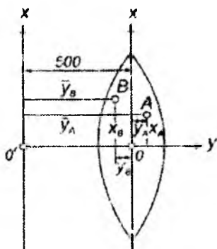
3.7-shakl. Zona koordinata boshini shartli ravishda 500 km g'arbga surilish sxemasi
