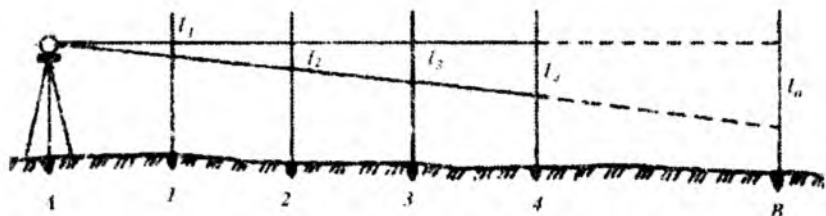
10.10-shakl. Dalnomer koefitsientini aniqlash sxemasi
