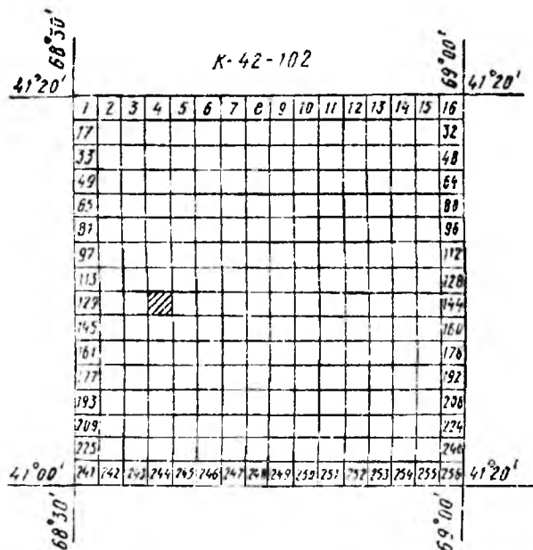
5.4-shakl. 1:1000000 masshtabli karta varag'ini bo'lish orqali 1:100 000 masshtabli karta varaqlarini olish sxemasi
