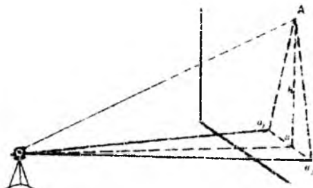
9.15-shakl. Ko'rish trubasining gorizontaal aylanish o'qini teodolit vertikal o'qiga perpendikulyarligini tekshirish sxemasi
