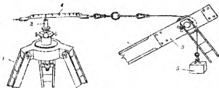
10.4-shakl. Invar sim bilan masofa o'lchash:
