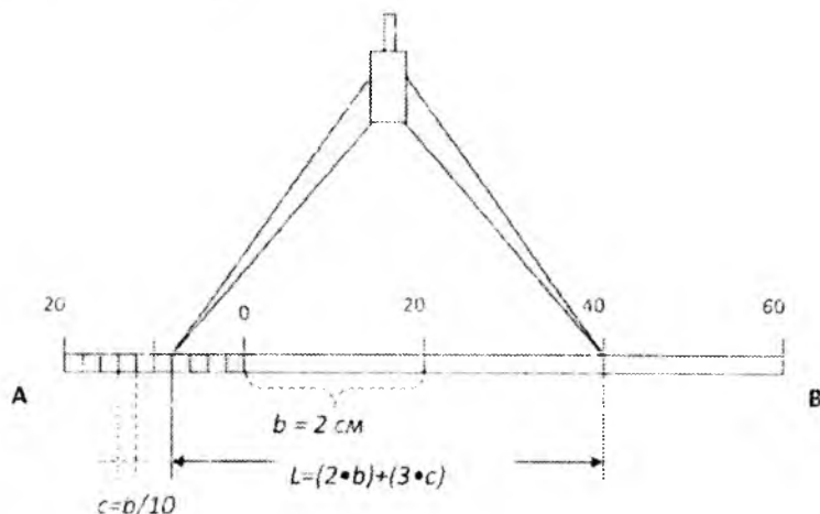
6.3-shakl. Oddiy chiziqli masshtabda masofa aniqlash
