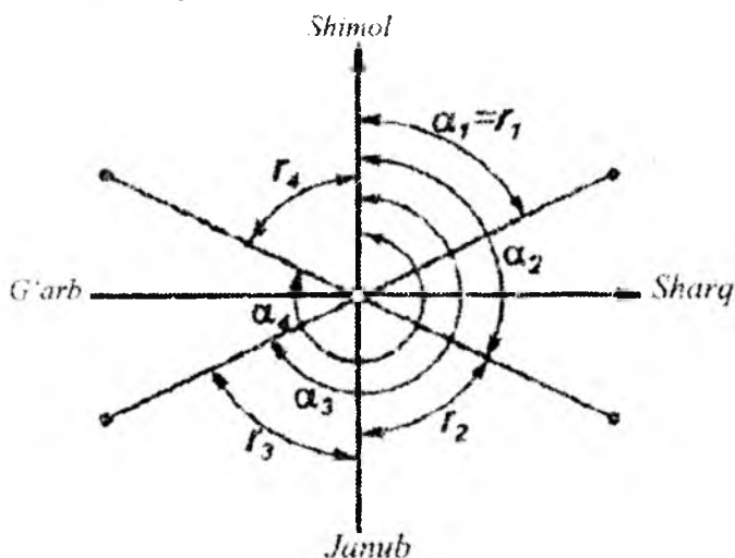
4.4. shakl. Rumblar va direksion burchaklar orasidagi munosabat sxemasi
