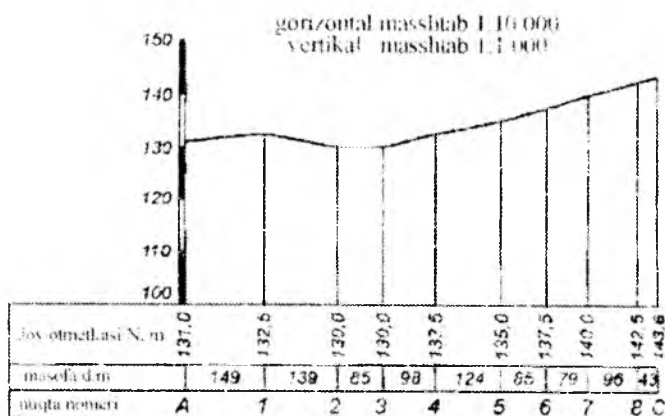
6.11-shakl. AC yo'nalish bo'yicha profil
