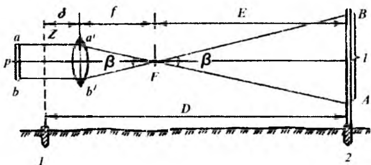
10.8-shakl. Ipili dalnomer bilan masofa o'lchash sxemasi
