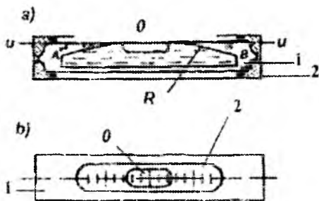
9.10-shakl. TSilindrik adilak:
