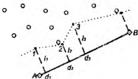
13.5 – shakl. Perpendikulyar usulida s'vodka sxemasi
