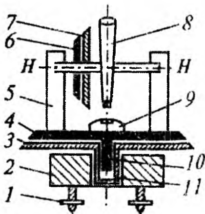
9.2 -shakl. Teodolitni umumiy tuzilish sxemasi:
