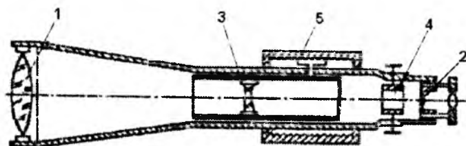
9.6-shakl. Qarash trubasini bo'ylama qirgimi:
