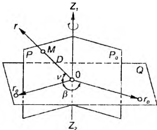
3.3. shakl. Fazoviy qutbiy koordinata tizimi sxemasi
