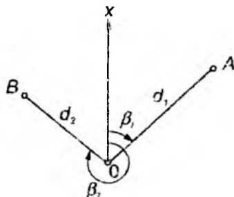
3.8-shakl. Qutbiy koordinata tizimi sxemasi
