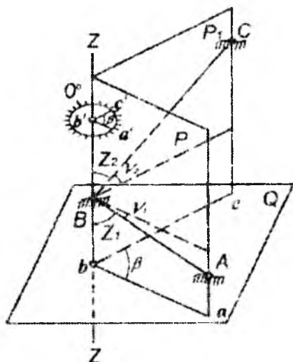
9.1-shakl. Joyda burchak o'lchash sxemasi.
