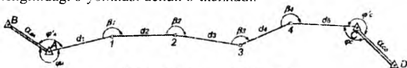
13.1-shakl. Notutash teodolit yo'li
