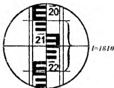
10.9-shakl. Ipli dalnomerda reykanan sanoq olish bilan masofa o'lchash
