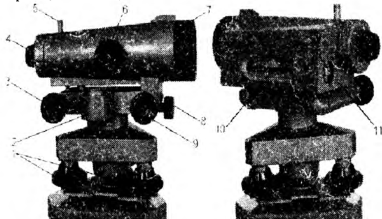
11.4-shakl. Ko'rish trubasida slindrik adilagi bor H3 nivelirining ko'rinishi:
