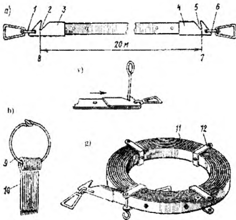
10.1- shakl. Po'lat lenta: a-po'lat lentani umumiy ko'rinishi, b-po'lat lenta shpilkalari; v-lenta boshini shpilka bilan belgilash; g-lenta o'rami.
