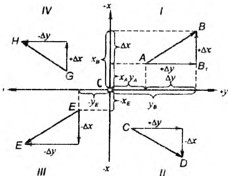
3.4-shakl. Geodezik to'g'ri burchakli yassi koordinata tizimi
