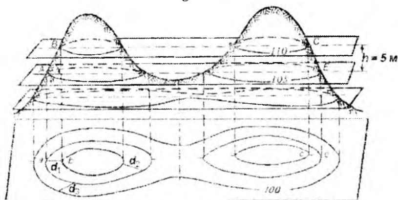
5.11-shakl. Gorizontallarni hosil bo'lishi
