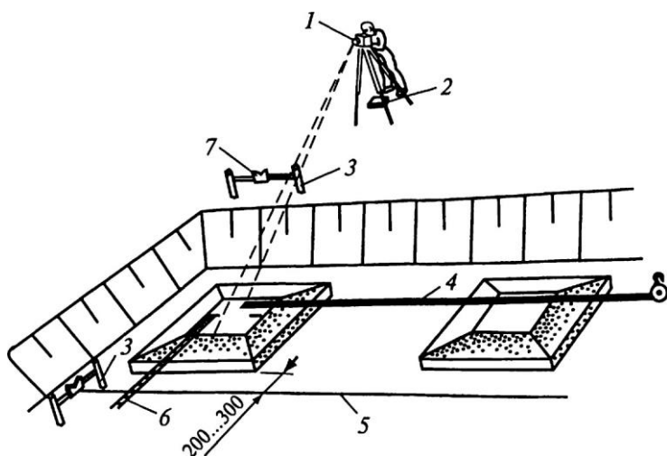
Рис. 20.6. Перенесение осей на фундаментные блоки:
