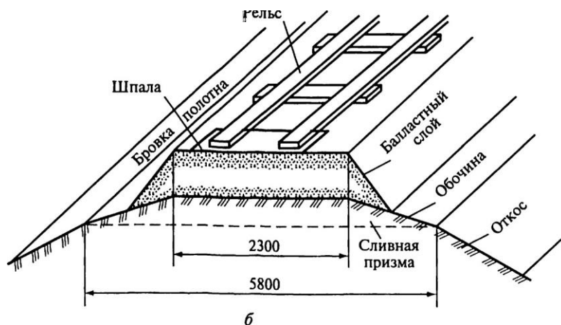
Рис. 25.11. Строение дорожного полотна: а — автодороги; б — железной дороги
