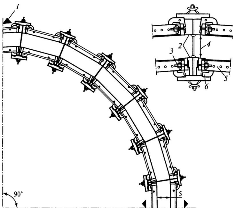
Рис. 20.24. Разметка для установки круговой опалубки:
