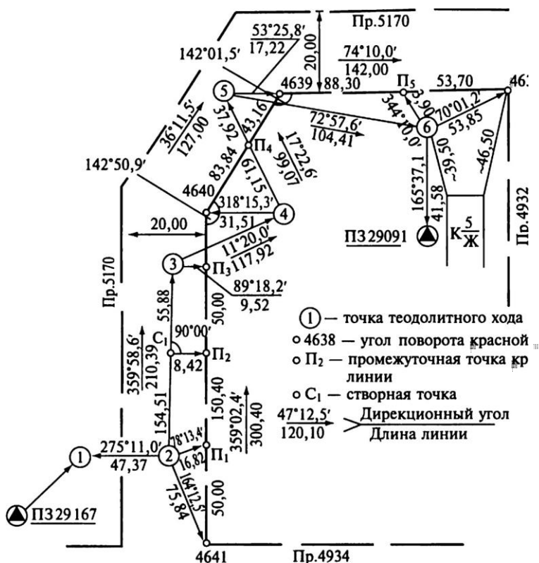
Рис. 18.1. Разбивочный чертеж красных линий
