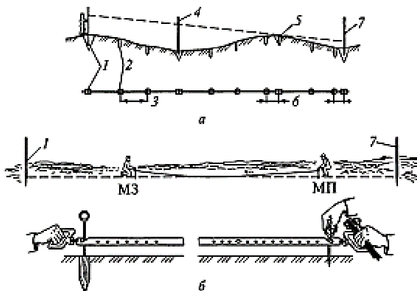
Рис. 6.5. Вешение линии:
