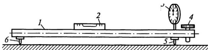
Рис. 22.6. Конструктивная схема микронивелира: 1 — подставка; 2 — цилиндрический уровень; 3 — часовой индикатор; 4 — подъемный винт; 5 — подвижная опора; 6 — неподвижная опора
