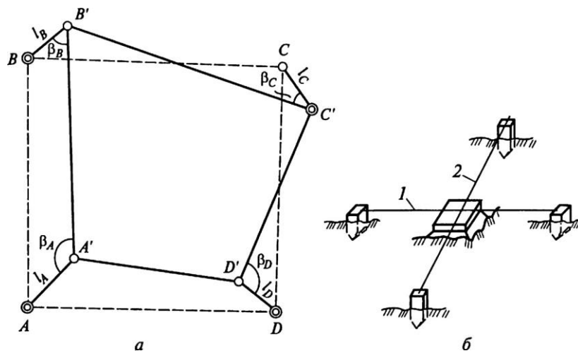
Рис. 13.7. Редуцирование пунктов строительной сетки:
