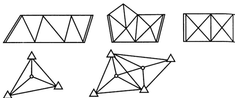
Рис. 13.1. Инженерно-геодезические сети триангуляции
