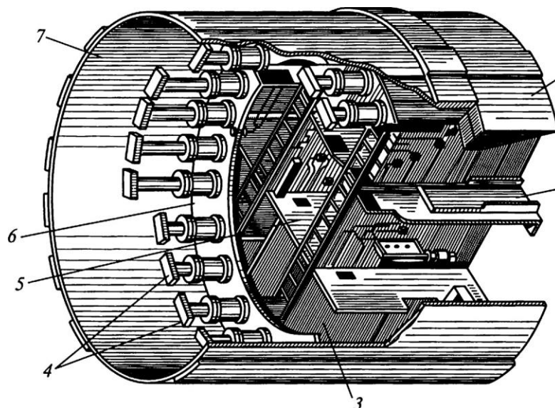
1 2 Рис. 27.2. Схема проходческого щита: 1 – нож; 2 — выдвижная платформа; 3, 5 — вертикальная и горизонтальная перегородки; 4 —
