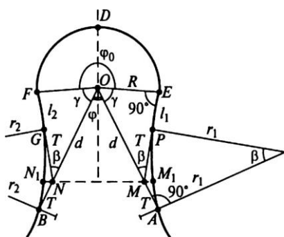
Рис. 25.10. Симметричная серпантина
