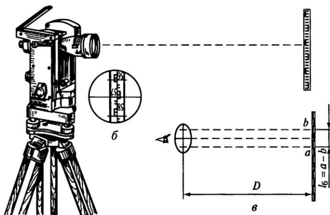
Рис. 6.8. Оптический дальномер:
