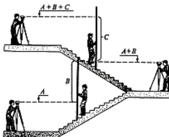
Рис. 7.10. Использование нивелира для переноса отметок на строительстве З Мнхслев
