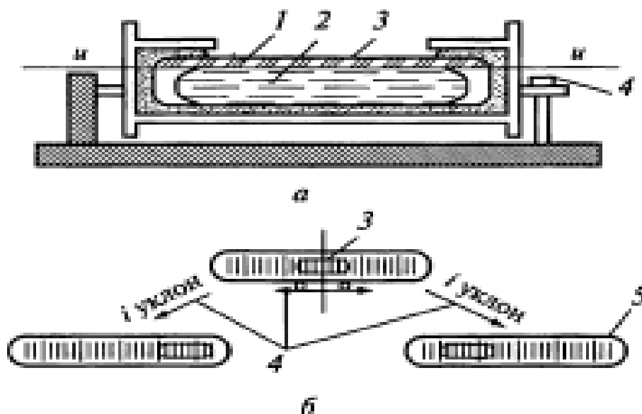
Рис. 7.2. Цилиндрический уровень и уклоны при положении пузырька: а — вид сбоку; б — вид сверху; 1 — ампула; 2 — жидкость; 3 — пузырек; 4 — исправительный винт; 5 — уклон ампулы
