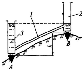
Рис. 7.13. Схема гидростатического нивелирования: 1-соединительный шланг; 2, 3 — сосуды
