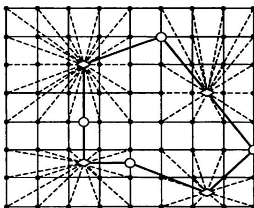
Рис. 7.11. Схема нивелирования по квадратам:
