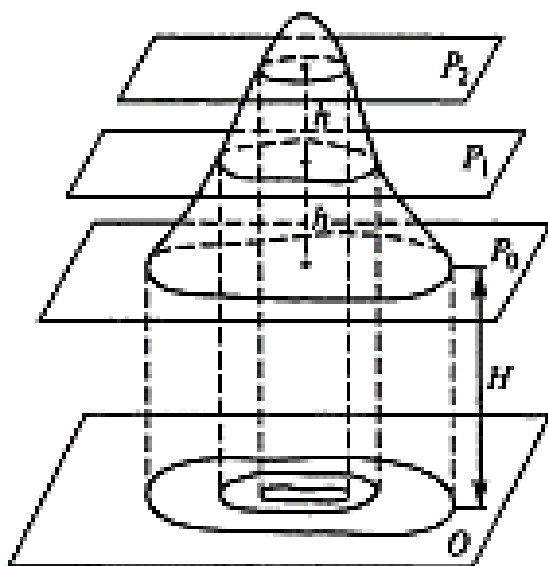
Рис. 4.2. Изображение рельефа горизонталями
