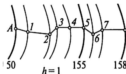
Рис. 4.9. Схема проведения на карте линии заданного предельного уклона
