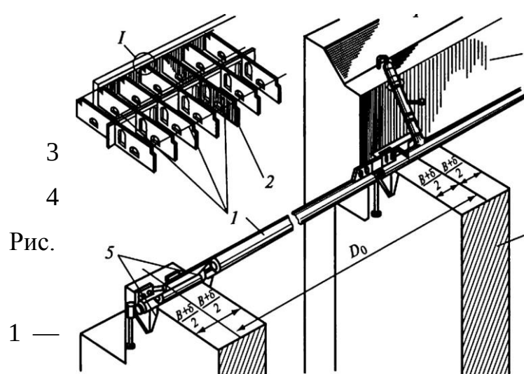
20.16. Групповое монтажное оснащение:
