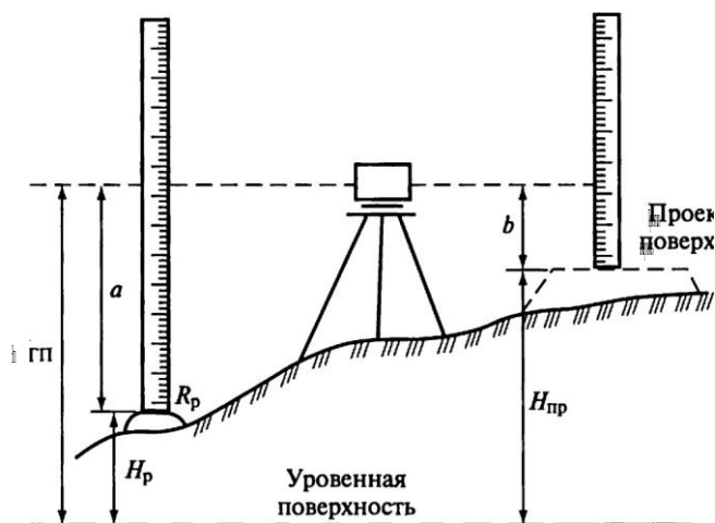
Рис. 15.4. Схема выноса в натуру проектной отметки
