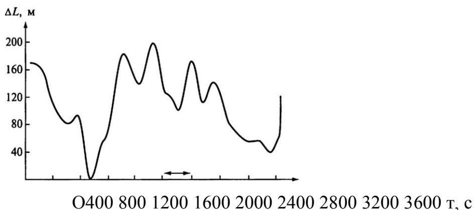
Рис. 14.16. Влияние искажения сигналов
