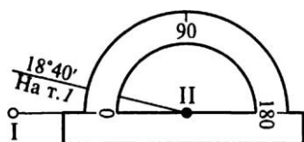
Рис. II.4. Построение направлений на пикеты со станции тахеометрического хода
