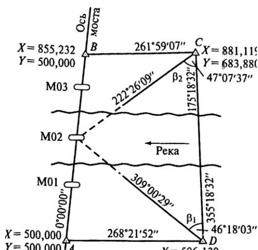
Рис. 25.16. Схема
