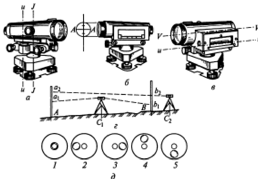
Рис. 7.14. Поверка нивелира:
