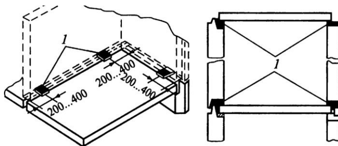
Рис. 20.13. Выравнивание монтажного горизонта:
