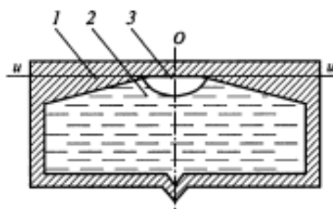
Рис. 7.3. Круглый уровень:
