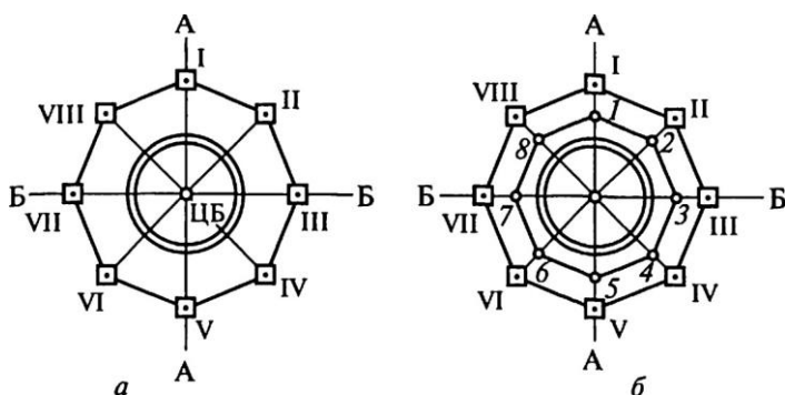
Рис. 21.7. Схемы опорной сети для строительства башенных сооружений: а — равномерное расположение пунктов на одной окружности; б — concentрическое расположение пунктов; 1...8 — ближние пункты; I...VIII — дальние пункты
