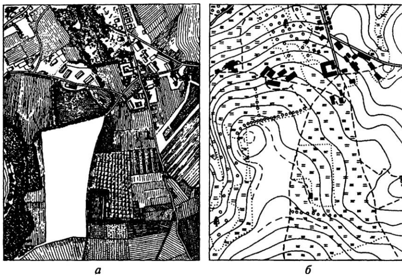
11.6. Аэрофотографическое изображение местности (а) и составленный по нему план (б)
