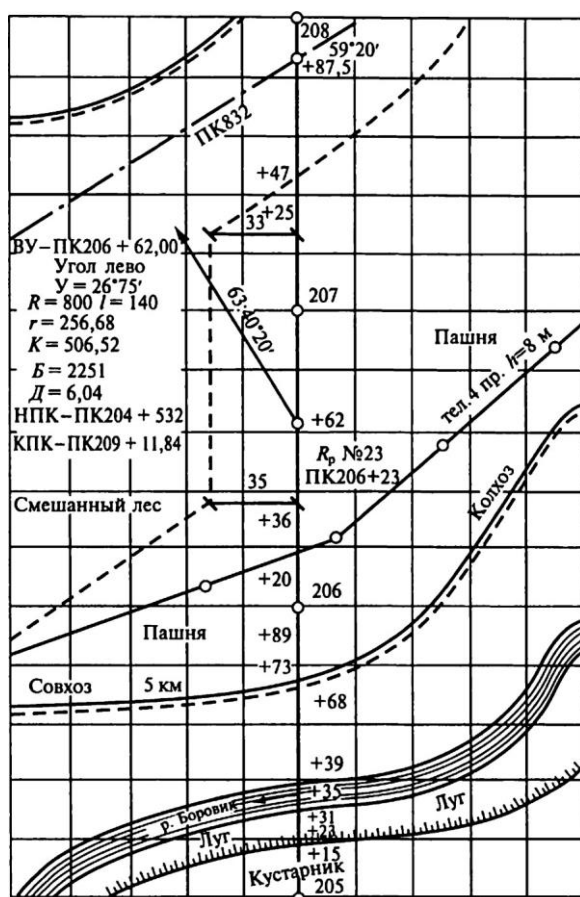
Рис. 25.6. Пикетажный журнал (условный пример)
