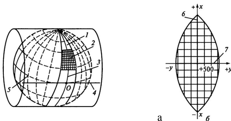
Рис. 3.3. Равноугольное проецирование:
