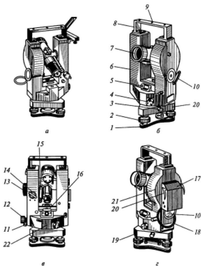
Рис. 8.3. Теодолит ЗТ5КП в рабочем состоянии:
