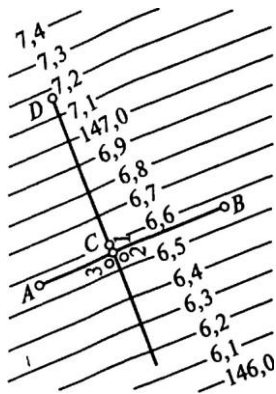
Рис. 18.7. Схема переноса в натуру плоскости проектного рельефа:
