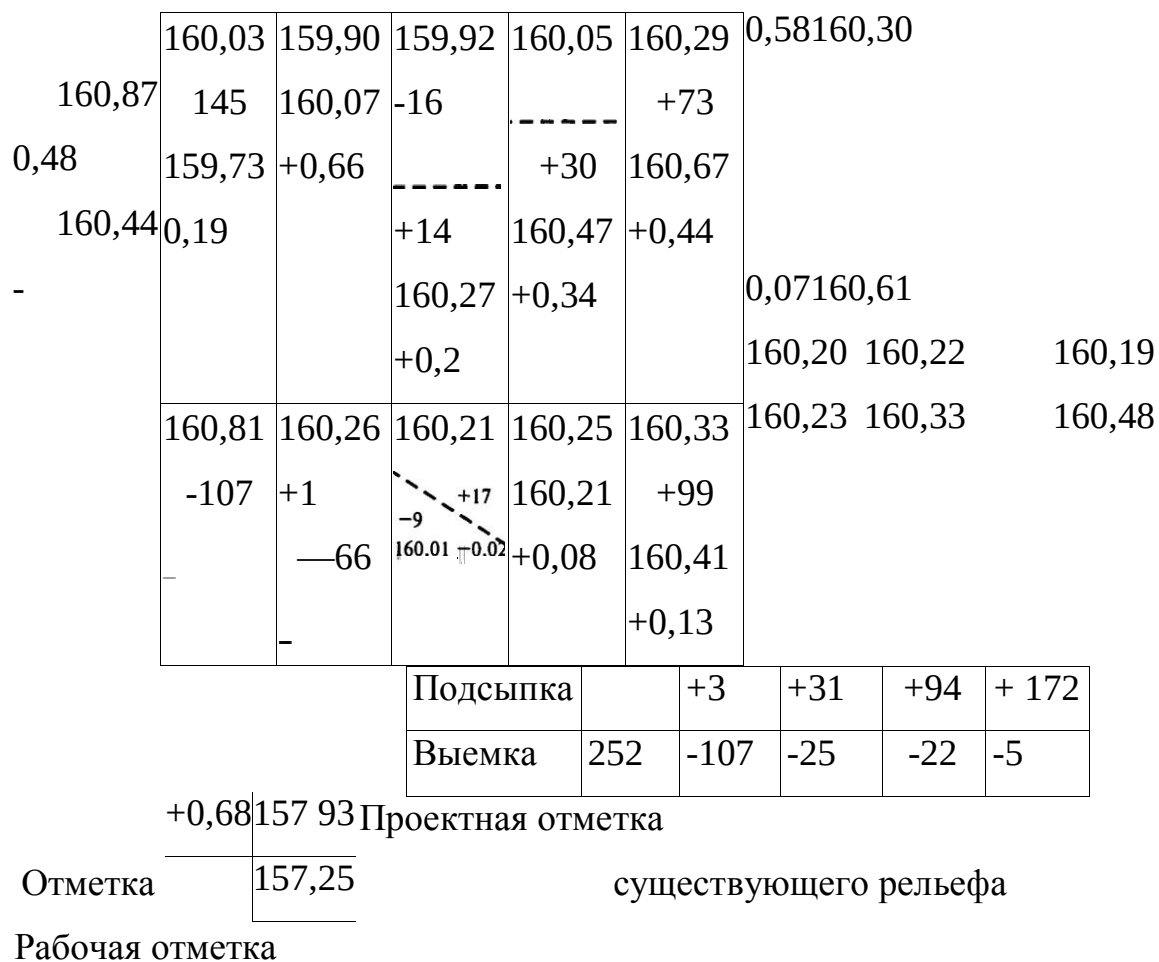
Рис. 18.6. План земляных масс с таблицей баланса
