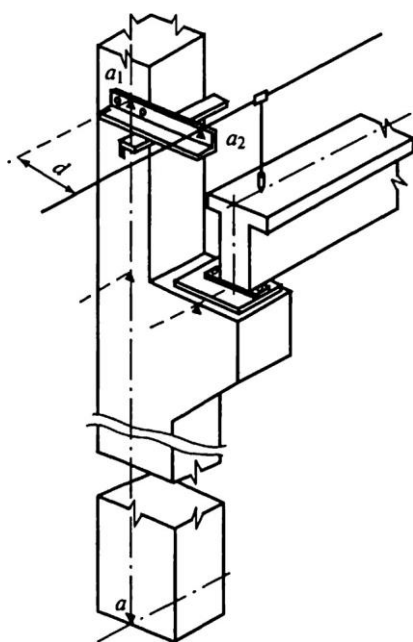
Рис. 21 А. Схема установки в проектное положение подкрановых балок 0,001 Н — при высоте, большей 15 м. Отклонение опорной поверхности колонн по высоте допускается 5 мм.
