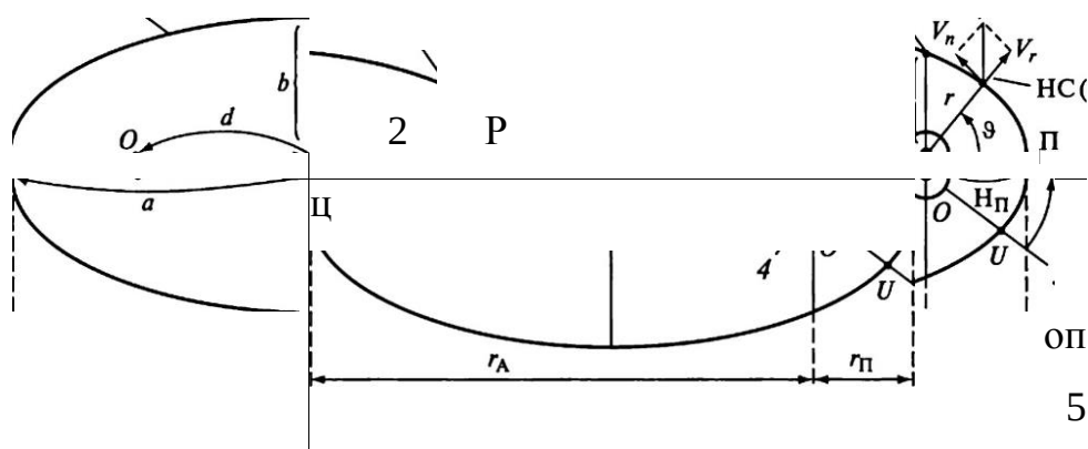
Рис. 14.11. Эллиптическая орбита спутника:
