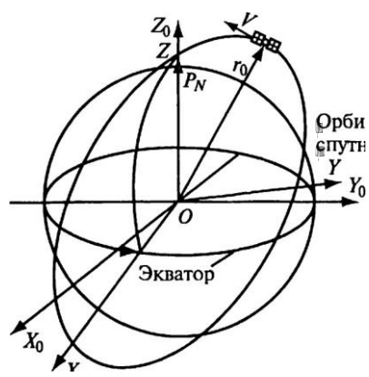
Рис. 14.9. Геоцентрическая инерциальная система координат
