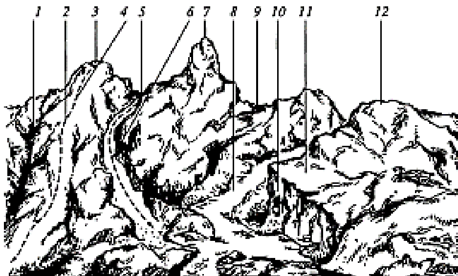
Рис. 4.1. Характерные формы рельефа:
