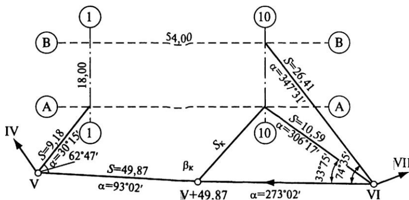
Рис. 17.2. Схема разбивки основных осей здания с точек полигометрических или теодолитных ходов
