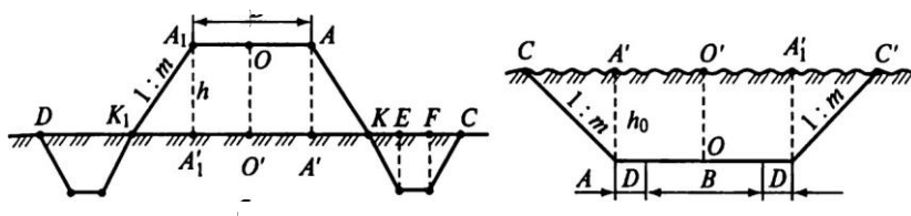
Рис. 25.12. Схемы разбивки дорожного полотна:
