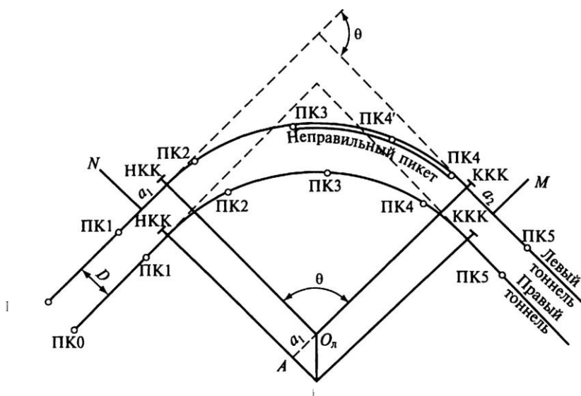
Рис. 27.4. Схемы расположения пунктов на кривых двухпутного тоннеля:
