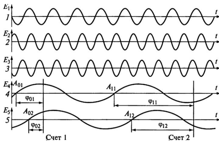
Рис. 14.13. Принцип фазовых измерений в двух каналах:
