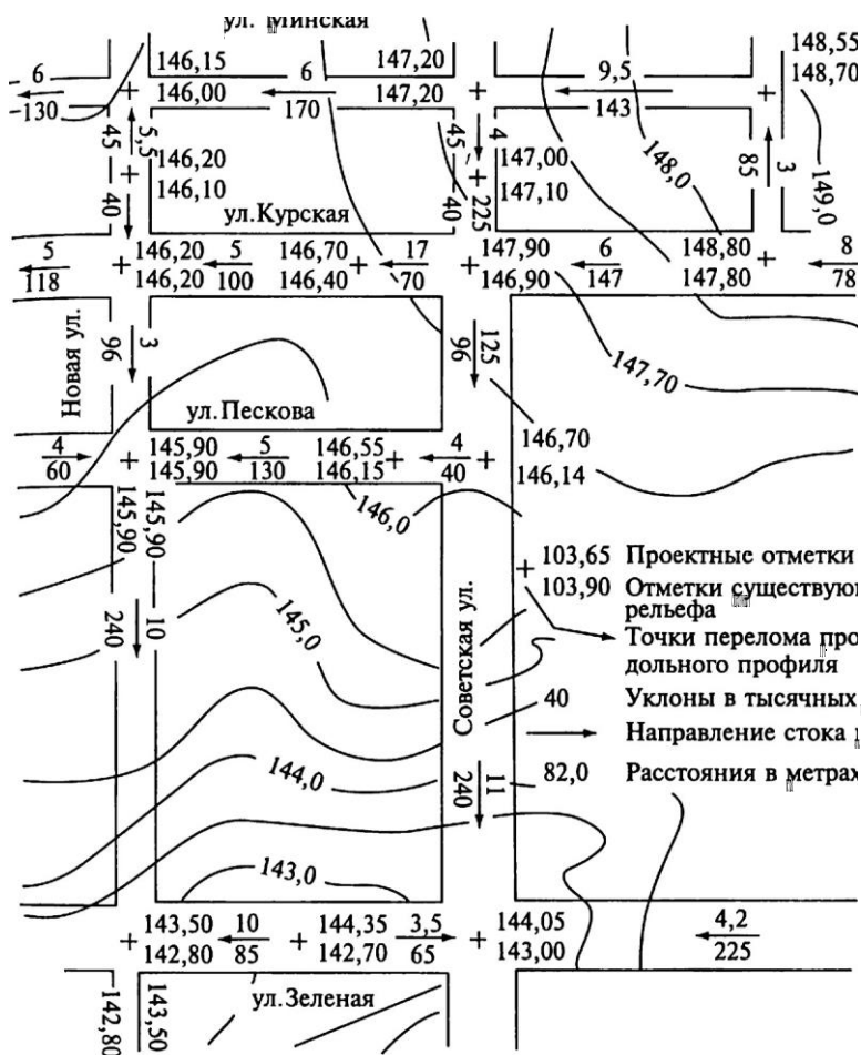
Рис. 18.3. Схема организации рельефа
