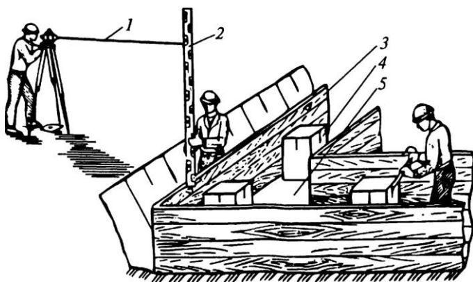
Рис. 20.4. Разбивка осей и отметок для установки арматуры и выверки опалубки (арматура условно не показана):
