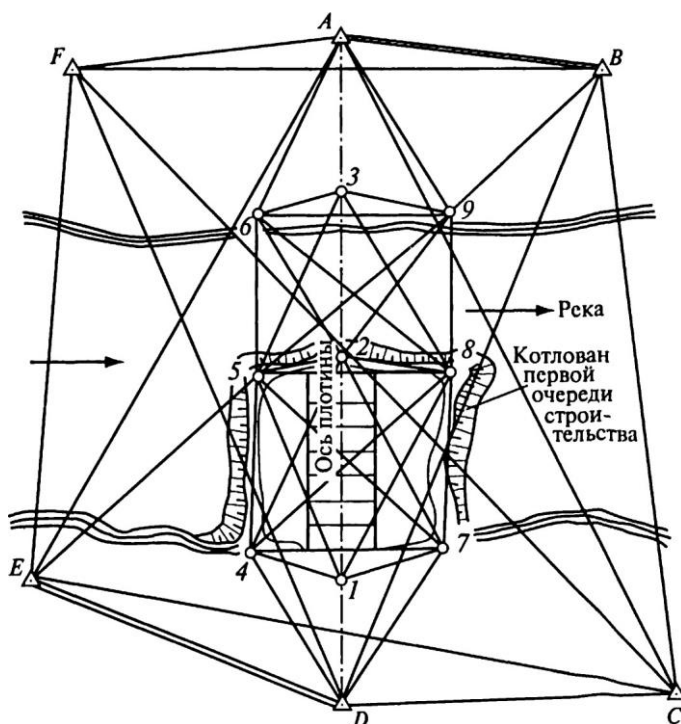
Рис. 26.2. Разбивочная триангуляционная сеть гидроузла
