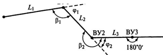
Рис. 25.2. Определение углов поворота по трассе
