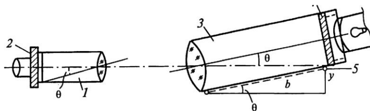
Рис. 22.3. Схема коллиматорного способа выверки прямолинейности:
