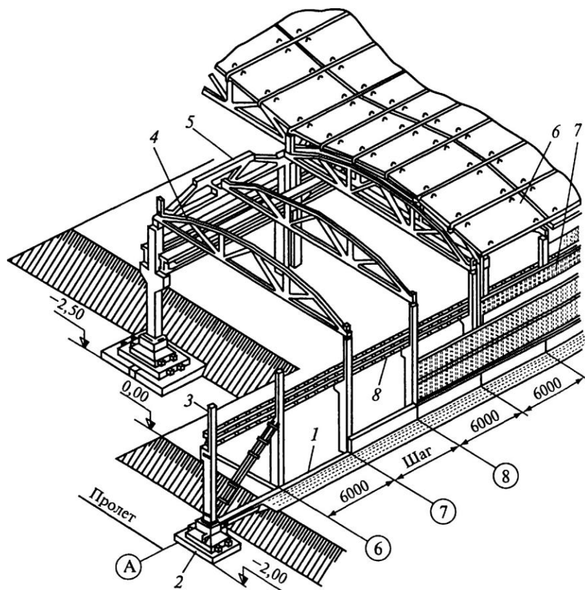
Рис. 21.1. Конструктивные элементы одноэтажного промышленного здания: 1, б — панели; 2 — фундамент; 3 — колонна; 4 — подстропильная ферма; 5 — стропильная ферма; 7 — подкрановая балка; 8 — фундаментная балка
