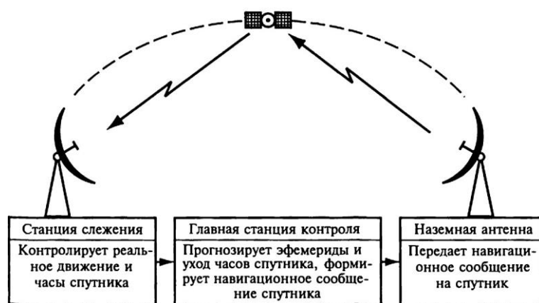
Рис. 14.8. Измерение, прогнозирование и обновление эфемерид спутника станций контроля и управления системой NAVSTAR GPS. Все станции системы NAVSTAR GPS расположены вдоль экватора.
