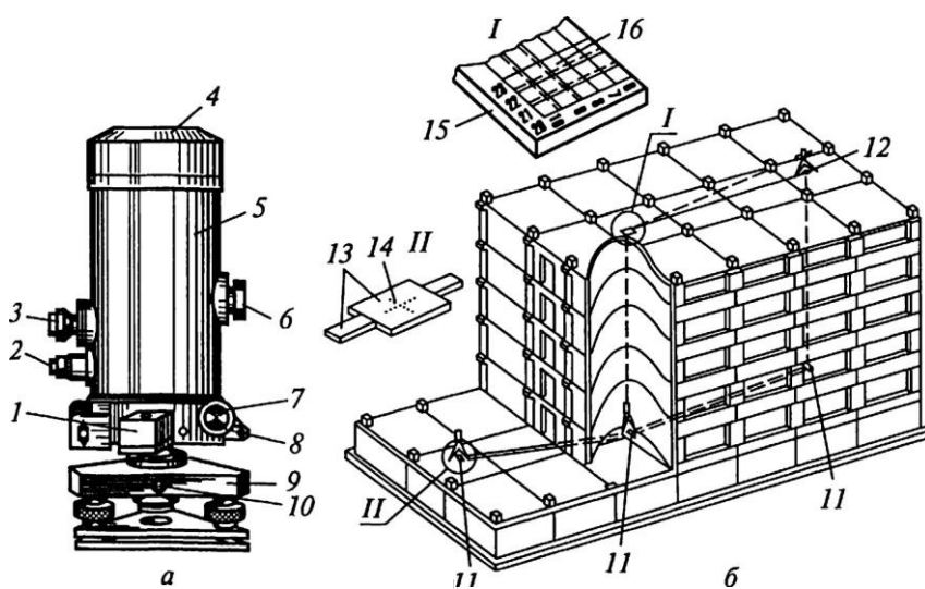
Рис. 9.7. Прибор вертикального проектирования ПЗЛ:
