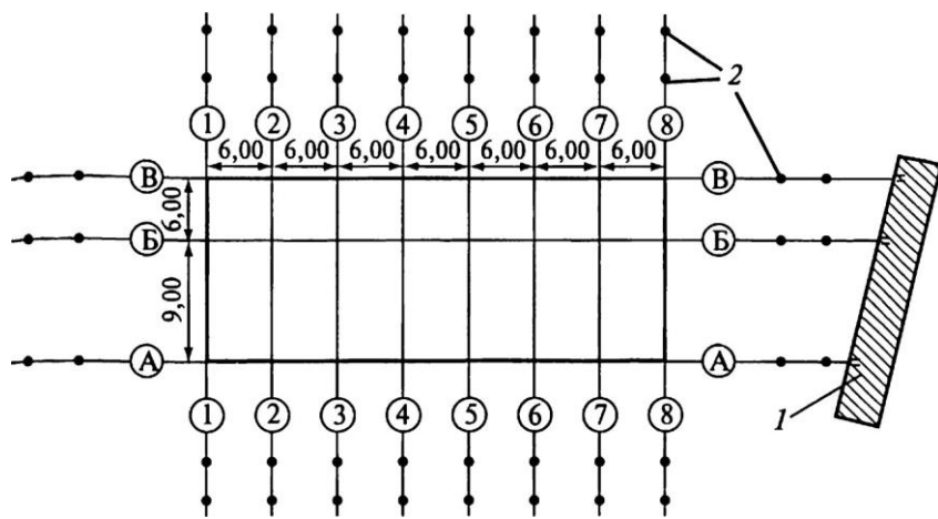
Рис. 17.5. Схема детальной разбивки осей:
