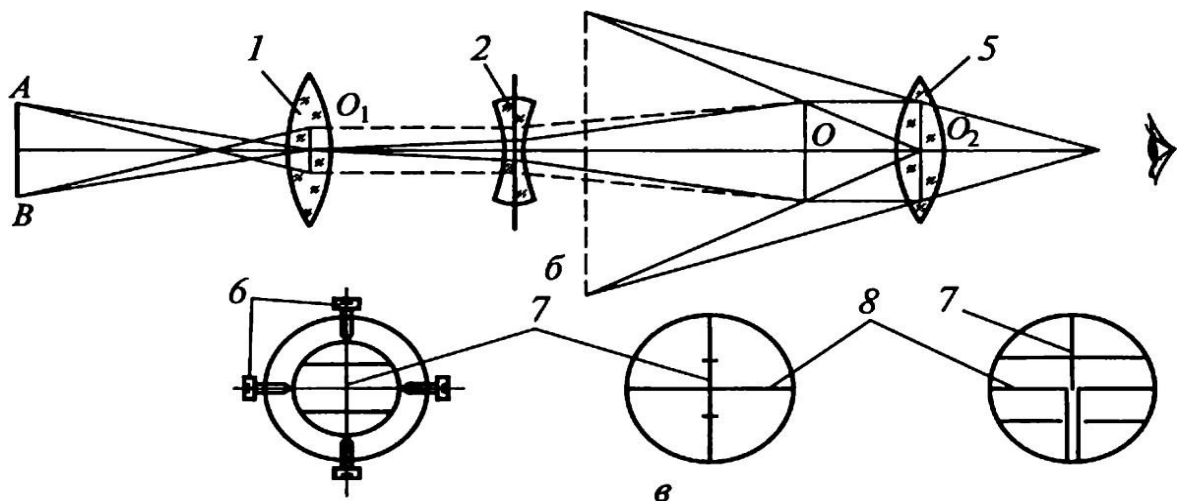
Рис. 7.1. Зрительная труба нивелира:
