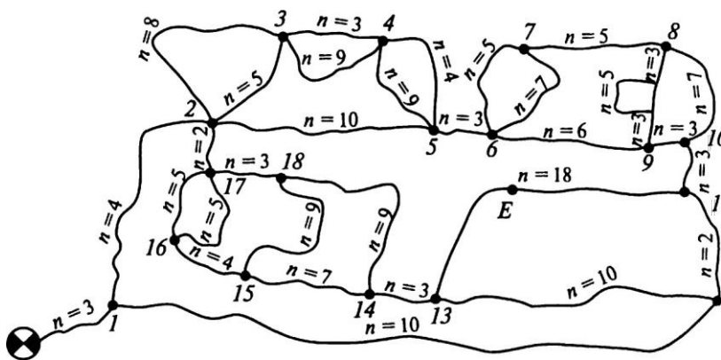
Рис. 24.3. Схема нивелирных ходов для наблюдений за осадками ТЭЦ
