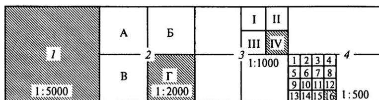
Рис. 3.2. Прямоугольная разграфка листа плана
