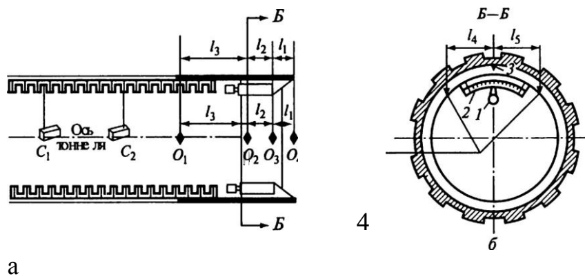
Рис. 27.14. Геодезическое обеспечение щитовой проходки:
