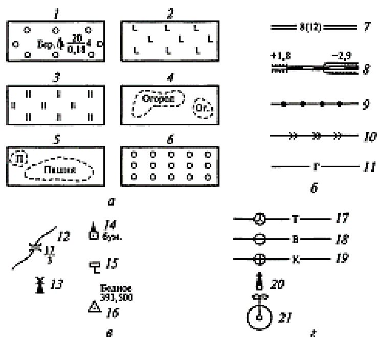
Рис.3.4. Условные знаки:
