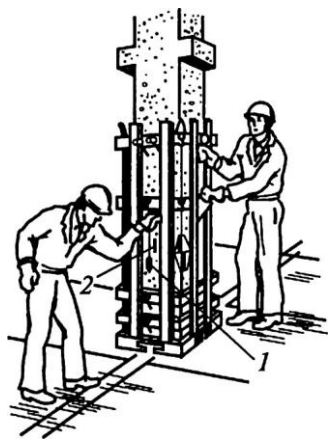
Рис. 20.20. Выверка колонны в нижнем сечении:
