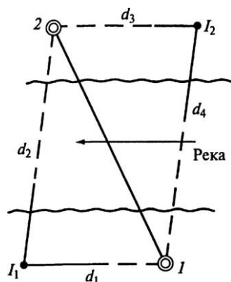
Рис. 25.15. Схема передачи отметки через водное препятствие:
