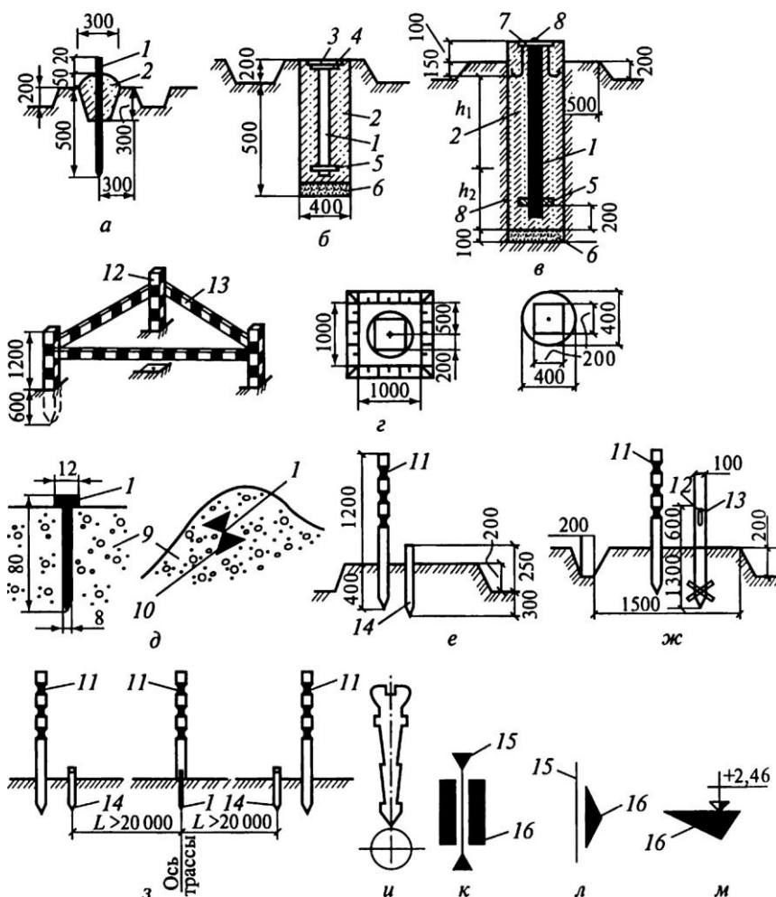
Рис. 10.4. Знаки закрепления:
