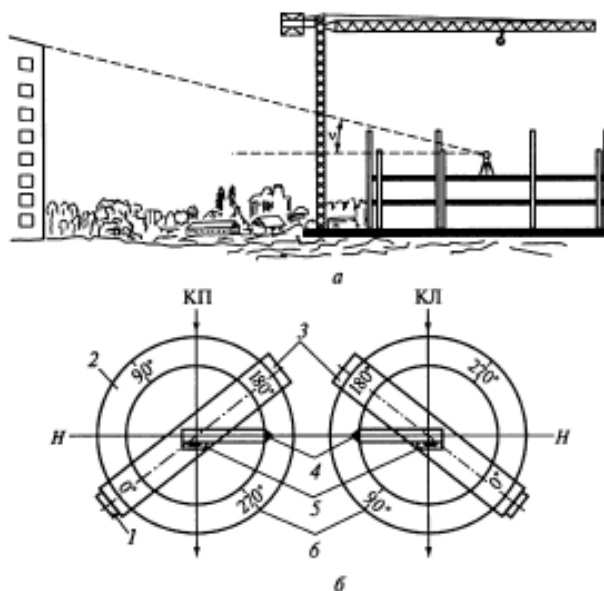
Рис. 8. В. Измерение вертикального угла:
