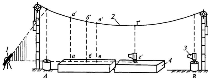
Рис. 22.2. Схема струнно-оптического способа установки конструкций: 1 — теодолит; 2 — струна; 3 — прибор вертикального проектирования; 4 —
