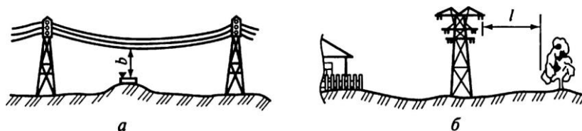
Рис. 29.1. Габаритные размеры приближения проводов:
