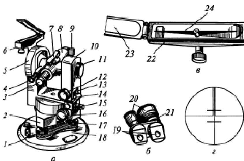
Рис. 8.5. Теодолит ЗТ30:
