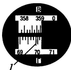
Рис. 8.6. Поле зрения отсчетного микроскопа теодолита ЗТЗО:
