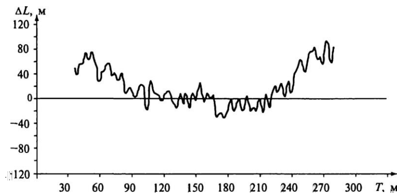
Рис. 14.15. Влияние искажения стандарта частоты
