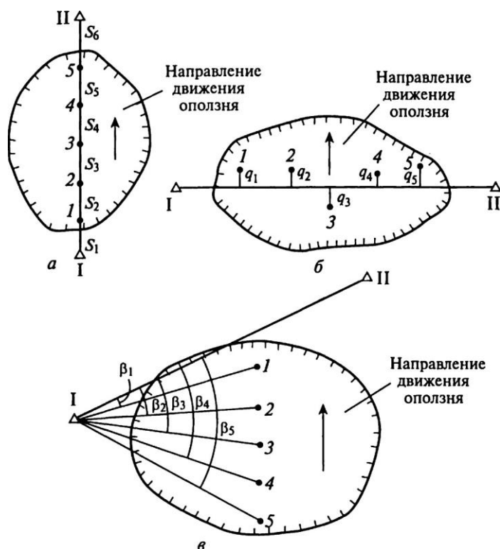
Рис. 24.8. Схемы наблюдений за оползнями:
