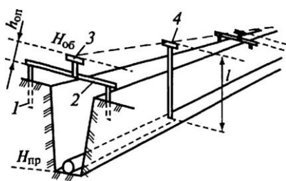
Рис. 19.1. Обноска для применения способа визирок при рытье траншей: 1 — деревянный столб; 2 — горизонтальная доска; 3 — опорная визирка;
