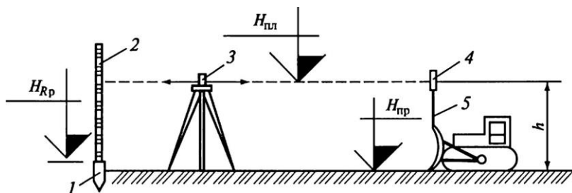
Рис. 9.4. Планировочные работы:
