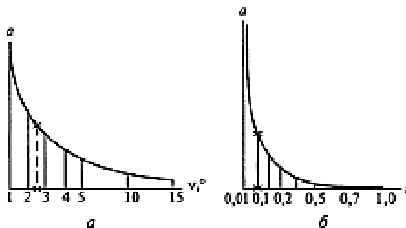
Рис. 4.7. Графики заложений к плану масштаба 1: 1000 при высоте сечения рельефа h = 1,0 \text{ м} :
