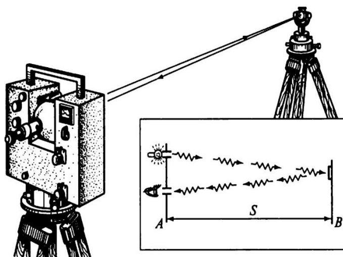
Рис. 6.10. Светодальномер:
