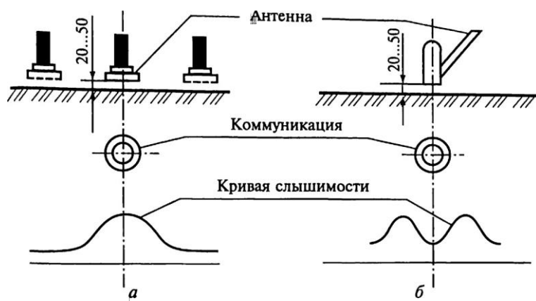
Рис. 19.3. Схемы определения планового местоположения подземных коммуникаций при помощи прибора поиска:
