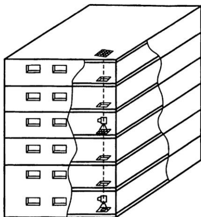
Рис. 20.11. Схема переноса точек закрепления осей с исходного на монтажный горизонт вертикальным проектированием
