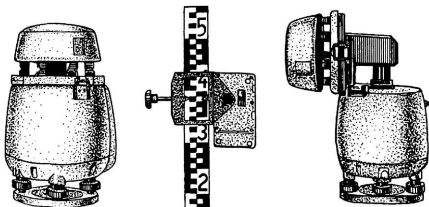
Рис. 9.1. Лазерный нивелир:
