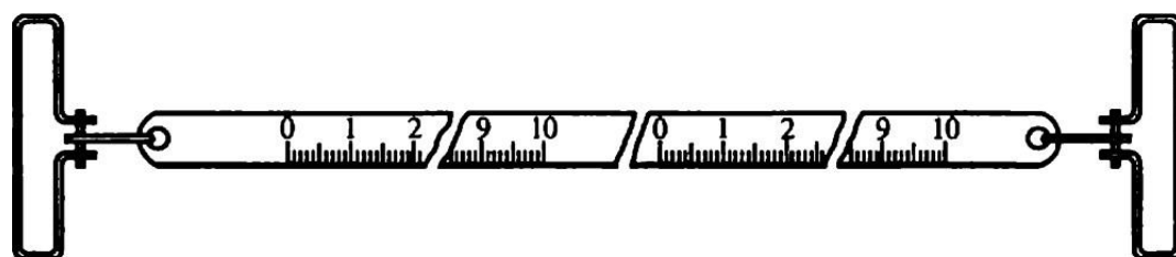
Рис. 6.3. Землемерная лента шкаловая
