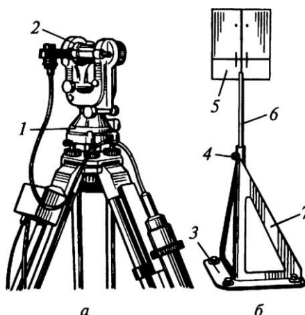
Рис. 9.2. Лазерный теодолит (а) и визирная марка (б): 1, 2 — горизонтальный и вертикальный круги; 3 — опора; 4 — закрепительный винт; 5 — марка; 6 — стержень, 7 — стойка
