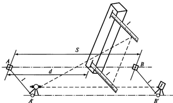
Рис. 16.7. Схема разбивки способом бокового нивелирования
