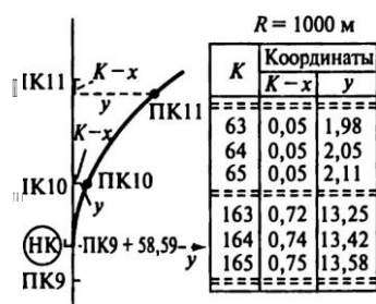
Рис. 25.4. Расчет пикетажа:
