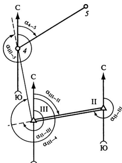
Рис. 8.16. Схема вычисления дирекционных углов
