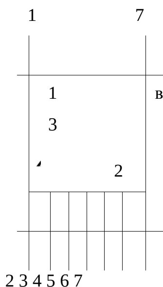
Рис. 20.22. Схема разбивки и контроля блочного здания:
