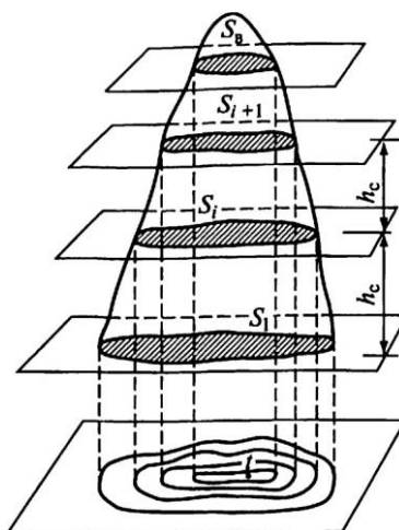
Рис. 4.11. Схема определения объема по карте с горизонталями
