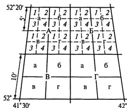
Рис. 3.1. Деление карты масштаба 1:100000 на листы карт масштабами 1:50000, 1:25000 и 1:10 000
