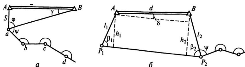
Рис. 13.8. Схемы привязки полигонометрического хода к стенным знакам: а — при прямой видимости; б — при отсутствии прямой видимости смежных знаков
