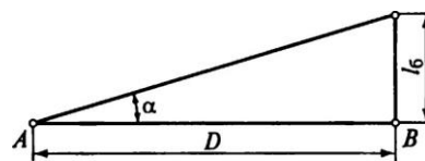
Рис. 6.9. Схема выполнения дальномерных измерений при постоянном базисе
