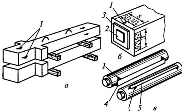
Рис. 20.18. Разметка колонн:
