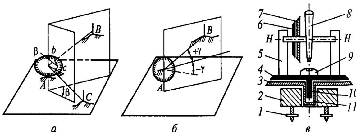
Рис. 8.1. Измерение углов теодолитом:
