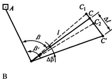
Рис. 15.2. Схема построения в натуре проектного угла
