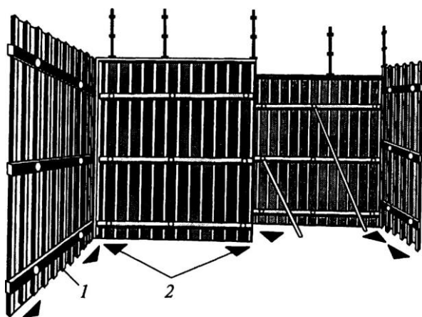
Рис. 20.23. Разметка рисок для установки вертикальных щитов опалубки:
