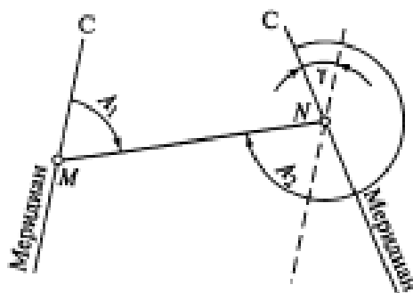
Рис. 2.1. Азимуты
