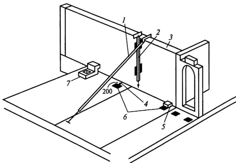
Рис. 20.15. Выверка панелей в отвесном положении:
