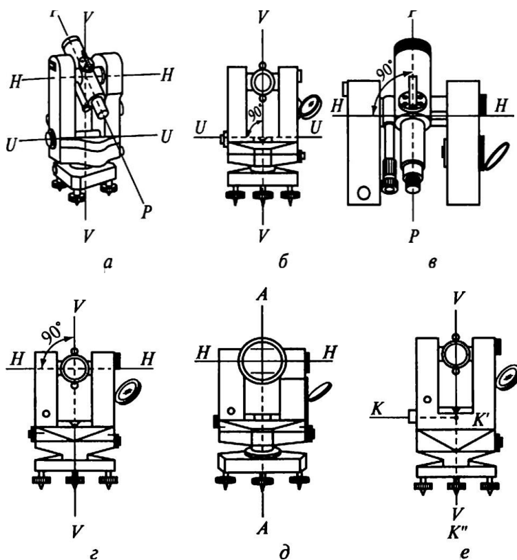
Рис. 8.11. Схемы (а... е) геометрических осей теодолита
