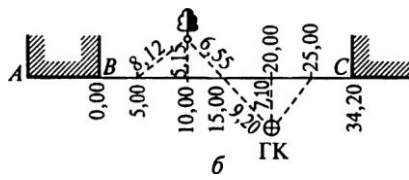
Рис. 11.2. Абрисы съемок, выполненных способами полярных координат (а) и створным (б)
