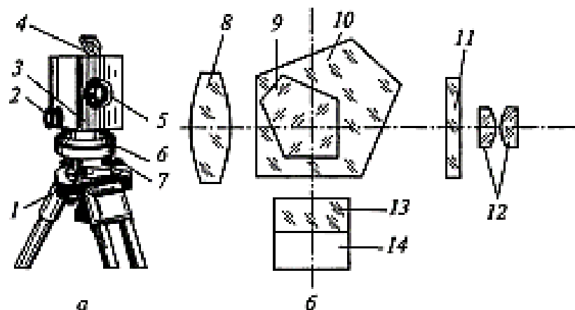
Рис. 7.5. Нивелир Н- ШКП:
