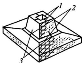
Рис. 20.7. Совмещение рисков при монтаже фундамента под колонну:
