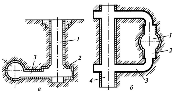
Рис. 27.1. Схема сооружения тоннеля через ствол:
