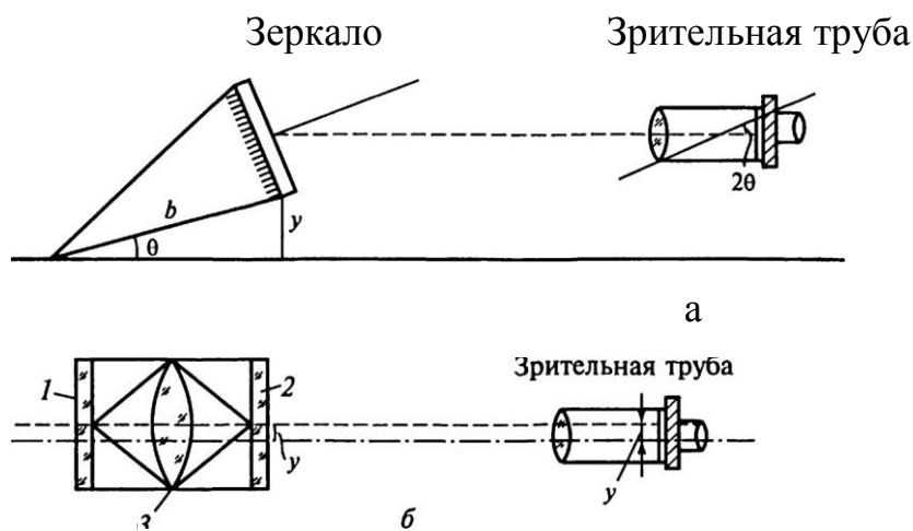
Рис. 22.4. Схемы автоколлимационных способов выверки прямолинейности: а — первый; б — второй; 1 — зеркало; 2 — защитное стекло; 3 — объектив
