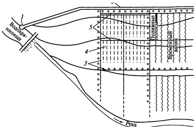
Рис. 26.7. Открытая оросительная система:
