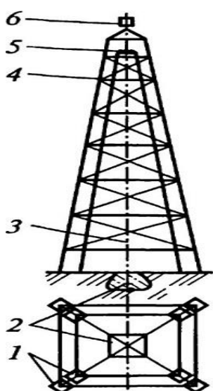
Рис. 10.3. Наружный металлический сигнал над подземным центром плановой сети: — фундаменты; 2 — подземный центр; 3 — сигнал; 4 — настил; 5 — столик; 6 — визирная цель
