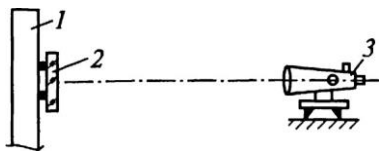
Рис. 22.9. Схема установки конструкции по вертикали автоколлимационным способом:
