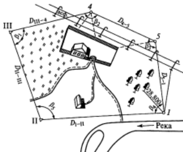
Рис. 8.14. Схема теодолитного хода:
