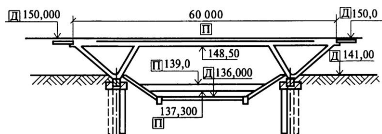
рис. 30.1. Обозначение действительных Д и проектных [О отметок на фасаде продольного профиля мостового перехода
