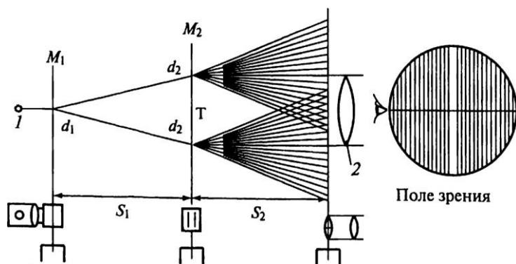
Рис. 22.5. Схема дифракционного способа выверки прямолинейности:
