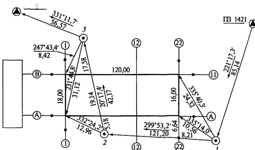
Рис. 18.2. Разбивочный чертеж для выноса в натуру основных осей здания:
