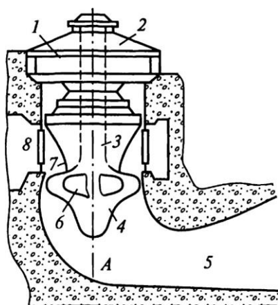
Рис. 26.6. Конструктивная схема
