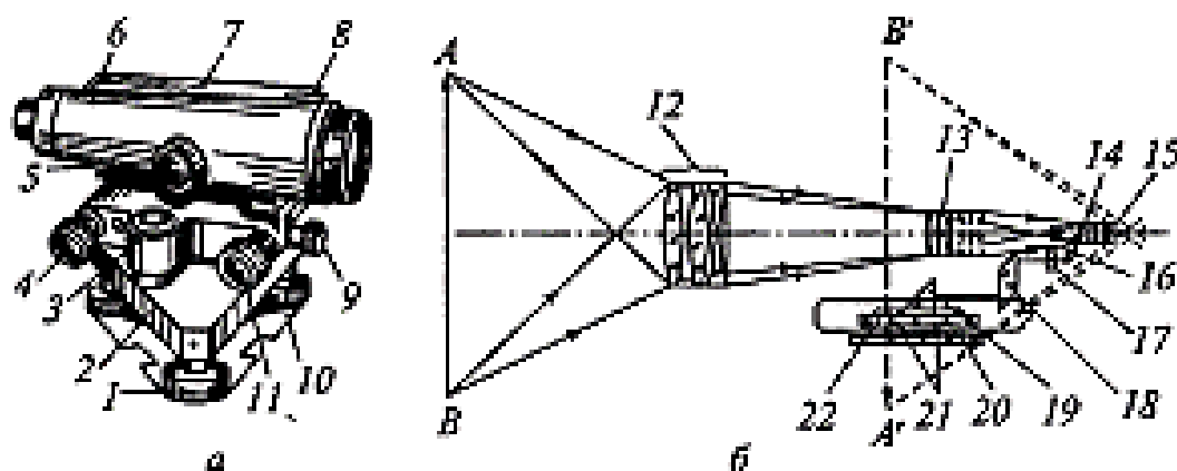
Рис. 7.6. Нивелир Н-3:
