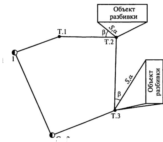
Рис. 21.3. Схема разбивки с удаленным расположением свободной станции I
