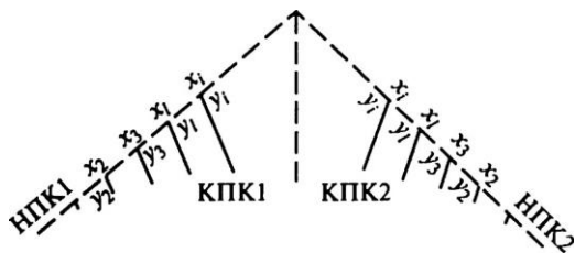
Рис. 25.8. Схема разбивки кривой способом прямоугольных координат
