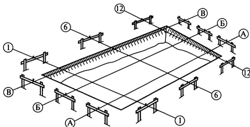
Рис. 17.6. Створная обноски для закрепления осей здания
