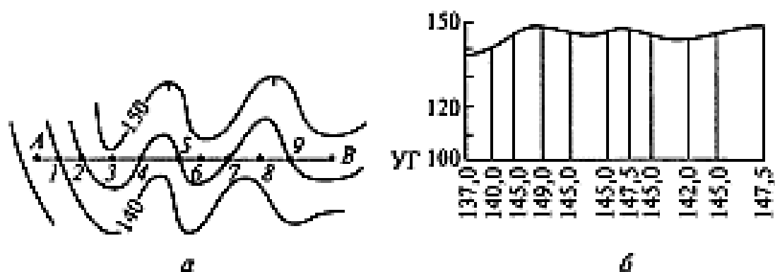
Рис. 4.10. Схемы построения профиля по заданному направлению: а — направление по карте; б — профиль по направлению
