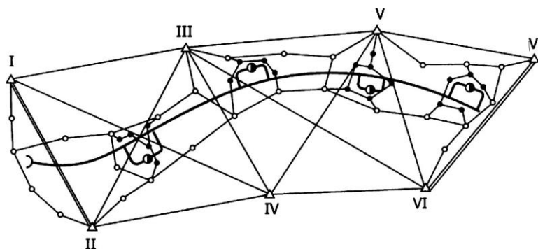
Рис. 27.9. Схема планового геодезического обоснования тоннеля:
