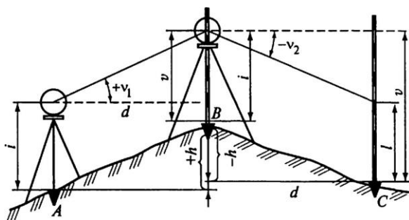
Рис. 7.12. Схема тригонометрического нивелирования
