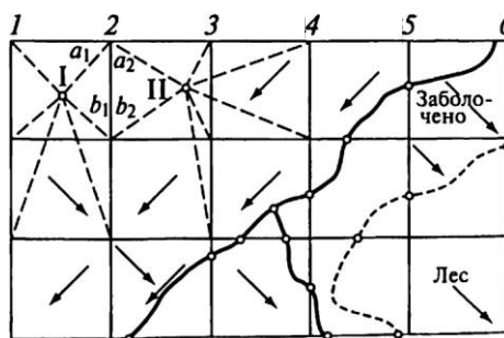
Рис. 11.5. Абрис съемки способом нивелирования по квадратам (стрелками указано направление скатов)
