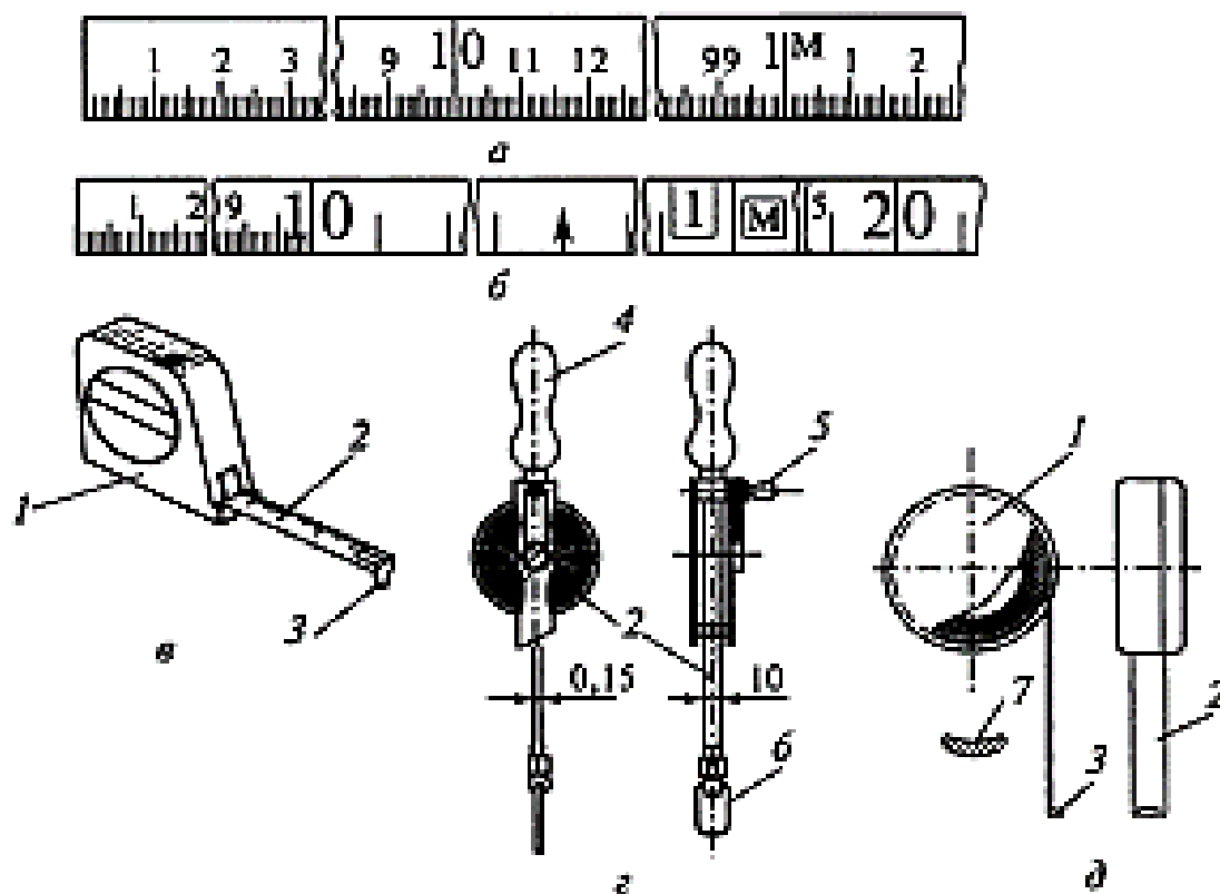
Рис. 6.1. Стальные рулетки:
