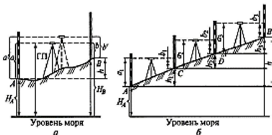
Рис. 7.9. Схемы нивелирования: а — простого; б — сложного
