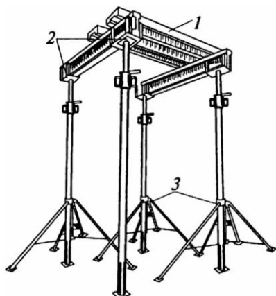
Рис. 20.26. Опалубка перекрытий:
