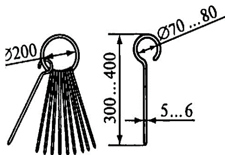
Рис. 6.4. Набор шпилек
