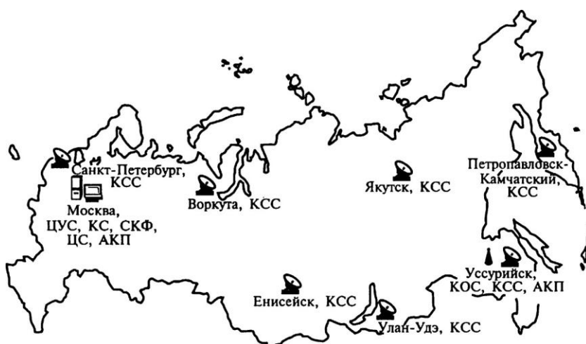
Рис. 14.6. Размещение станций контроля и утирждения системы ГЛОНАСС: ЦУС — центр управления системой ГЛОНАСС; ЦС — центральный синхронизатор; КС — контрольная станция; СКФ — система контроля фаз; КОС — квантово-оптическая станция; АКП — аппаратура контроля параметров; КСС — контрольная станция слежения
