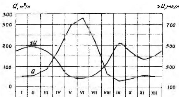
1.11.4-rasm. Chirchiq daryosi (Chinoz yaqinida) oʻrtacha koʻp yillik suv sarfi va minerallashuvining yil davomida oʻzgarishi
