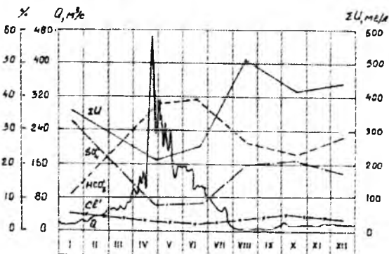
1.11.2-rasm. Ohangaron daryosi suvining (Samarskoy qo'rg'oni yaqinida) minerallashuvi va undagi asosiy anionlar miqdorining yil davomida o'zgarishi
