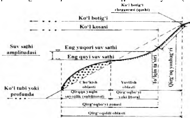
1.12.1-rasm. Koʻl botigʻi va uning qismlari.
