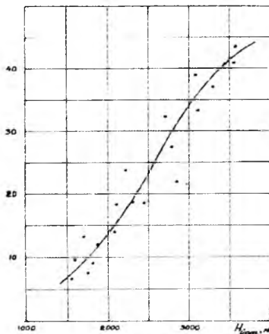
1.10.1-rasm. Oqim moduli ( M )ning havzaning o'rtacha balandligi ( H_{ort} ) ga bog'liqligini ifodalovchi chizma
