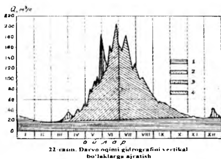
1.9.1-rasm. Daryo oqimi gidrografini vertikal bo'laklarga ajratish.
