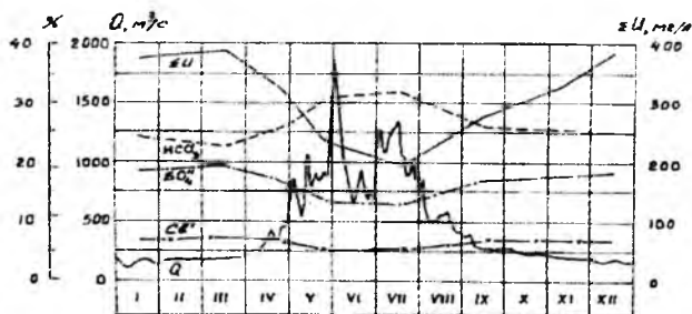
1.11.1-rasm. Norin daryosi suvining (Uchqo'rg'on yaqinida) mineral-lashuvi va undagi asosiy anionlar miqdorining yil davomida o'zgarishi
