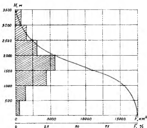
1.7.3-rasm. Daryo havzasining gipsografik egri chizig'i
