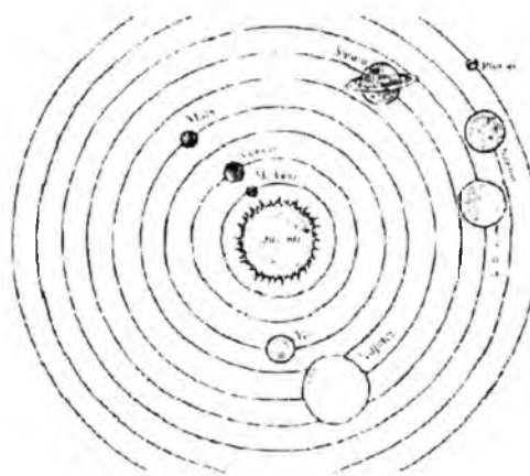
2-rasm. Quyosh sistemi.
