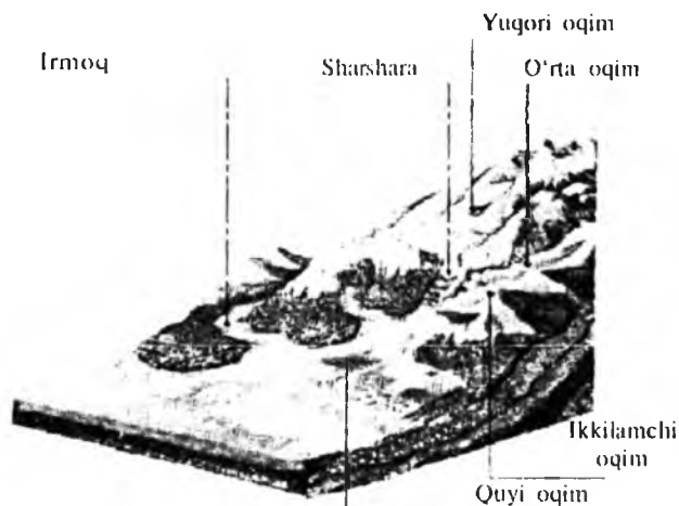
56-rasm. Daryo qismlari.
