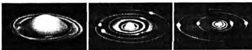
3-rasm. Quyosh sistemi paydo bo'lishining uch bosqichi.
