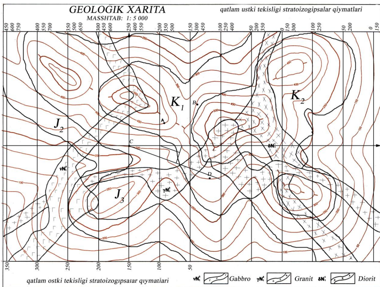
5-rasm. Aniqlangan qatlamning ustida yotgan qatlamlarni topish
