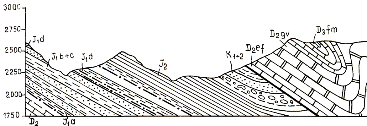
8-rasm. Geologik kesmaning umumiy ko'rinishi
