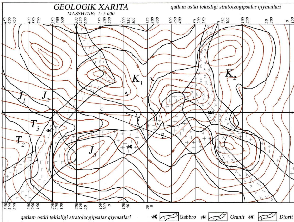
6-rasm. Aniqlangan qatlamning ostida yotgan qatlamlarni topish
