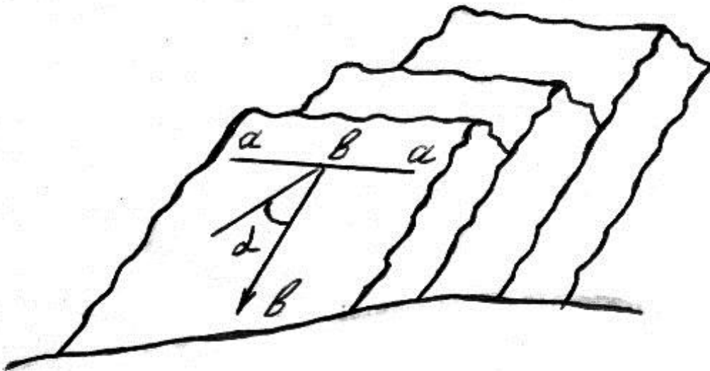
1–rasm. Qiya yotgan qatlamlarning yotish elementlari
