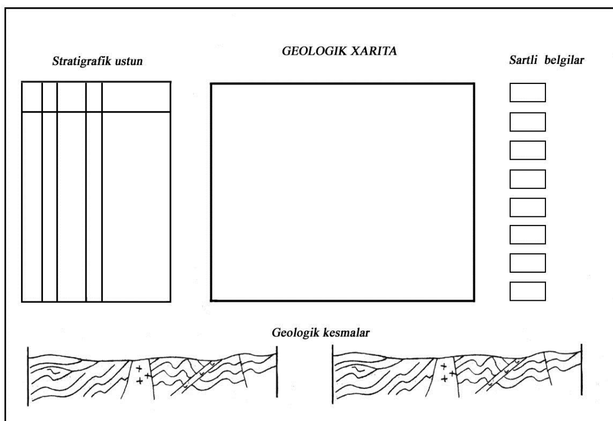
11-rasm. Chizmalarni joylashish tartibi
