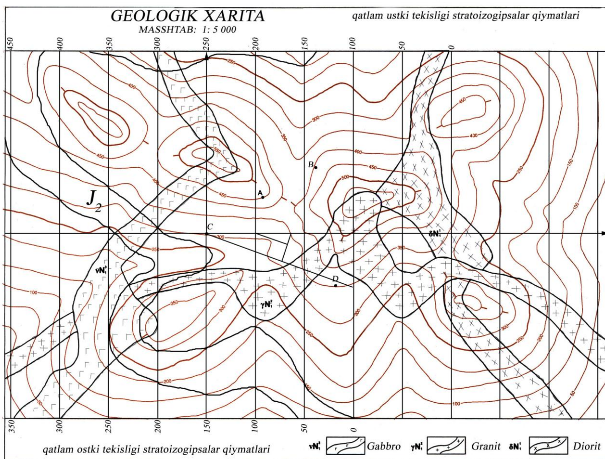
4-rasm. Burg'i qudug'i ma'lumotlari asosida qatlamning chegaralarini o'tkazish
