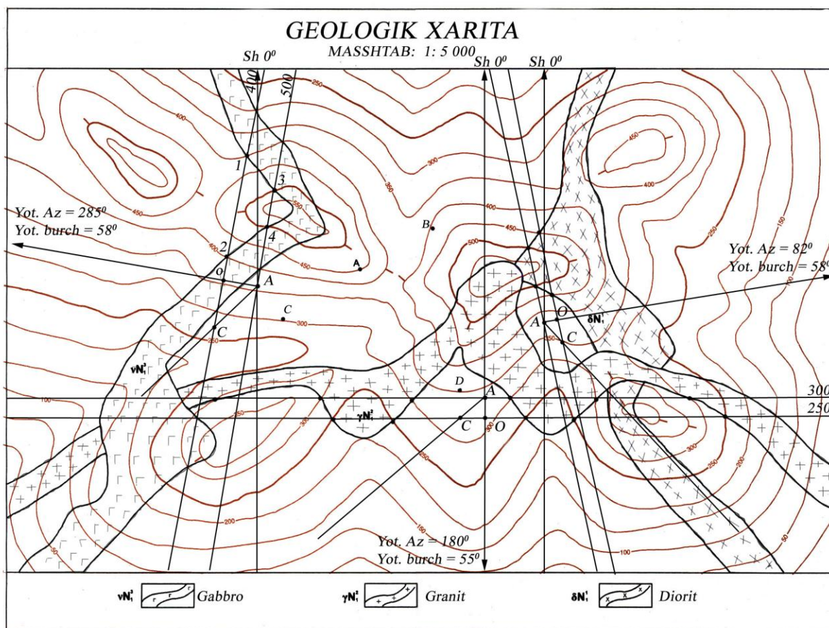
3–rasm. Qiya yotgan qatlamning yotish elementlarini aniqlash
