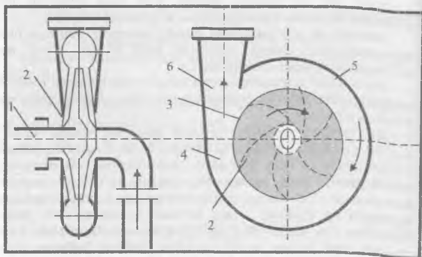
3.4.1-rasm . Markazdan qochma nasos sxemasi.
