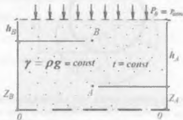
2.12.3-Rasm. O'tkazilayotgan P_{uz-st} bosimni aniqlash.
