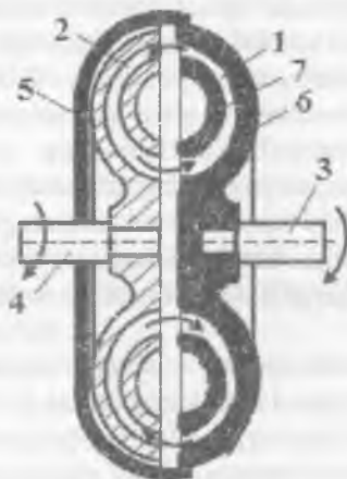
8.16.1-rasm. Hidrodinamik mufta yoki turbomufta nasos g'ildiragi 1-turbina g'ildiragi. 2 – yetaklovchi val. 3 – yetaklanuvchi val. 4 – diafragmali bosqich. 5 – yarim korpus. 6 – yarim tor. 7 – lardan iborat.
