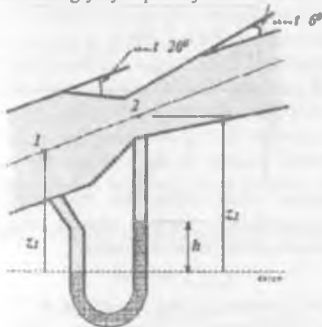
3.20.1-rasm. Venturi suv o'lchagichlari
