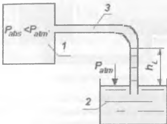
2.32.3-rasm. Vakuummetrik balandlik
