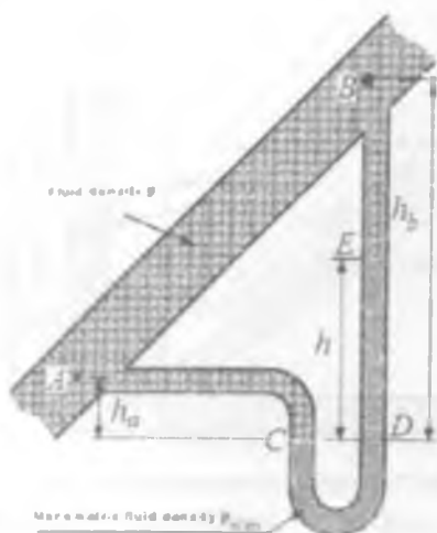
2.26.8-rasm. "U" – Trubkali manometr yordamida bosimlarning to'g'riliqligini o'lchash
