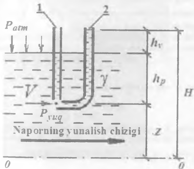
3.5.1-rasm. Gidrodinamik naporni tushintirishga doyr sxema:
