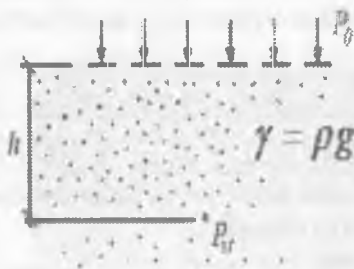
5.7.1-rasm. Statik bosimini aniqlash sxemasi.
