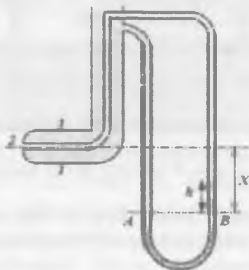
3.19.1-rasm. Pito statik trubka.
