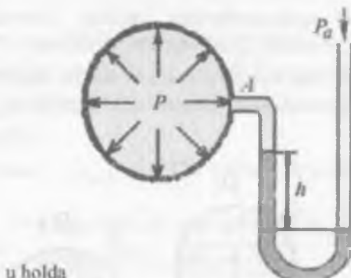
2.26.4-rasm. Vakuummetr
