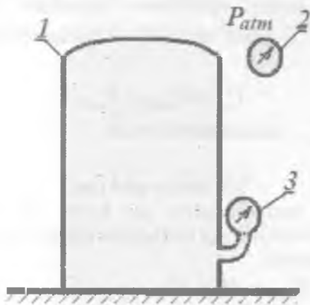
5.7.2-rasm. P_{st} O'lchosh sxemasi. 1-Idish; 2-barometr; 3-manometr yoki vakuummetr
