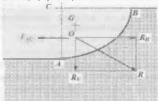
2.8.2-rasm. Gorizontalgaga ta'sir qiluvchi natijaviy kuch
