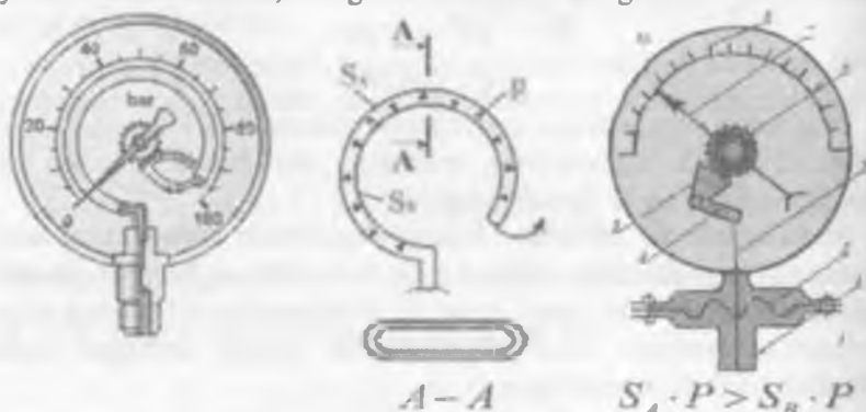
2.26.11. a-rasm. Purjinali manometr. 2.26.11. b-rasm. Membranali manometr
