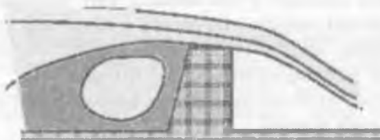
3.8.2-rasm. Suv chiqishi to'sig'i ustidan o'tgan ikki o'lchamli oqim
