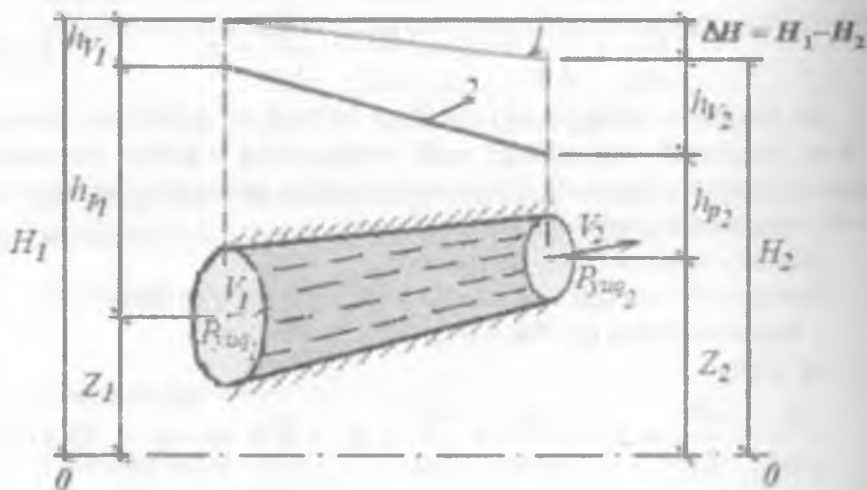
3.12.1-rasm. Bernulli tenglamasiga doir sxema:
