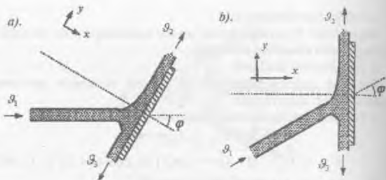
3.27.1-rasm. a – b. Qiya tekislikdagi reaktiv oqim Q_3
