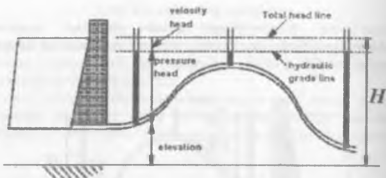
3.14.3-rasm. Suyuqlik o'tayotganda p'ezometr darajalari.
