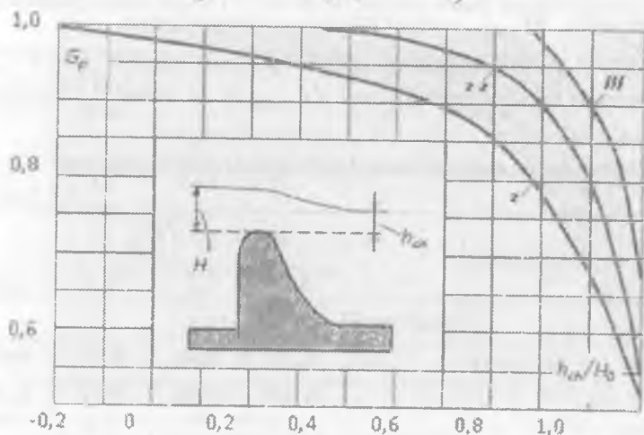
7.7.7-rasm. Amaliy profilni suv to'kgichlarning cho'ktirish koeffitsiyenti \sigma_{ch} ni aniqlash grafigi
