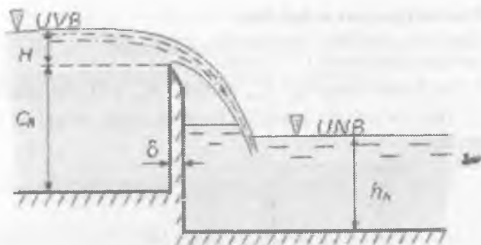
7.7.1-rasm. Yupqa devorli cho'ktirilmagan suvto'kgich
