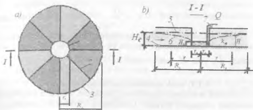
6.2.3. a, b-rasmlar. Tayyor chuqurga filtratsiya. a-reja; b-ko'ndalang kesim; 1-chuqur, 2-filtratsiya yo'nalishi, 3-chegara filtratsiya maydoni; 4-suv bosimi, 5-issiq suvni tabiiy bosimi, 6-pasaytirilgan tabiiy bosimga aylanma harakat, 7-nasos.
