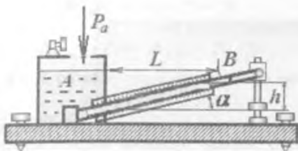
2.26.2-rasm. Mikromanometr
