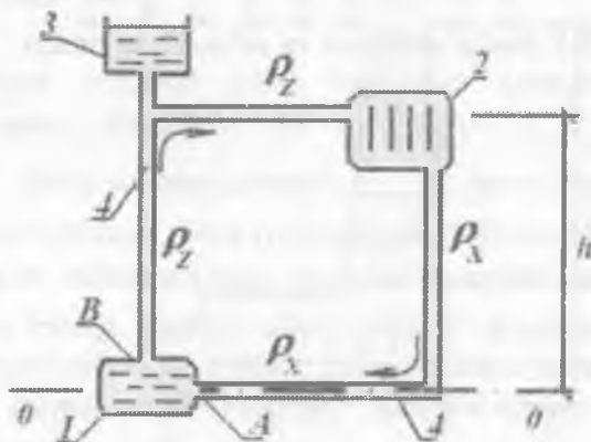
5.4.1-rasm. Tabiiy sirkulyatsion suv isitish sxemasi. 1-Suv isitgich qozoni; radiator; 3 – kengaytirilgan idish; 4-suv quvuri tizimi.
