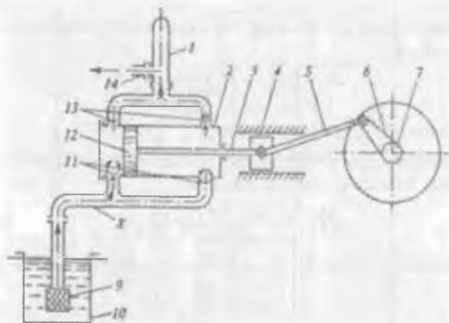
8.14.3-rasm. Ikki silindrli burg'ilash nasosi ishini sxemasi.
