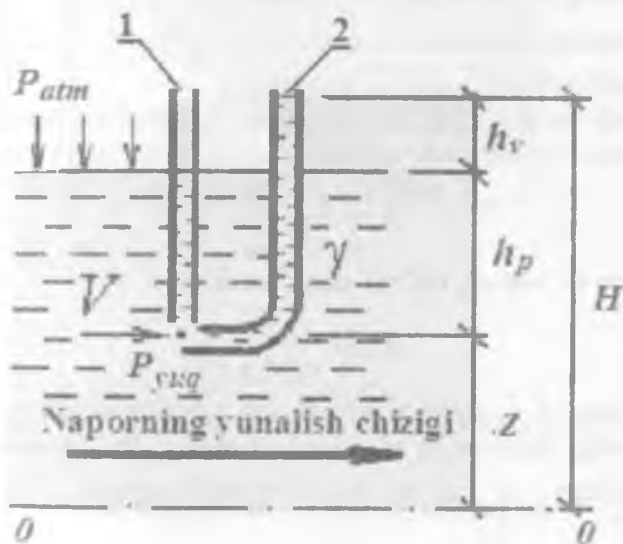
3.5.1-rasm. Gidrodinamik naporni tushintirishga doyr sxema.
