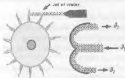
3.26.1-rasm. Pelton g‘ildiragi.
