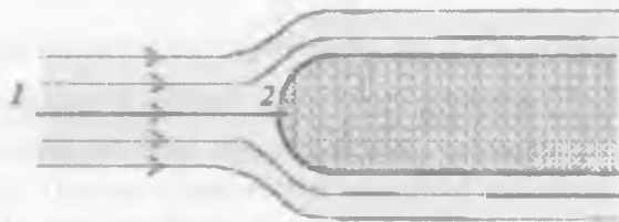
3.18.1-rasm. O'tmas jismda suyuqlikni oqishi
