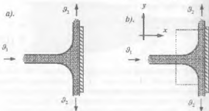
3.24.1-rasm. a-b. Tekislikka tushgan perpendikulyar oqim
