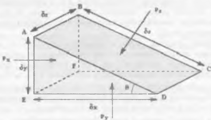
2.22.1-rasm. Suyuqlikning uchburchakli prizmatik elementi.
