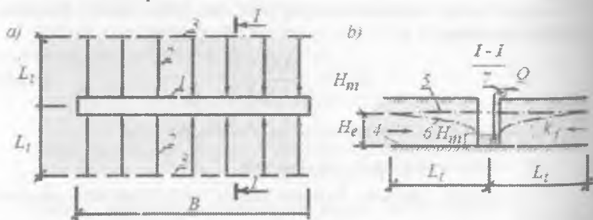
6.2.2. a, b-rasmlar. Chuqurga filtaratsiya. a-reja; b-kundalang kesim; 1-yauqur, 2-filtratsiya yunalishi, 3-chegara filtarasiya maydoni; 4-suv bosimi, 5-issiq suvni tabiiy bosimi, 6-pasaytirilgan tabiiy bosim, 7-nasos.
