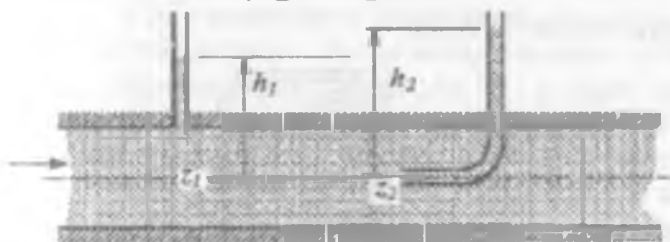
3.18.2-rasm. P'ezometr va Pito trubkasi
