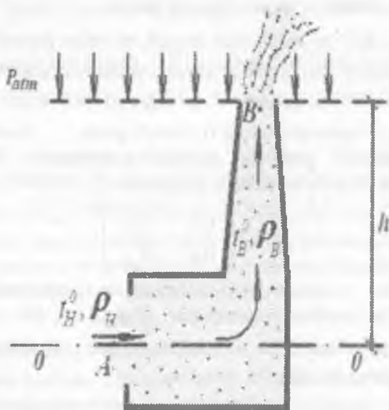
5.3.1-Rasm. Tutun quvurining sxemasi.
