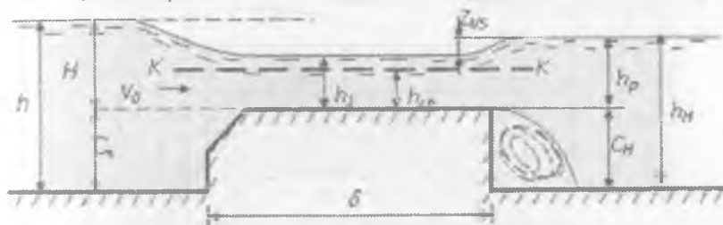
7.7.5-rasm. Keng zinali cho'ktirilgan suvto'kgich
