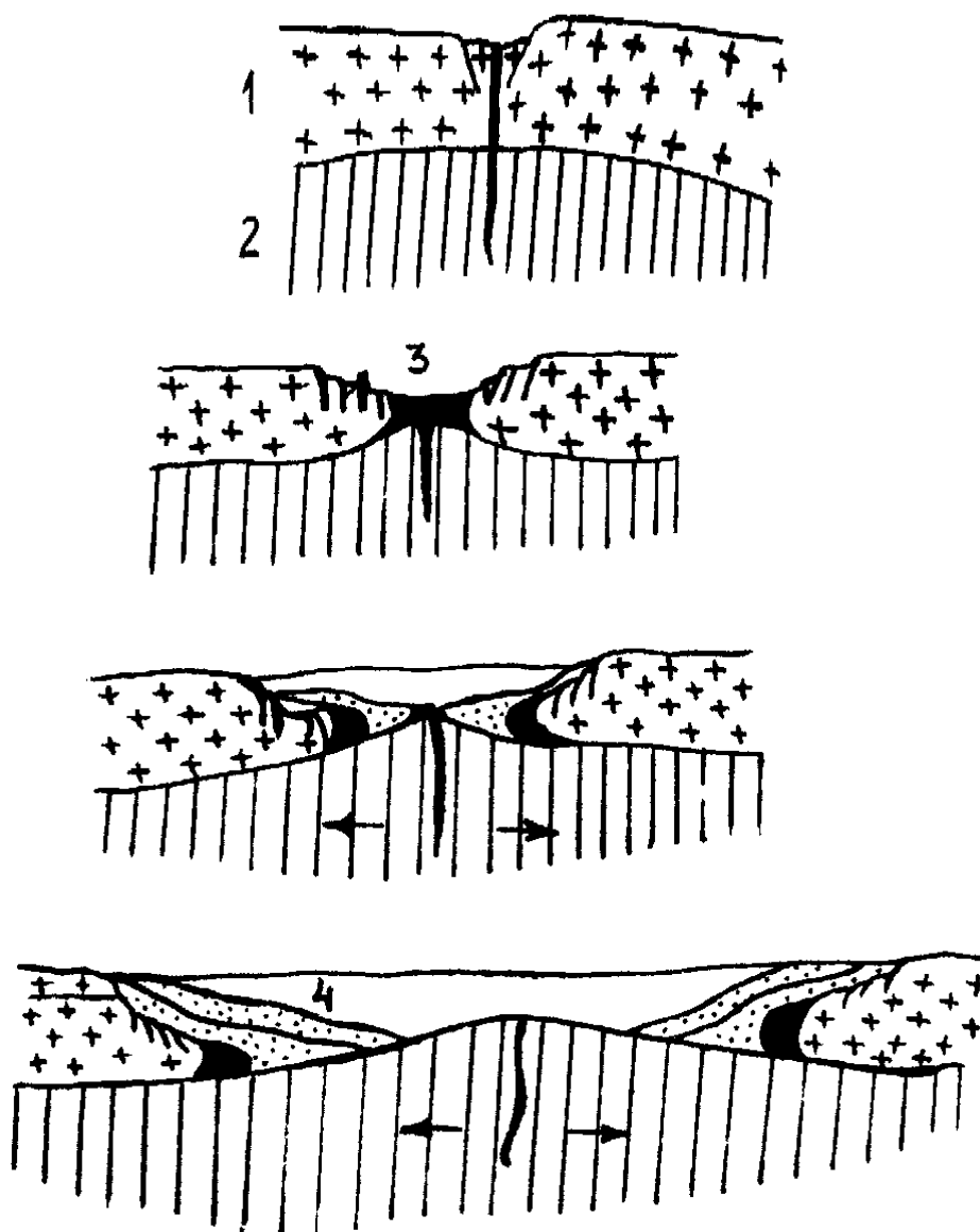
4.2-rasm. Chekka okean qismlaridagi harakatlar
