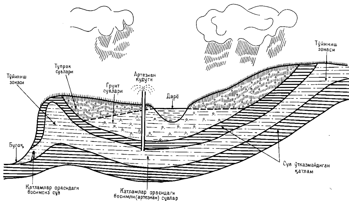
43-расм. Артезиан ҳавза (А.С.Иброҳимов ва А.Н.Султонхўжаевлар бўйича).
