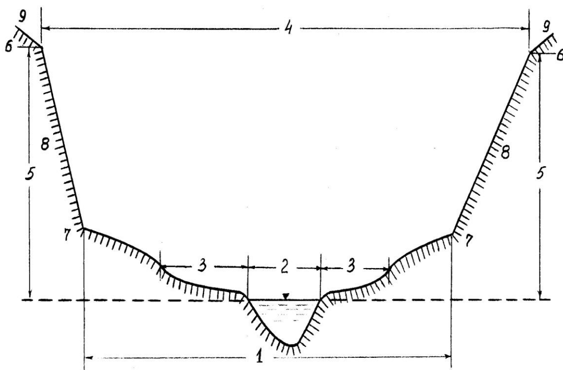
11-расм, А. Дарё водийсининг кўндаланг қирқими 1—водий туби, 2—дарё ўзани, 3—қайир, 4—водий кенглиги, 5—водий баландлиги, 6—водий қоши, 7 — ёнбағир пойи, 8—водий ёнбағирлари, 9—водийга туташ ерлар.
