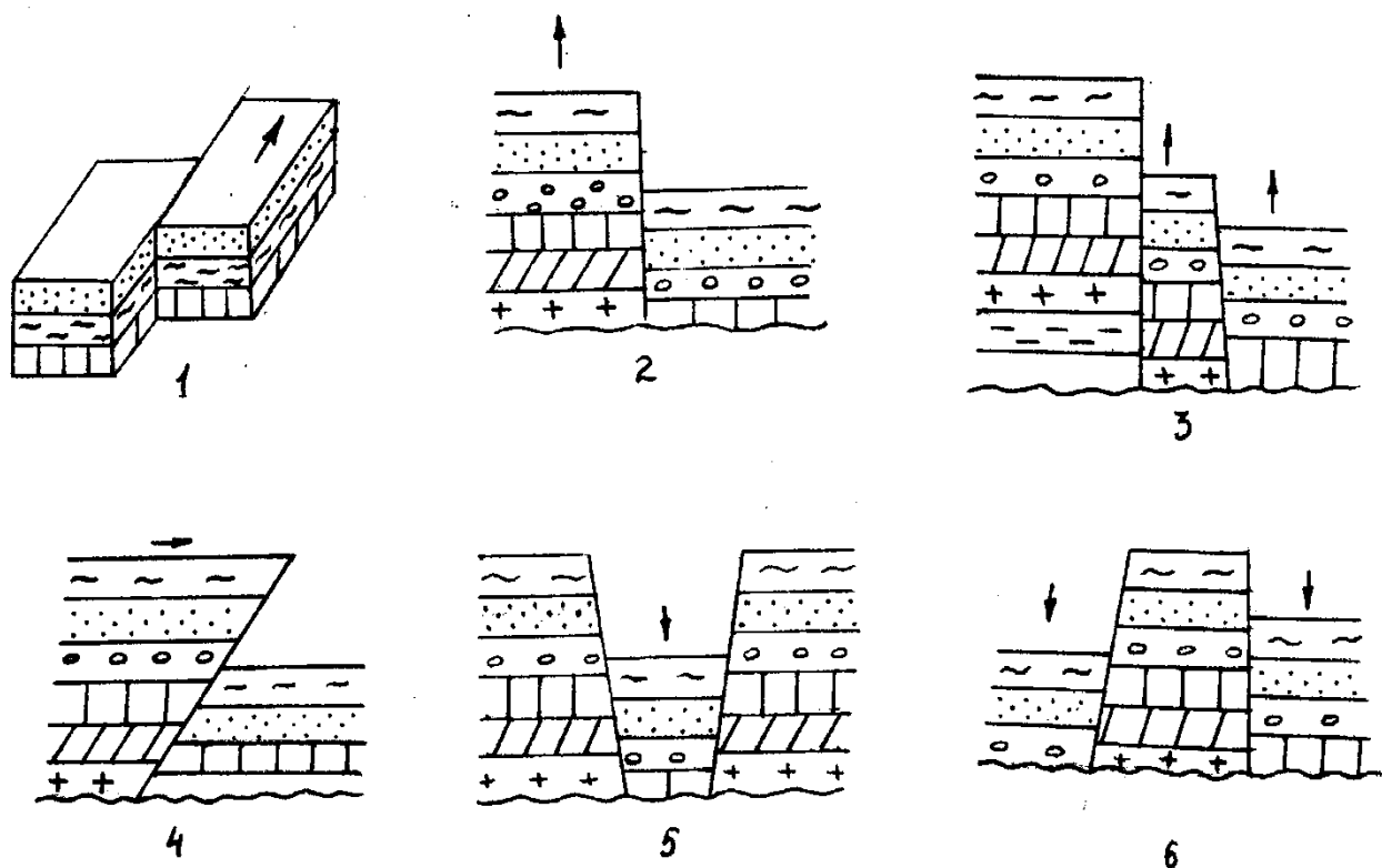
4.1-rasm. Uzilmali tektonik harakatlar
