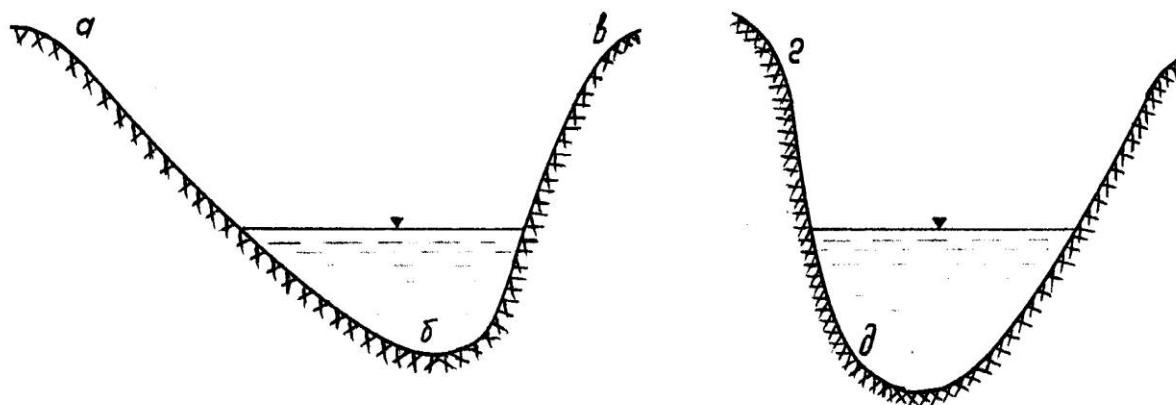
11-расм, Б. Дарё қирғоғининг турлари аб—ётиқ қирғоқ, бв—нисбатан тик қирғоқ, гд—жарсимон қирғоқ,
