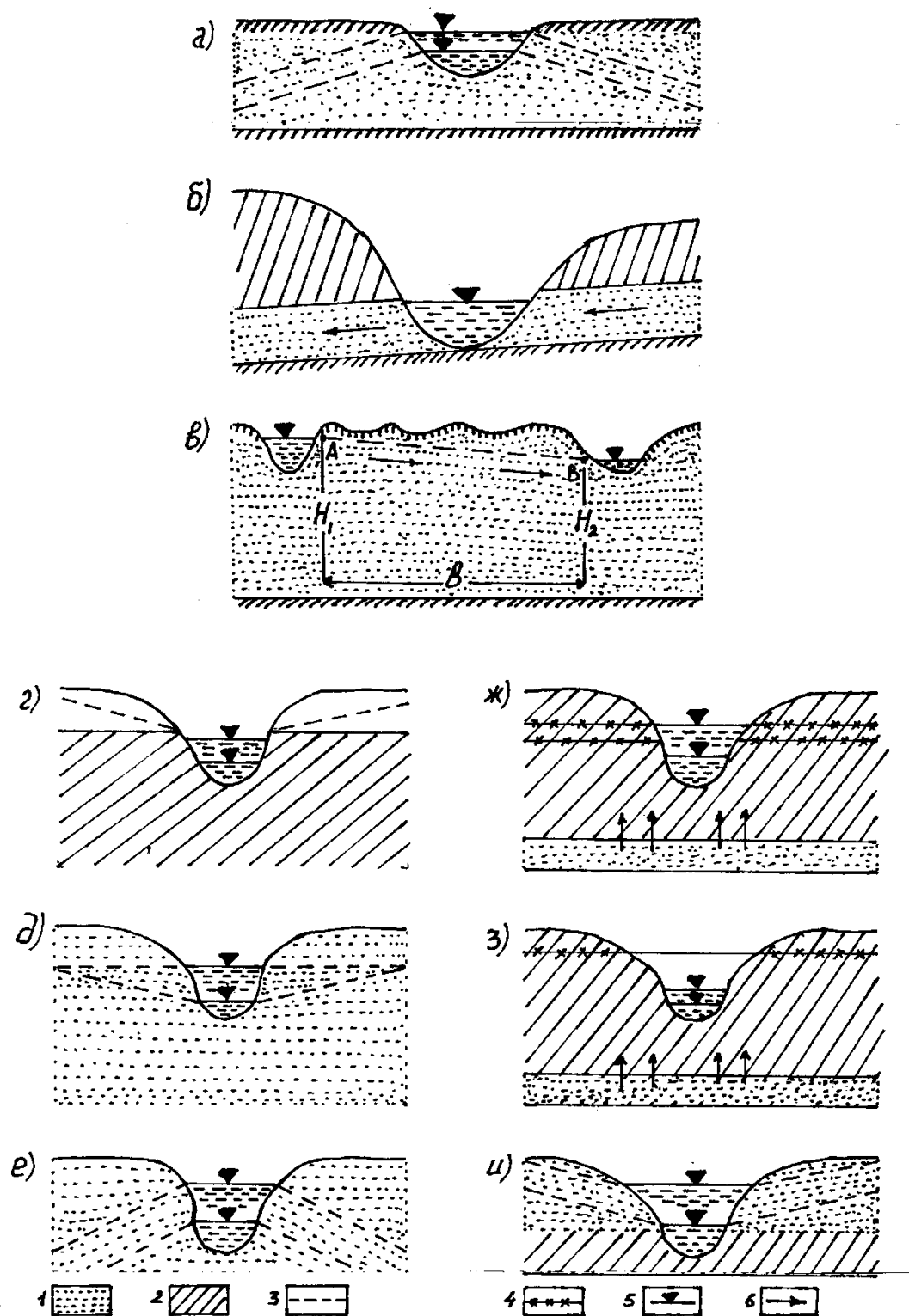
44-расм. Грунт сувларининг дарё оқими ҳисобида тўйиниши (а,б,в), грунт ҳамда дарё сувларининг гидравлик боғлиқлиги (д,е,ж,з,и). 1—сув ўтказувчи қатламлар, 2—сув ўтказмайдиган қатламлар, 3—грунт сувлари сатҳи, 4—босимли сувларнинг пьезометрик сатҳи, 5—дарё суви сатҳи, 6—ер ости сувларининг ҳаракат йўналиши.
