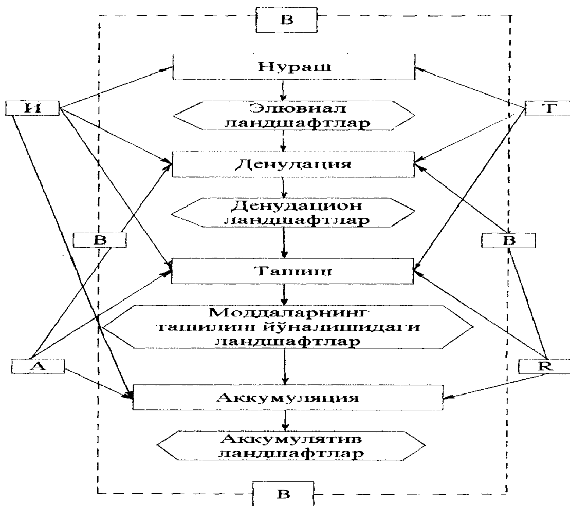
5.1-rasm. Nurash va boshqa ekzogen jarayonlar
