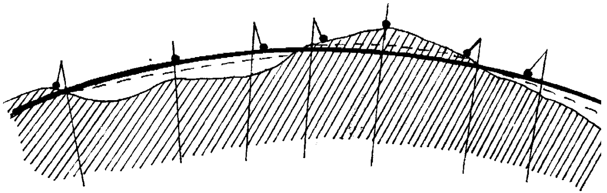
2.2-rasm. Geoid va ellipsoid aylanmasining yuzasi
