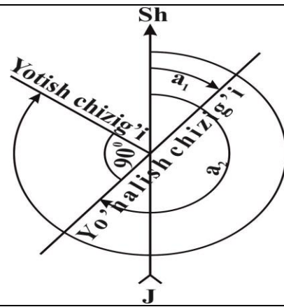
14.2-rasm. Planda qatlamning yotish elementlari orasidagi munosabat. a_1 va a_2 - yo'nalish chizig'ining azimutlari, a_3 - yotish chizig'ining azimuti.
