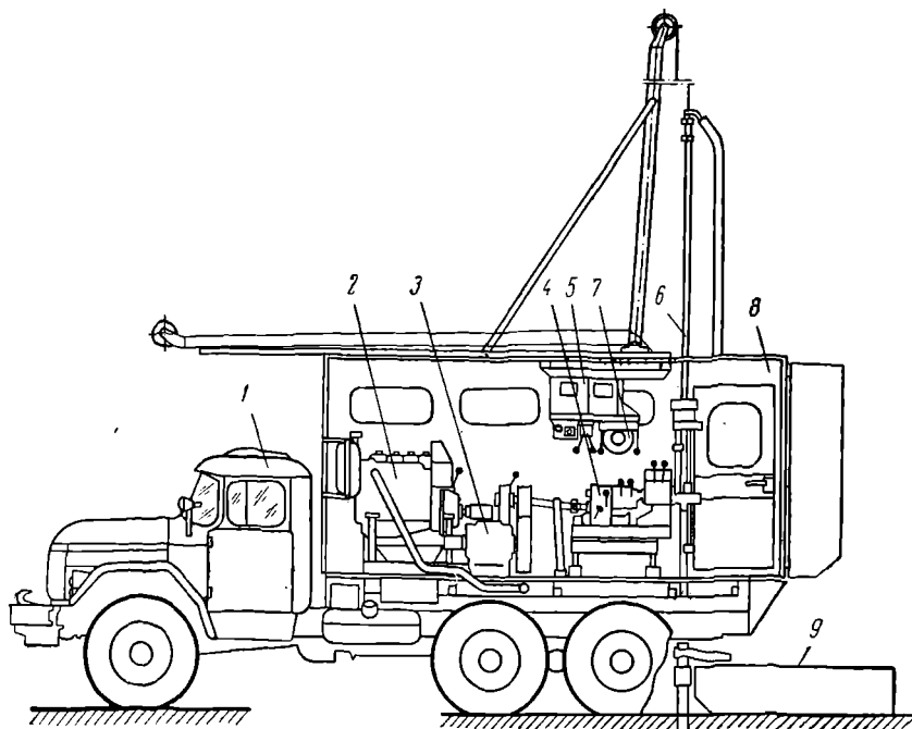
Рис. 67. Самоходная поисковая установка СПУ-100 (конструкции СКБ МГ СССР).
