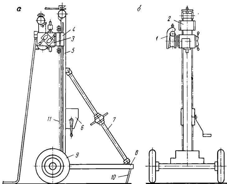
Рис. 65. Буровая установка УКБ-12/25 (конструкции СКБ МГ СССР).
