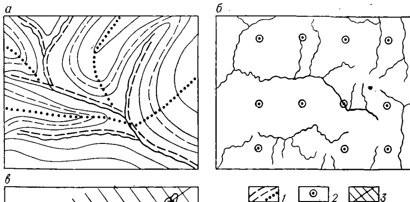
Рис. 51. Схемы расположения поисковых и геологосъемочных маршрутов (профилей) в различных условиях.
