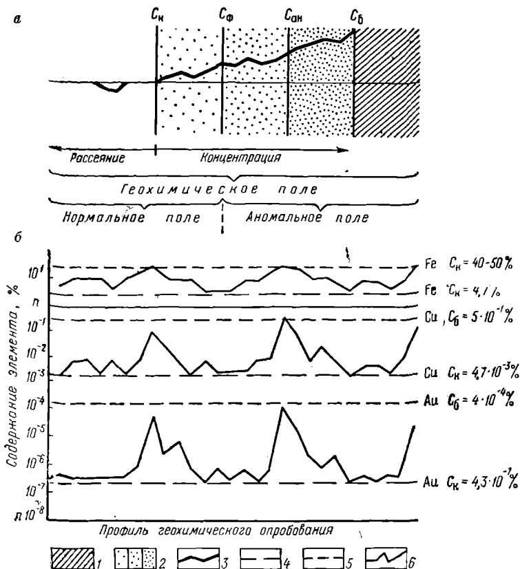
Рис. 28. Схема геохимического поля (а) и диаграмма контрастности геохимических аномалий (б).
