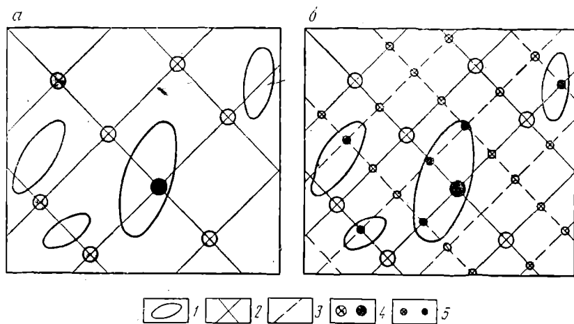
Рис. 53. Схема вероятности обнаружения объектов при различной плотности поисковой сети (а, б).
