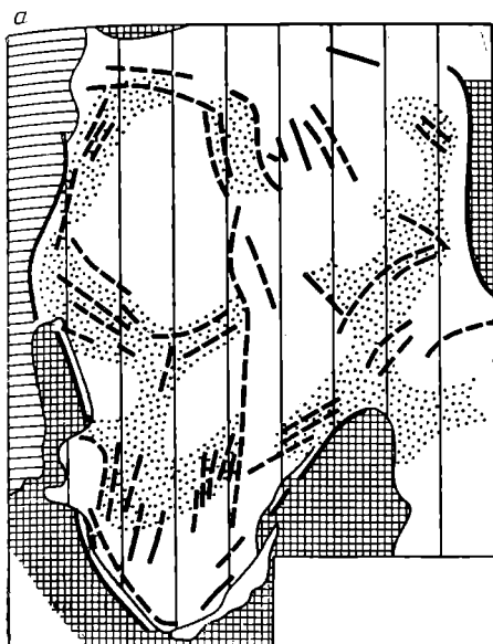
Рис. 17. Положение региональных проницаемых структур, контролирующих металлогенические провинции и зоны:
