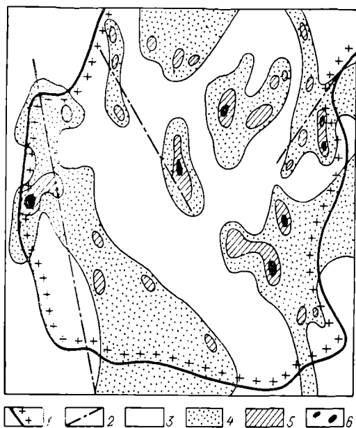
Рис. 58. Литогеохимическая карта площади интрузива.
