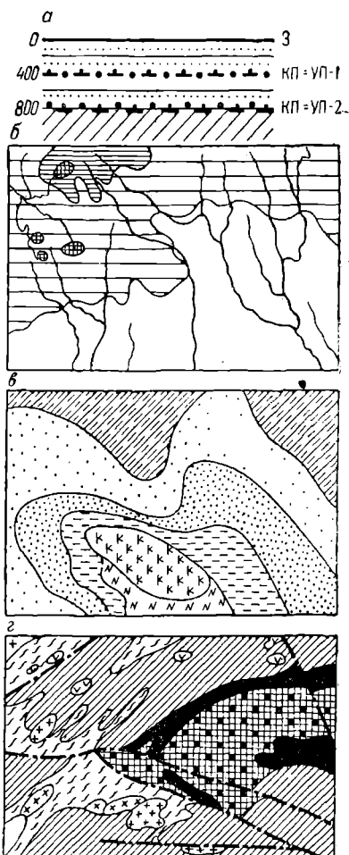
Рис. 43. Положение уровней прогнозирования в разрезе плит (а) и примеры прогнозных схем для разных уровней одного и того же района:
