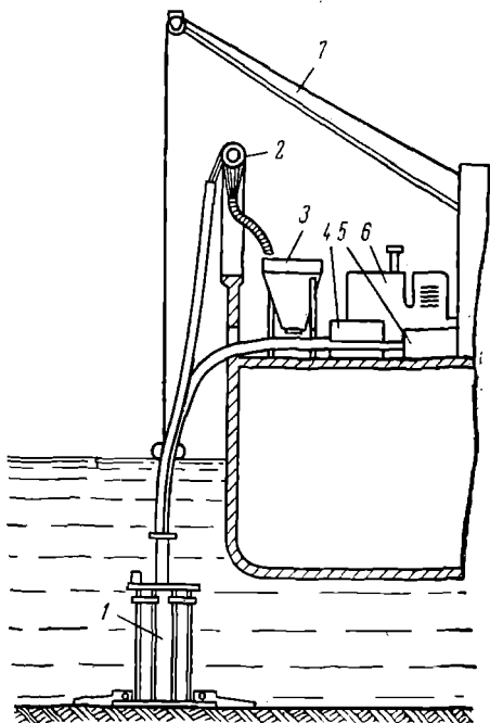
Рис. 68. Поисково-разведочная эрлифтная буровая установка на экспедиционном судне (по Б. А. Белову и др.).
