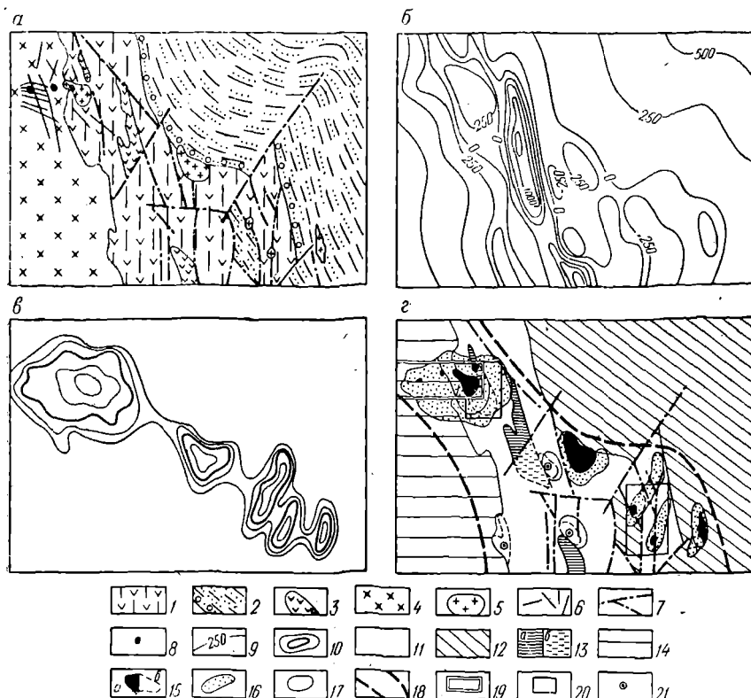
Рис. 41. Карты полей одного из рудных районов Забайкалья (составлены В. В. Аристовым, Л. Л. Ляховым, Б. Н. Королевым, И. Н. Кадыровым):
