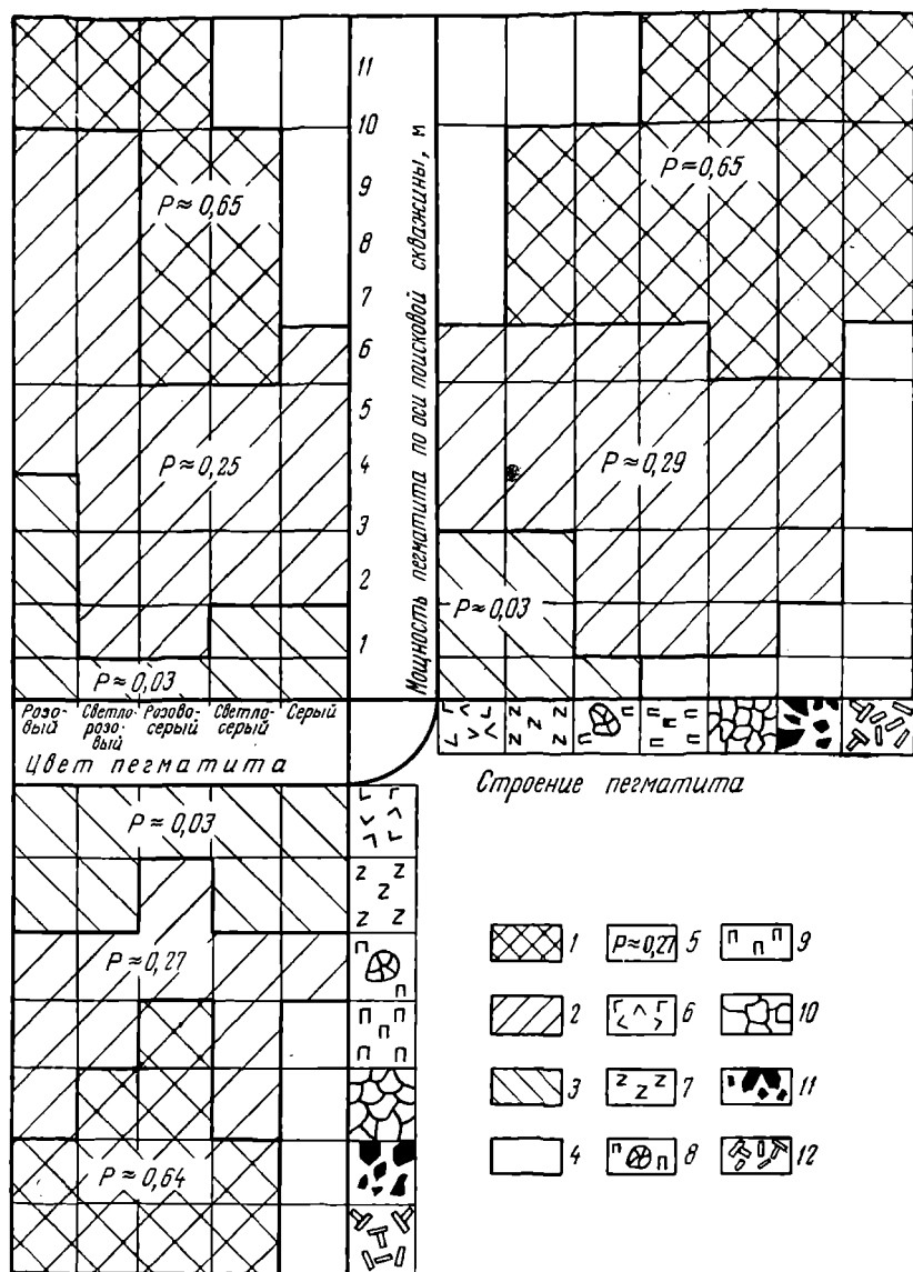
Рис. 76. Корреляционная диаграмма определения перспективности пегматитов по их ведущим оценочным параметрам (по В. И. Панченко и др.).
