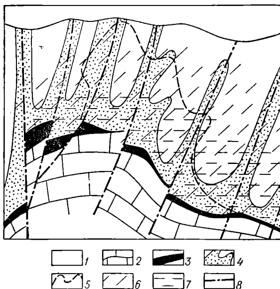
Рис. 33. Зональность эндогенных ореолов над месторождением сурьмы в разрезе (по Н. А. Никифорову).
