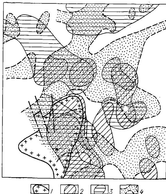
Рис. 31. Зональность эндогенных ореолов вольфрама, лития и фтора по отношению к гранитному интрузиву в плане (по И. Я. Смутьскому и В. В. Аристову).
