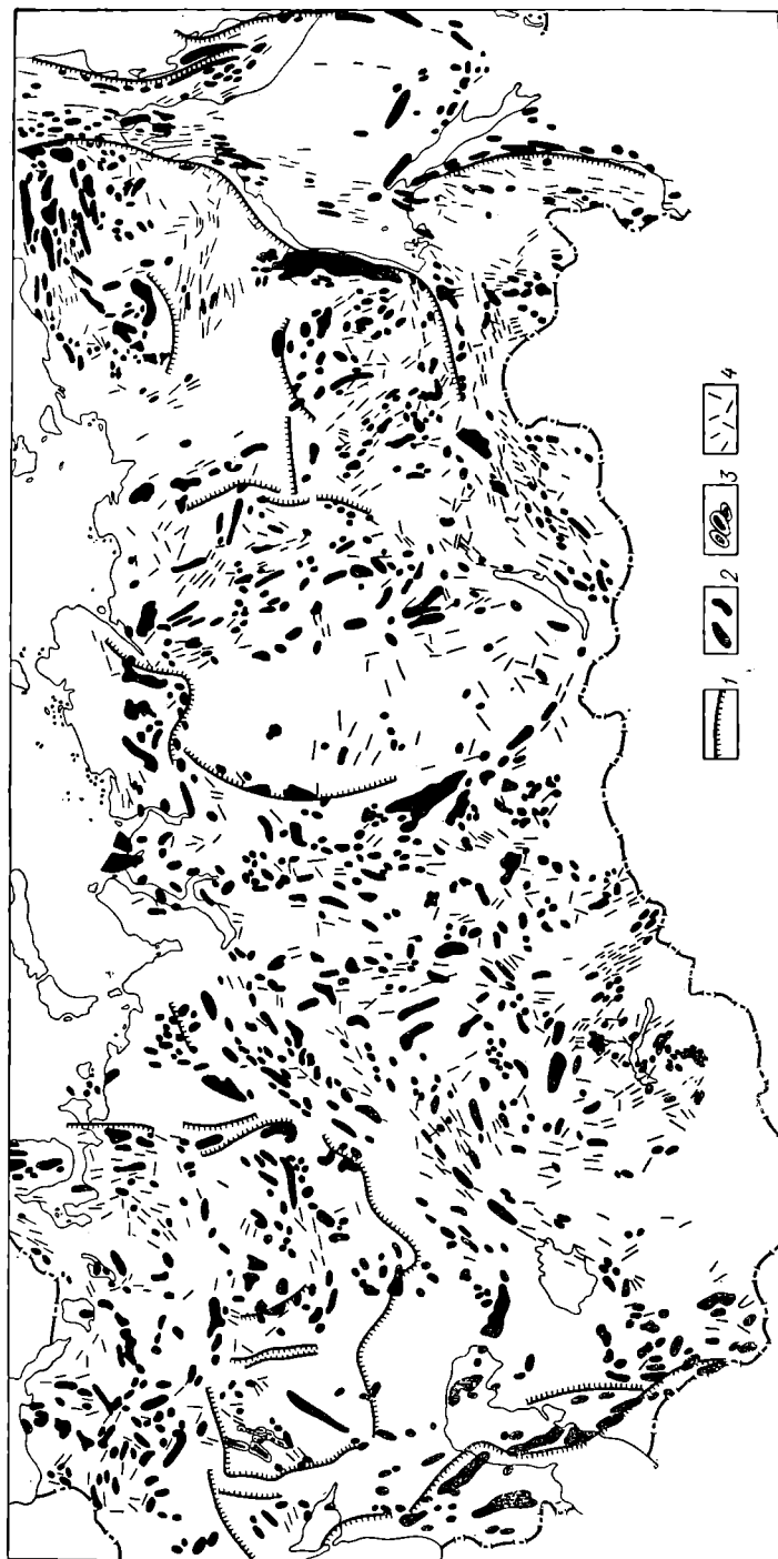
Рис. 40. Региональные геофизические поля территории СССР (по А. А. Борисову и др.). [20]) 1 — гравитационные ступени; 2 — относительно положительные магнитные аномалии; 3 — курские положительные магнитные аномалии; 4 — оси сравнительно мелких положительных магнитных аномалий
