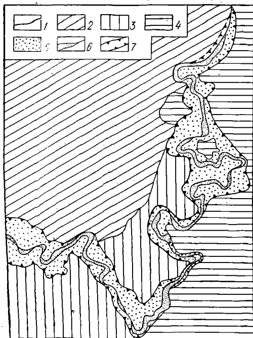
Рис. 39. Нормальное минералогическое поле рыхлых отложений бассейна р. Оленек (по Б. И. Прокопчуку и Э. Г. Сочневой).
