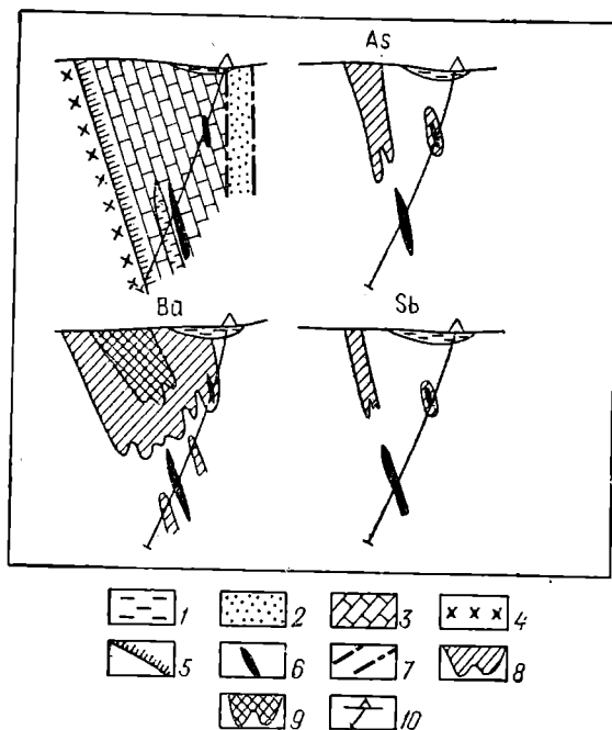
Рис. 32. Эндогенные ореолы мышьяка, бария и сурьмы в надрудной части сланцев свинцово-цинковых рудных тел (по Л. Н. Овчинникову, С. В. Григоряну и Э. Н. Баранову).
