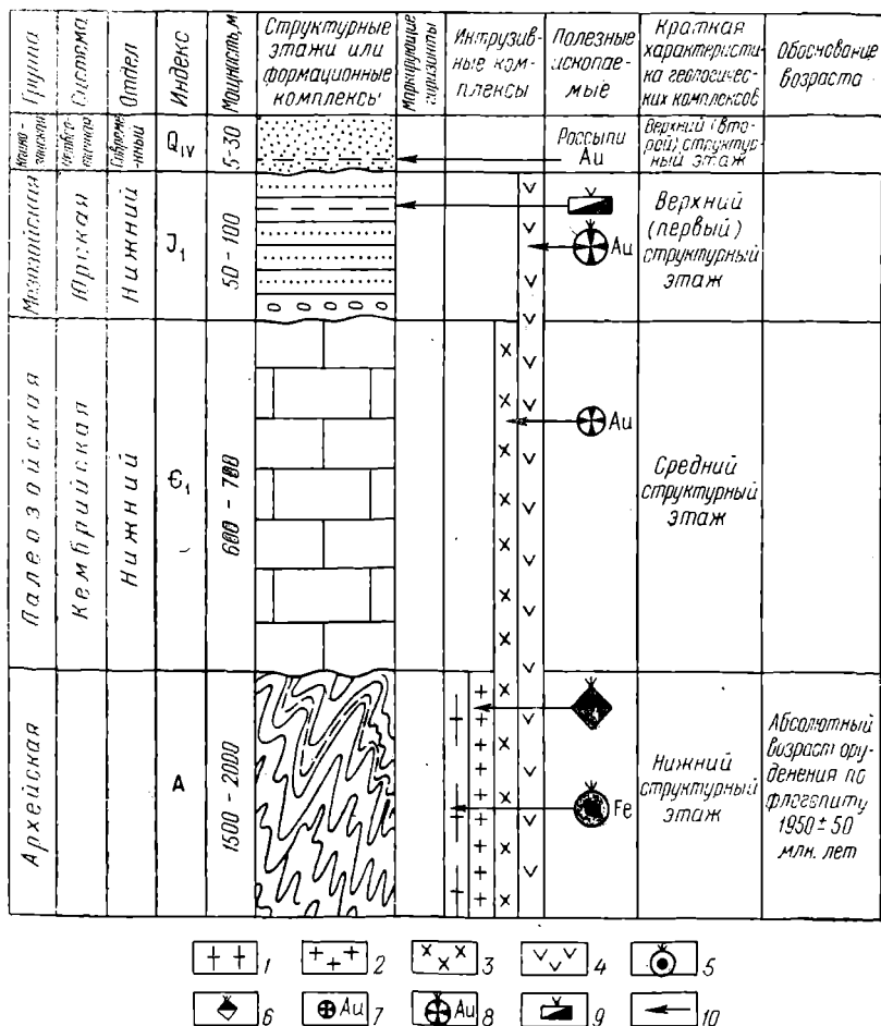
Рис. 12. Форма рабочей стратиграфической колонки.
