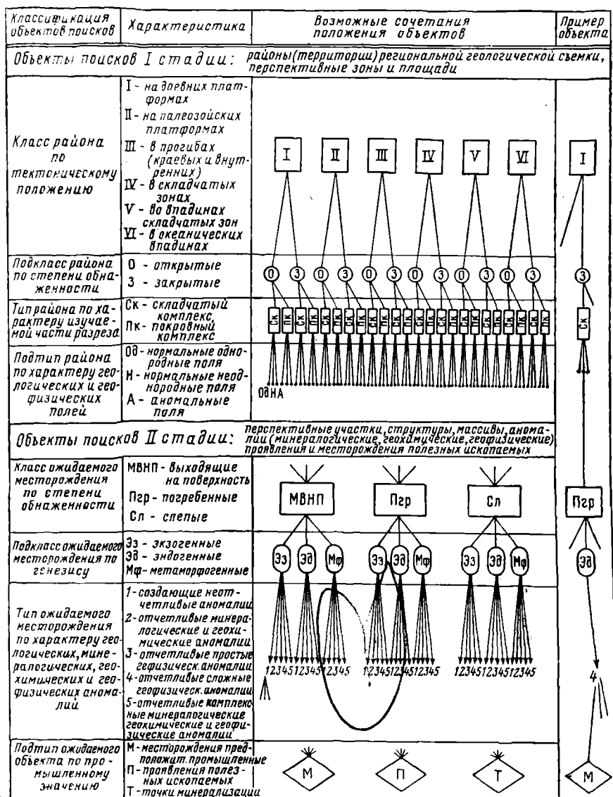
Рис. 6. Классификация объектов поисковых работ
