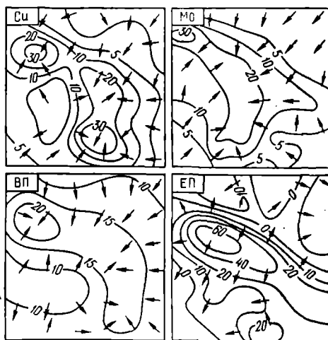
Рис. 5. Схемы сопоставления геохимических и геофизических полей на площади одного из меднопорфировых месторождений (по В. Ф. Мягкову и А. С. Работкину).
