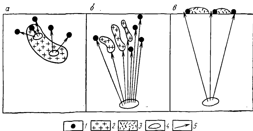
Рис. 22. Схема связи эндогенных месторождений с магматическими образованиями.
