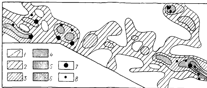
Рис. 7. Схема условной вероятности наличия месторождений (по В. Н. Землянову).
