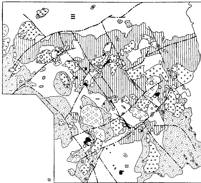
Рис. 23. Схема размещения магматических комплексов и связанных с ними медно-молибденовых месторождений в Северном Прибалхашье (по В. В. Аристову, Ю. К. Кудрявцеву, В. С. Попову).
