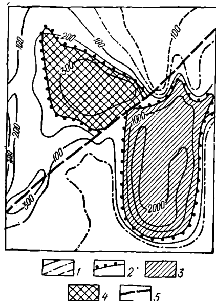
Рис. 48. Изменение интенсивности геофизических (магнитных) аномалий в зависимости от глубины залегания объекта (по А. М. Виноградову)
