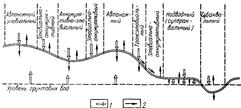
Рис. 70. Основные типы элементарных ландшафтов (по Б. Б. Полюнову с дополнениями М. А. Глазговской).
