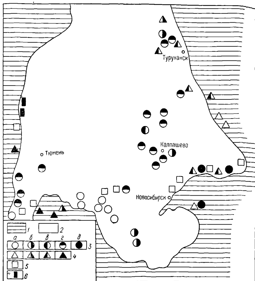
Рис. 21. Схема размещения экзогенных рудных скоплений в мезо-кайнозойских отложениях чехла Западно-Сибирской плиты (по В. П. Казаринову). 1 — континент в период образования руд; 2 — морской бассейн в тот же период; 3 — железные руды: а — средний олигоцен, б — эоцен — палеоцен, в — маастрихт, г — турон — сanton, д — апт — альб; 4 — бокситы: а — эоцен, б — сanton, в — апт — альб, г — апт; 5 — россыпи (средний олигоцен); 6 — марганцевые руды (палеоцен)
