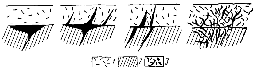
Рис. 25. Влияние экранирующих образований на формирование рудных тел различной морфологии.
