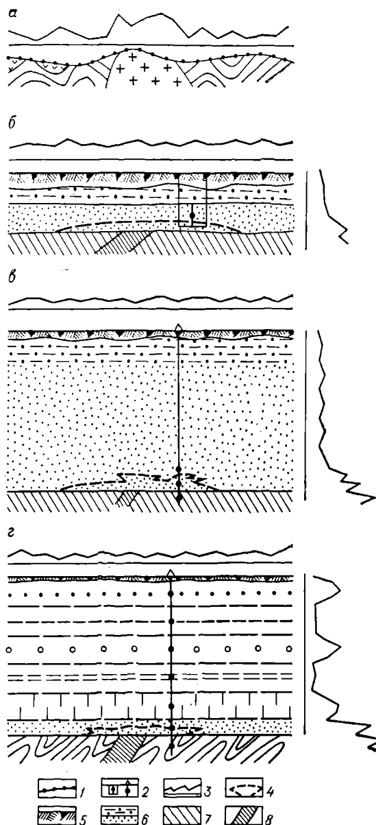
Рис. 56. Схемы литогеохимического опробования в различных условиях.
