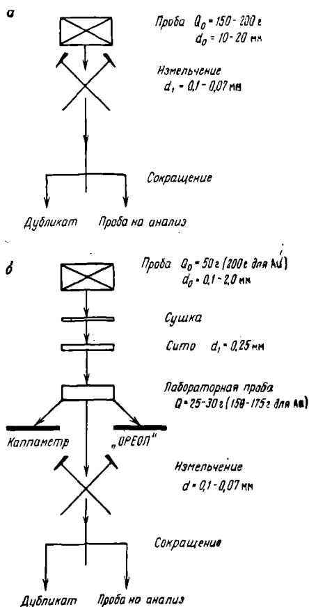
Рис. 57. Схемы обработки литогеохимических проб из коренных пород (а) и рыхлых отложений (б)
