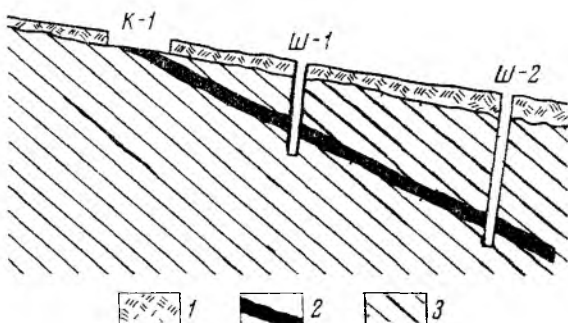
Рис 41. Вскрытие пологонаклоняющегося рудного тела канавой и двумя шурфами в одном поперечном разрезе (по П. П. Каллистову)
