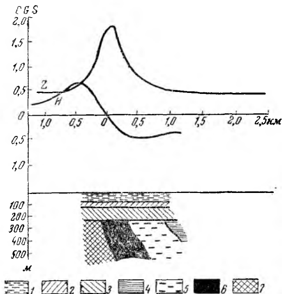
Рис. 24. Распределение магнитных сил над пластовыми железными рудами (по А. И. Заборовскому)
