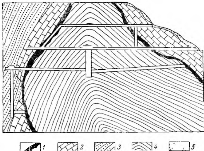
Рис. 70. Система разведки штольнями со слепыми шахтами (по П. М. Татаринову)
