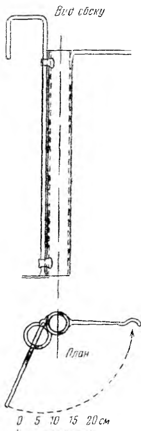
Рис. 91. Ручной пробоотборник системы Тихомирова и Коломенченко
