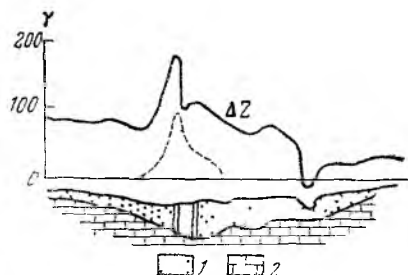
Рис. 29. Кривая \Delta Z над золотоносной россылью и кривая содержания магнетита (по А. А. Логачеву)
