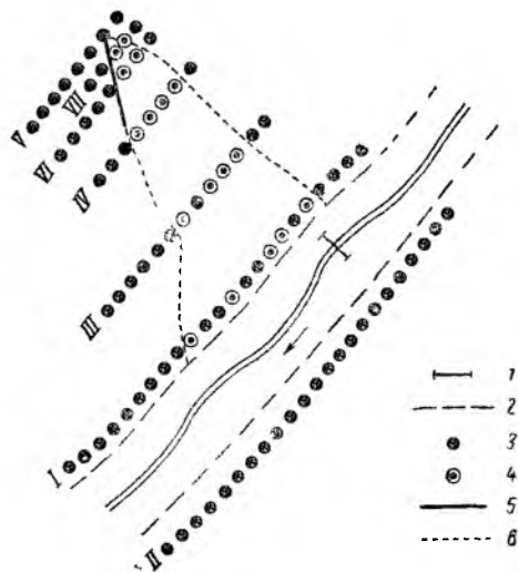
Рис. 14. Схема поисков делювиальной россыпи и коренного месторождения (по Д. В. Воскресенскому)
