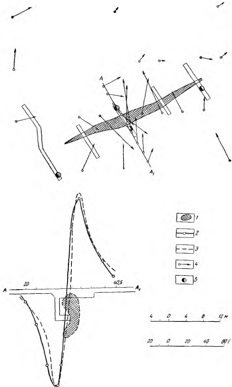
Рис. 27. Результаты гравипроводочных работ и геологический план рудного тела, открытого гравипроводкой (по В. А. Андрееву) 1 — контур рудного тела, 2 — наблюдаемая кривая градиента, 3 — теоретиче-
