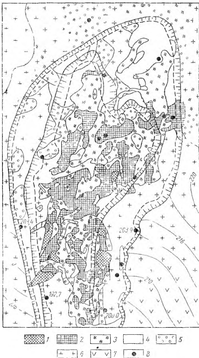
Рис. 116. План карьера на железорудном месторождении (по М. Н. Альбову)
