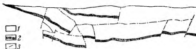
Рис. 30. Схематический разрез участка месторождения Мир-галимсай (по материалам рудничной документации)
