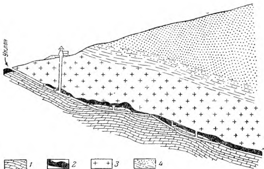
Рис. 72. Система вертикальных шахт, пересекающих пологие рудные зоны, с штреками, восстающими и уклонами (месторождение Ледвилль, Колорадо)
