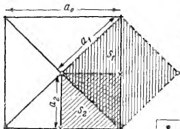
Рис. 56. Сгущение разведочной сети способом конверта
