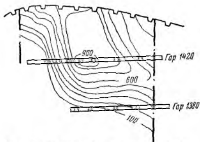
Рис. 109. Изображение флюоритовой залежи в изолиниях метропроцента в проекции на среднюю плоскость залежи
