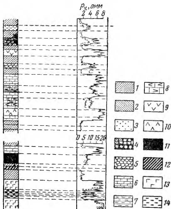
Рис. 62. Кривые кажущегося сопротивления зарегистрированные микрозондом малого размера (точечная кривая) и микрозондом большого размера (сплошная кривая). По В. Н. Дахпову.
