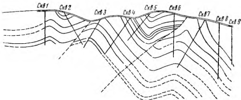
Рис. 65. Разрез по разведочной линии Осиповского месторождения Кузнецкого бассейна (канавы вкрест простирания и серия колонковых скважин с различным углом наклона)
