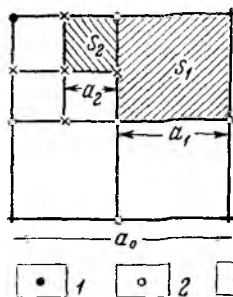
Рис. 55. Сгущение разведочной сети с уменьшением расстояния между выработками вдвое
