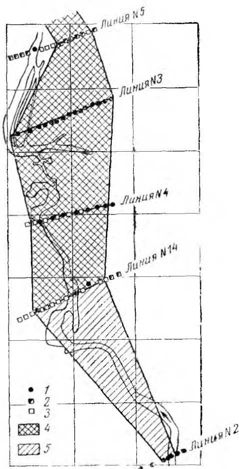
Рис. 64. Система разведки россыпи мелкими вертикальными скважинами (по В. И. Смирнову)
