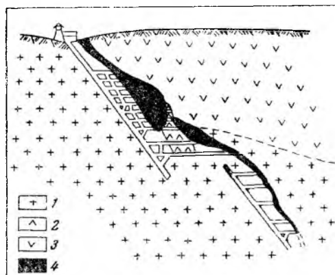
Рис. 73. Система разведки наклонной шахтой с кварцлагамми (рудники Крейтон, Сёдберри)
