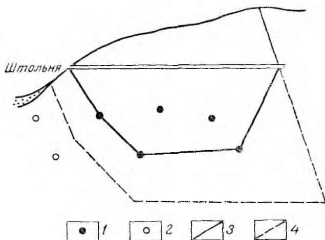
Рис. 49. Оконтуривание крутопадающего тела полезного ископаемого в проекции на вертикальную плоскость
