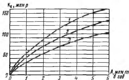
Рис. 110. Зависимость общей суммы капитальных затрат от годовой производительности (по руде) горнорудных предприятий цветной металлургии для трудных (1), средних (2) и легких (3) условий строительства
