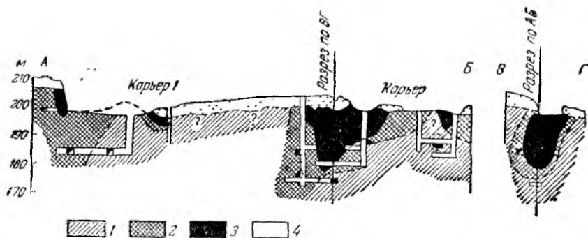
Рис. 68. Система шурфов с рассечками на месторождении Семиз-Бугу (по П. М. Татаринкову)
