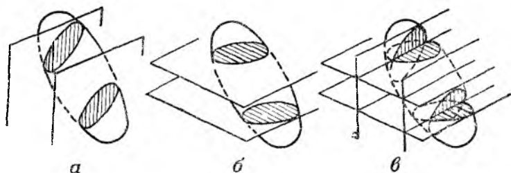
Рис. 46. Основные виды разведочных разрезов
