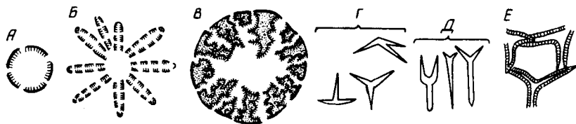
Рис. 13. Строение водно-иригационной системы (А–В) и спикул (Г–Е) губок: А–В – поперечные разрезы известковых губок с асconoидной (А), сикonoидной (В) и лейконоидной (В) иригационными системами; Г – трирадиата; Д – диапoзонные спикулы (видоизмененные трирадиаты); Е – фрагмент скелета современных губок под микроскопом (видно сочленение трирадиат)
