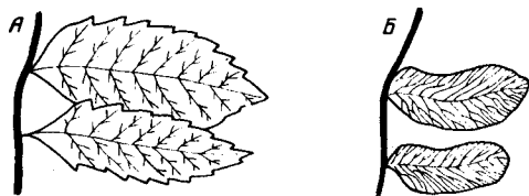
Рис. 74. Папоротниковидные листья, классифицируемые искусственно:
