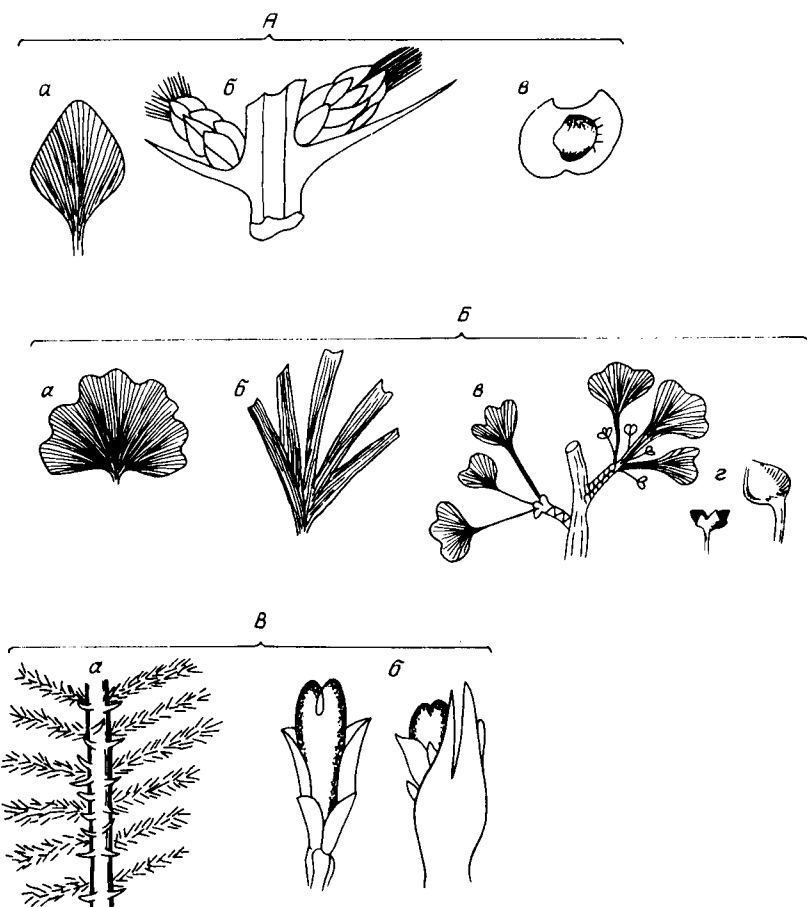
Рис. 76. Представители различных порядков подкласса Phyllospermidae: А — кордаитовые (Cordaiales):
