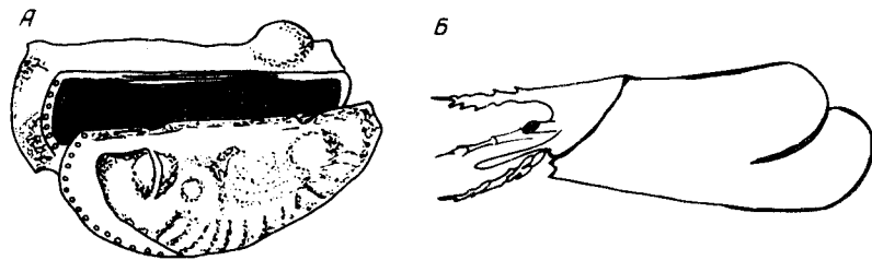
Рис. 31. Представители ископаемых (А — покрытая сложной скульптурой раковина рода Betrychia с раздвинутыми створками) и современных (Б) остракод
