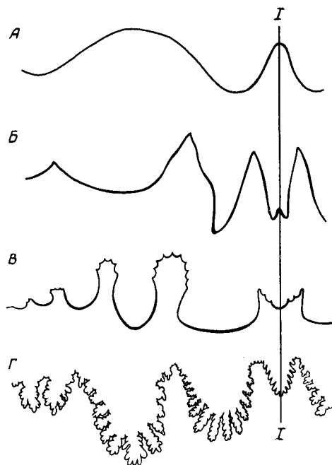
Рис. 41. Типы перегородочных линий аммоидей:
