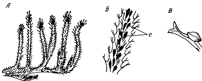
Рис. 71. Представитель протолепидодендроновых Protolipidodendron scharyatum : А — реконструкция внешнего облика растения; Б — лист (филлоид), несущий спорангии (с); В — поверхность части стебля
