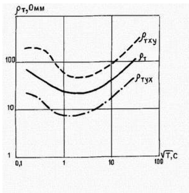
Рис. 32. Кривые МТЗ над неоднородной средой
