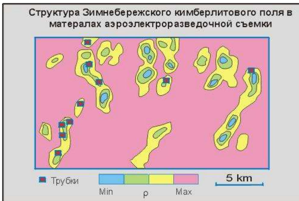
Рис. 28. Данные аэроэлектроразведки.
