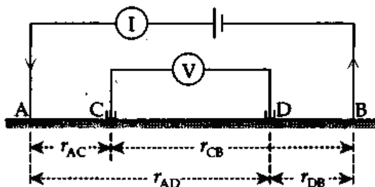
Рис. 21. Основная четырёхэлектродная установка измерения удельного сопротивления, состоящая из пары электродов (А,В), и из пары электродов для измерения потенциала (С,Д).
