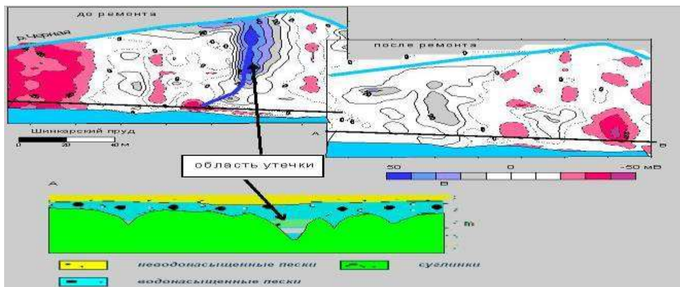
Рис. 19. Геоэлектрический разрез вдоль дамбы по результатам зондирования.
