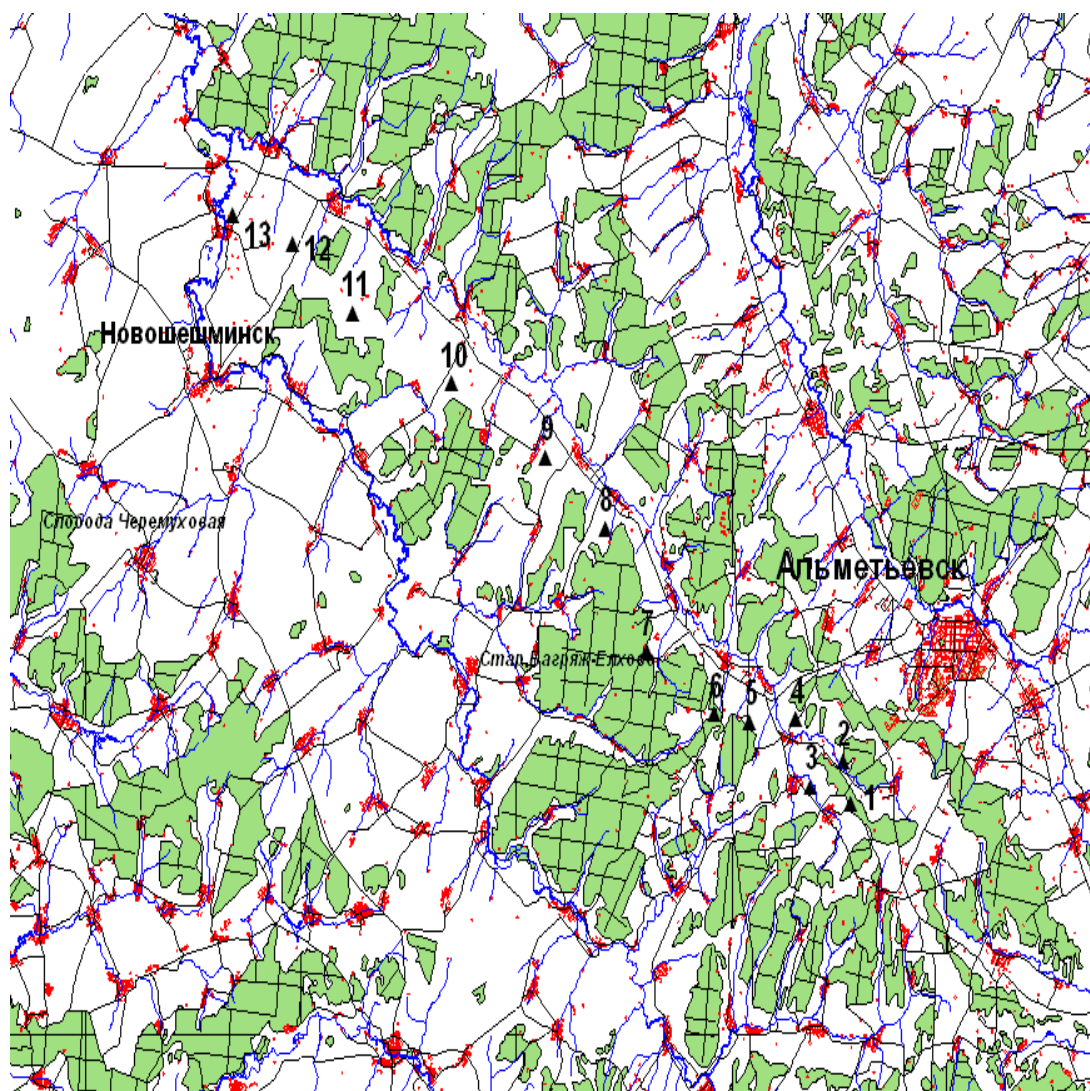
Рис. 6. Расположение точек наблюдений методом МТЗ.
