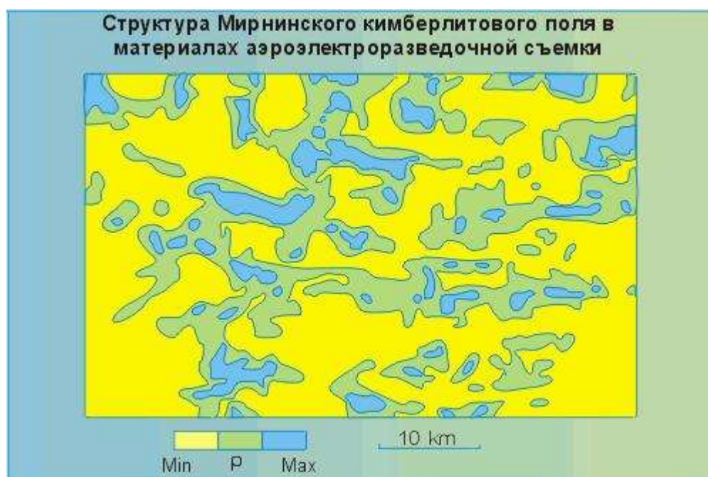
Рис. 27. Данные аэроэлектроразведки.
