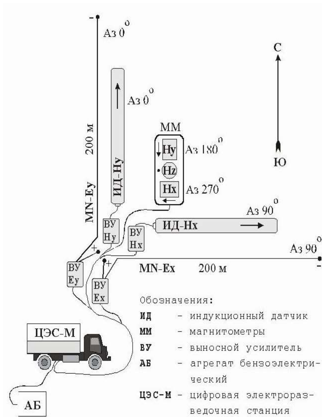
Рис. 33. Схема установки.
