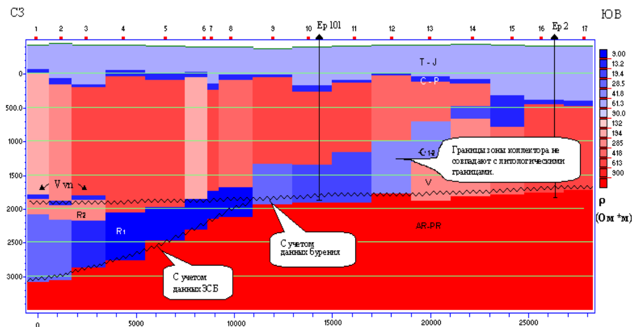
Рис. 35. Геоэлектрический разрез ( результаты послойной интерпретации ) по профилю 310 Ерминской площади, с учетом данных глубокого бурения.
