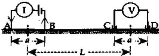
Рис. 22. Специальные электродные конфигурации.
