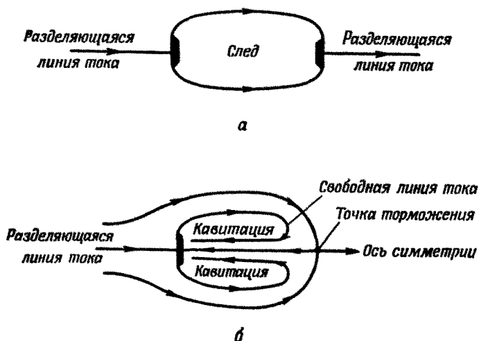
Рис. 15. а — течение Рябушинского; б — возвратная струя.
