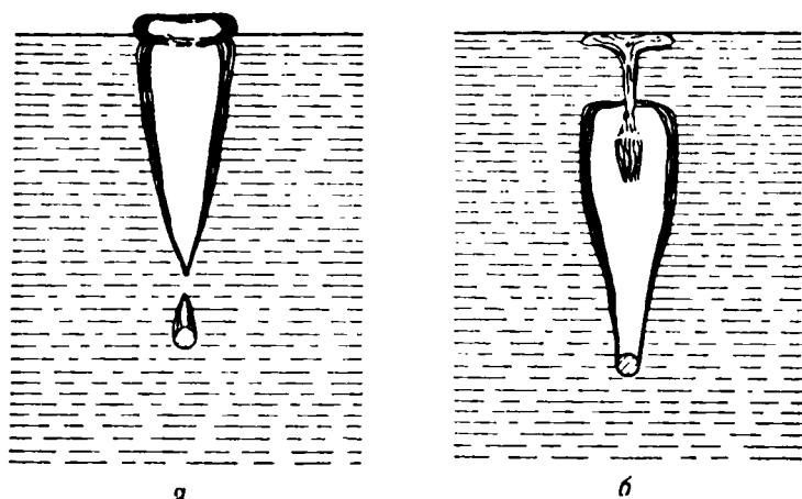
Р и с. 22. а — глубинное смыкание; б — поверхностное смыкание.
