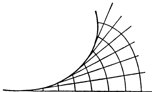
Рис. 26. Координаты для волны разрежения Прандтля — Мейера.
