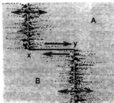
Рис. 7.26. Иллюстрация образования трансформного разлома [1].
