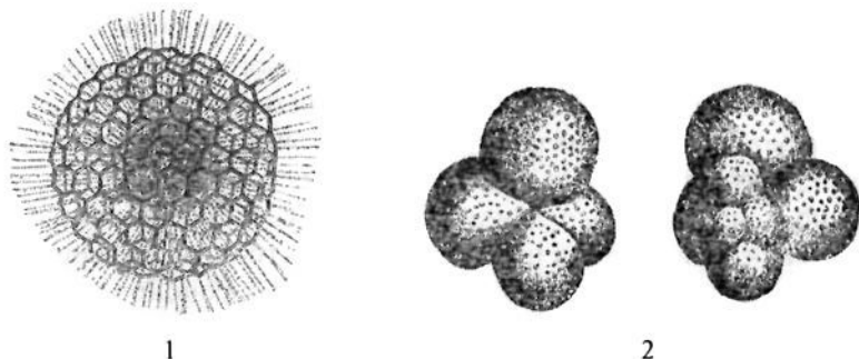
Рис. 7.9. 1 – Радиолария современная (по Бючли и Рюсту из книги М. Неймайра. История земли. Т.2, 1903). 2 – Глобигерина (по Н.Н. Яковлеву, 1932).
