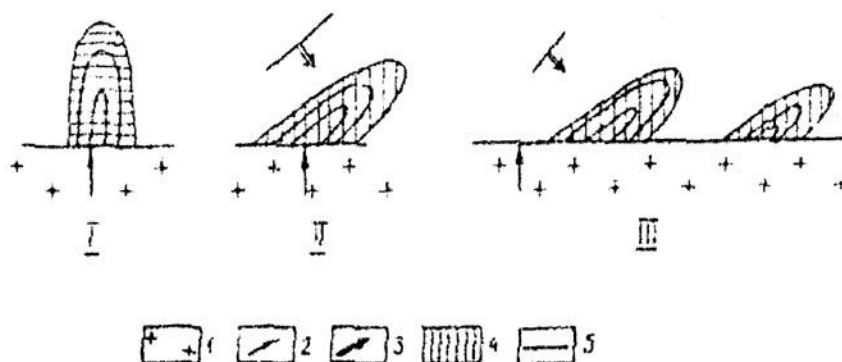
Рис.7.8. Формирование группового характера перемещения наносов.
