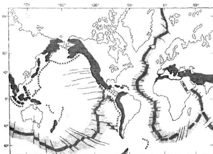
Рис. 7.27. Главные элементы земной коры [1].
