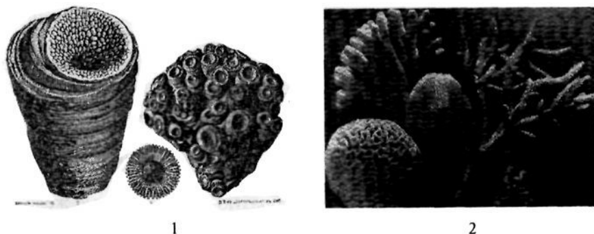
Рис. 7.10. 1 – Силурийские и девонские кораллы (из книги М. Неймайра. История земли. Т.2, 1903). 2 – Современные рифообразующие кораллы [2].
