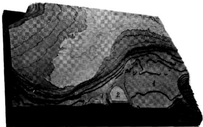
Рис. 7.21. Макет южной окраины материка близ восточного побережья США (по К. Эмери, 1965 [4 доп.]).
