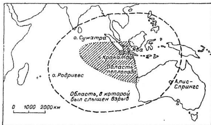
Рис. 7.29. Взрыв вулкана Кракатау в 1883 г. [3].
