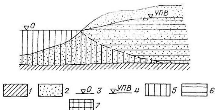
Рис. 7.23. Взаимоотношение морских и пресных вод на морских побережьях [5 доп.].
