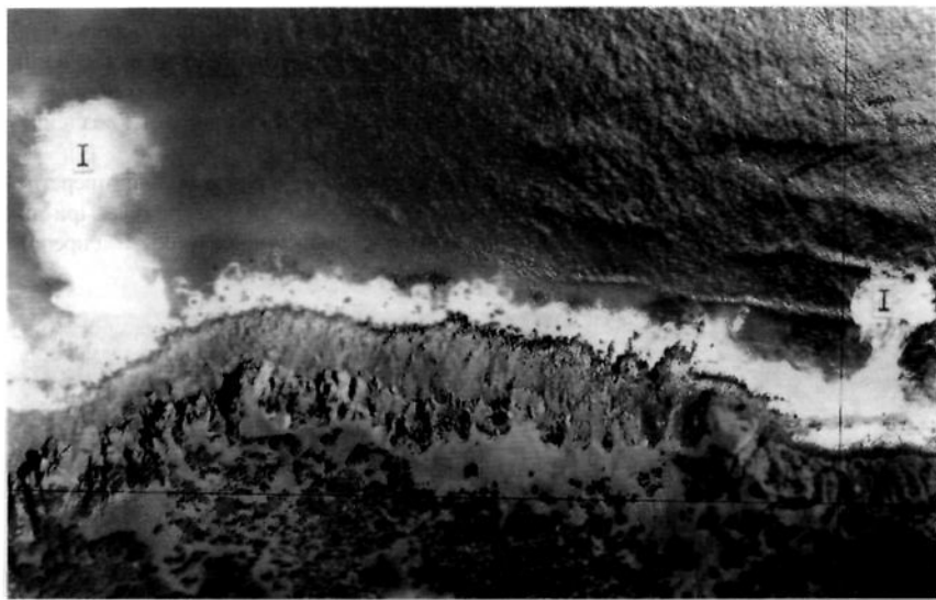
Рис. 7.4. Аэрофотоизображение разрывных течений (I).
