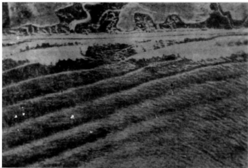
Рис. 7.5. Аэрофотоснимок рефракции волн у берега с постепенным нарастанием глубин.
