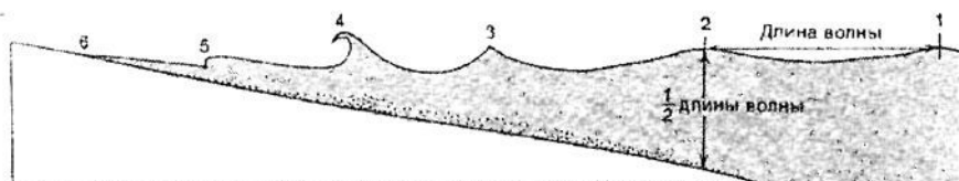
Рис. 7.3. Схема образования прибоя и бурунов [1].
