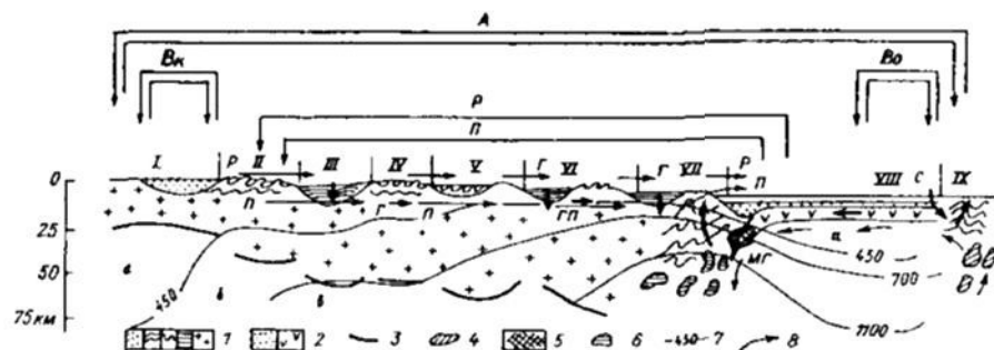
Рис. 6.3.2. Общая схема основных циклов круговорота воды на Земле.
