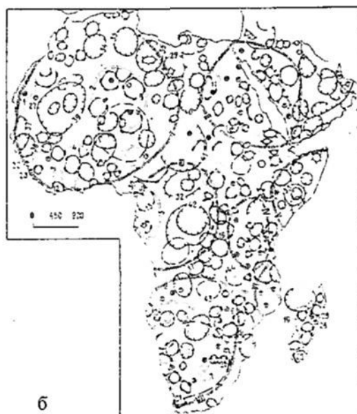
Рис. 6.1.7. Расположение нуклеаров на континентах (а) и кольцевых структур Африкано – Аравийского региона (б) (условные обозначения не приводятся).
