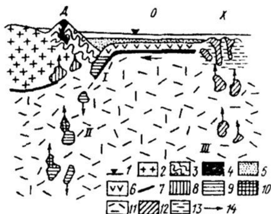
Рис. 6.3.1. Схема обновления океанического дна и процесс преобразования базальта в эклогит (по Х. Хессу, в интерпретации А. Э. Рингвуда и Д. Х. Грина [1968 г.]). 1 – уровень океана; 2 – континентальная кора; 3 – складчатость геосинклинали; 4 – вулканы с андезитовой лавой; 5 – осадочный и базальтовый слой; 6 – океанический слой; 7 – граница Мохо; 8 – интрузии магм кислого и среднего состава; 9 – эклогит; 10 – андезитовая магма; 11 – мантия (пиролит); 12 – базальтовая магма; 13 – остаточный перидотит; 14 – направление движения океанического дна, блоков эклогита и образующихся магм. I – III – зоны: I – перехода базальта в эклогит, II – погружающихся блоков эклогита, III – частичного плавления пиролита. Д – островная дуга; О – океан; Х – срединно-океанический хребет.
