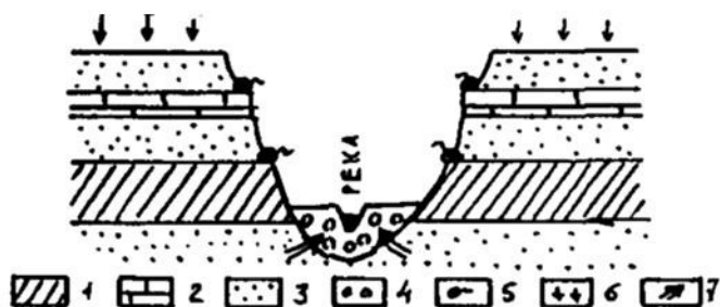
Рис. 6.1.3. Иллюстрация речной долины в разрезе.
