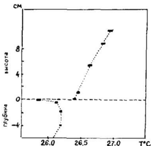
Рис.6.1.1. Изменение температуры воды и воздуха вблизи поверхности океана (по А.В.Шумилу, 1976). Длина черточки определяет предел колебаний температуры за время измерений (приблизительно 1,5 мин).
