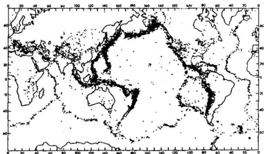
Рис. 6.1.6. Сейсмическая активность Земли за период с 1962 по 1974 г.
