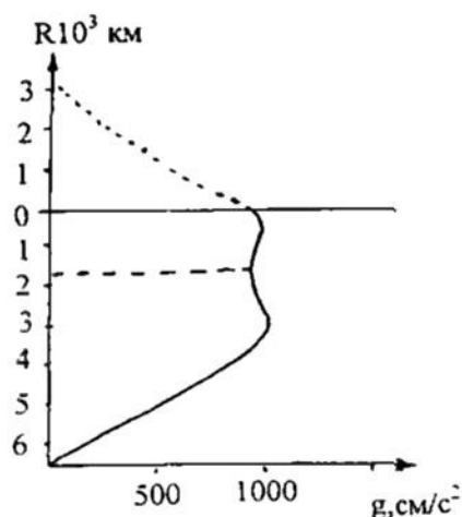
Рис. 6.2.5. Изменение ускорения свободного падения ( g, \text{cm/s}^2 ) на планете Земля.
