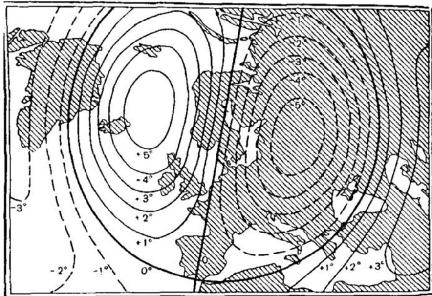
Рис. 6.4.2. Теоретическая схема термобарических сейш (по В.В. Шулейкину).
