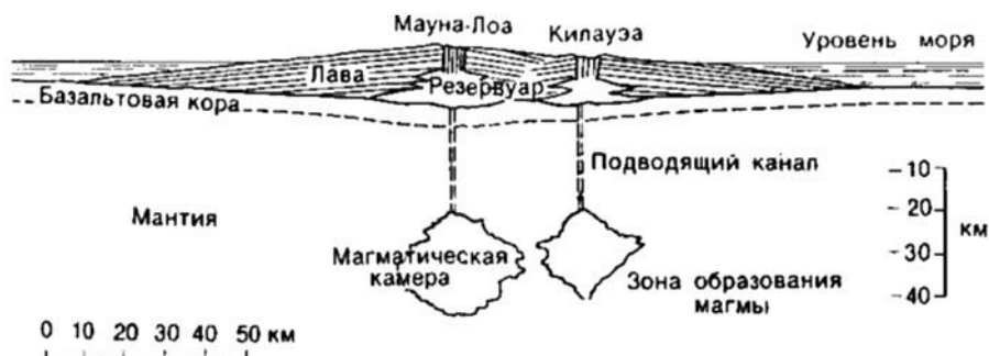
Рис. 6.1.4. Гипотетический разрез через вулканы Мауна-Лоа и Килауэа на Гавайях.
