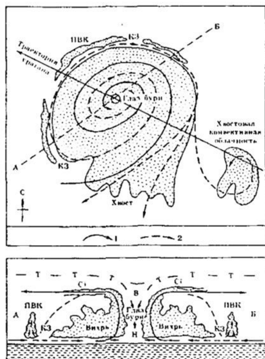
Рис. 6.1.2. Схематическая модель тропического циклона [по М.А. Герману, 1975].
