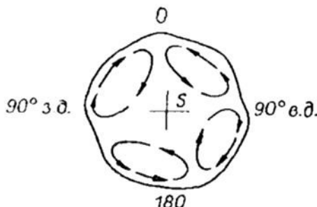
Рис. 6.4.1. Схематический разрез геоида по экватору со стороны южного полюса. Стрелками показана конвекция в верхней мантии.
