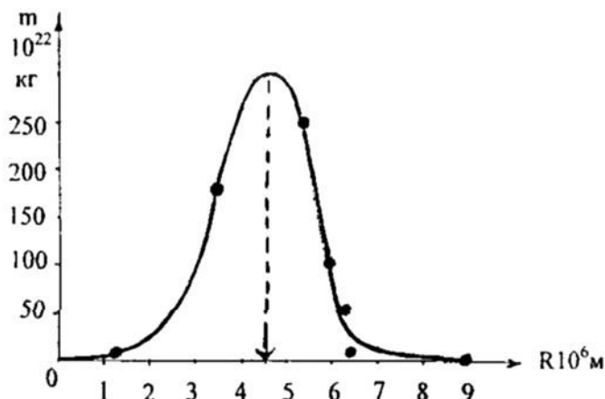
Рис. 6.2.4. Геосферный цикл Земли.
