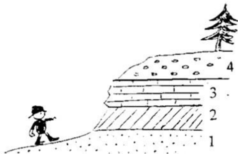
Рис. 5.1.1. Схема обнажения горных пород.
