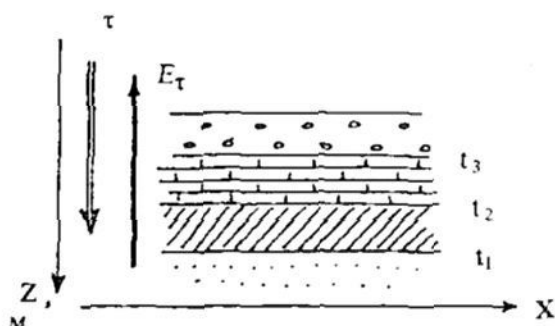
Рис. 5.5.1. Схема взаимоотношения прошлого и будущего.
