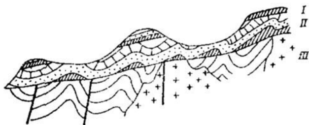
Рис. 5.6.2. Выделение структурных этажей.
