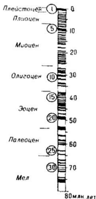
Рис. 5.4.1. Хронологическая геомагнитная шкала.
