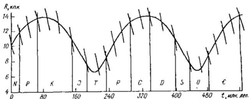
Рис. 6.2.2. Изменение расстояния Солнца от центра Галактики во времени (по А. Баренбауму, 2002).
