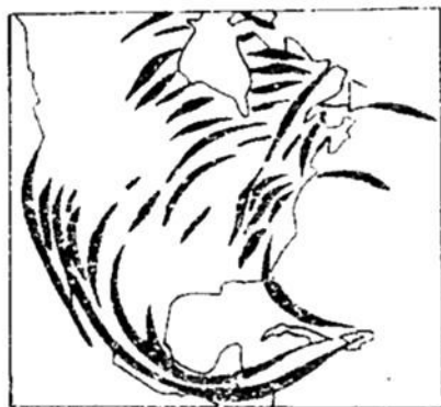
Рис. 6.4.4. Схема сочетаний складчатых зон Северной Америки.
