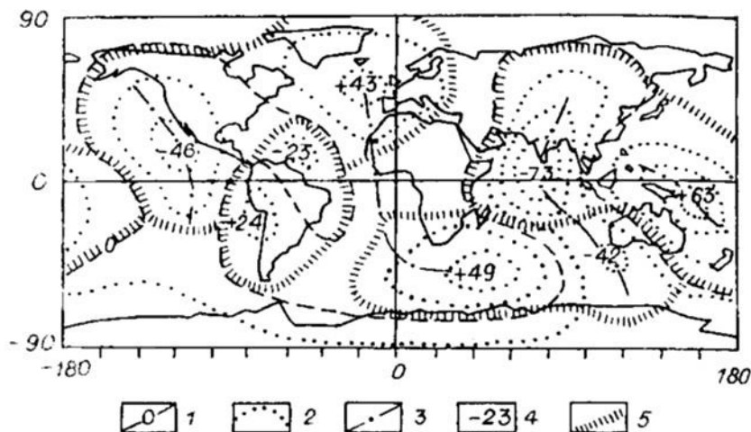
Рис. 6.4.3. Карта высот геоида с деталями тектоносферных тепловых машин первого и второго родов (по А.Н. Павлову, 1990).
