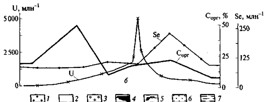
Рис. 6.77. Поперечный разрез неокисленного рудного тела района Хайленд (a) и распределение содержаний урана и сопутствующих элементов (б) (по Д. Дэвису):
