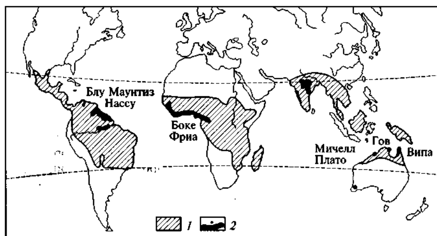
Рис. 6.17. Бокситоносные пояса и месторождения мира (по В.И.Синякову, 1994):
