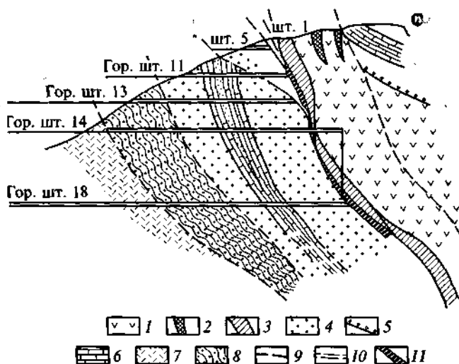
Рис. 6.42. Схема строения месторождения Чаган-Узун (по В. А. Кузнецову, А. Н. Оболенскому и др.):
