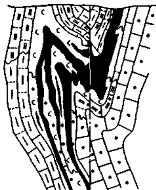
Рис. 6.31. Строение главного рудного тела Горевского месторождения (по В. В. Кузнецову, В. Г. Пономареву и др., 1990):
