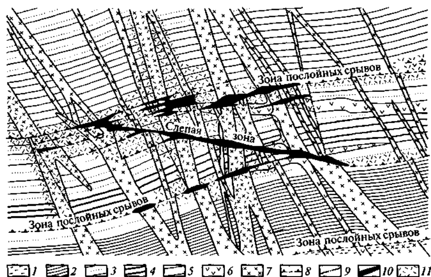
Рис. 6.73. Морфология и структура рудных тел Ишимского месторождения (по В. И. Казанскому, Н. П. Лаврову, 1974):
