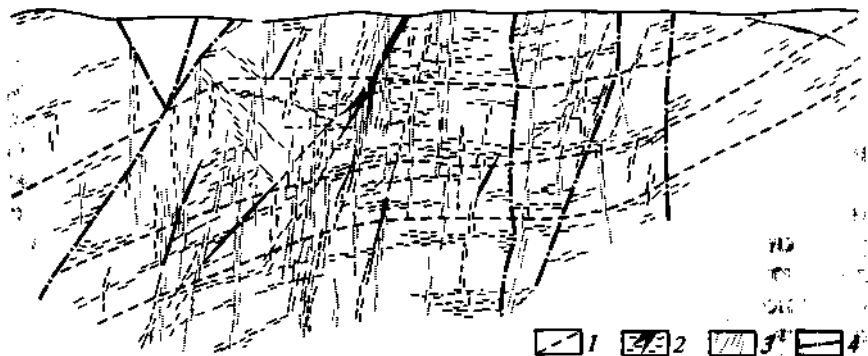
Рис. 6.64. Рудный штокверк Мурунтау (по С.Д. Шеру):
