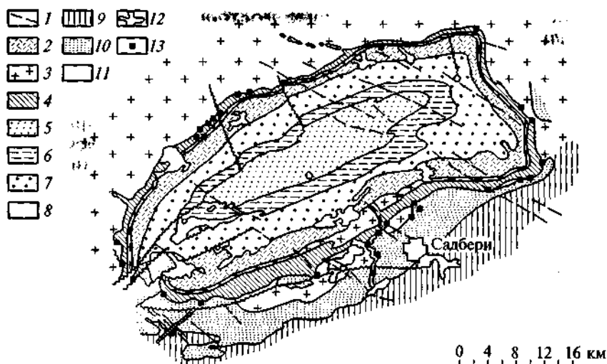
Рис. 1.1. Геологическая карта бассейна Садбери (по А.Д.Надретту):
