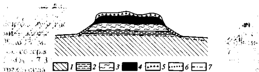
Рис. 6.18. Схема строения месторождения латеритных бокситов Гвиней (Западная Африка) (по В. И. Синякову, 1994):
