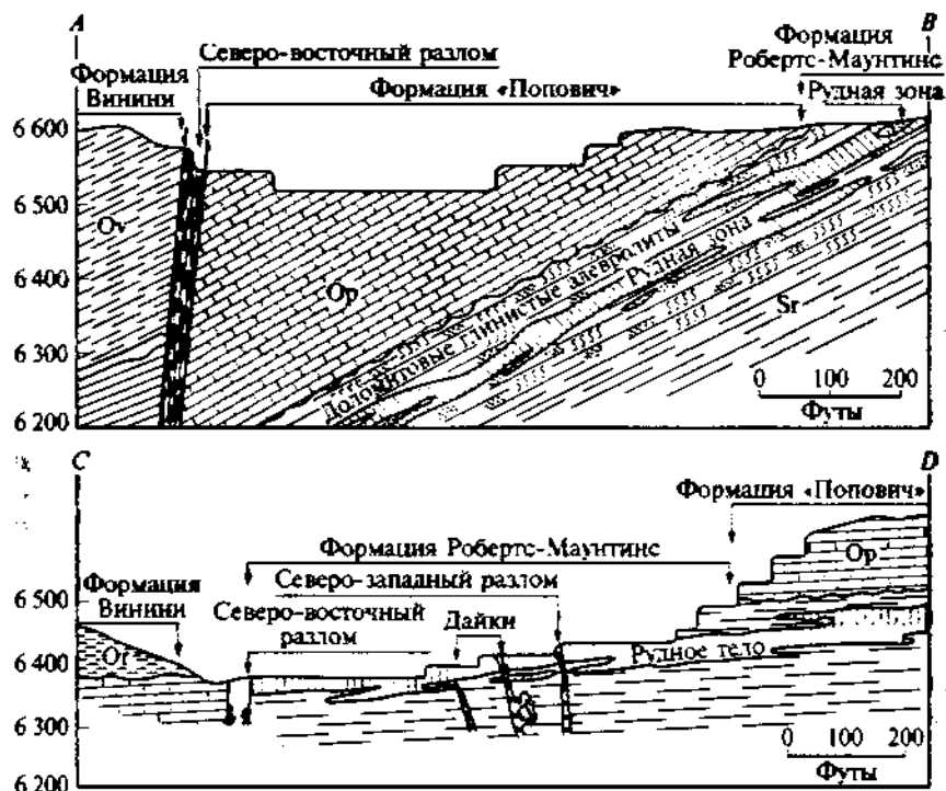
Рис. 6.62. Месторождение Карлин. Поперечные разрезы Главного рудного тела (по Хауссену, Керру, 1973) (цит. по: Ю. И. Бакулин и др., 2001)
