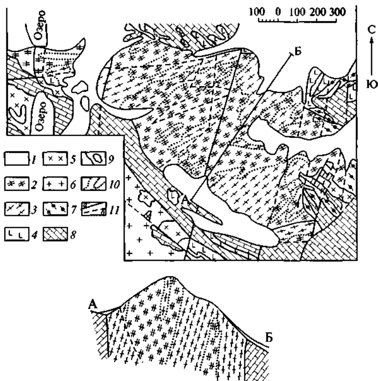
Рис. 6.53. Схематическая геологическая карта и разрез Улут-Танзекского месторождения (составлены с использованием данных разведочных работ) (по В.В. Рябцеву и др., 2006):
