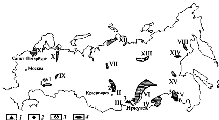
Рис. 7.10. Схема магнетитоносности России (по А. И. Шевелеву, 2001):
