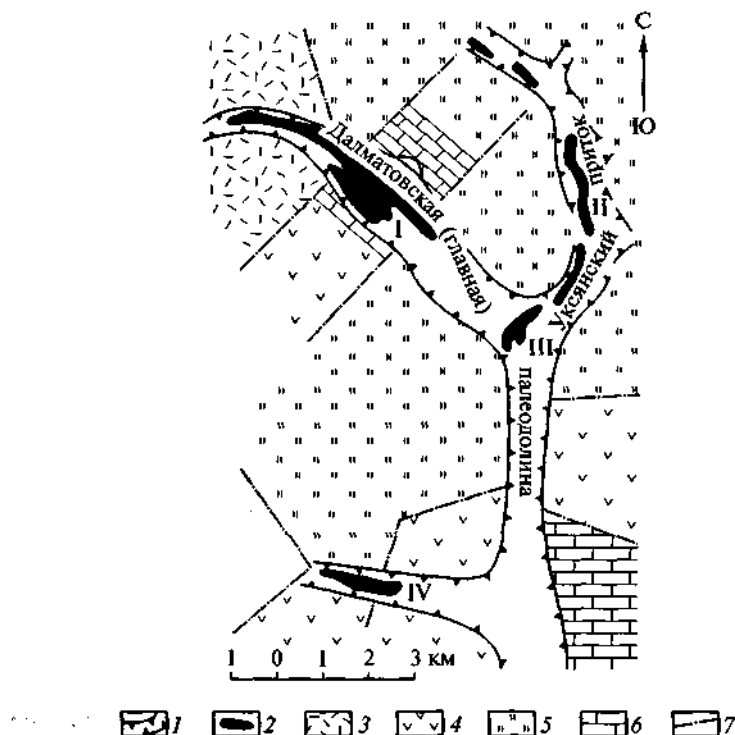
Рис. 6.80. Схематическая геологическая карта фундамента Далматовского месторождения с контурами позднеюрских речных долин и рудных залежей (по А. Б. Халезову, С. Н. Маркову, 2003):
