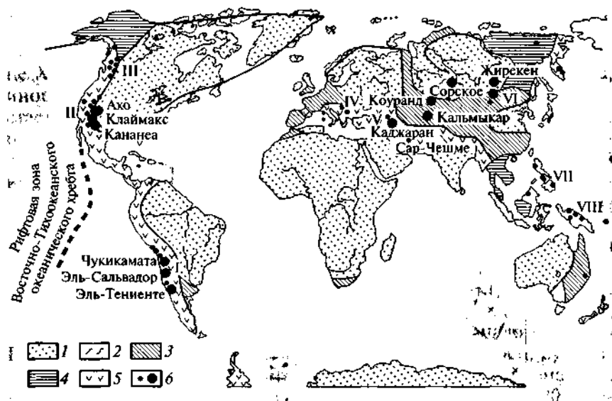
Рис. 6.39. Размещение молибден-порфировых и медно-молибден-порфировых месторождений мира (по В. И. Синякову):
