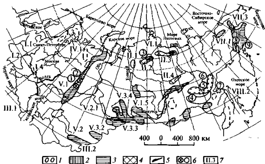
Рис. 6.71. Схема провинций и районов распространения россыпей платиновых металлов в России и других стран СНГ (по А. Н. Мочалову, 2004 г.):
