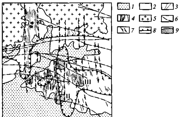
Рис. 6.35. Схематическая геологическая карта Пыркаайского оловорудного узла (по Б. В. Макееву, А. Б. Павловскому и др., 1988):
