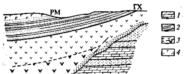
Рис. 6.11. Схема залегания хромитовых горизонтов в Критической зоне Бушвельдского доломита (составлено по Ю. Камерону):
