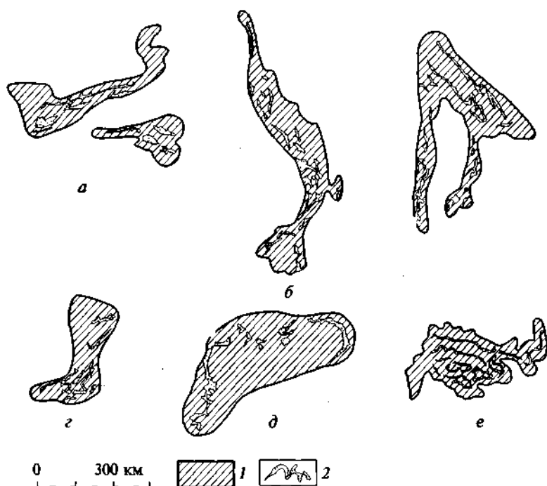
Рис. 6.2. Сравнение площадей распространения раннепротерозойских железисто-кремнистых формаций крупнейших железорудных провинций докембрия (по В. И. Синякову, 1994):
