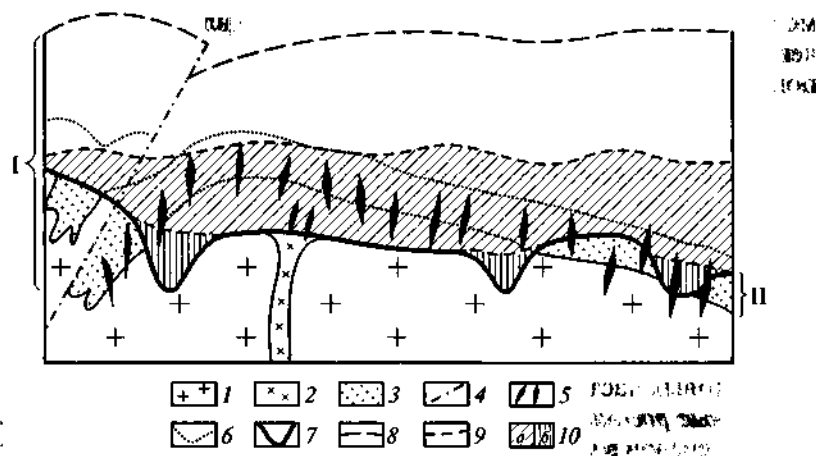
Рис. 2.2. Развитие эрозии в рудно-россыпном районе в условиях блоковой тектоники (по Н. Г. Патык-Кара, 1981):
