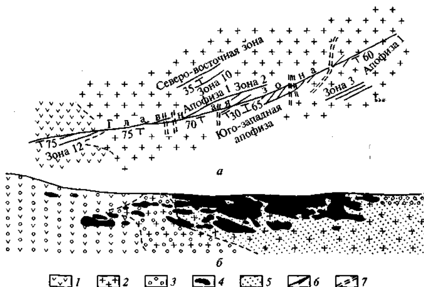
Рис. 1.9. Схема строения скарнового месторождения Чорух-Дайрон (по Б. В. Кристальному):
