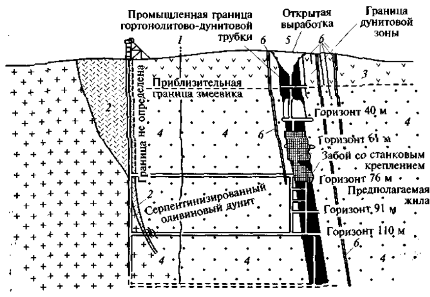
Рис. 6.69. Разрез через Мойхукскую платиновую трубку:
