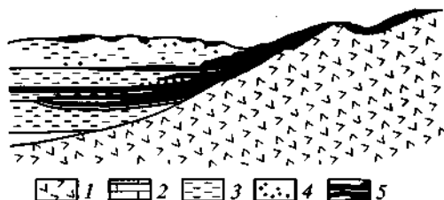
Рис. 6.20. Типы важнейших залежей бокситов Арканзаса и их геологическое положение (по М. Гордону, 1958):
