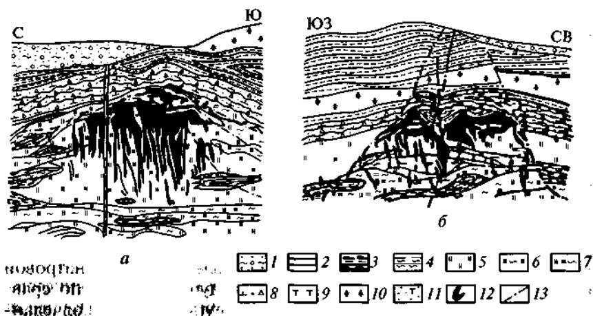
Рис. 6.30. Разрезы рудных залежей Риддер-Сокольского месторождения: а — Юго-Западная; б — Победа (по данным Лениногорского рудника); 1 — рыхлые отложения; 2 — алевропелиты; 3 — известковистые алевропелиты; 4 — серицитизированные алевропелиты; 5 — микрокварциты; 6 — серицит-хлорит-кварцевые породы; 7 — серицитизированные микрокварциты; 8 — агломератовые туфы смешанного состава; 9 — миндалекаменные плагиоклазовые порфиры; 10 — кварцевые альбит-порфиры; 11 — диабазы и диабазовые порфиры; 12 — полиметаллическая руда; 13 — разломы
