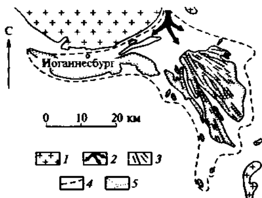
Рис. 6.60. Вееорообразный бассейн Витватерсранда (по Д. Преториусу):
