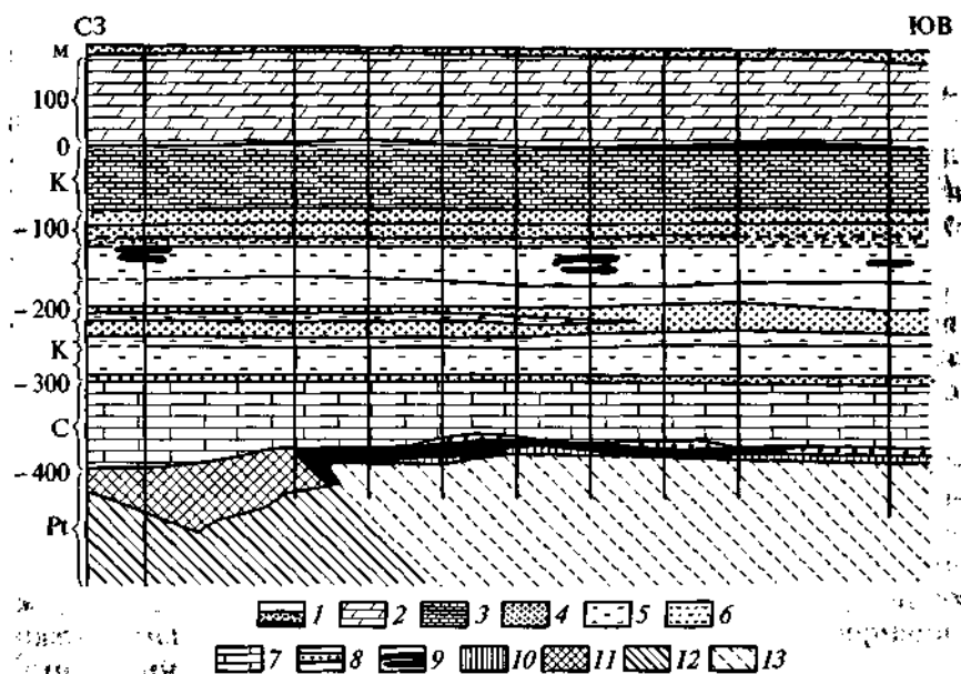
Рис. 6.19. Геологический разрез Висловского месторождения (по В. М. Григорьеву, 2005):
