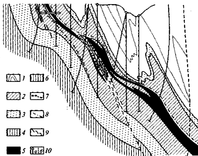
Рис. 1.15. Геологический разрез центральной части Филизчайского месторождения (по Н. Н. Шатагину и С. А. Сандомирскому):
