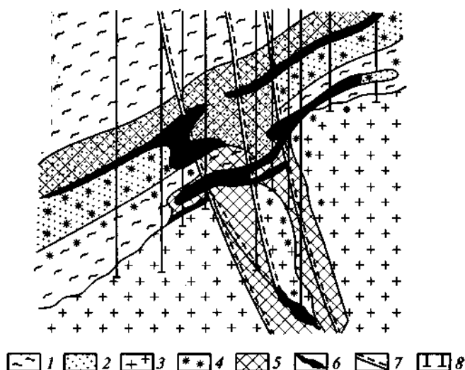
Рис. 2.5. Геологический разрез по приразломным «рудам восстановления» в отложениях альб-сеномана и гранитах фундамента (по М. Ф. Максимо-вой и Е. М. Шмариновичу, 1993):
