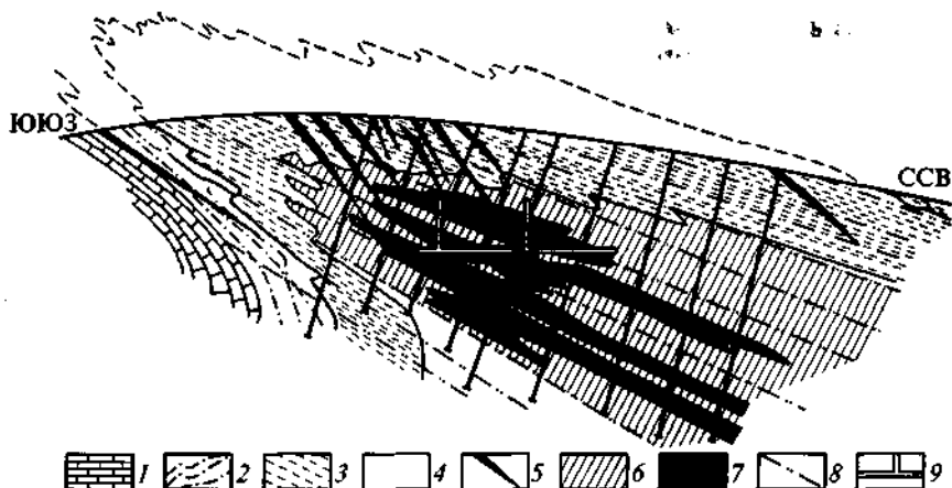
Рис. 6.63. Поперечный разрез зоны прожилково-вкрапленной золотосульфидной минерализации, сопровождающей золотоносными кварцевыми жилами месторождения Сухой Лог (по В. А. Буряку):
