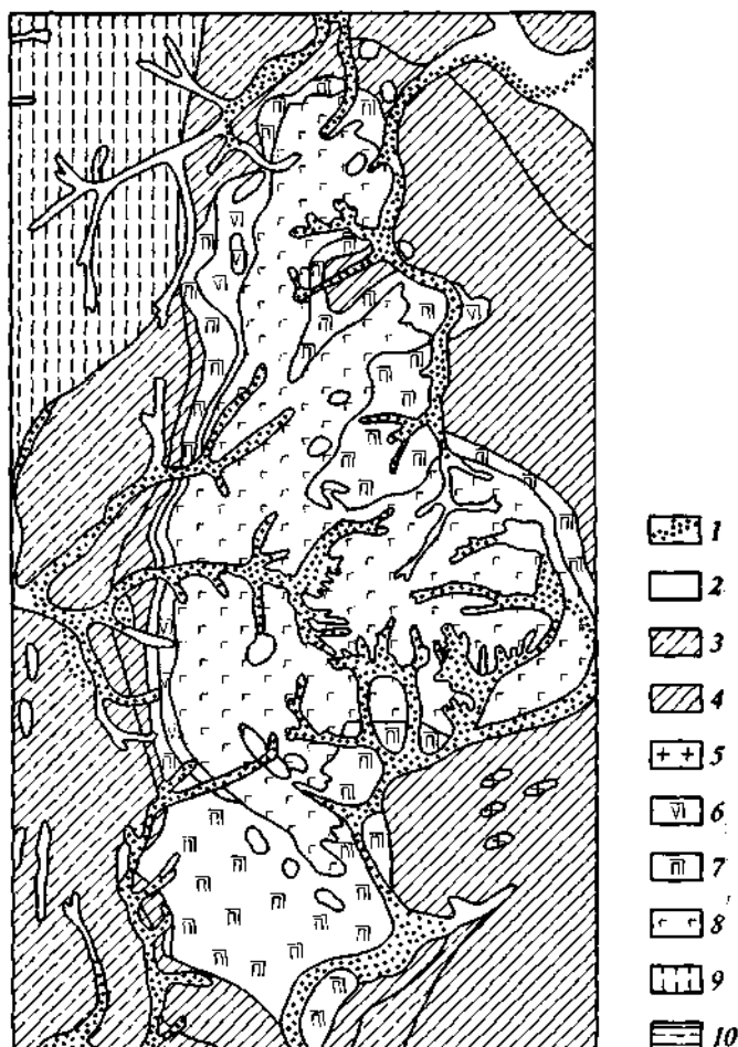
6.70. Схематическая геологическая карта Нижнетагильского платиноносного массива (по Н. И. Высоцкому):
