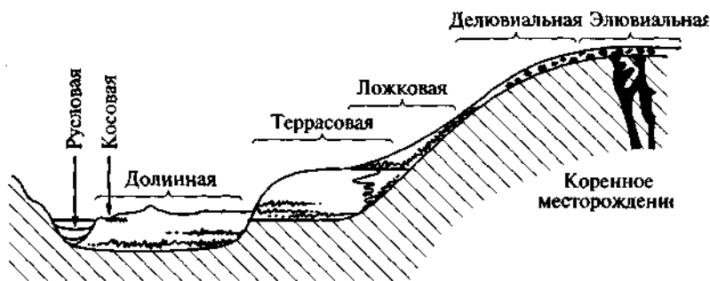
Рис. 2.3. Схема размещения россыпных месторождений различных видов в поперечном сечении речной долины (по В. И. Смирнову)
