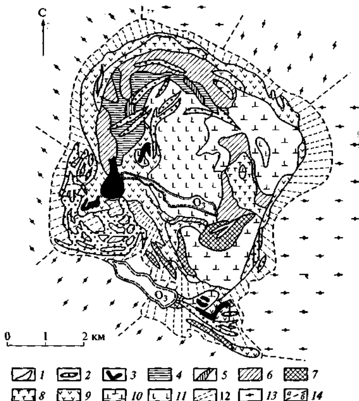
Рис. 1.8. Строение Ковдорского щелочного массива (по материалам В. И. Терновского (1977), Е. М. Эпштейна и Н. А. Данильченко (1988) с некоторыми дополнениями О. Б. Дудкина и Ю. М. Кирнарского (1994)):
