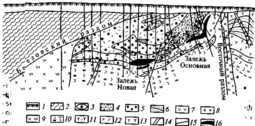
Рис. 6). Поперечный геологический разрез Орловского месторождения (по А. М. Гинатулину):
