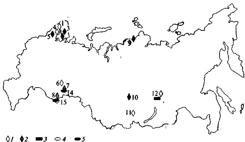
Рис. 7.7. Схема размещения мусковитонесущих районов России (по А. В. Ткачеву и др., 2002):
