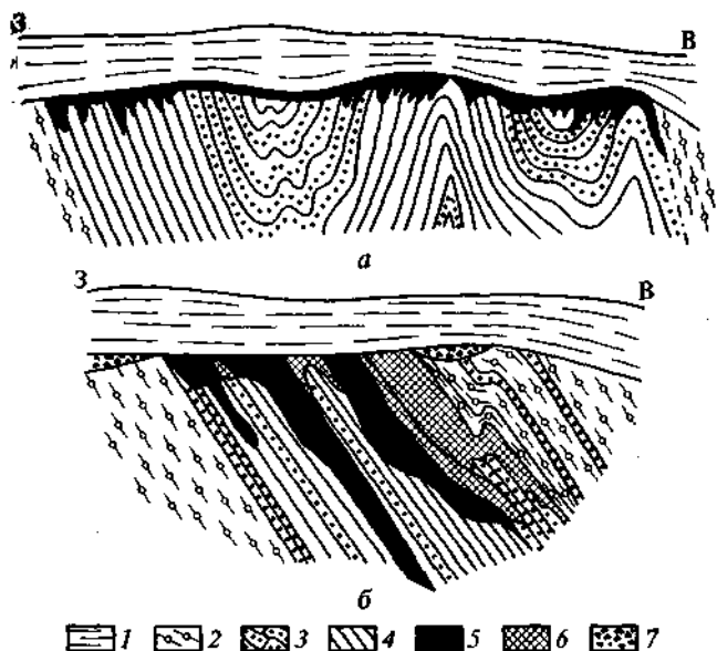
Рис. 6.4. Месторождения богатых руд в корах выветривания (Белгородский район КМА) (по В. И. Синякову, 1994):
