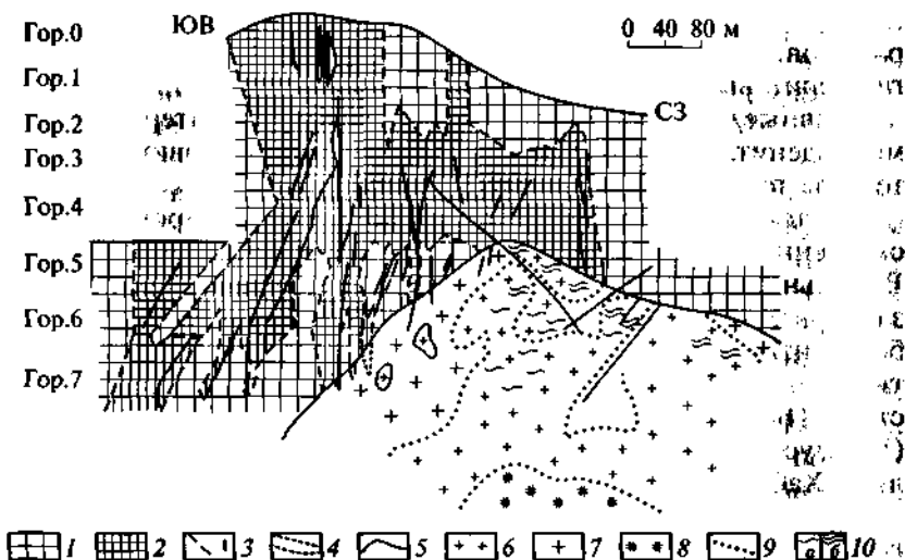
Рис. 6.38. Схематический геолого-петрографический разрез Иультинского месторождения (по Д. В. Дудкинскому и др., 1994):
