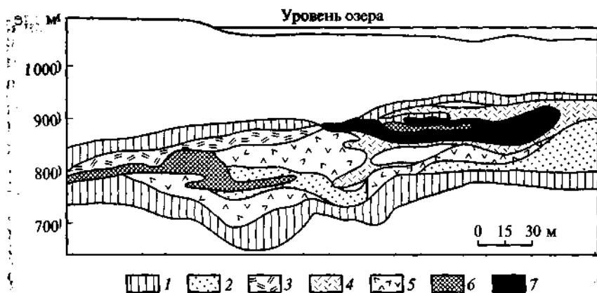
Рис. 6.44. Вертикальный разрез пегматитового тела Танко (месторождение Берник-Лейк, Канада) (по П. Черний и Р. Фергюсону):
