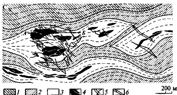
Рис. 3.2. Геолого-структурная схема Кировогорского месторождения (по П. М. Горяинову и Г. Ю. Иванюку, 2001):
