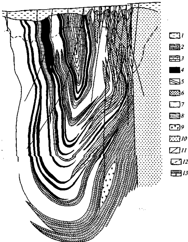
Рис. 6.32. Геологический разрез месторождения Ушкатын-Ш (по А. А. Рожнову, 1983)-'
