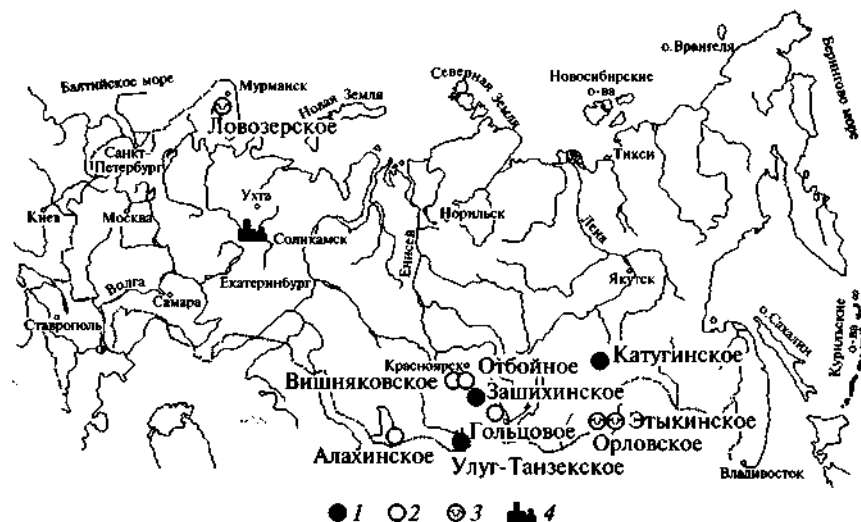
Рис. 6.51. Схема размещения основных месторождений тантала в России (по В. В. Рябцеву и др., 2006):
