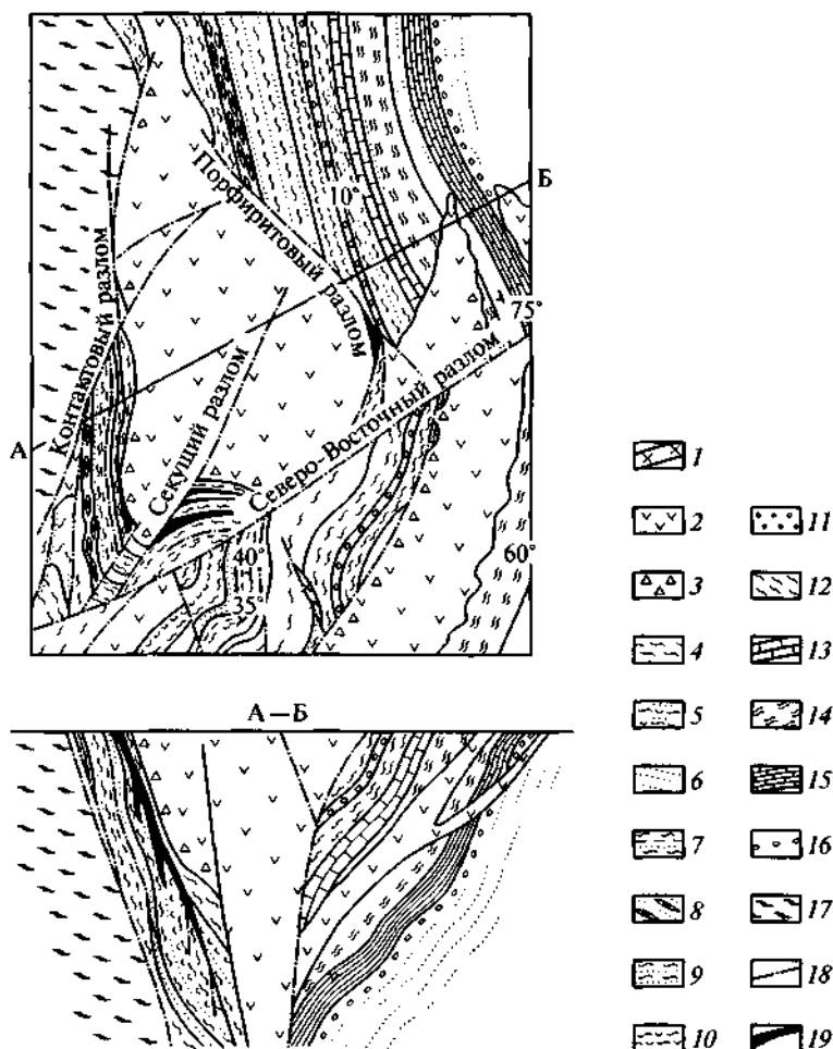
Рис. 6.74. Схема геологического строения молибден-уранового месторождения (по А. И. Зачернюку и др., 1970):
