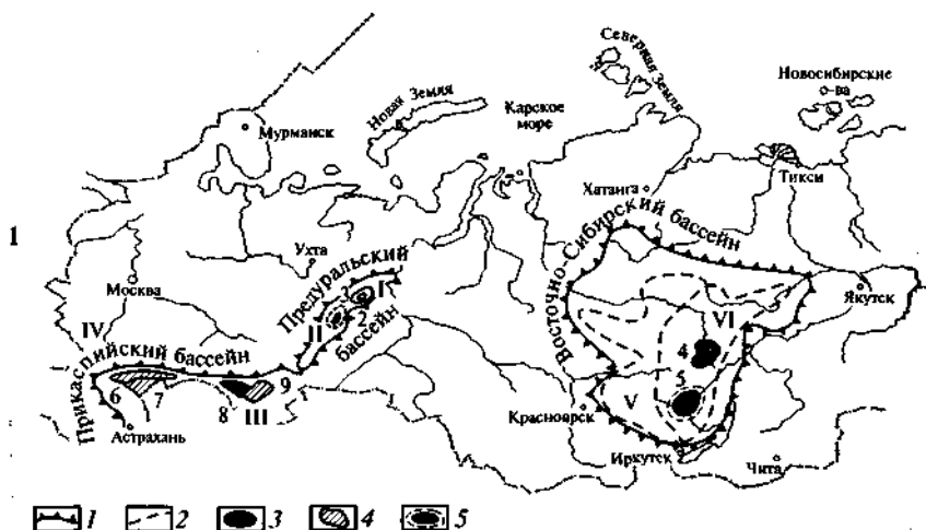
Рис. 7.4. Калиеносные бассейны России и их прогнозно-минерагенические подразделения (по Ю. В. Баталину и др., 1999):
