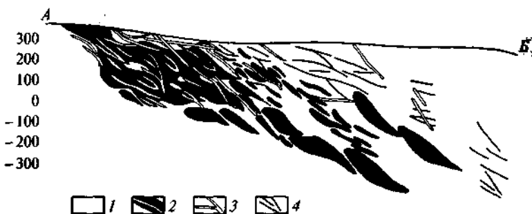
Рис. 3.3. Продольный разрез Кировогорского месторождения (по П. М. Горяинову и Г. Ю. Иванюку, 2001):
