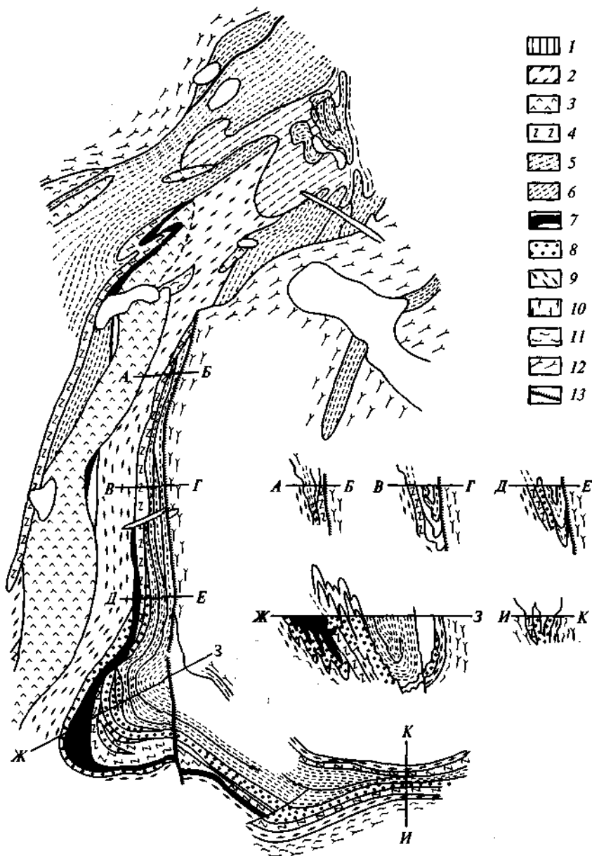
Рис. 3.1. Схема геологического строения Костомукшского месторождения:
