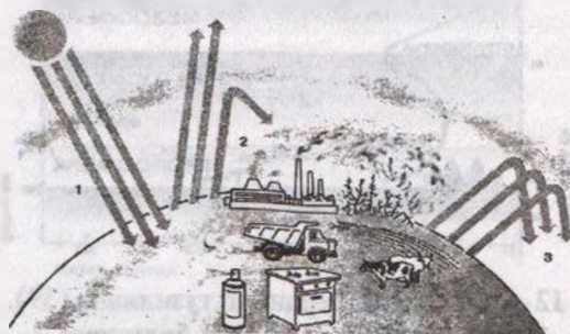
13- расм. «Иссиқхона эффекти»: 1-Ер юзасининг иссиши; 2-қайтарилган иссиқлик; 3-иссиқлик нурланишининг ушлаб қолиниши (18).
