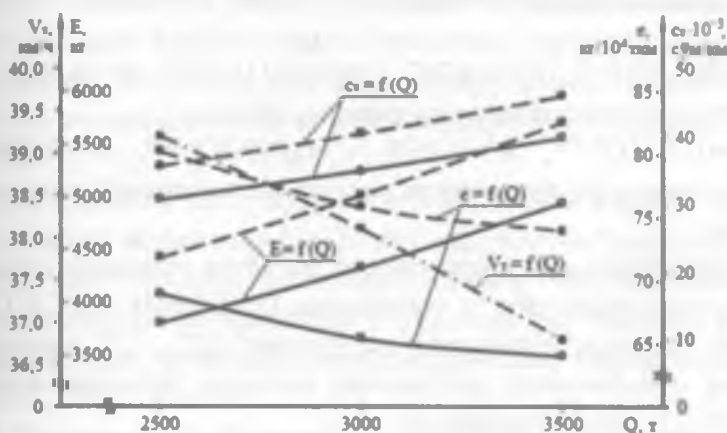
Рис.1. Динамика основных показателей использования тепловозной тяги на участке Ташгузар-Кумкурган.
