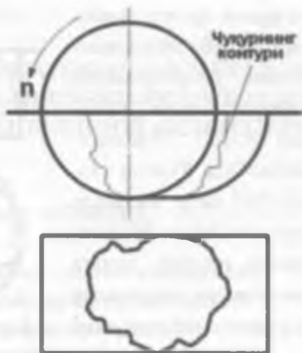
1- расм. Горизонтал фрезалашда ҳосил бўладиган чуқур профили
