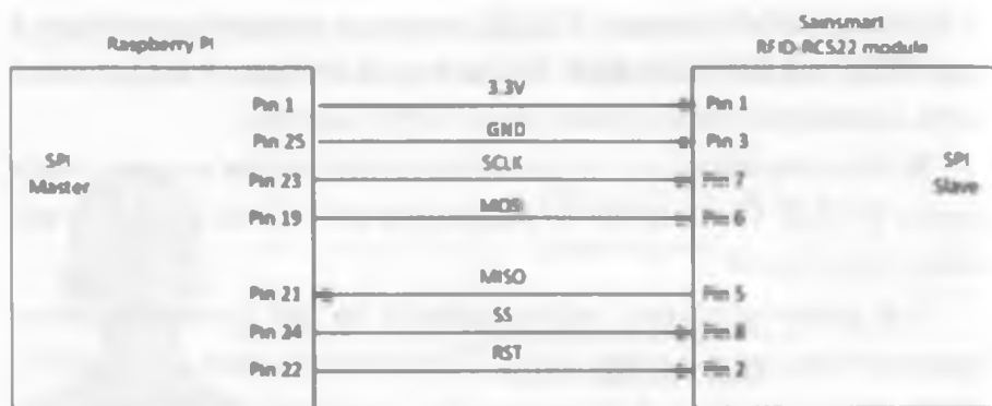
Рисунок 2. Схема подключения RC522 к Raspberry Pi.
