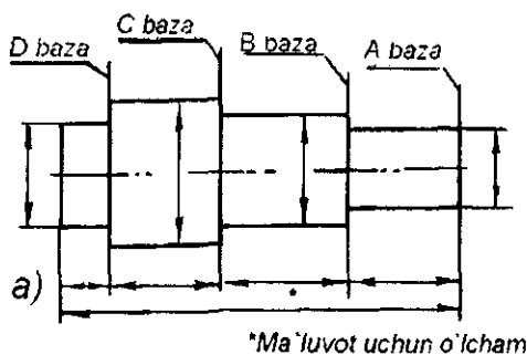
58-shakl. O'lcham qo'ish usullari: a) zanjirsimon; b) koordinatali; s) kombinatsiyalashgan (aralash)
