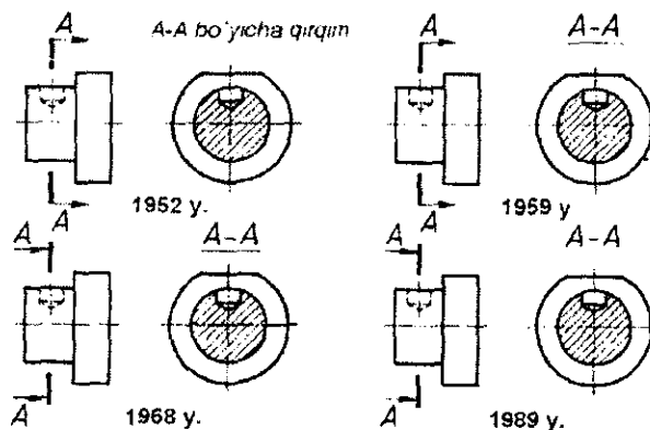
95-shakl. Qirqimlarni chizmani taxt qilishning eski va yangi qoidalari bo'yicha belgilanishi
