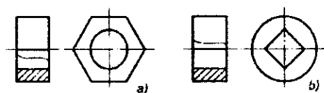
97-shakl. Detalning tashqi (a) va ichki (b) qirralari simmetriya o'qi bilan ustma-ust tushganda qirqimlardan o'rinli foydalanishga misol
