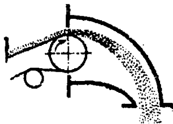
37-shakl. Kojux sirtini loyihalashda tashilayotgan material traktoriyasini hisobga olishga mosol
