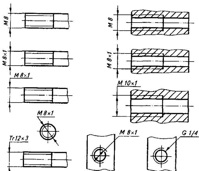
118-shakl. Chizmada rezbalarining tasvirlanishiga misollar
