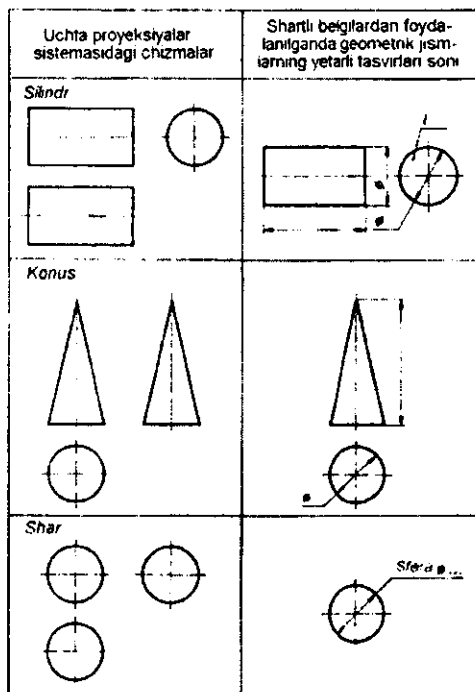
59-shakl. Geometrik jismlarga o'lcham qo'yilmaganda (a), hamda o'lcham, belgi va yozuvlardan foydalanilgandagi zarur va yetarli tasvirlar soni
