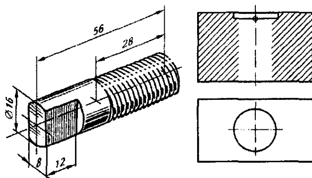
119-shakl. Rezbali birikmalarning tasvirlari
