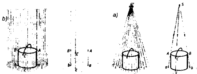
46-shakl. Proyeksiyalar hosil bo'lishini tushuntirishga misollar: a) markaziy proyeksiyalash; b) parallel proyeksiyalash
