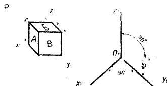
Qiyshiq burchakli gorizontal izometrik proyeksiya
