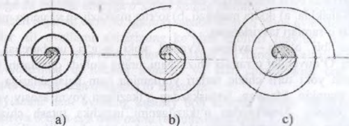
41-shakl. Lekalo yordamida bajarilgan ikki (a), to'rt (b) va uch (s) markazli o'ramlar.
