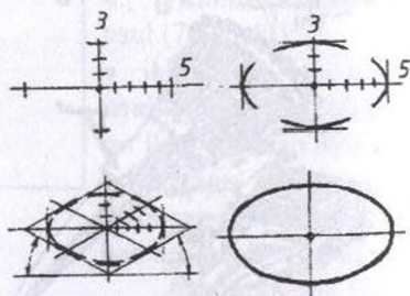
82-shakl. Aylanani izometriyada yasash bosqichlari
