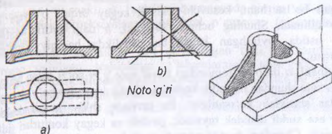
145-shakl. Yupqa qovurg'a bo'ylab qirqim yasash
