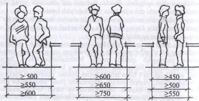
154-shakl. Sinfidagi asosiy o'tish joylarining o'lchamlari:
