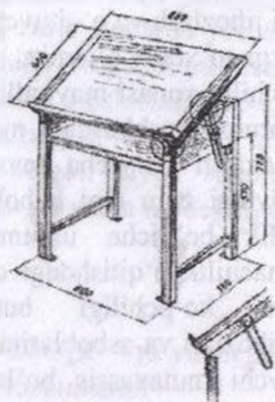
9-shakl. Soddalashtirilgan chizmachilik va rasm stoli
