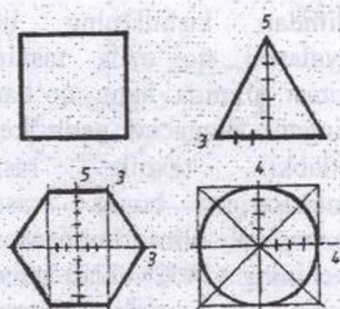
81-shakl. Yassi figuralar texnik rasmini bajarish usullari
