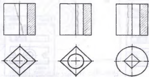
105-shakl. Ko'rishning bir qismi va qirqimning bir qismini birlashtirib tasvirlashning xususiy hollariga misollar
