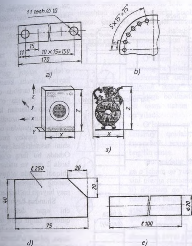
57-shakl. O'lchamlarning klassifikatsiyasiga misollar: bir tekis joylashgan elementlarning (a - chiziqli, b - burchakli), s - gabarit va d, e - detal uzunligi o'lchamlarini qo'yish
