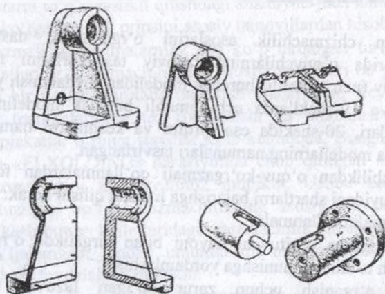
20-shakl. Qirgim va kesimlarni namoyish qilish uchun yig'ma modellar
