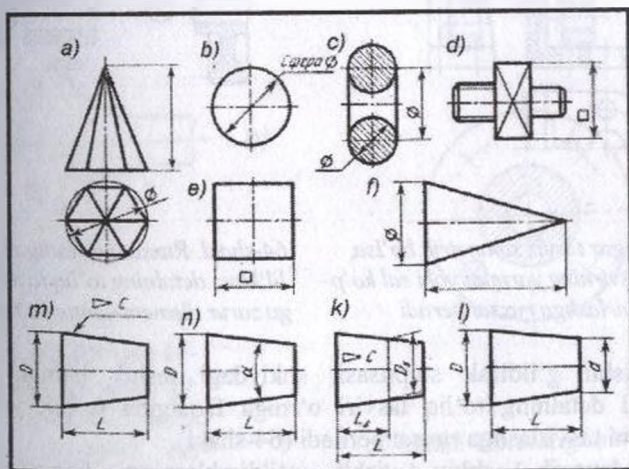
61-shakl. Chizmalardagi shartlilik va soddalashtirishlar
