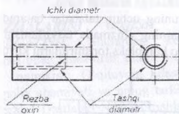
117-shakl. Ko'rinmas rezbaning tasvirlanishi
