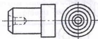
101-shakl. «Barmaq» detali chizmasi
