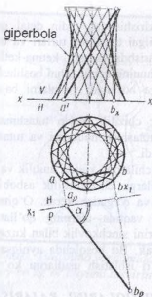
38-shakl. Giperboloid yasovchilari bo'yicha loyihalangan konstruktsiya tasviri
