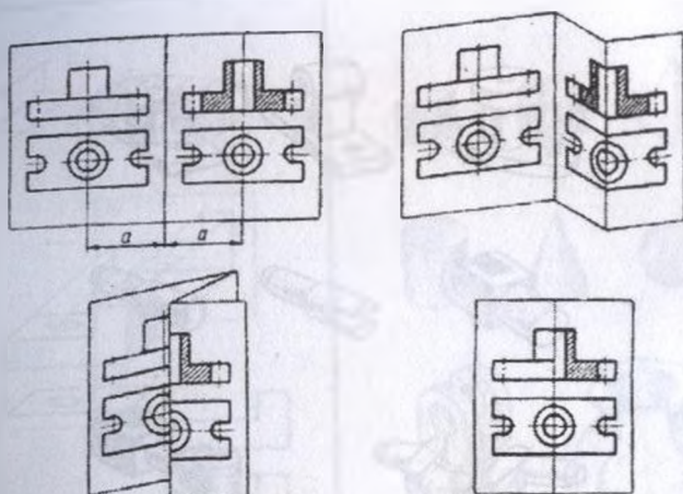
14-shakl. Qirqim hosil bo'lishini namoyish qilish uchun dinamik plakat
