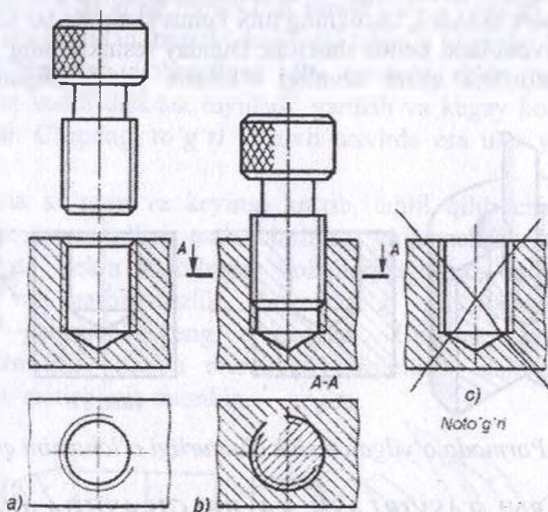
149-shakl. Rezba yordamida biriktirish va chizmada rezbaning noto'g'ri tasvirlanishi: a) birikadigan detallar; b) birikma tasviri; c) rezbali teshikni shtrixlashdagi tipik xato
