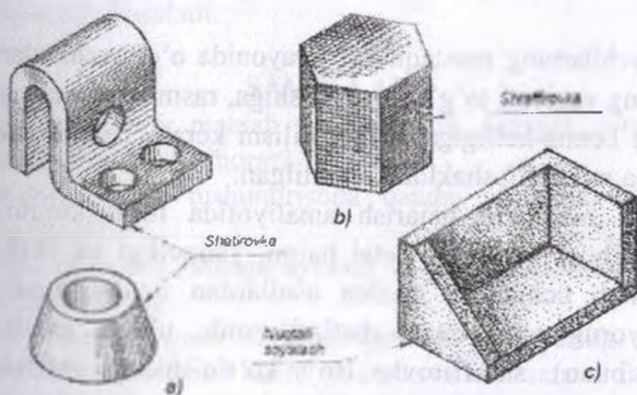
86-shakl. Texnik rasmda hajmni ko'rsatish: a) shatirovka, b) shraffirovka, s) nuqtali soyalash usullariga misollar
