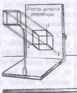
69-shakl. Frontal dimetrik proektsiya hosil bo'lishini namoyish qilish uchun model
