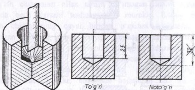
148-shakl. Parmada o'yilgan teshik chuqurligi o'lchamini qo'yish
