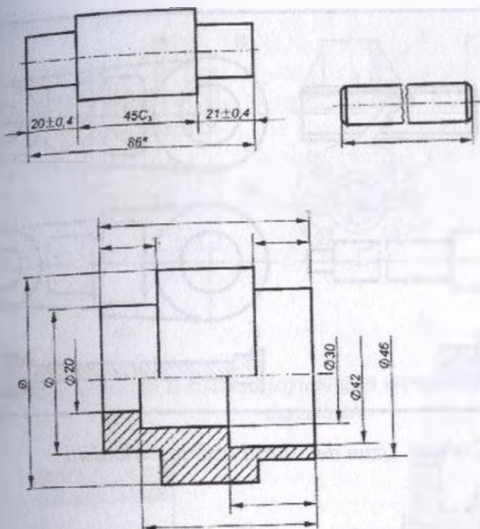
60-shakl. O'lcham qo'yish variantlariga misollar
