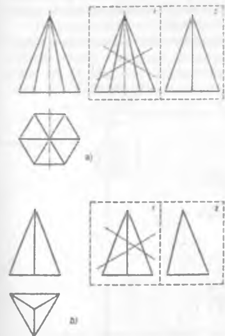
141-shakl. Ko'pyoqliklarning uchinchi proeksiyalarini qurishda o'quvchilarning tipaviy xatolari
