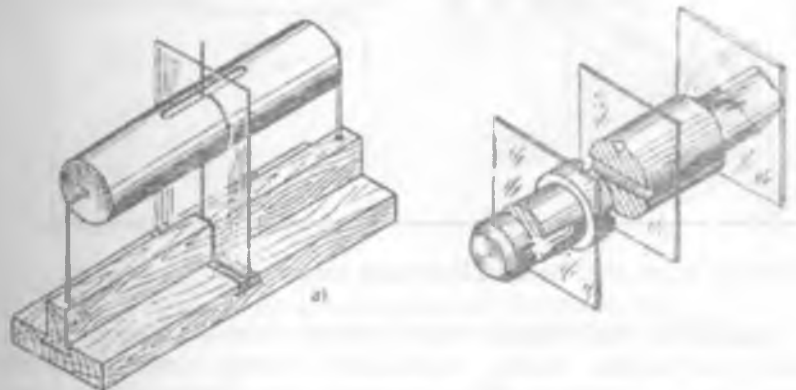
89-shakl. Pog'onali valikning kesma modeli
