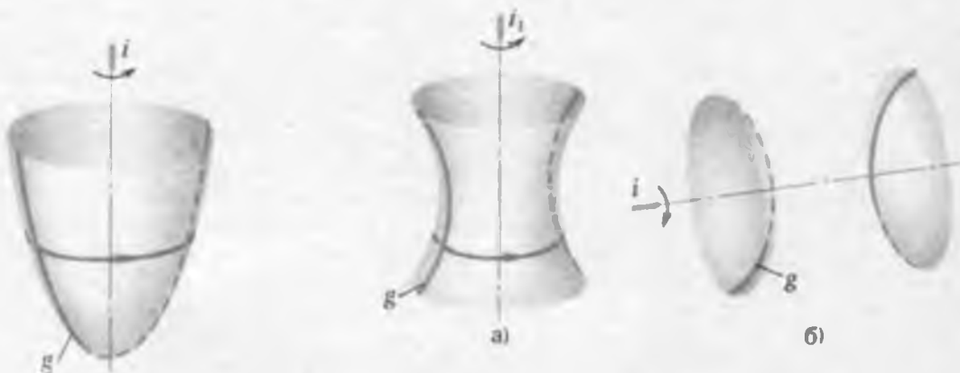
Рис. 161 Гиперболоид вращения: а — однополостный, б — двухполостный
