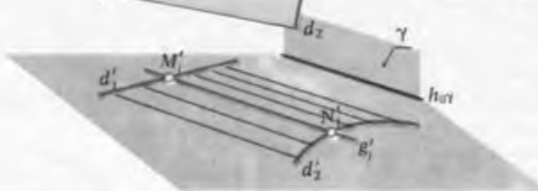
Рис. 141 Поверхность прямого конуса
