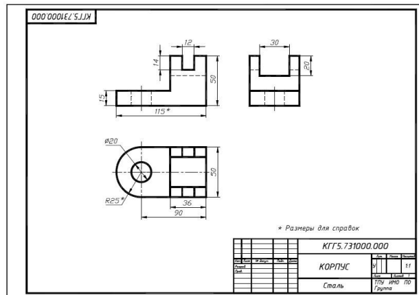
Чертеж детали
