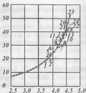
2.5-rasm. Betondan o'tayotgan ultratovush to'lqinlari tezligi bilan uning siqilishdagi mustahkamligi orasidagi bog'lanish grafiqi.
