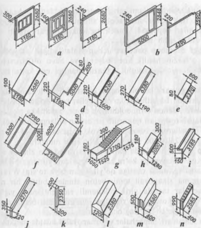
7.7-rasm. Turar joy binolarida ishlatiladigan yig'ma temir-beton buyumlari.
