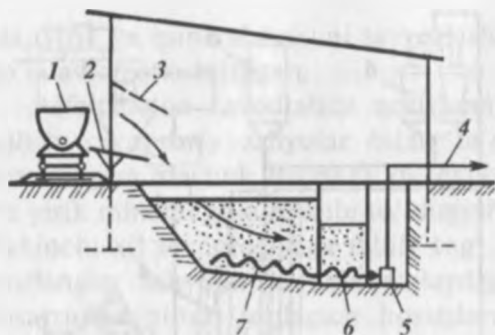
9.8-rasm. Bitum hovuz:
