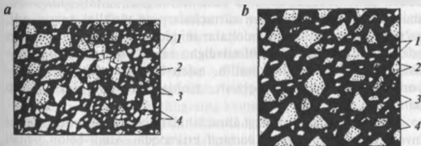
9.1-rasm. Asfalt-betonning tuzilishi:
