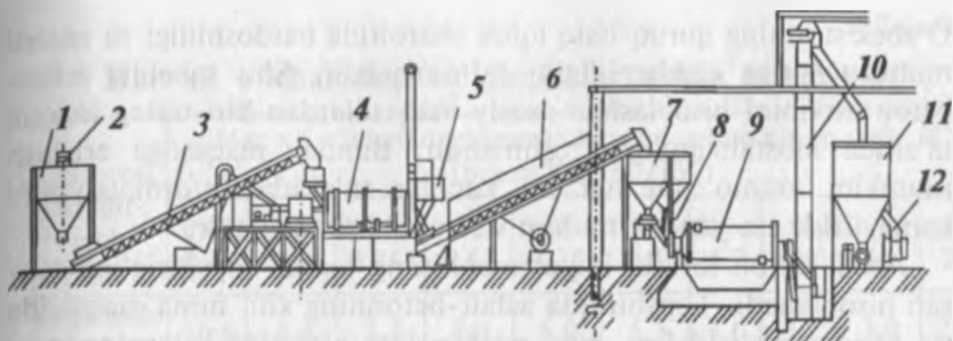
9.9-rasm. Faollashtirilgan mineral kukunini ishlab chiqarishning texnologik sxemasi.
