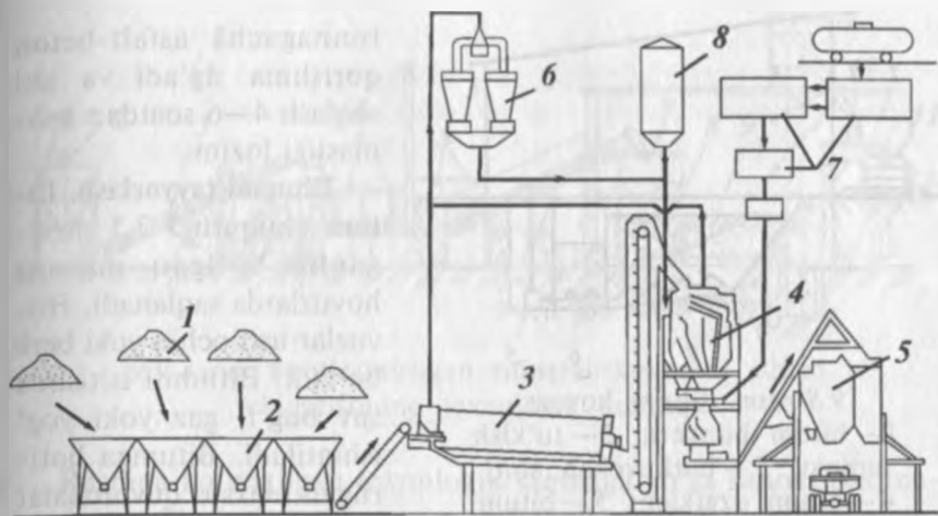
9.7-rasm. Issiq va iliq asfalt-beton qorishmasini tayyorlash sxemasi:
