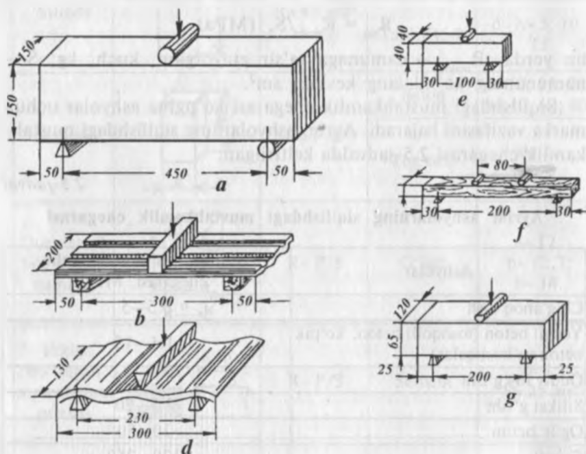
2.3-rasm. Ashyolarni egilishga sinash sxemasi va ishlatiladigan namunalar: a — beton prizma; b — cherepitsa; d — to'lqinsimon asbosement taxtacha; e — sementli plastik qorishma; f — yog'och; g — g'isht.
