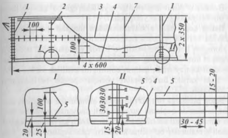
5.12-rasm. Beton qoplama ko'rinishi:
