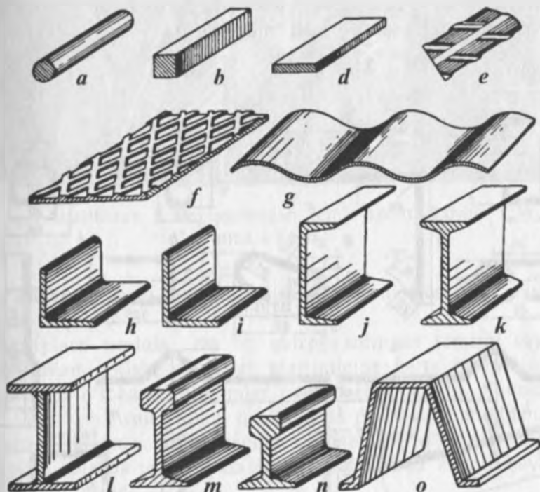
6.2-rasm. Po'lat navlari. a — dumaloq; b — kvadrat; d — tasmasimon; e — takroriy uzun; f — taram-taram; g — to'lqinli; j — teng burchakli; h — teng bo'lmagan burchakli; i — shveller; j — qo'shtavr; k — payvandlangan qo'shtavr; n — temiryo'l izi (relsi); m — devorbop shpunt.
