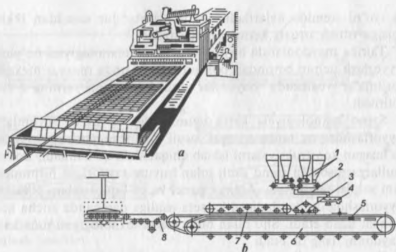
7.5-rasm. Temir-beton buyumlar tayyorlaydigan tebratma-prokat stani:
