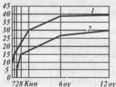
5.1-rasm. Qumdagi organik aralashmalarning beton mustahkamligiga ta'siri: 1 — toza qum, 2 — tarkibida organik aralashma bo'lgan qum.
