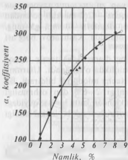
2.9-rasm. Elektron usul bilan qumning namligini aniqlash.
