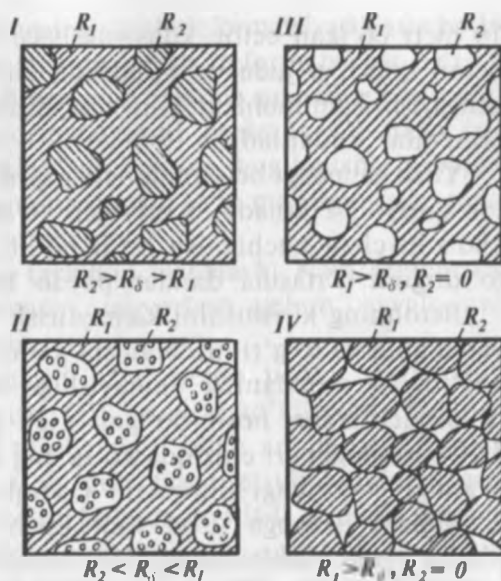
5.9-rasm. Beton strukturasi turlari: I — zich, II — zich yengil to'ldirgich blok, III — serg'ovak, IV — yirik g'ovakli, R_b — betonning o'rtacha mustahkamligi, R_1 va R_2 — beton tarkibidagi ashyolarning mustahkamligi.
