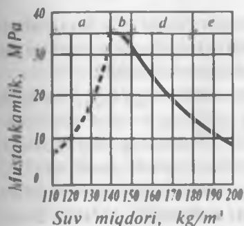
5.5-rasm. Betonning siqilishdagi mustahkamligining suv miqdoriga bog'liqligi:
