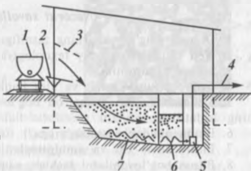
8.9-rasm. Bitum saqlagichning shakliy tasviri:
