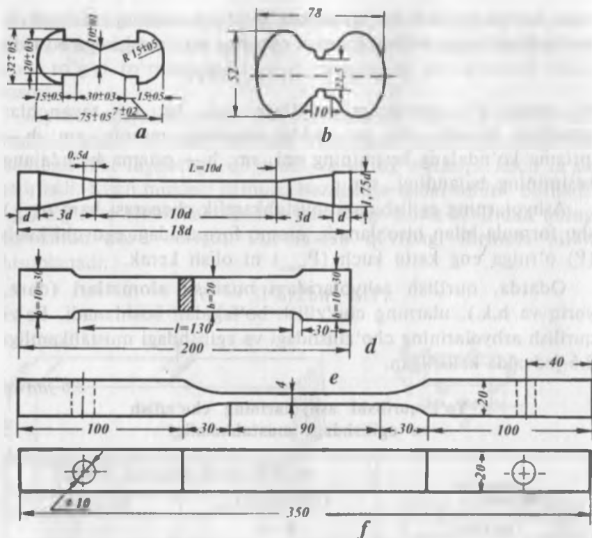
2.4-rasm. Cho'zilishga sinaluvchi namunalar:
