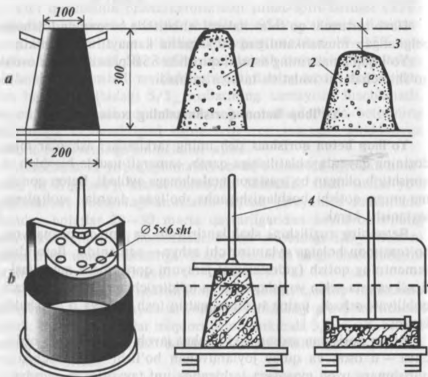
5.4-rasm. Beton qorishmasining qulay joylanuvchanligi (a) va yoyiluvchanligi (b)ni aniqlash. 1 — o'ta quyuq qorishma; 2 — plastik qorishma; 3 — konusning cho'kishi; 4 — yoyiluvchanlikka sinash.
