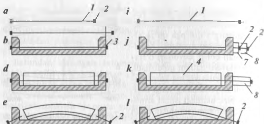
7.4-rasm. Armaturani oldindan taranglash usullari:
