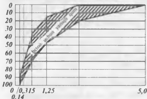
5.2-rasm. Qumning mayda-yirikligini ifodalovchi grafik.
