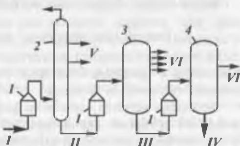
8.2-rasm. Quyuq qoldiq bitum olishning texnologik sxemasi:
