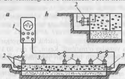
2.6-rasm. Yo'l qurilishidagi beton konstruksiyani ultratovush to'lqinlari bilan sinash sxemasi:
