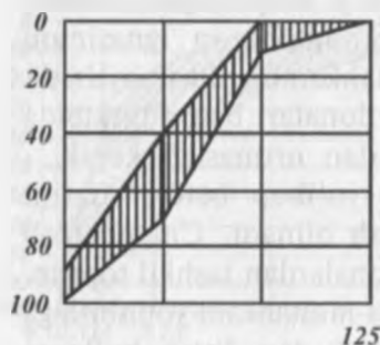
5.3.-rasm. Shag'alning mayda-yirikligini ifodalovchi grafik.
