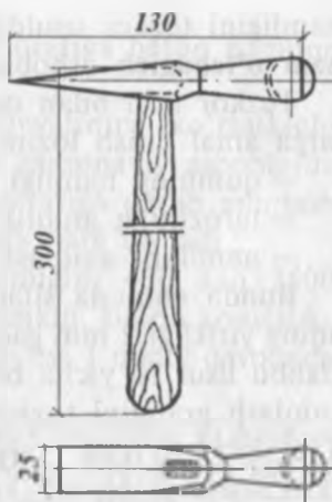
2.7-rasm. Fizdelning zoldirli bolg'asi.
