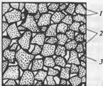
9.2-rasm. Zichlangan qora chaqiq toshli qorishmaning tuzilishi:
