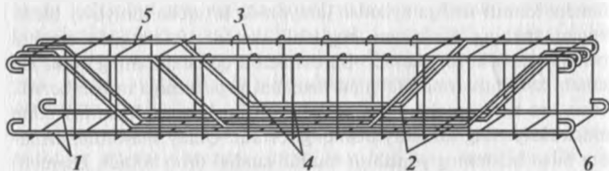
7.2-rasm. Temir-beton to'sinbop armatura karkas:
