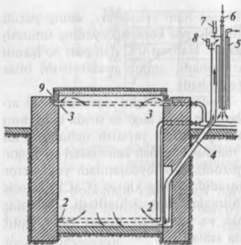
5.8-rasm. Beton konstruksiyalarni bug'lab qotiruvchi avtomatik kamera sxemasi:
