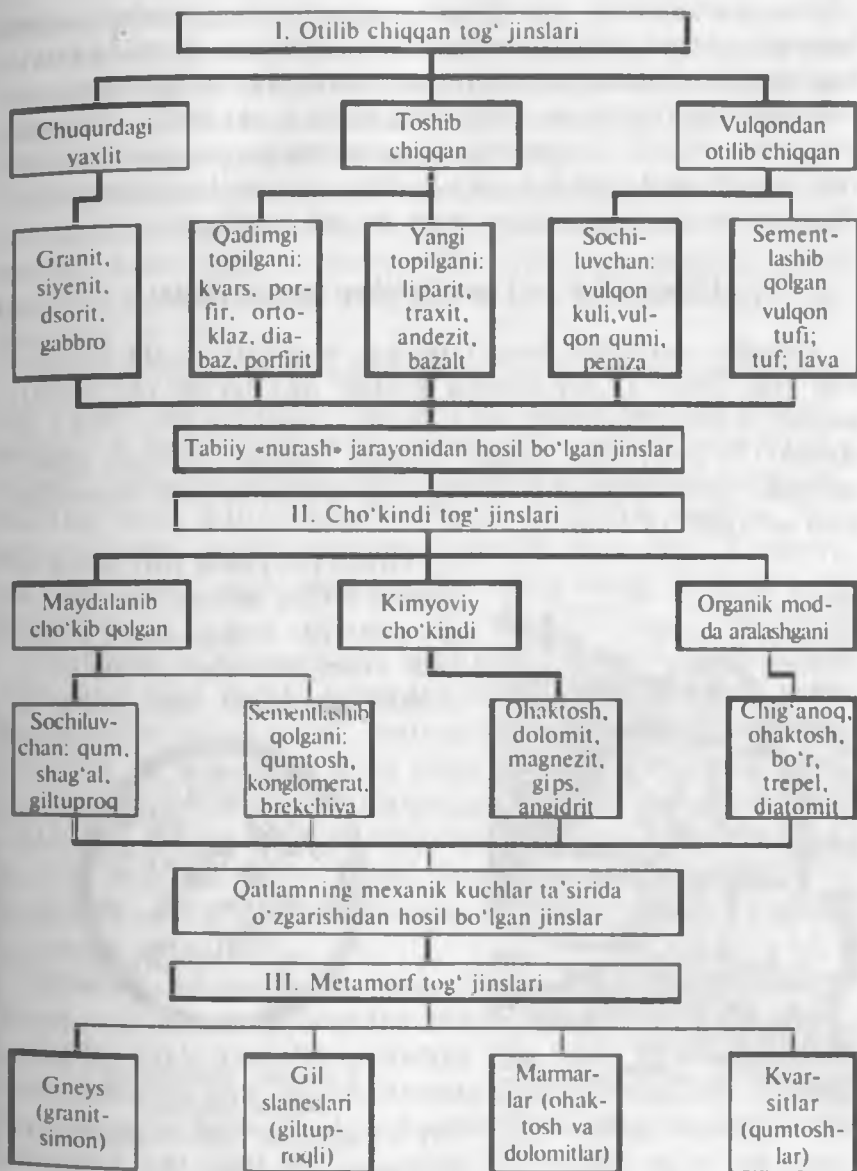
3.1-rasm. Tog' jinslarining xillari.
