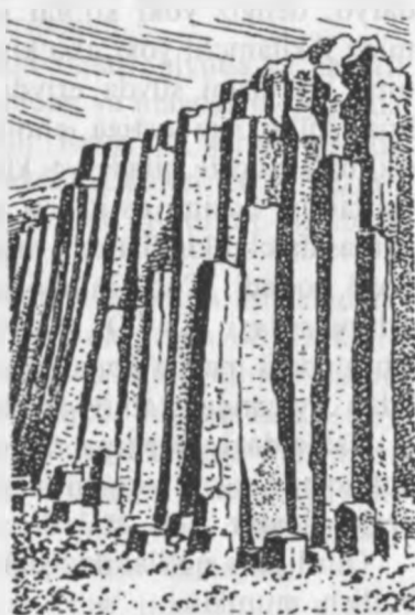
3.5-rasm. Ustun singari joylashgan tog' jinslari (bazaltlar).
