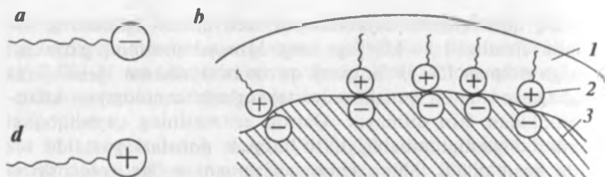
9.6-rasm. SFM qo'shilgan bitumning to'ldirgich dona sirtiga yopishish sxemasi:
