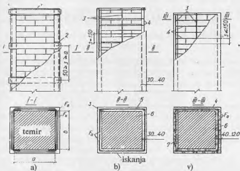
114-rasm. G'ishtli devor konstruksiyalarini kuchaytirish usullari.
