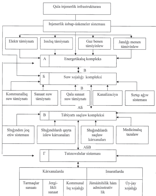
7-súwret. Injenerlik infrastrukturalardıń óz-ara baylanısı sızılması.
