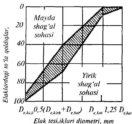
6.2-rasm. Shag'al donador tarkibi grafiği.
