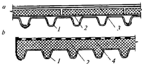
14.3-rasm. Sanoat buyumlari tom qoplamalari konstruksiyalari:
