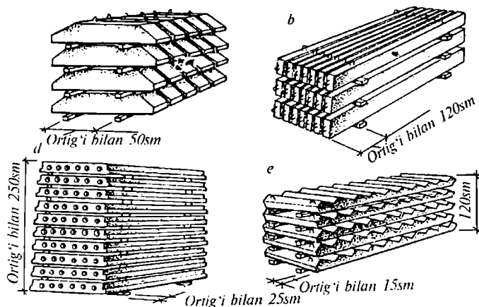
7.8-rasm. Yig'ma temirbeton konstruksiyalarni omborlarga joylashtirish:
