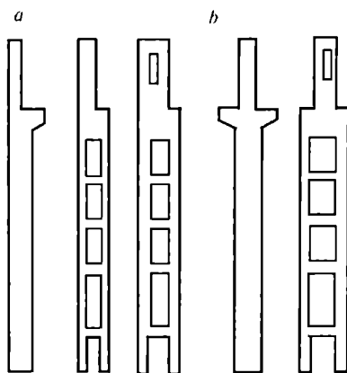
7.3- rasm. Bir va ikki tarmoqli temirbeton ustunlar:
