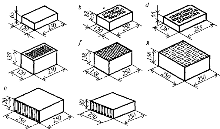
3.3-rasm. Keramik g'isht turlari:
