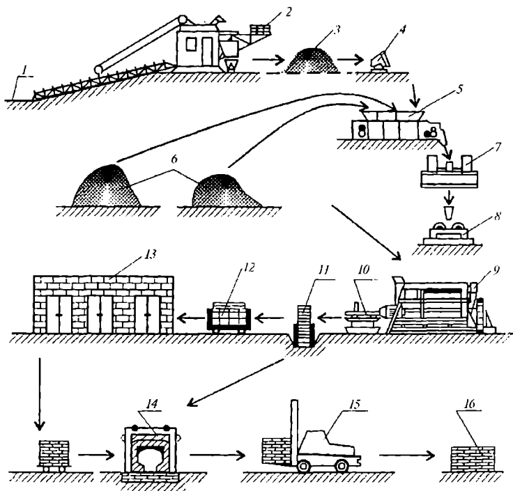
3.1-rasm. Keramik g'isht ishlab chiqarish texnologik sxemasi:
