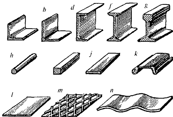
15.4-rasm. Prokatka qilingan po'latlar sortamenti:
