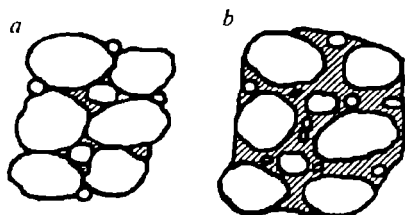
6.5-rasm. Beton qorishmasi strukturasi:
