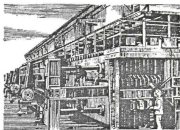
7.7-rasm. Kasseta ustanovkasi.
