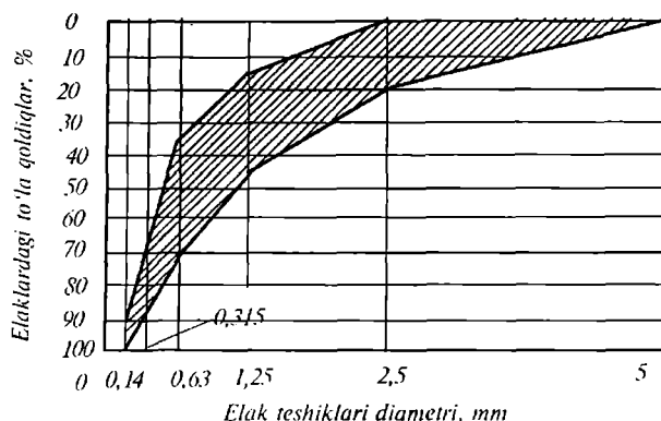
6.1-rasm. Qum donador tarkibining grafigi.
