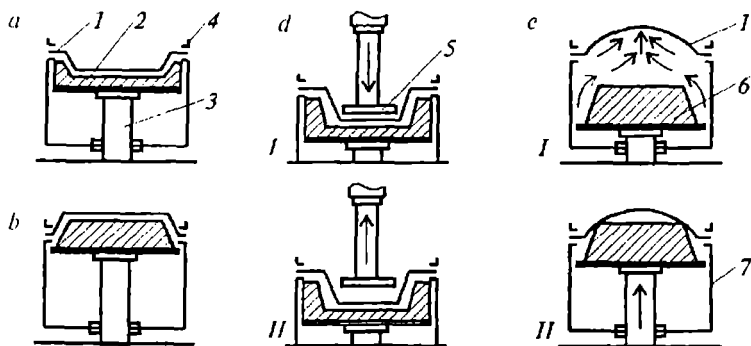
11.6-rasm. Vakuum-qoliplash sxemasi:
