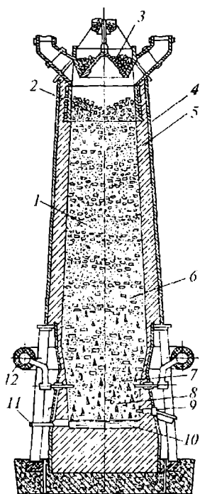
15.1-rasm. Domna pechining sxemasi:
