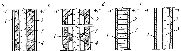
14.2-rasm. Uch qatlamli tashqi devor panellari turlari:
