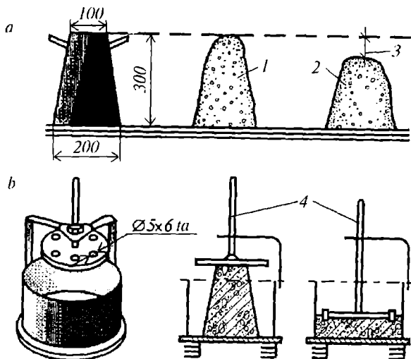
6.3-rasm. Beton qorishmasining qulay joylanuvchanligini aniqlash:
