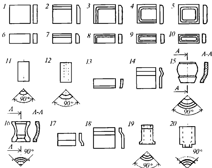
3.4-rasm. Ichki devorlarga qo'llaniladigan plitkalar:
