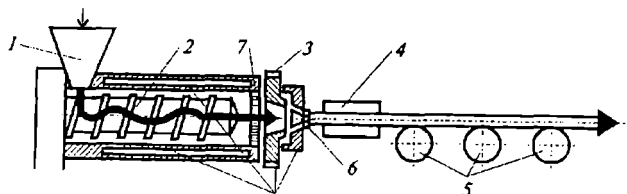
11.3-rasm. Ekstruziya mashinaning ishlash sxemasi:
