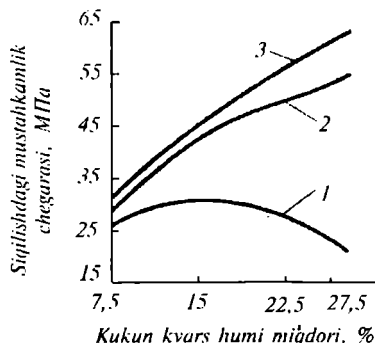
9.3- rasm. Kvarts qumi kukuniligi va miqdorining silikat beton mustahkamligiga ta'siri: 1 - kvarts qumining kukuniligi 1500 sm 2 /g; 2 - 2500 sm 2 /g; 3 - 4500 sm 2 /g.
