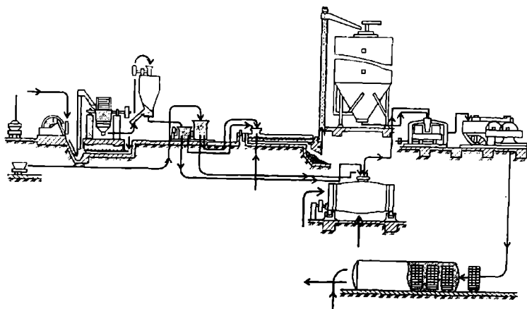
9.2-rasm. Silikat g'isht ishlab chiqarish texnologik sxemasi.
