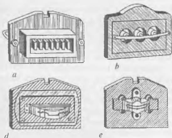
6-rasm. Tasmali zichlagichga o'rnatiladigan mundshtuk:
