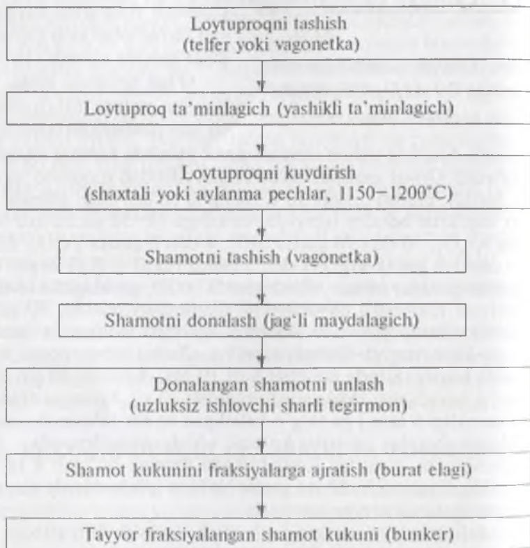
Shamotning fraksiyalangan kukunini tayyorlash chizmasi
