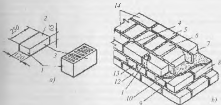
9-rasm. Teriladigan devor konstruksiyasi elementlari:
