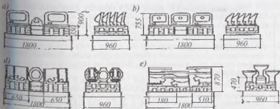
15-rasm. Sanitar-qurilish buyumlarining ratsional o'tkazilish variantlari: a, b – yuvinish stollar; d, e – unitazlar.
