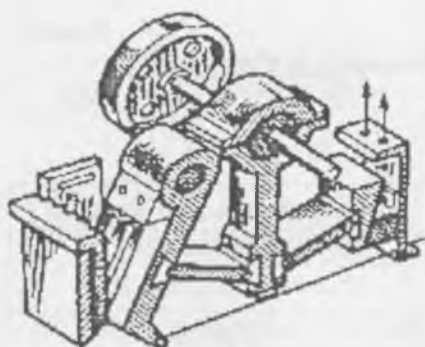
12-rasm. Oddiy tebranma jag'li maydalagich.
