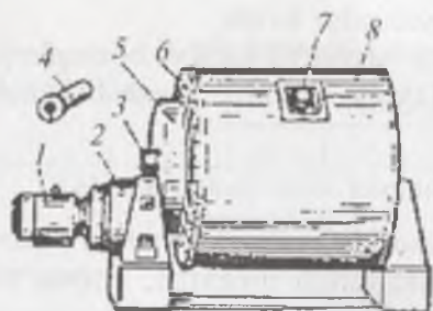
10-rasm. Uzlukli tarzda ishlovchi zoldirli tegirmon.
