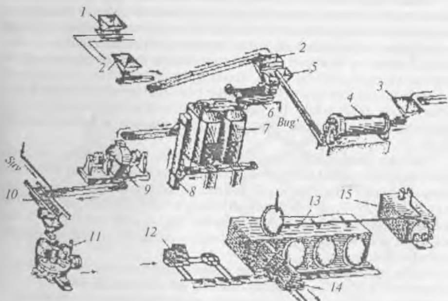
8-rasm. Silikat g'isht quyish texnologik sxemasi:
