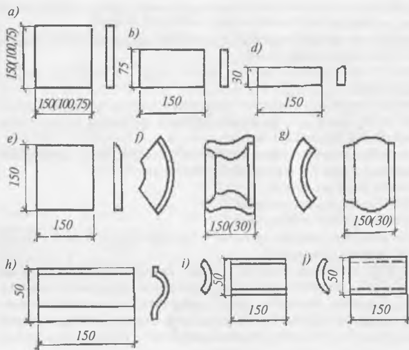
2-rasm. Devorlarni qoplash uchun plitkalar (taxtachalar):
