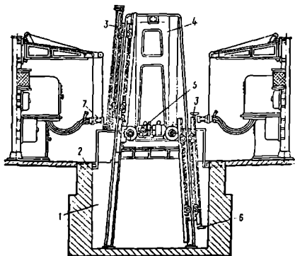
2.35-rasm. Fazoviy karkaslarni payvandlash moslamasi:
