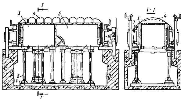
1.61-rasm. "Qalpoq" turidagi hajmiy-qoliplash moslamasi:
