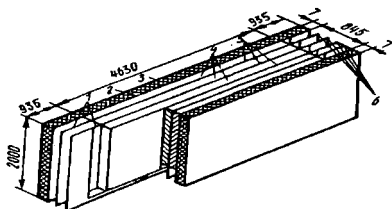
1.10-rasm. Temir-beton panellari elektroqizdirish uchun jihozlangan kassetada 5 ta panelning joylanish chizmasi:
