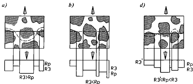
2.1-rasm. Betonning buzilish xarakteri.
