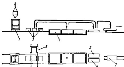
1.39-rasm. Agregat ishlab chiqarishni tashkil qilish chizmasi:
