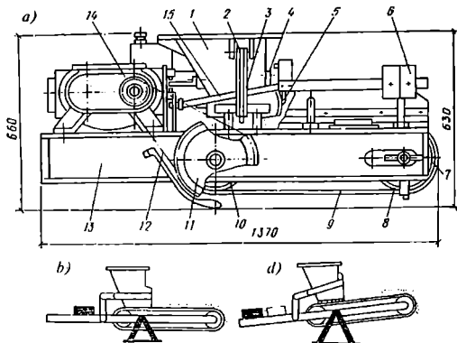
1.25-rasm. SB-26A rusumli to'ldiruvchilarni miqdorlash:
