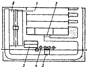
1.38-rasm. Yiliga 11 ming kub metr hajmda temir-beton quvurlarni ishlab chiqaradigan zavodning bosh loyihasi: 1 – ishlab chiqarish korpusi; 2 – beton qoruvchi sex; 3 – qabul qilish qurilmasi; 4 – sement omborxonasi; 5 – to'ldiruvchilar omborxonasi; 6 – tayyor mahsulot omborxonasi.
