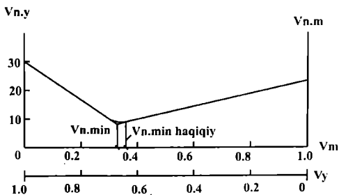
1.1-rasm. Qorishma g'ovakliligi hajnining (massa bo'yicha % da) mayda va yirik to'ldiruvchi miqdoriga bog'liqligi.
