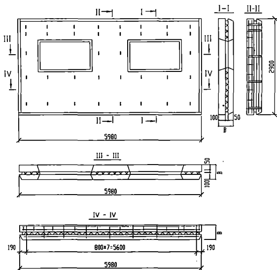
2.40-rasm. Qishloq xo'jaligi binolari uchun mo'ljallangan uch qatlamli panel.
