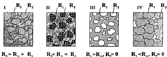
1.11-rasm. Betonning asosiy makrostrukturaviy turlari.
