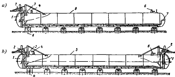
2.23-rasm. Avtoklavlar:
