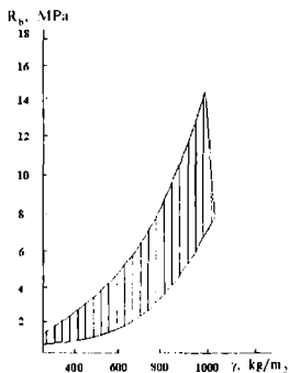
2.24-rasmi. Katakehali beton mustahkamligi R_b uning zichligiga bog'liqligi.
