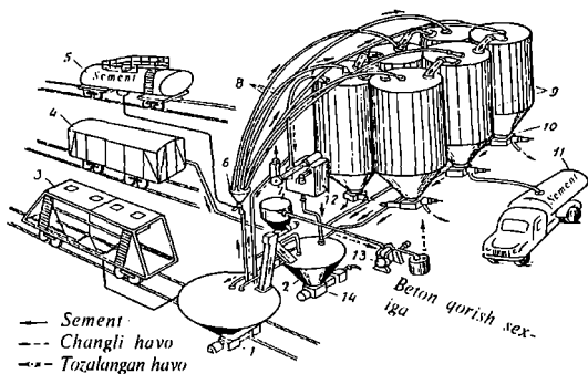
1.17-rasm. Temir yo'li yonida qurilgan sement omborining texnologik chizmasi: 1 – pnevmatik ko'targich, 2 – bunker; 3 – sement tashuvchi vagon; 4 – yopiq vagon; 5 – vagon-sisterna; 6 – sement uzatkichlarni biridan boshqasiga ulovchi moslama; 7 – pnevmatik to'kuvchi; 8 – sement uzatkichlar; 9 – siloslar; 10 – tag qismidan sement uzatadigan pnevmatik to'kuvchi; 11 – avtosement tashuvchi; 12 – rukavali filtri; 13 – vakuum moslamasi; 14 – pnevmatik vintsimon nasos.
