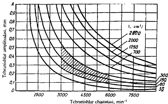
1.49-rasm. Vibratsiyaning intensivlik chizmasi.
