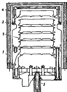
2.18-rasm. Uzlüksiz ishlaydigan vertikal kamera: 1 – kamera to'sig'i; 2 – pod-donga qo'yilgan buyum; 3 – bug' yetkazib beruvchi perfoquvur; 4 – yetkazib beruvchi aravacha; 5 – ko'targich stol.
