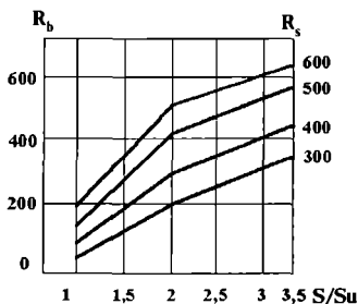
1.13-rasm. Talab etiladigan beton R_b mustahkamligi va qo'llanilayotgan R_s sement markasiga bog'liq holda Su/S nisbatini tayinlash grafigi.
