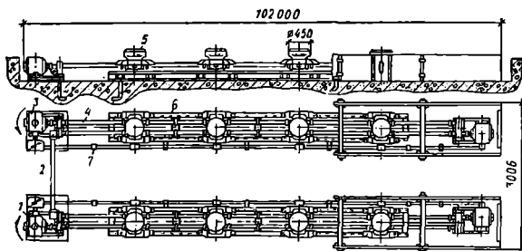
1.57-rasm. SMJ-200B rusumli vibromaydoncha chizmasi:
