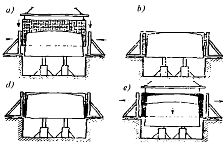
1.13-rasm. TAG-1 qurilmasi hajmli blokining
