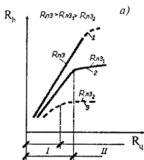
2.20-rasm. Keramzitli shag'al va qorishma mustahkamligining keramzitbeton mustahkamligiga ta'siri.
