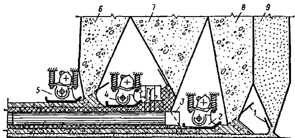
1.66-rasm. Betonlovchi kombayn ishchi organlarining joylashish chizmasi:
