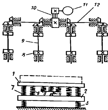
1.55-rasm. Zarbali (kulachokli) maydoncha chizmasi:
