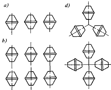
1.14-rasm. Beton qorish mashinalarini joylashtirish chizmalari:
