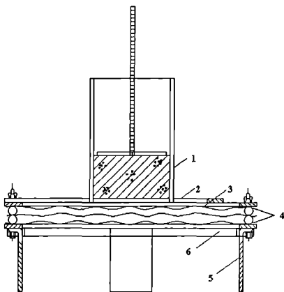
2.29-rasm. Armoementning qoliplanuvchanligini aniqlash uchun mo'ljallangan moslama.
