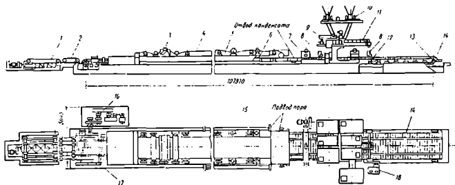
2.8-rasm. Vibroprokat stanida mahsulot tayyorlash chizmasi:
