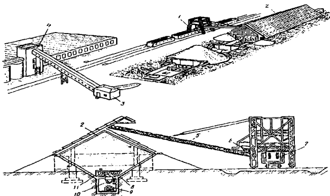
1.19-rasm. To'ldiruvchining shtabel-yarim bunkerli yopiq omborxonasi:
