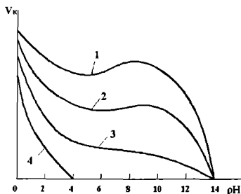
2.17-rasm. Po'lat zanglashi o'z tezligining tarkibda kislorod bo'lgan pH qorishmasiga bog'liqligi. 1 – yuqori; 2 – o'rtacha; 3 – past; 4 – kislorod ishtirok etmaganda.
