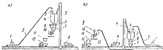
1.13-rasm. Beton qoruvchi moslamalarni vertikal o'rnatish chizmasi:
