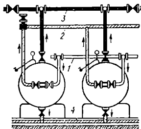
2.25-rasm. Avtoklavdagi bug' o'tkazgichlar chizmasi:
