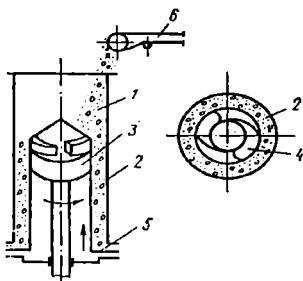
1.70-rasm. Trubaga radial presslab shakl berish uskunası:
