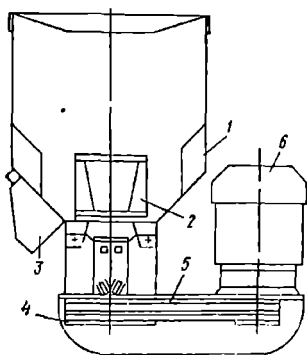
1.30-rasm. Girdobii (turbulentli) qoruvchining chizmasi:
