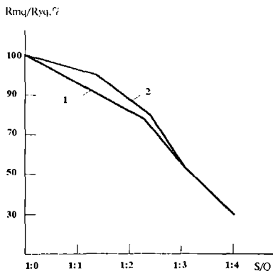
2.26-rasm. Mayda qumning qumli beton mustahkamligiga ta'siri.
