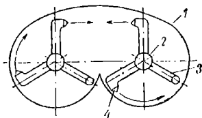
1.31-rasm. Oqimli beton qoruvchining uzluksiz harakatli chizmasi:
