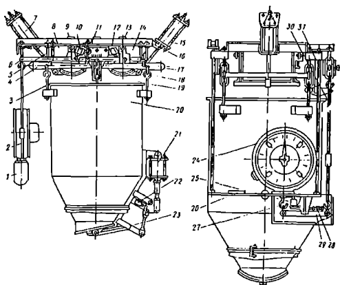
1.21-rasm. AVDI – 1200 rusumli to'ldiruvchilarni tarozida miqdorlovchi uskuna: 1 – g'ilof; 2, 27 – osqilar; 3 – ilguklar; 4, 17 – yuk ko'taruvchi richaglar; 5 – osma moslamalar; 6, 29, 30, – uzatma (передаточные) richaglar; 7, 15, 21 – pnevmatik silindrlar; 8, 14 – voronkalar; 9, 11, 13 – elektrpnevmatik klapanlar; 10, 12, 22 – oxirgi o'chiruvchilar; 16 – rama; 18, 19 – sektorga kirituvchi zarvorlar (murvatlar); 20 – tarozili bunker; 23 – chiqaruvchi zarvor (murvat); 24 – siferblatli ko'rsatkich; 25 – dempfer (moy bilan ishlovchi mo'tadillashtiruvchi); 26 – maydoncha, 28 – boshqariluvchi vint; 31 – tortqi.
