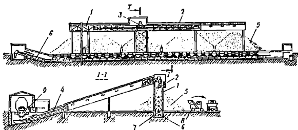
1.19-rasm. Estakada-transheyali (yerosti) noruda qurilish materiallari ombori: 1 – estakada; 2 – estakadadagi konveyer; 3 – to'kuvchi aravacha; 4 – omborga uzatuvchi konveyer; 5 – to'ldiruvchilar shtabeli; 6 – transheyaning lentali konveyeri; 7 – ochilib yopiluvchi moslama (zatvor); 8 – bir cho'michli ortuvchi; 9 – yukni qabul qiluvchi T-182A rusumli uskuna.
