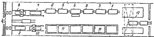
2.4-rasm. Rolikli konveyerli agregat liniya chizmasi:
