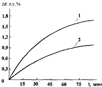
2.9-rasm. Birlamchi \Delta \epsilon_{b.ch.} cho'kishning oquvchan (1) va harakatchan (2) qorish-malarning quyilgandan keyingi o'tgan t vaqtga bog'liqligi.
