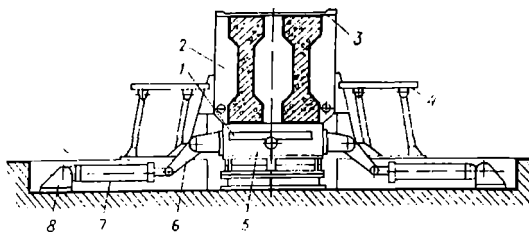
2.10-rasm. Katta o'lchamdagi temir-beton buyumlar tayyorlashda ishlatiladigan stend chizmasi:
