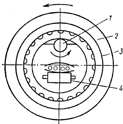
1.74-rasm. Quvumi markazdan qochma prokat bilan qoliqlash chizmasi:
