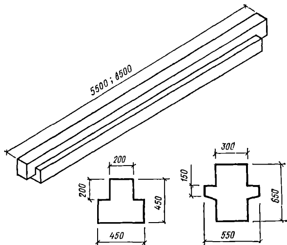
1.4-rasm. Ko'p qavatli binoning karkas rigeli.
