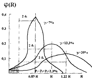
2.8-rasm. Me'yoriy qarshiliklar doimiy ta'minlanishi uchun beton o'rtacha mustahkamligining bir jinslilikiga bog'liqligi.
