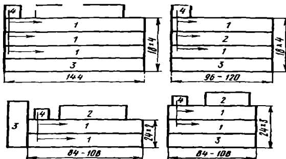
1.24-rasm. Turli quvvatdagi zavodlar bosh korpusining komponent (joylashtirish) chizmasi:
