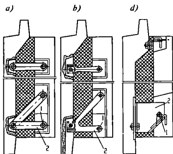
2.41-rasm. Harakatlanuvchi bog‘lanishlari panclning chekkalari (a, b) va ichkarisi (d) bo‘yicha joylashtirilgan yig‘ma panellar.
