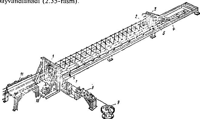
2.34-rasm. Kolonna karkaslarini tayyorlash mashinasi:
