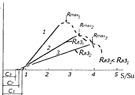
2.19-rasm. G'ovakli to'ldiruvchi oddiy (1) va yengil (2, 3) betonlar mustahkamligining suvsement nisbatiga bog'liqligi.
