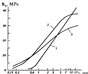
2.30-rasm. Bir xildagi faollikka ega bo'lgan va I-III mineralogik guruhlardagi (1-3 egrilarga mos holda) sementlardan tayyorlangan betonlar mustahkamligining bug' bilan ishlov berish vaqtiga bog'liqligi (yarimlogarifmik masshtabda).
