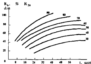
2.33-rasm. Bug'lash jarayonidagi mustahkamlik o'sishini ko'rsatuvchi egri chiziqlar: a – portlandsementda; b – shlakoportlandsemetda (egrilardagi raqamlar izotermik tutib turish C haroratini bildiradi).
