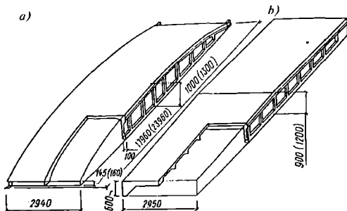
1.12-rasm. Oldindan zo'riqtirilgan "oraliqlarni yopish" plitalari. O'lchamlari: 3x18 va 3x24 m (3x24 metrli plitalar uchun o'lchamlar qavs ichida berilgan); a – KJS turi, b – II turi.
