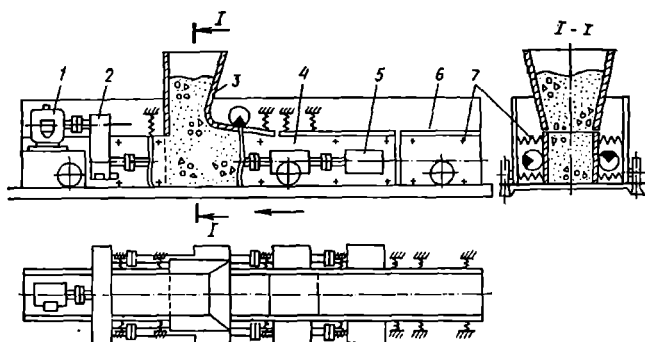
1.62-rasm. Harakatlanuvchi vibroqolipning chizmasi:
