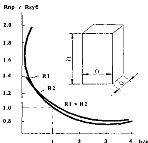
2.3-rasm. Namuna o'lchamlarining beton mustahkamligiga ta'siri.
