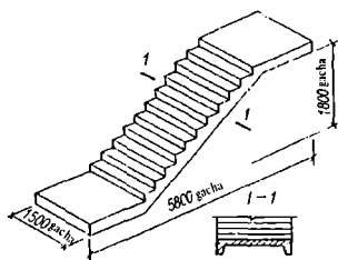
1.6-rasm. Zinapoya.
