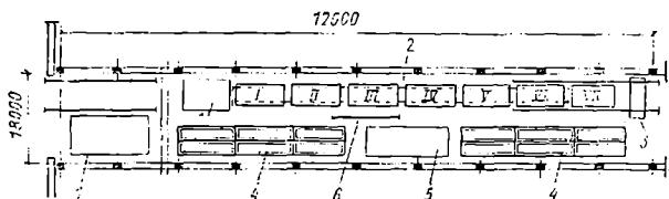
2.5-rasm. Rigellar ishlab chiqarishning yarim konveyer liniyasi:
