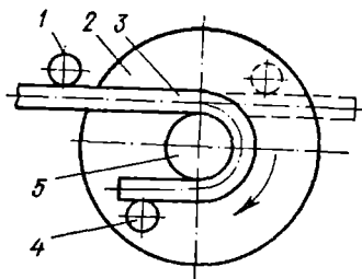
2.33-rasm. Armatura sterjenlarini bukish chizmasi: 1 – tayanch barmog'i; 2 – ishchi disk; 3 – sterjen; 4 – bukuvchi barmoq; 5 – markaziy barmoq.
