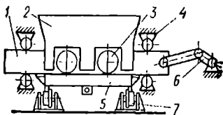
1.69-rasm. Gorizontal rolikli presslash uskunası:
