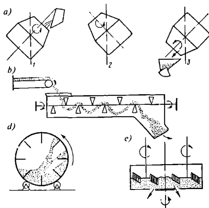
1.26-rasm. Beton qoruvchida beton qorish chizmasi:
