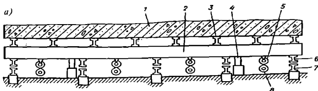
1.54-rasm. Zarba-vibratsion (rezonans) maydoncha chizmasi:
