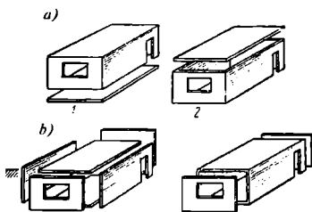
1.12-rasm. Hajmli bloklarning konstruksiyalari.
