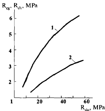
2.6-rasm. Betonning egilishga (1) R_{sgl} va cho'zilishga (2) R_{cho'z} mustahkamligining siqilishga bo'lgan mustahkamligiga nisbatan bog'liqligi.
