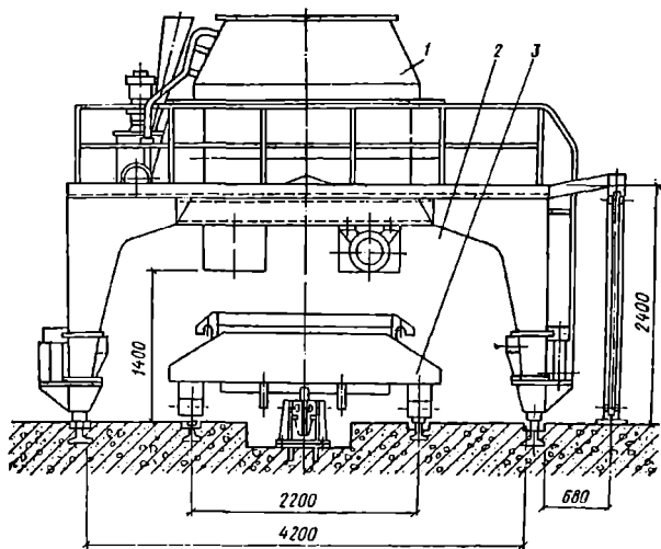
1.35-rasm. Titratib qolipaydigan qurilma:
