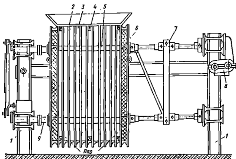
2.20-rasm. Mexanizatsiyalashgan kassetali qurilma:
