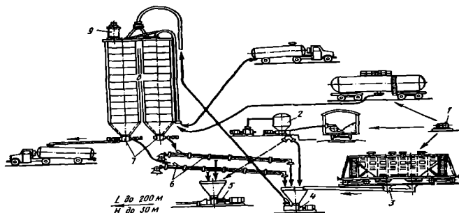
1.18-rasm. Sement omborxonasi.
