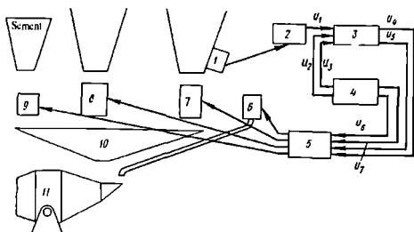
1.24-rasm. Mayda to'ldiruvchi namligini inobatga olgan holda avtomatik ravishda suv miqdorini koreksiyalovchi uskunaning prinsipial chizmasi:
