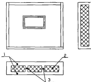
2.36-rasm. Mustahkamlik qovurg'asi bo'lgan uch qatlamli panel:
