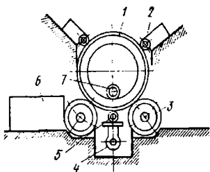
1.11-rasm. Rolikli sentrifuga.
