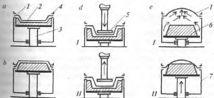
11.6-rasm. Vakuum-qoliplash sxemasi:
