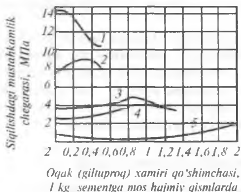
8.2-rasm. Kukun qo'shimchalarning (ohak, giltuproq) qorishma mustahkamligiga ta'sirini ifodalovchi bog'lanish.
