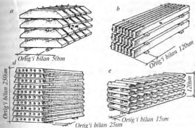
7.8-rasm. Yig'ma temirbeton konstruksiyalarni omborlarga joylashtirish:
