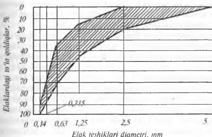
6.1-rasm. Qum donador tarkibining grafigi.
