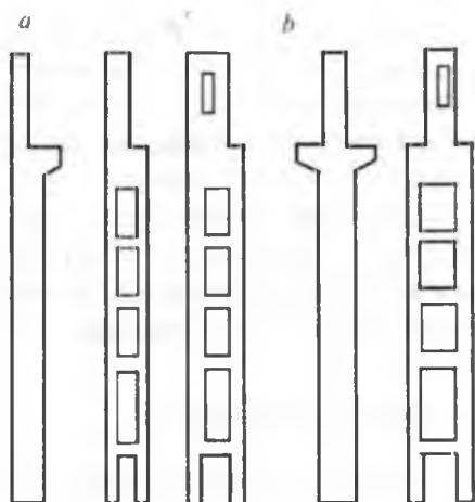
7.3- rasm. Bir va ikki tarmoqli temirbeton ustunlar:
