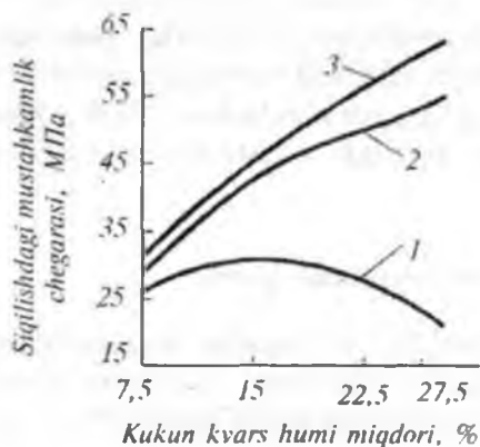
9.3- rasm. Kvars qumi kukuniligi va miqdorining silikat beton mustahkamligiga ta'siri: 1 – kvars qumining kukuniligi 1500\text{ sm}^2/\text{g} ; 2 – 2500\text{ sm}^2/\text{g} ; 3 – 4500\text{ sm}^2/\text{g} .
