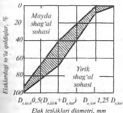
6.2-rasm. Shag'al donador tarkibi grafigi.
