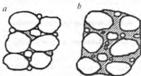
6.5-rasm. Beton qorishmasi strukturasi: a — biki; b — harakatchan.
