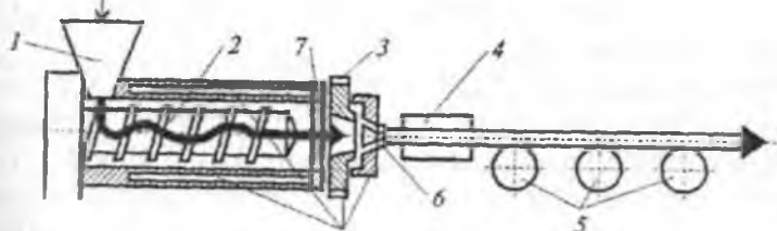
11.3-rasm. Ekstruziya mashinaning ishlash sxemasi:
