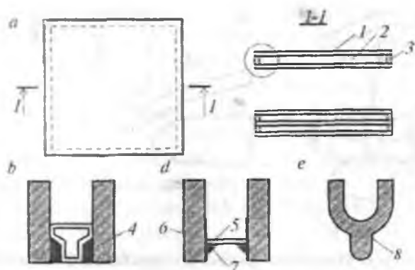
4.2-rasm. Ikki va uch qatlamli shishapaketlar (a). Shishapaket tugunlarining konstruktiv yechimi – yelimlangan (b), kavsharlangan (d) va payvandlangan (e):
