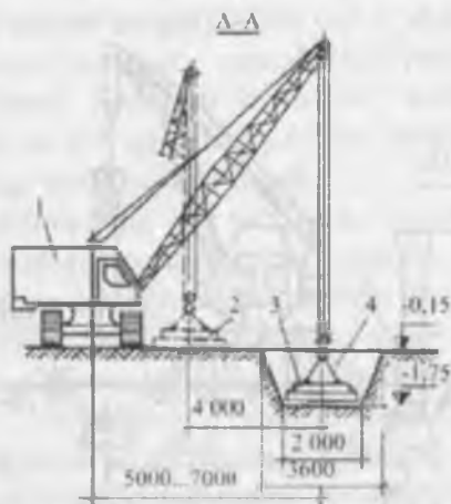
48-rasm. Stakansimon poydevorlarni montaj qilish sxemasi: 1 - montaj krani; 2 - poydevorlarni ko'tarishdan avvalgi holati; 3 - loyihaga qo'yilgan poydevor; 4 - to'rt shoxchali strop
