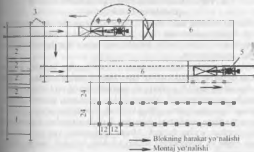
57-rasm. Bir qavatli sanoat binosi tom yopma konstruksiyalarini konveyer blok usulida montaj qilish sxemasi:
