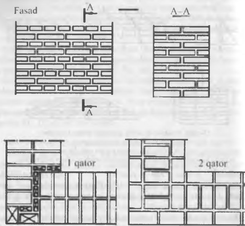
28-rasm. Bir qatorli (zanjirli) g'isht-tosh terish sxemasi
