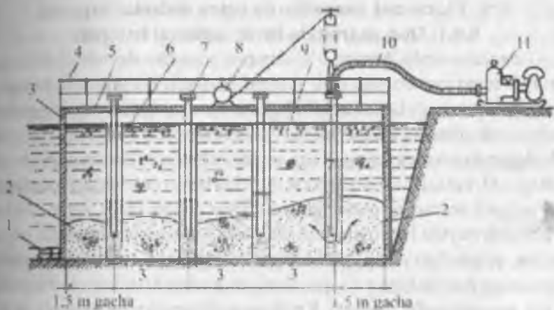
39-rasm. Ko'tariluvchi qorishma usulida betonlash sxemasi:
