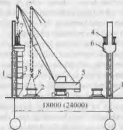
50-rasm. Kran osti to'sinlarini t'yem. n. n. n. n. o'rnatish sxemasi: 1—chyotki qator ustuni; 2—yog'och qistirma; 3—narvon; 4—kran osti to'sini; 5—montaj krani; 6—o'rta qator ustuni; 7—strop; 8—narvonni ystunga mahkamlanish joyi.
