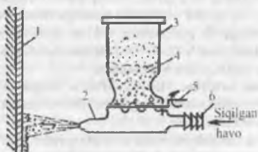
79-rasm. Bezakli suvoqni kroshka sochgich yordamida yordamida bajarish sxemasi: 1-birikturuvchi qatlami; 2-forsunka(purkagich); 3-kroshka sochgich korpusi; 4- kroshka; 5-shnekli uzatgich; 6-titashtiruvchi shtutser.
