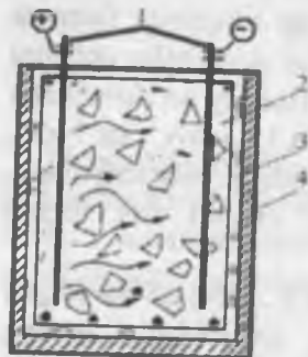
41-rasm. Betonni elektrodlar yordamida qizdirish sxemasi: 1—elektrodlar; 2—beton; 3—armatura; 4—qolip.
