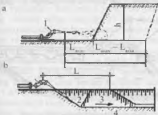
21-rasm. Hidromonitor yordamida grunt yuvish usullari a—ro'paradan yuvish, b—yuqoridan pastga yuvish. 1—gidromonitor; 2—loyda oqizish ariqchasi; 3,4—qazish krtma-ketligi
