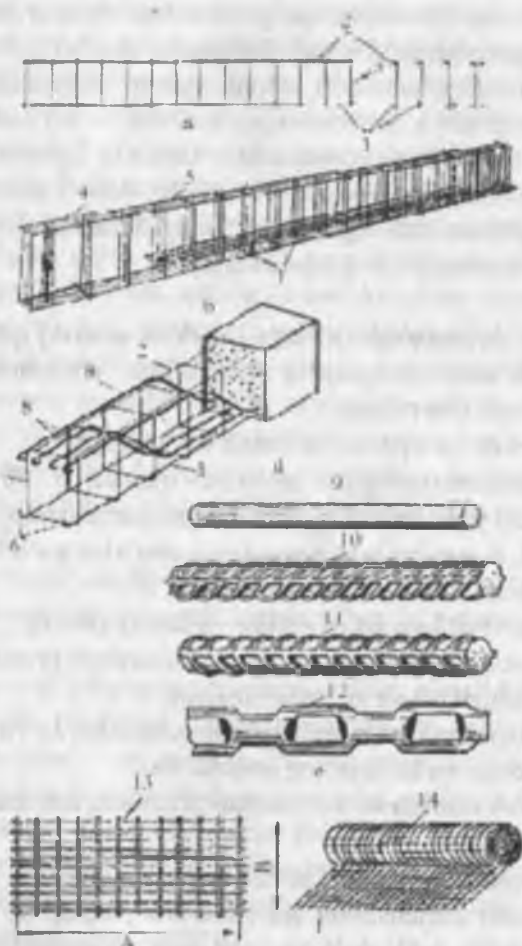
34-rasm. Armaturalarning turlari:
