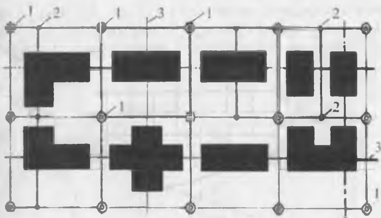
6-rasmi. Qurulish to'ri.
