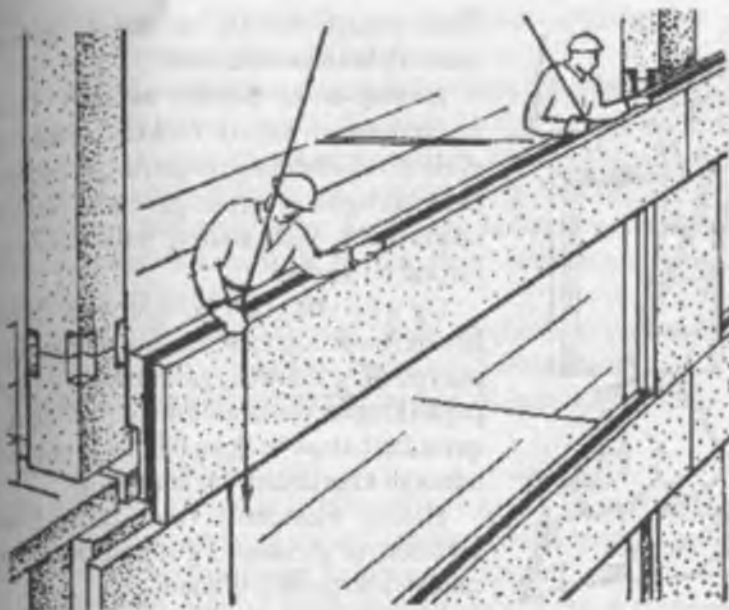
55-rasm Tashqi devor panellarini montaj qilish.
