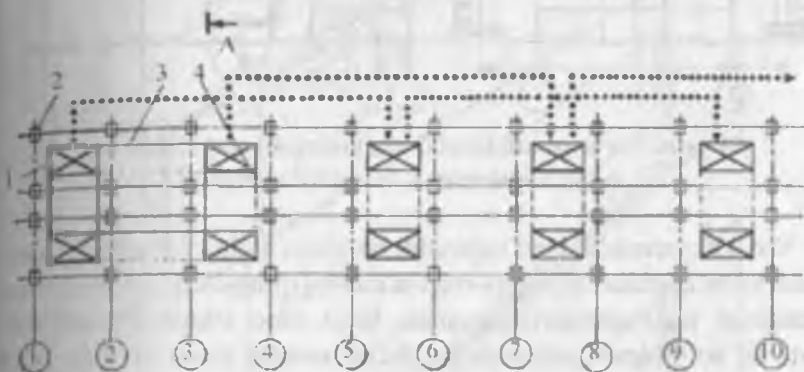
53-rasm. Guruhlangan konduktorlarning joylashish sxemalari (strelka bilan konduktorlarni ko'chirib o'rnatilish yo'nalishi ko'rsatilgan):
