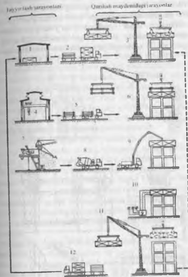
32-rasın. Beton va temir-beton ishlarini bajarishning texnologik ketma-ketligi: 1, 2, 3-qoliplarni tayyorlash, tashish va o'rnatish; 4, 5, 6-armaturalarni tayyorlash, tashish va o'rnatish; 7, 8, 9-beton qorishmani tayyorlash, tashish va joylashtirish; 10-betonning qotishini ta'minlash; 11-qoliplarni ajratib olish; 12-qoliplarni ta'mirlashga jo'natish.
