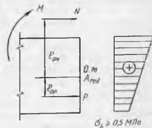
11.5-расм. Нормал дарзларнинг беркилишига доир
