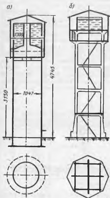
18.5-расм. Босимли сув минораси:
