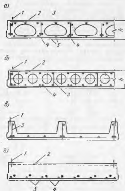
14.2-рasm. Ораёпма панелларнинг кесимлари ва уларни арматуралаш: а-овал бўшлиқли; б-доиравий бўшлиқлар; в-юқорига қараган қовурғали; г-яхлит; 1-кўтариш учун илмоқлар; 2 — сиқилган қисмидаги тўр; 3 — «лесенка» типдаги вертикал тўр; 4 — зуриктириладиган арматура; 5-чўзилган қисмидаги тўр.
