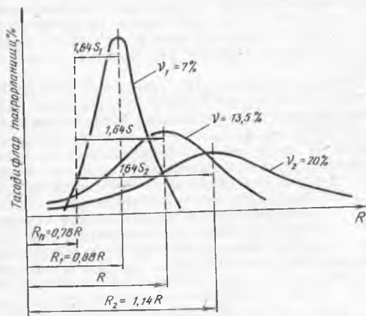
3.4-расм. Вариация коэффициентлари v турлича бўлганида нормал тақсимланиш эгри чизиклари ва белгиланган меъёрий қаршилиқ R_n ҳосил қилишни таъминлайдиган бетон ўртача мустаҳкамлиги R нинг тегишли қийматлари
