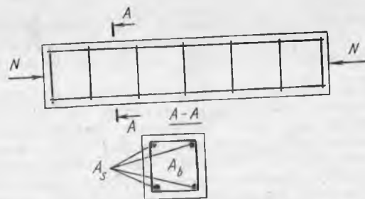
4.1-расм. Темир-бетон элементнинг ўқий сиқилиши
