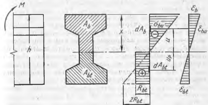
5.1-расм. Кучларнинг таъсир чизиқлари ва эгиладиган бетон элементнинг қўндаланг қесимидаги кучланишлар ва деформацияларнинг схемалари
