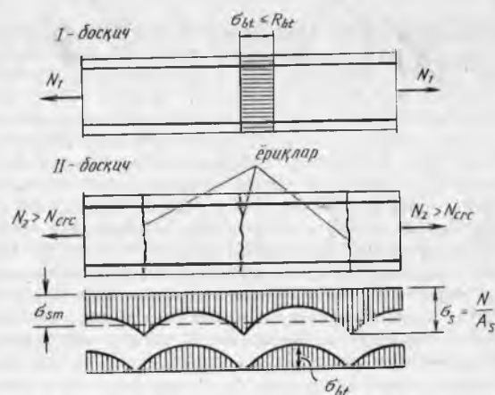
4.2-расм. Ўқий чўзилишдаги кучланганлик ҳолати
