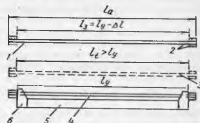
9.1-расм. Арматурани электротермик усулда таранглаб тортиш схемаси:
