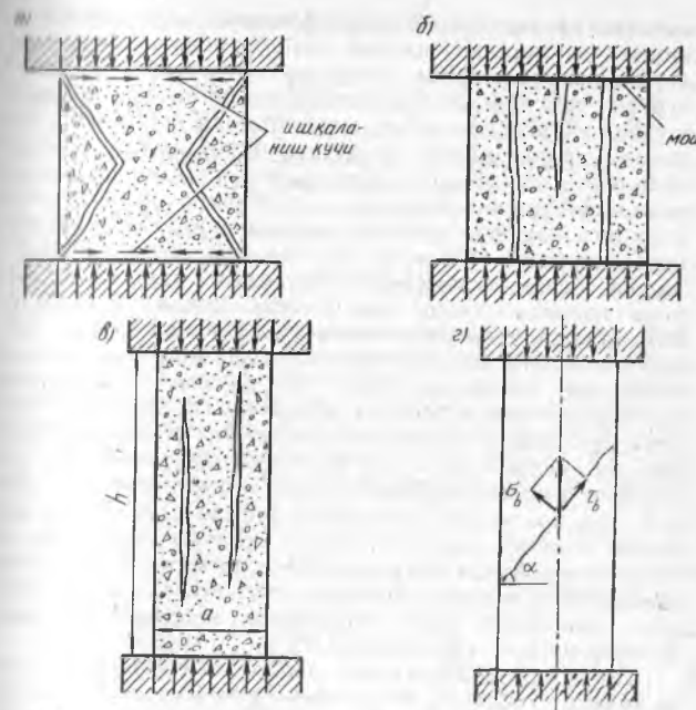
3.2-расм. Бетон куб ва призмаларни сиқилишда емирилиш схемалари
