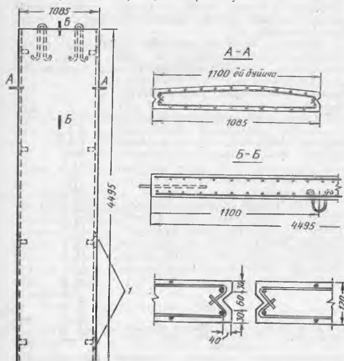
18.3-расм. Йиғма резервуарнинг деворчалари панели
