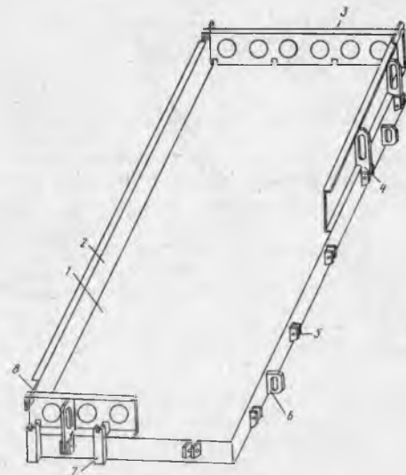
20.5-расм. Олдиндан зўриктирилган арматурали темир-бетон серковак панелларни тайёрлаш учун пўлат қолип: 1 — таглик; 2 — буйлама борт; 3 — торец борт; 4 — шарнир скобаси; 5 — пружина; 6 — кўтариш скобалари; 7 — тирак; 8 — қулф
