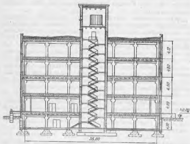
17.3-расм. Тўснли ораёнмали ром тизимли кўп қаватли синчли бино (ўлчамлар метр ҳисобида)
