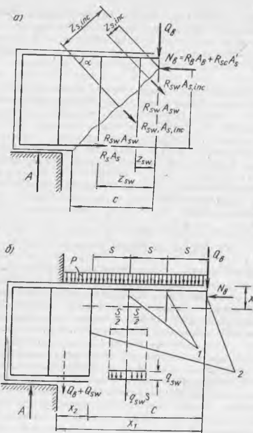
6.10- расм. Кия кесимларнинг мустаҳкамлигини ҳисоблашга доир. а — кия кесимда таъсир этувчи кучларнинг схемалари; б — Q_b + Q_{sw} ни аниқлашга доир; 1 — ишда иштирок этувчи кўндаланг стерженлар; 2 — дарз кесиб ўтган четки кўндаланг стерженлар
