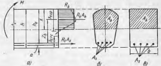
6.7- расм. Якка арматурали элементни ҳисоблашга доир.
