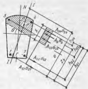
8.3-расм. Кийшиқ номарказий сиқилишда таъсир этувчи кучларнинг схемаси
