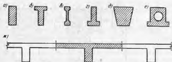
6.1- расм. Темир-бетон тўсинлар қўндаланг кесимларининг турлари
