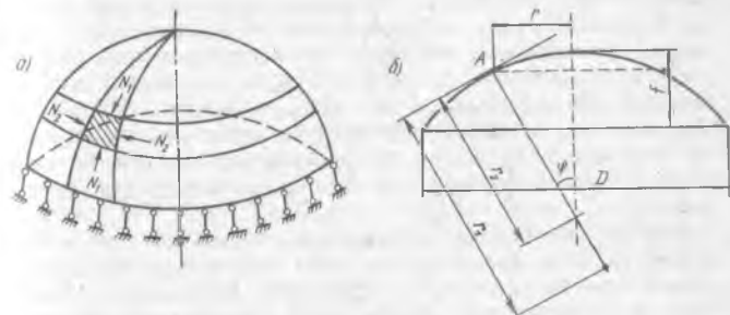
15.16-расм. Гумбазни моментсиз назария бўйича ҳисоблашга доир а — меридиан ва доиравий кучларнинг жойлашиши; б — ҳисоблаш учун белгилашлар.
