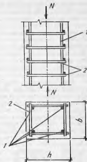
7.1-рasm. Сиқилган темир-бетон элементларни арматуралаш: 1 — бўйлама арматура; 2 — хомутлар
