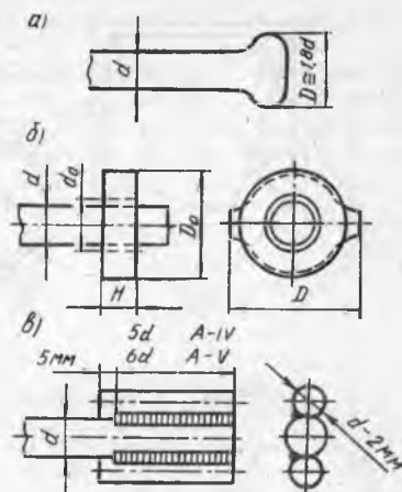
9.3-расм. Зўриктириладиган стержень арматурадаги вақтлик технологик анкерлар
