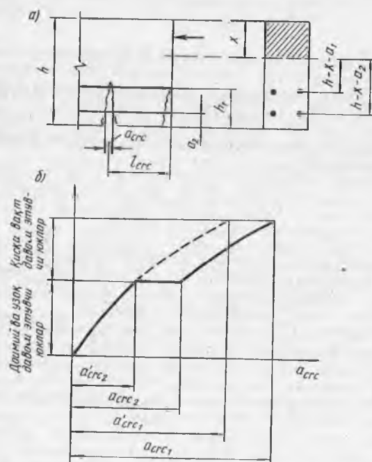
11.4- расм. Дарзларнинг очилиши энини аниқлашга доир: а — дарзларнинг очилиш схемаси; б — юкларнинг узок муддатли ва қисқа муддатли таъсирида дарзларнинг очилиш графиклари
