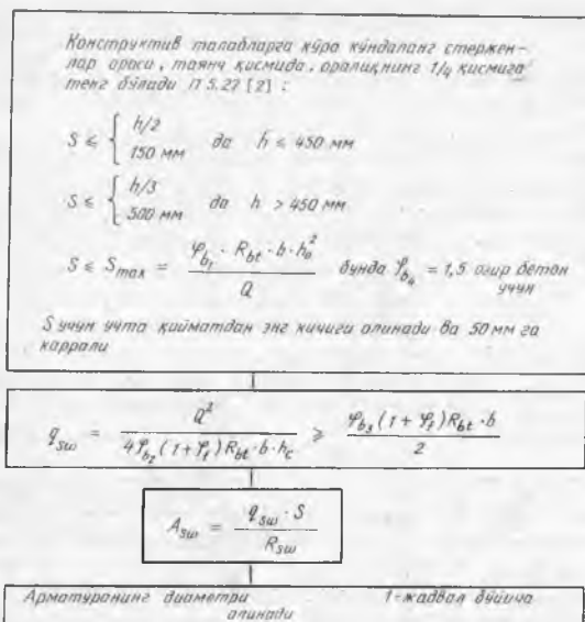
23.5-расм. Таврсимон кесимли элементлар кўндаланг арматураси қадамини ва арматура кўндаланг кесимини аниқлашга доир блок-схема
