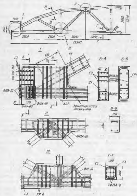
15.4-расм. Синик қиёфали юқориғи белбоғи бўлган сегментсимон панжарали ферма
