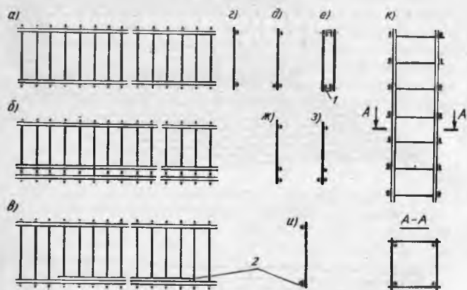
3.16-расм. Пайванд арматура буюмлари: 1,2 — пайвандлаш
