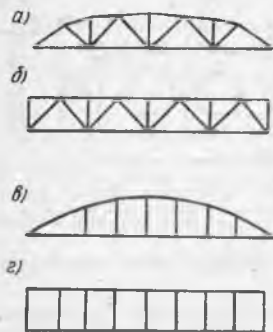
15.4- расм. Фермаларнинг схемалари
