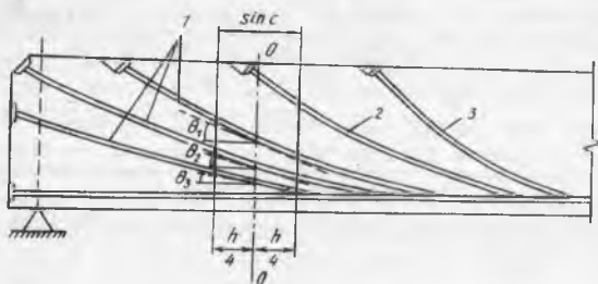
11.3-расм. О — О кесими бош чўзувчи кучланишлар бўйича ҳисоблашда назарда тутиладиган арматураларнинг жойлашиш схемаси:
