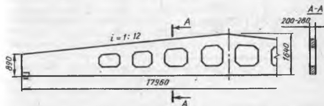
15.3-расм. Олдиндан зўриктирилган икки нишабли панжарали тўсин
