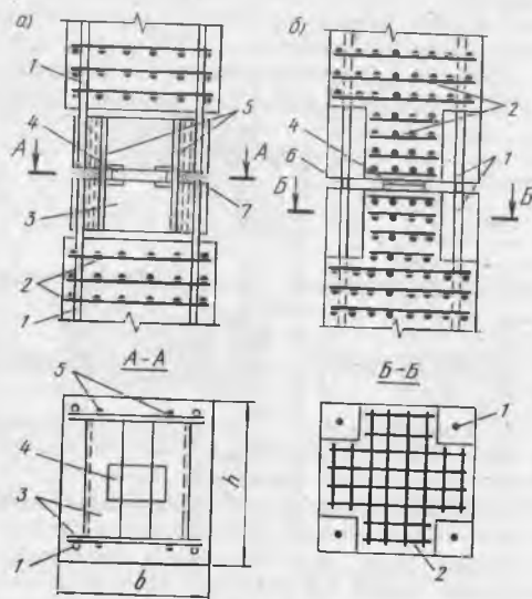
17.5-расм. Устунларнинг бикр уланган жойлари:
