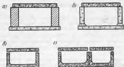
18.10-расм. Каналларнинг турлари: а — гинт деворчали; б — бетон деворчали; в — бир қатқачали темир-бетон нов; г — икки қатқачали темир-бетон нов
