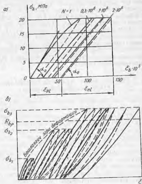
3.6-расм. Кўп марта такрорий юклашда ва юкни олишда бетоннинг деформацияланиши
