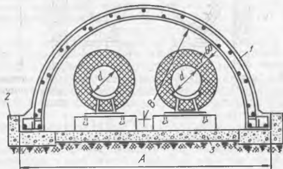
18.11-расм. Йиғма темир-бетон гумбазлардан иборат канал: 1 — темир-бетон гумбаз; 2 — лентасимон пойдевор; 3 — бетон таглик
