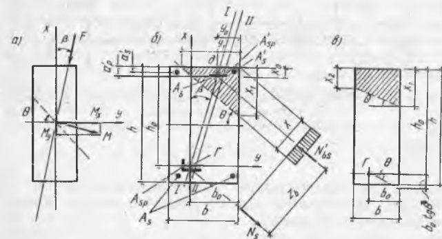
8.1-расм. Қийшиқ эгилишга мўлжаллаб тўпланган арматури темир-бетон элементларни ҳисоблашга доир:
