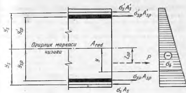
10.1-расм. Олдиндан зўриктирилган элементда кучланишларни аниқлашга доир.
