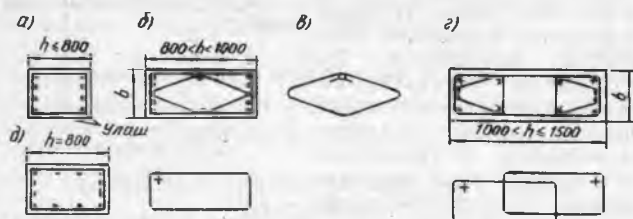
7.2-расм. Сикилган устунларнинг тўғри тўртбурчак кесимини арматуралаш.
