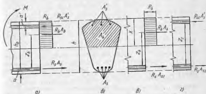
6.8-расм. Қўшалок арматурали элементни ҳисоблашга доир.
