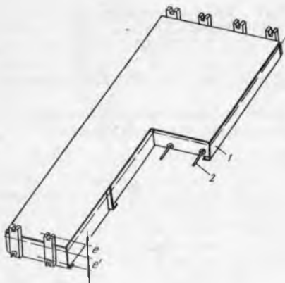
20.6- расм. Олдиндан зўриктирилган қалипнинг таглиги (бортлар шартли равишда кўрсатилмаган): 1 — таглик; 2 — тортки; 3 — тирак
