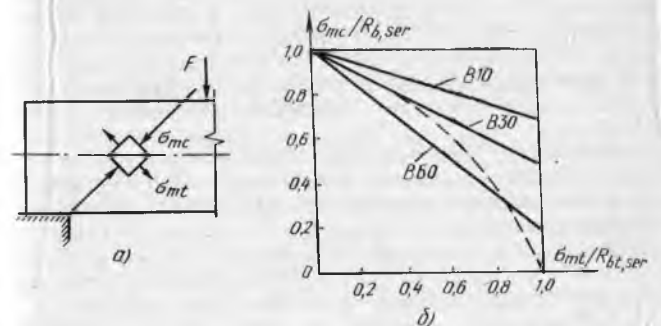
11.2-расм. Қия дарзлар пайдо бўлиши бўйича ҳисоблашга доир: а — текис кучланганлик ҳолатининг схемаси, б — чўзилишда оғир бетоннинг нисбий мустаҳкамлигининг перпендикуляр йўналишдаги сиқувчи кучланишлар сатҳига боғлиқлиги графиклари
