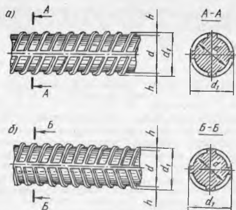
3.11-расм. Ўзгарувчан кесимли киздириб прокатланган арматура пўлати
