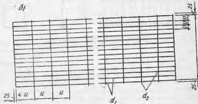
3.15-расм. Пайванд арматура тўрлари а — ўрама; б — текис
