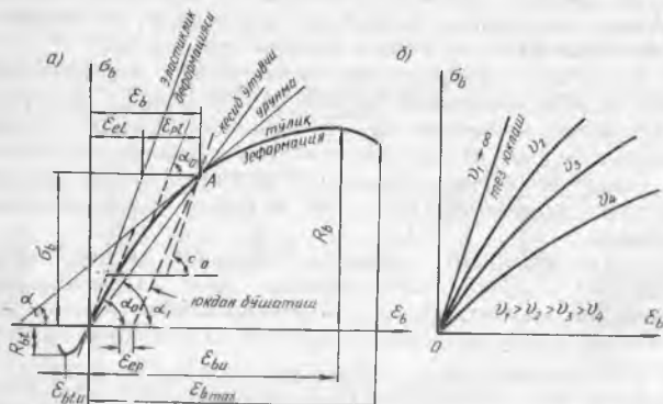
3.5-расм. С қилишда бетон кучланишлари — деформацияларнинг диаграммалари
