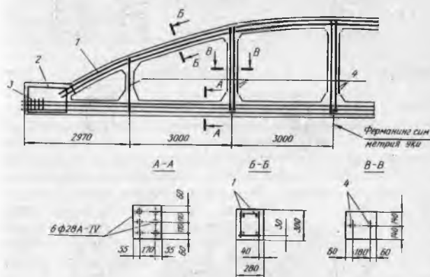
15.5-расм. Олдиндан зўриктирилган пастки белбоғи ва тирговичи бор тираксий фермаларни арматуралаш мисоли:
