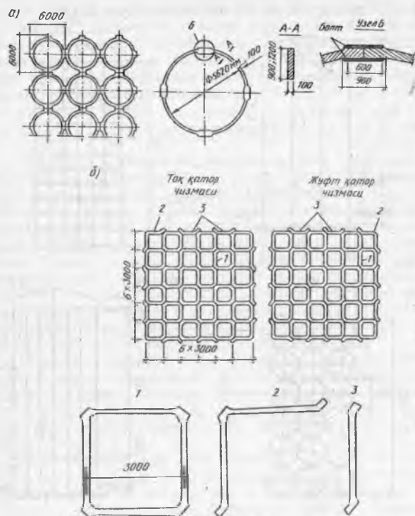
18.9-рasm. Йиғма силос корпуслари:
