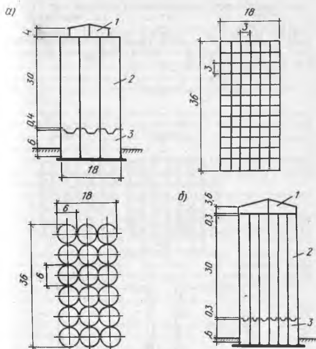
18.8-расм. Силосларнинг схемалари:
