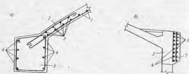
15.17-расм. Бир бутун (яхлит) гумбазларни арматуралаш:
