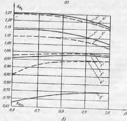
3.9-расм. Дастлабки сиқишнинг бошлангич даражаси \eta = b\rho/R_{bp}(a) ва бетоннинг нисбий узатиш мустаҳкамлиги \beta = R_{bp}/R(b) га кўра бетон мустаҳкамлик хоссаларининг ўзгариши:
