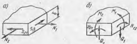
15.11-расм. Қобик кесимларида таъсир этувчи қучлар а — бўйлама ва силжитувчи қучлар; б — этувчи моментлар ва қўндаланг қучлар.
