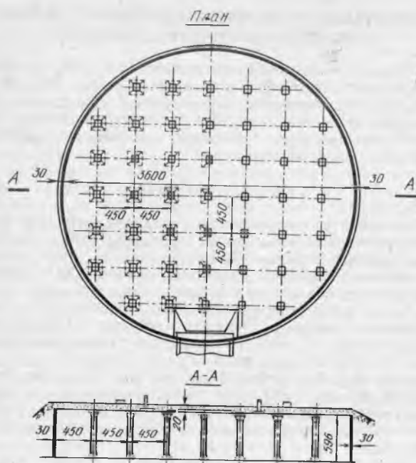
18.1-расм. Текис тўсинсиз ораёпмали доиравий резервуар
