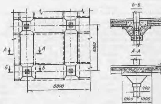
14.11- расм. Тўсинсиз йиғма ораёпмалар
