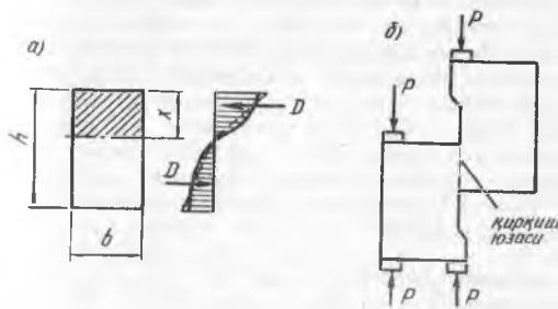
3.3-расм. Бетоннинг мустаҳкамлигини аниқлашга доир: а — эгилишда; б — кесилишда
