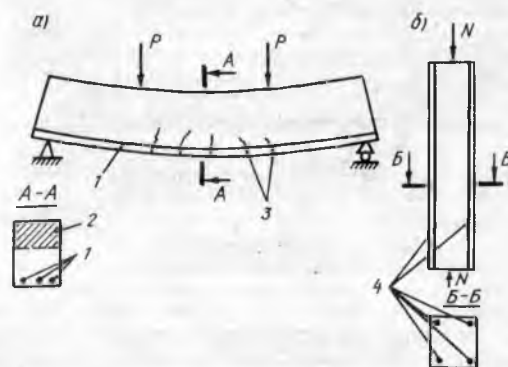
2.1-расм. Темир-бетон элементларда асосий (ишчи) арматурасининг жойлашиши: а — эгилишда; б — сиқилишда
