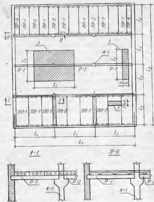
23.2-расм. Ораёпма плани ва қирқимлар
