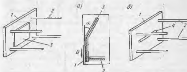
3.17-расм. Темир-бетон буюмларнинг қўйма деталлари: а — буктилган устма-уст қўйилган анкерли; б — нормал анкерлар ва пўлат тиракли; 1 — пўлат пластинка; 2 — нормал анкерлар; 3 — буктилган анкер; 4 — арматура қозғидан қилинган тирак; 5 — пўлат пластинадан қилинган тирак
