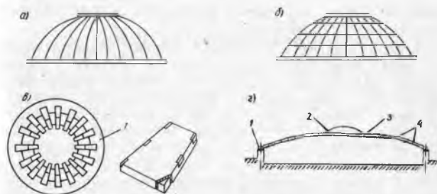
15.18-расм. Йигма гумбазлар:
