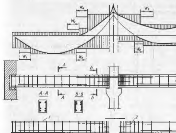
14.4- расм. Узлуксиз (туташ) ригелни арматуралаш:
