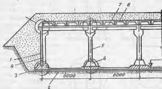
18.4-расм. Панель — тўсин ораёпмали йиғма тўғри тўртбурчак резервуарнинг конструктив ечими:
