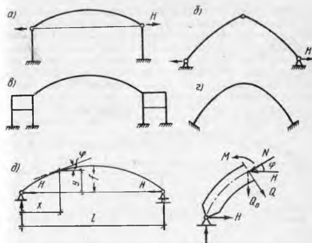
15.7-расм. Аркаларнинг схемалари ва улардаги таъсир этувчи кучлар а — торткичи; б, в, в — таянчи; д — ҳисобий схема.
