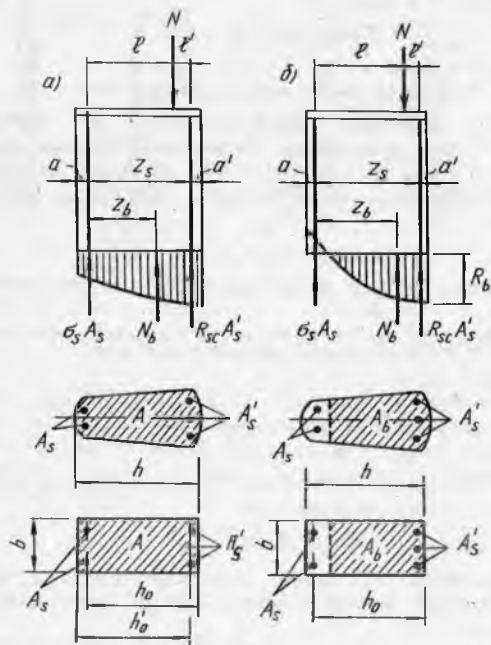
7.5-расм. Сиқилган элементнинг кўндалағ кесимида кучларнинг таъсир қилиш схемаси.
