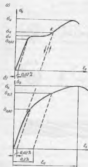
3.13-расм. Пўлат арматура қўзилишининг ўзига хос диаграммалари: а — оқувчанлик чегараси бўлганда, б — бўлмаганда.
