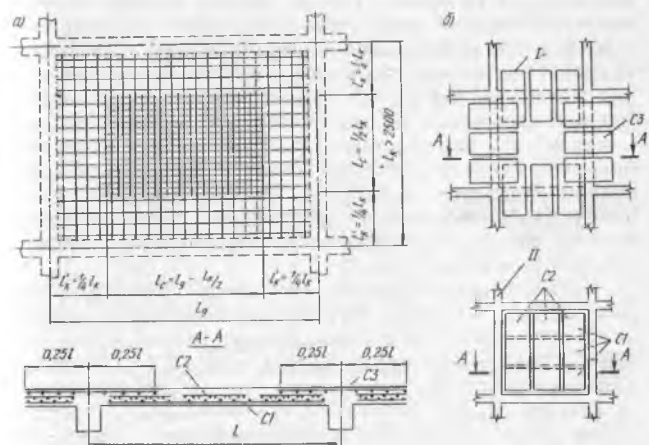
14.9-расм. Контур бўйича тиралган плиталарни арматуралаш:
