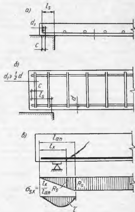
6.12- расм. Эгиладиган элементлар эркин тиралганида бўйлама чўзилган арматура билан анкерлаш. а — плита; б — тўсин; а — арматурани бетонга анкерлаш қисмининг бутун узунлигида кучланишларнинг ўзгариши
