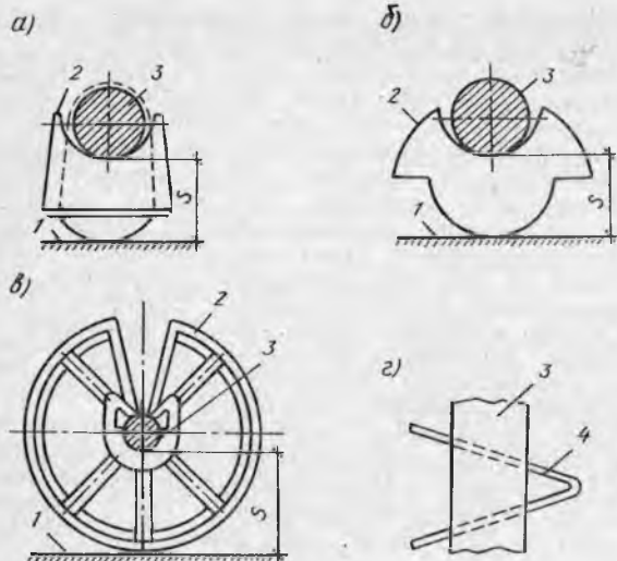
19.1 расм. Темир-бетон конструкциялар тайёрлашда арматуранинг вазиятини котиригичлар:
