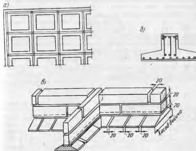
16.4-расм. Лентасимон пойдеворлар:
