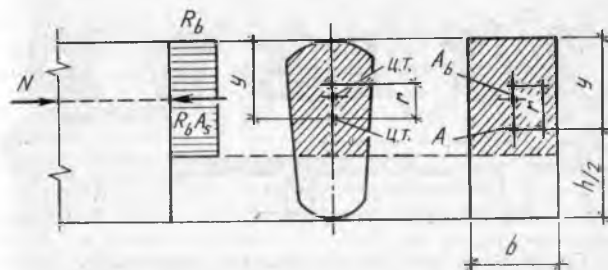
5.2-расм. Кучларнинг таъсир чизиклари ва сиқилган бетон элементнинг қўндаланг кесимидаги кучланишлар эпюраси
