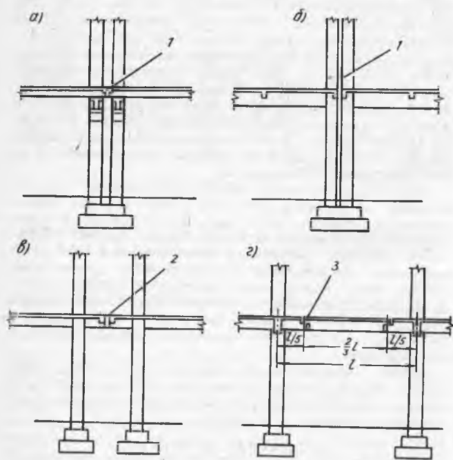
13.2-расм. Деформация чоклари:
