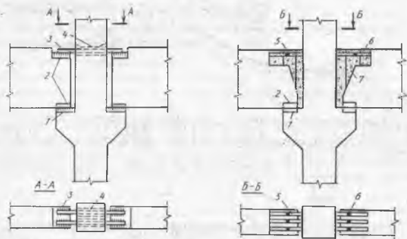
14.3- расм. Ригелнинг устун билан уланиш жойи:
