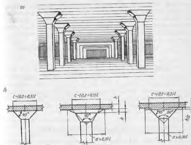
14.10- расм. Тўсинсиз ораёпмалар: а — тўсинсиз ораёпмали хоналарнинг ички кўриниши; б — бир бутун ораёпма бўлганида капителларнинг тури
