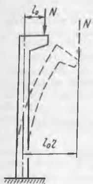
7.6- расм. Букилувчан элементларда бўйлама куч эксцентриситетининг ортиши.
