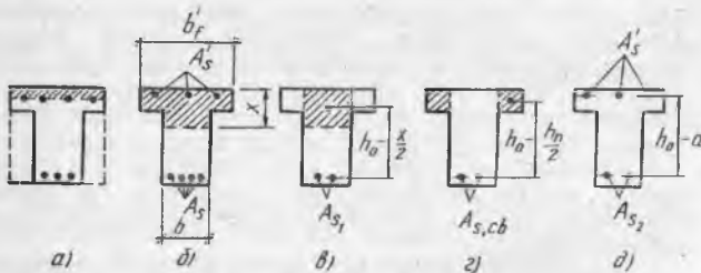
6.9-расм. Таврсимон кесимли элементни ҳисоблашга доир.
