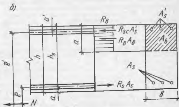
7.7-расм. Чўзилган элементларнинг кўндаланг кесимида кучларнинг таъсир қилиш схемаси:
