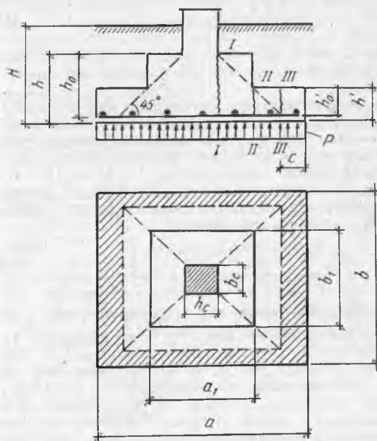
16.3-расм. Алоҳида пойдеворни ҳисоблашга доир
