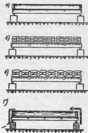
21.2-расм. Тенг тақсимланган синов юкларининг турлари:
