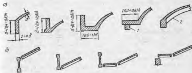
15.14- расм. Цилиндрик қобиклар борт элементларининг турлари: а — яхлитлариники; б — йиғмалариники; 1 — таянч; 2 — қовурға
