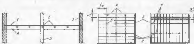
14.5-расм. Тўсин плитали яхлит (бир бутун) қовурғали ораёпмаларнинг схемалари:
