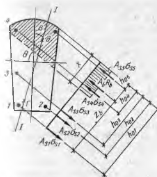
8.2-расм. Эйиб арматураланган, кийшиқ эгиладиган темир-бетон элементларда таъсир этувчи кучларнинг схемаси
