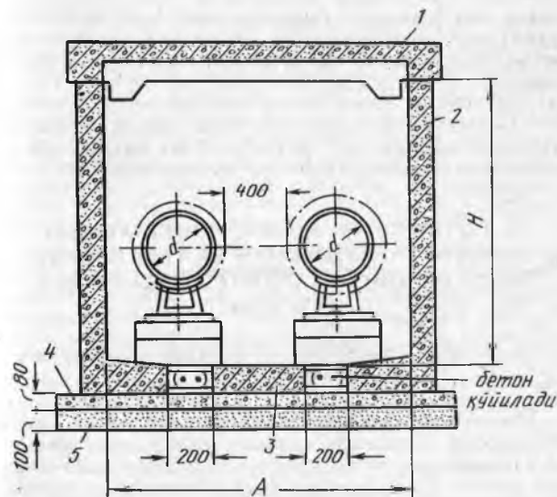
18.12-расм. Йиғма темир-бетон блоклардан иборат ярим ўтишли канал: 1 — ораёпманинг қовурғали блоқи; 2 — девор блоқи; 3 — таглик блоқи; 4 — бетон тўшама; 5 — чақик тош тўшама
