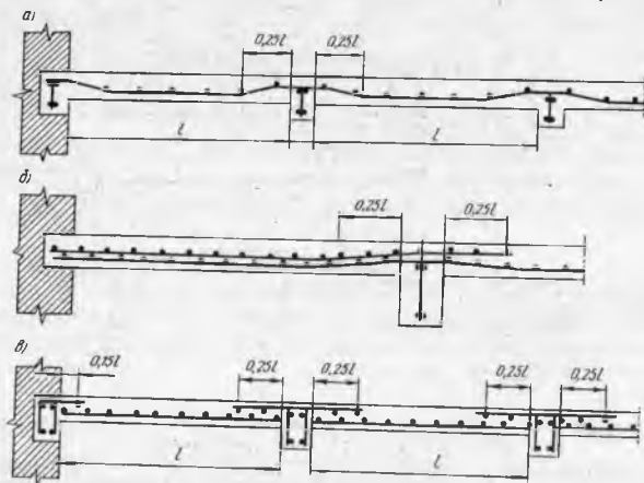
14.6- расм. Тўсин туташ плиталарини арматуралаш
