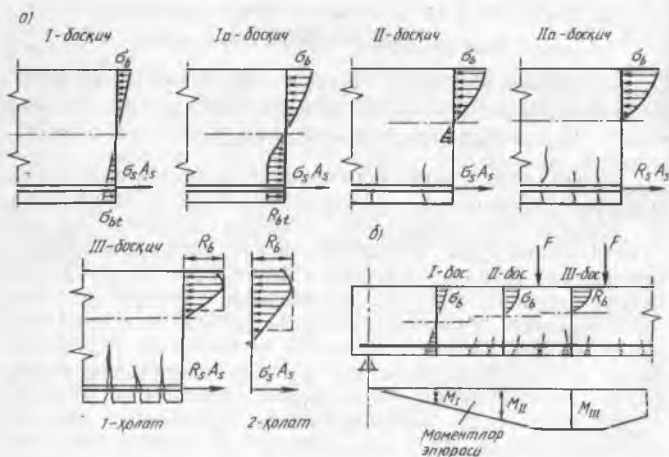
4.3- расм. Эгилишда кучланганлик ҳолатининг боскичлари
