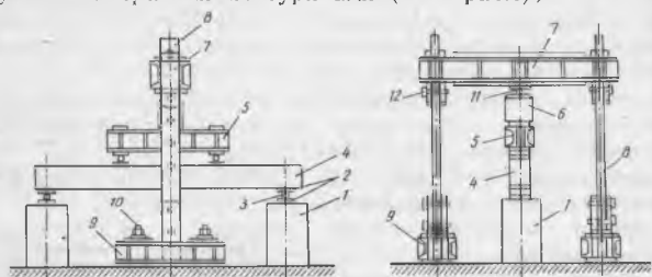
21.1-расм. Тўсинларни стационар стендларда синаш
