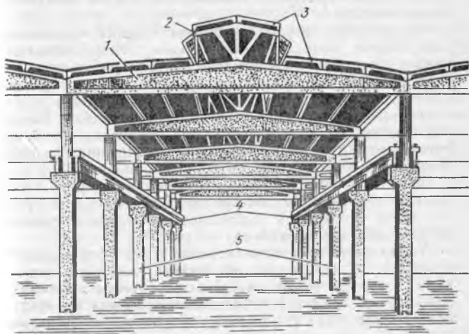
17.1-расм. Йиғма темир-бетон элементлардан қурилган бир каватли синчли саноат биноси:
