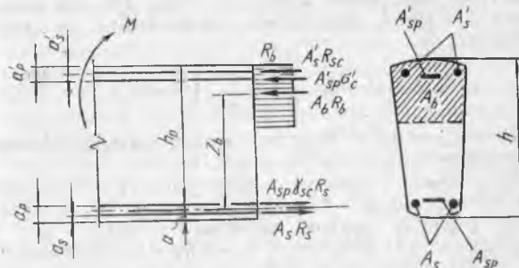
10.3-расм. Мустаҳкамликка ҳисоблашда кучларнинг схемаси ва олдидан зўриктирилган эгиладиган элемент кўндаланг кесимидаги кучланишлар эпюраси
