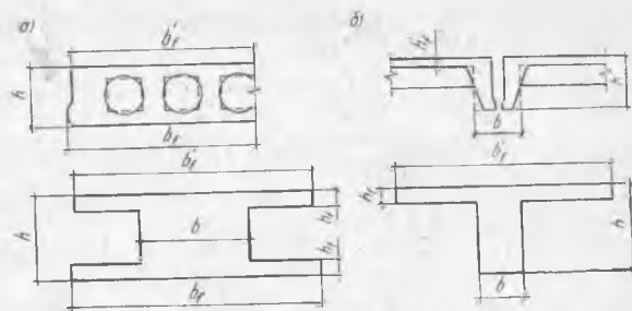
23.3-расм. Ораёпма панеллари кесимини эквивалент панелларга келтириш:
