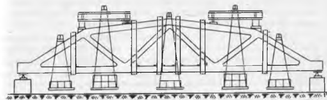
21.3-расм. Фермаларни осма платформадаги юклар билан синаш
