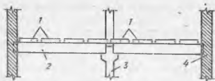
14.1-рasm. Тўснли йиғма панель ораёпмаларнинг конструктив схемаларини жойлаштиш вариантлари: 1-панель, 2-ригель, 3-устун, 4-деворлар
