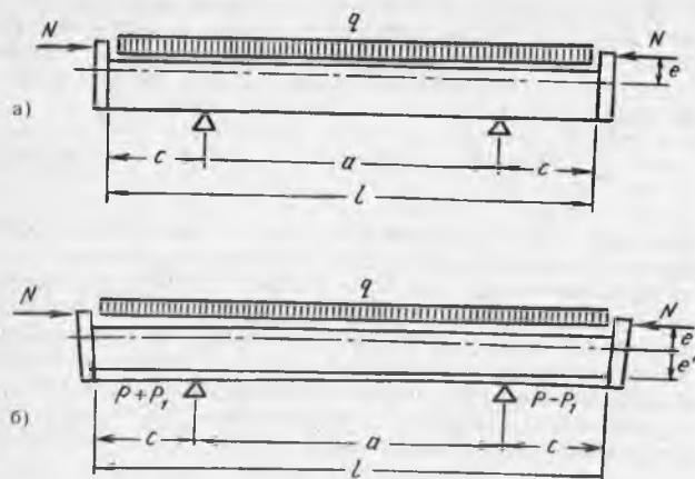
20.9-расм. Пўлат қолипларни ҳисоблаш схемаси:
