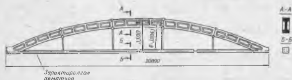
15.8-расм. Тортқиси олдиндан зўриктирилган темир-бетон арка
