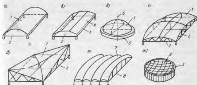
15.9-расм. Юпка деворли фазовий темир-бетон ёпмаларнинг турлари:
