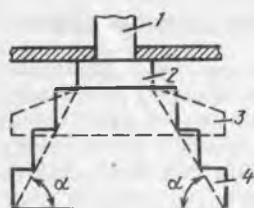
16.1-расм. Бетон пойдевори темир-бетон пойдевор билан алмаштирганда баландликнинг камайиши:
