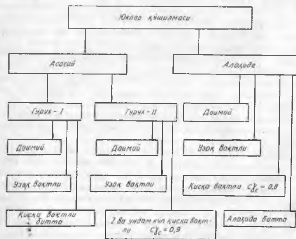
1.3-расм. Юklarнинг қўшилиб (биргаликда) таъсир этиш схемалари
