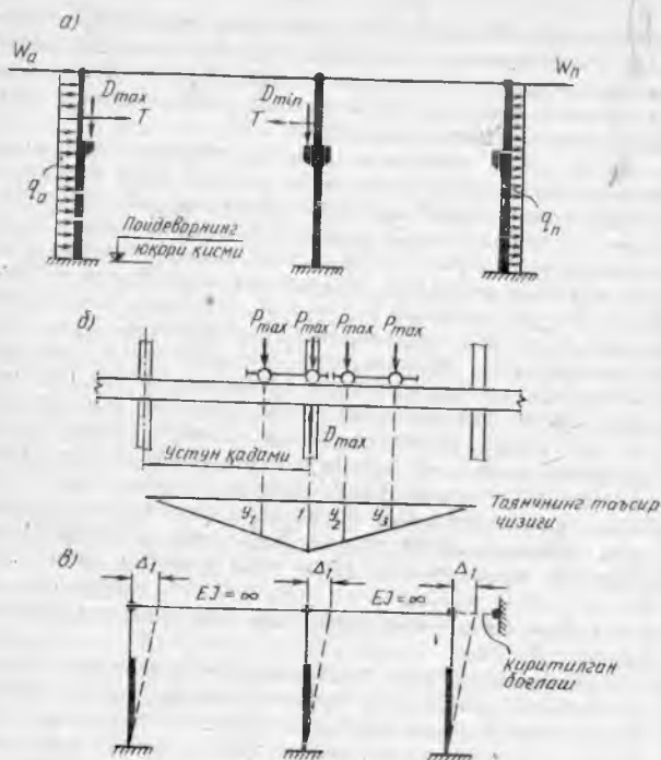
17.2-расм. Йиғма темир-бетон элементлардан қурилган бир қаватли синчли бинонинг ҳисобий схемаси: а — қўндаланг ром; б — бўйлама қирсим элементи; в — силжишлар усулининг асосий тизими
