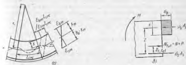
12.1- расм. Элементнинг эгриликларини аниқлашга доир
