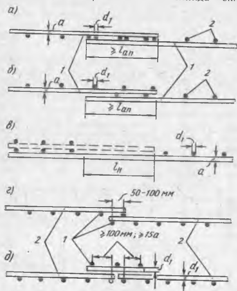
3.18-расм. Устма-уст қўйилган пайвандланган тўрларнинг уланган жойлари (пайвандсиз): а, б, в — иш йўналишида; г, д — тақсимловчи арматура йўналишида; 1 — ишчи арматураси; 2 — тақсимлаш арматураси
