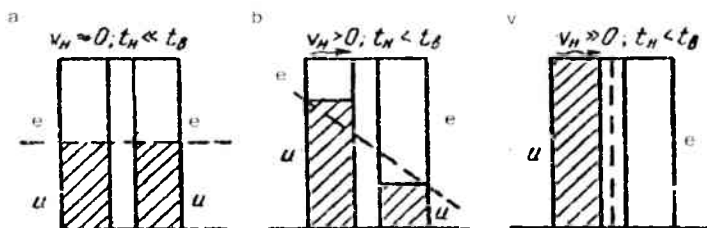
12.5-rasm. Bino fasadida joylashgan infiltratsiya va eksfiltratsiya zonalar: a-shamol ta'sirida kichik bosim bo'lganda; b- 0 < P < 1 bo'lganda v- binoni shamollatishda.
