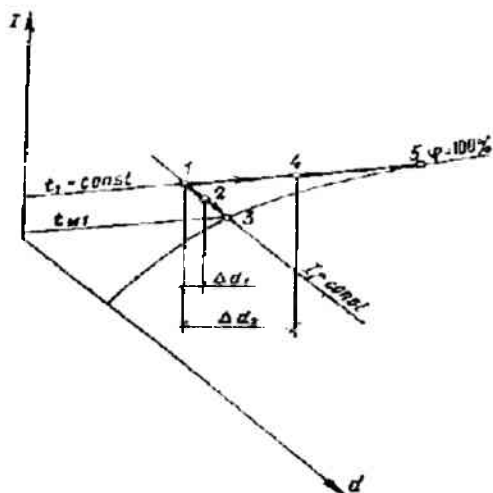
3.5-rasm. Havoni izoentalpiyalik va izotermik namlanish rejimi ko'rsatilgan I-d diagrammasi.
