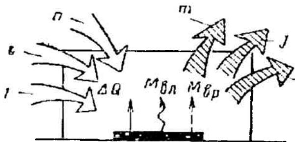
4.1- rasm. "n" havo kiruvchi va "m" havo chiqaruvchi tirqishlar va tizimlarga ega bo'lgan xonani ventilatsiyasini sxemasi.
