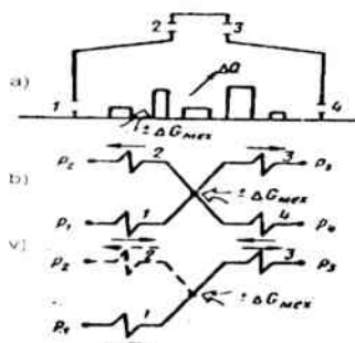
13.1-rasm. Sanoat binosining vertikal qirqimi (a) va binoning tashqi havo bilan bog'liqlik sxemalari P_4 > P_0 > P_2 (b) va P_3 < P_0 (v) bo'lganda havoning yo'nalishi ko'rsatilgan.
