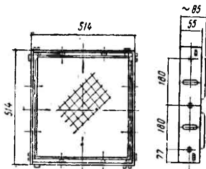
10.11-rasm. Uyali filtrlar FyaP va FyaR
