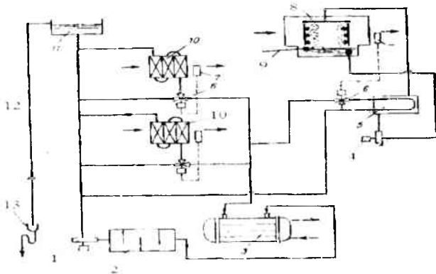
18.9-rasm. Havo konditsiyalash uskunalaridagi sirtli issiqlik almashish va purkash (VTMO-3) bo'limini (OKF-3) sovuq bilan ta'minlashdagi yopiq chizma. 1-sovutish stansiyasining nasosi, 2-bak-kompensator, 3-isparitel (bug'latgich), 4-purkash bo'limining nasosi, 5-suv-suvli issiqlik almashgich, 6-uch yo'lli klapan, 7- nazorat qiluvchi ko'rsatkich, 8-OKF-3 purkash bo'limi; 9-suv manbai, 10-sirtli sovutish bo'limi (VTMO-3), 11-kengayishi idishi, 12-suv toshishi quvuri; 13-oqova suv uchun varonka.
