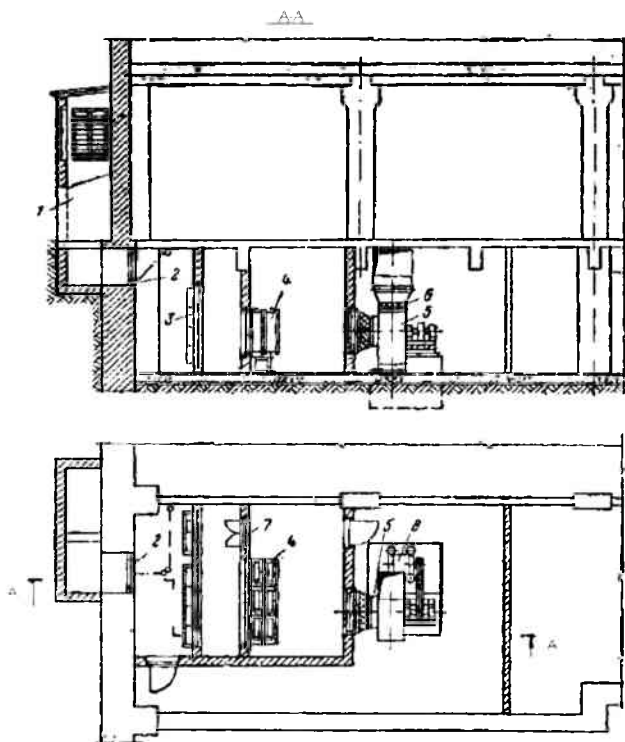
7.4-rasm. Yerto'lada joylashgan oqib kelish kamerasi.
