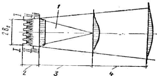
6.10-rasm. Panjara bilan berkitilgan tirqishdan chiqayotgan oqimni shakllanishi va rivojlanishi.
