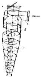
10.2-rasm. Siklonni sxemasi.
