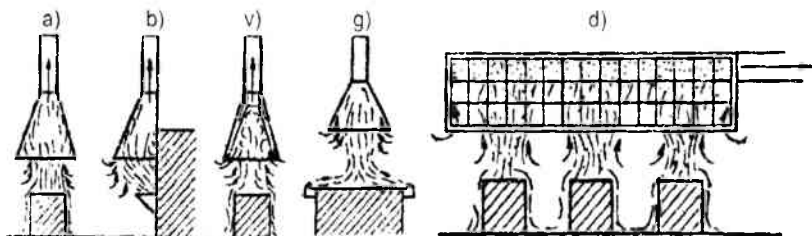
11.3-rasm. Soʻrish zontlar. a) oddiy individual zont; b) zont – kozirek; v) aktiv zont (perimetr boʻyicha tirqishlar bor); g) zont oqimli (co сдувом воздуха); d) guruhli zont.
