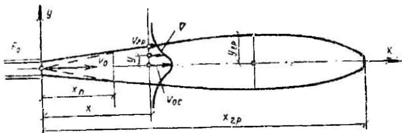
6.3-rasm. Erkin izotermik oqimni sxemasi.
