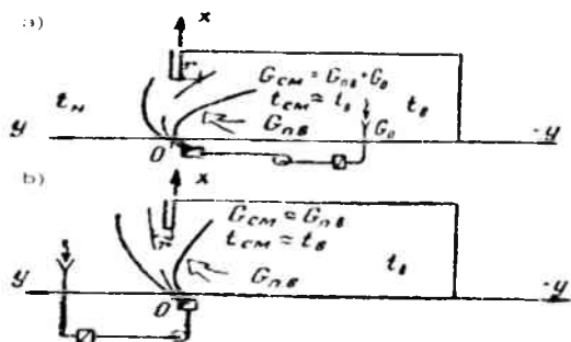
14.4-rasm. Vaqti bilan ishlaydigan havo pardalarni sxemalari. a) xonadan havo olish; b) tashqaridan havo olish ( G_o -pardaga xonadan olinadigan havo miqdori; G_{rm} -parda oqimi so'rib olinayotgan ichki havoni miqdori; G_{sm} -parda oqimi bilan xonaga kirayotgan havo miqdori; t_n -xonaga kirayotgan parda oqimini qismidagi havoni o'rtacha harorati; r -oqim mag'zini yarim eni).
