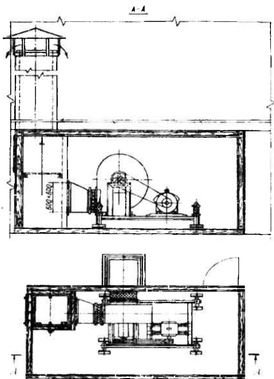
7.7-rasm. Radial ventilatorli soʻrib chiqarish kamerasi.
