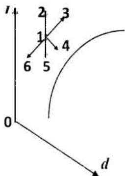
3.6-rasm. Nam havo holatining xarakterli o'zgarishlari. 1-2 – quruq isish; 1-3 – namlanib isish; 1-4 – adiabatik namlanish; 1-5 – quruq sovush; 1-6 – quritilib sovush.
