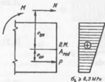
8.4-rasm. Normal yoriqlarni yopilishga doir.
