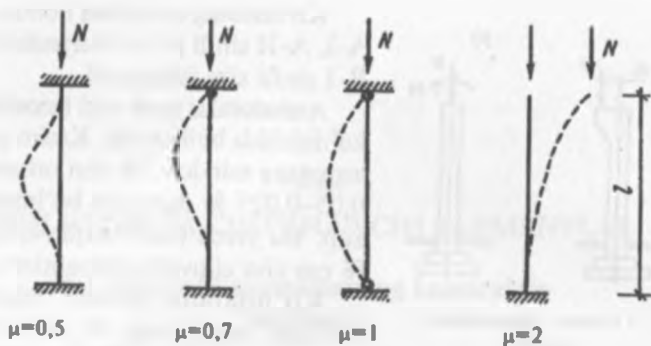
7.2-rasm. Ustunning hisobiy uzunligini aniqlash.
