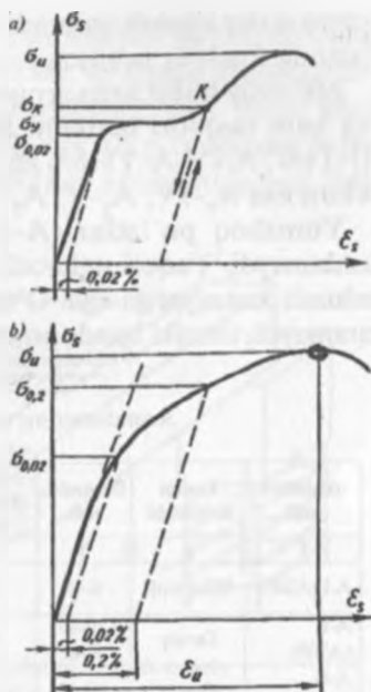
1.11-rasm. Armatura po'latining cho'zilishdagi xarakterli diagrammalari.
