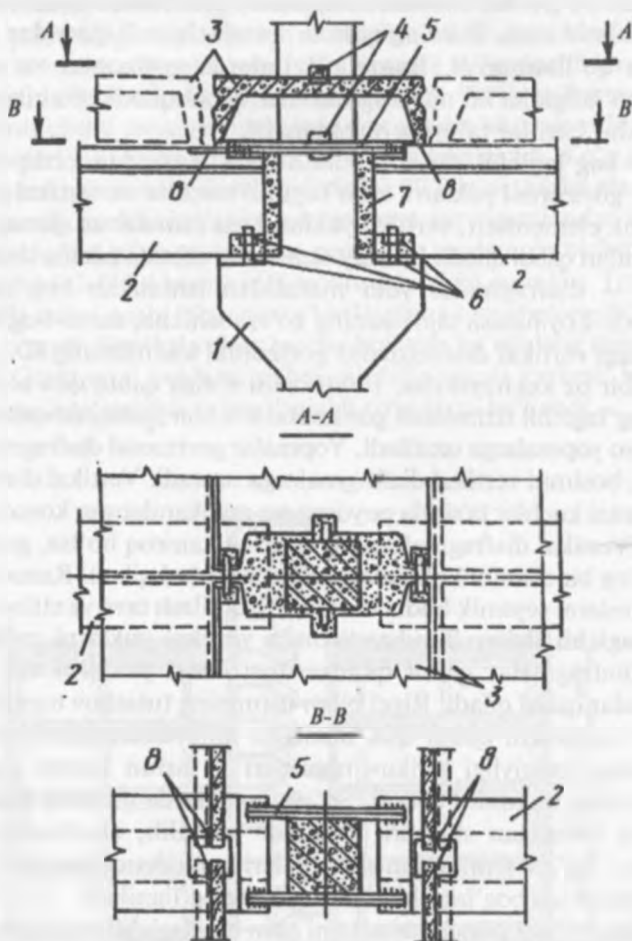
10.5-rasm. Ustun va rigellarning birikuv:
