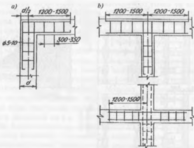
13.16-rasm Bo'ylama va ko'ndalang devorlarning tutashuv yertari: a — burchaklar; b — kesishuv yerlari.
