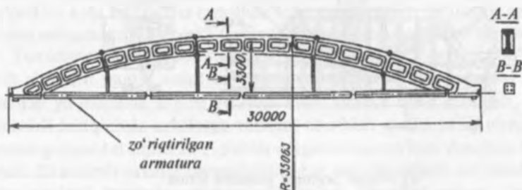
11.9-rasm. Oldindan zo'riqtirilgan tortqichli yig'ma temirbeton arka.
