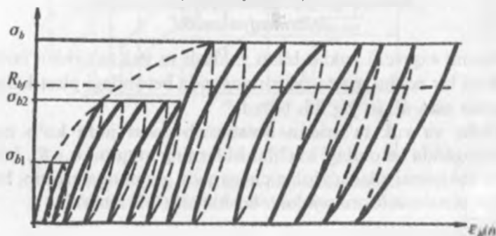
1.7-rasm. Yuklarning ko'p karrali yuklanishi va bo'shatishi ta'sirida betondagi deformatsiya.
