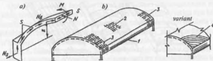
11.14-rasm. Ta'sir etuvchi kuchlar sxemasi (a) va uzun silindrik qobiqlarni armaturalash (b):
