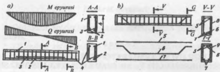
4.2-rasm. Bir oraliqli to'sinlarni armaturalash: a — payvand karkaslar; b — to'qima karkaslar.
