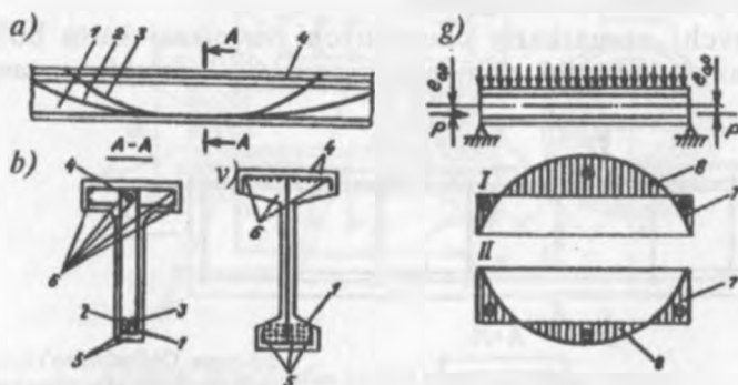
3.6-rasm. Oldindan zo'riqtirilgan egiluvchi elementlarni armaturalash: 1 - 4 - zo'riqtirilgan armatura; 5, 6 - zo'riqtirilmagan armatura; 7 - siquvchi zo'riqishdan hosil bo'lgan kuchlanishlar epyurasi; 8 - tashqi yuklar ta'sirida hosil bo'lgan kuchlanishlar epyurasi.
