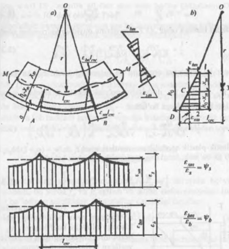
8.5-rasm. Egiluvchi elementning yoriqlari orasidagi deformasiyalar tarhi: a — egilishdagi deformasiya holati; b — deformasiya epyurasi.
