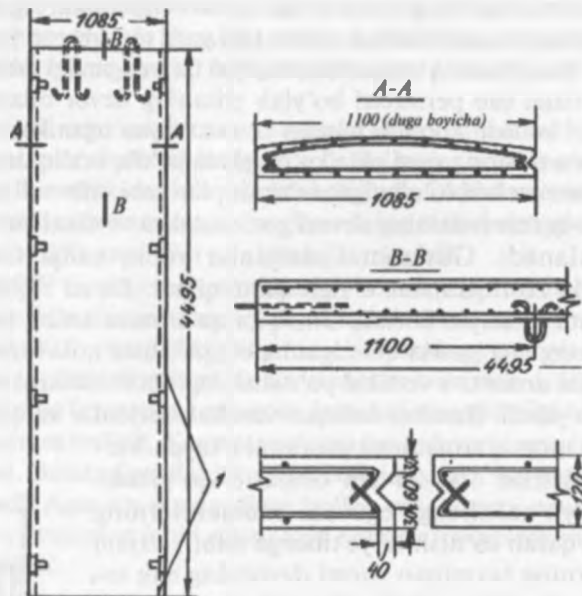
12.3-rasm. Yig'ma rezervuar devorining paneli.
