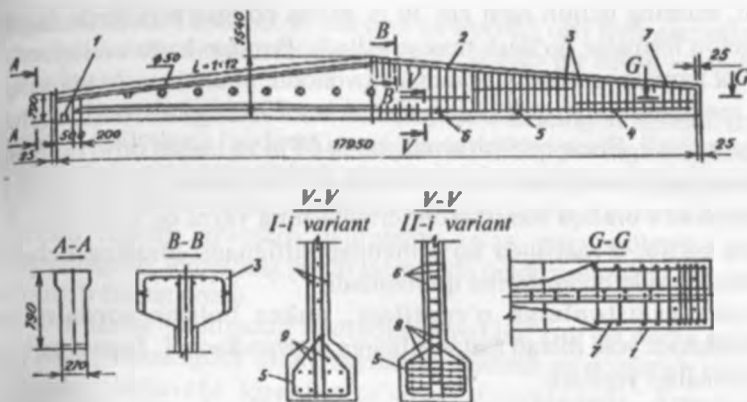
11.3-rasm. 18 m uzunlikdagi oldindan zo'riqtirilgan ikki nishabli to'sin:
