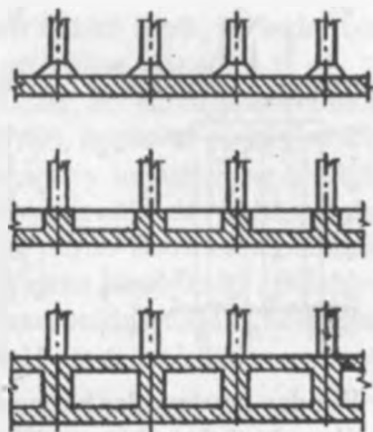
9.5-rasm. Yaxlit poydevorlar.
