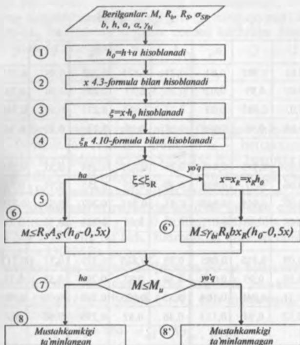
4.8-rasm. Egiluvchi elementlarni mustahkamlikka hisoblash.
