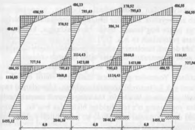
13.14-рasm. Ҳисобий моментлар эпюраси.
