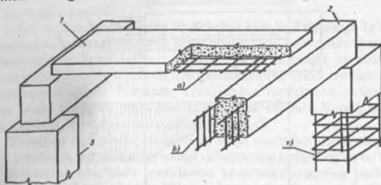
1.12-rasm. Temirbeton konstruksiyalarini armaturalash: 1 — plita; 2 — to'sin; a — sim — to'r; b — yassi karkas; v — hajmiy karkas.
