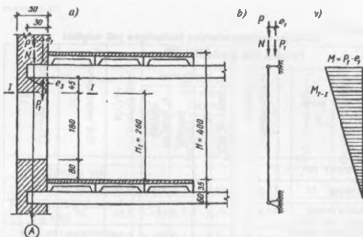
15.13-rasm. Devorni hisoblash: a – devor qirgimi; b – devorni hisoblash tarhi; v – vertikal yuklardan hosil bo'lgan momentlar pyurasi.
