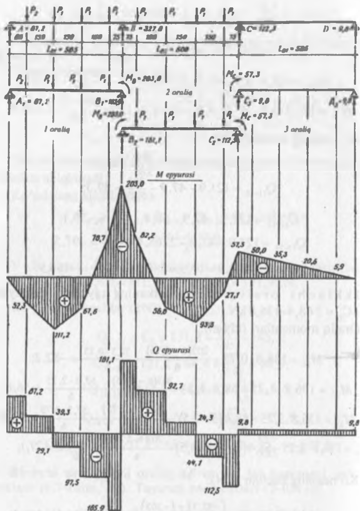
6.7-rasm. Birinchi va ikkinchi oraliq muvaqqat yuk bilan yuklanganda rigeldagi hisobiy zo'riqishlar epyurasini qurish.
