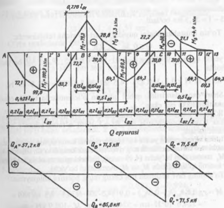
5.6-rasm. Ikkinchi darajali to'sindagi hisobiy zo'riqishlarning umumlashma epyuralari.
