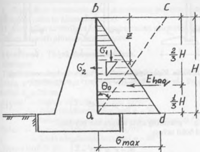
12.8-rasm. Qalin tirgak devorga grunt bosimining ta'siri.
