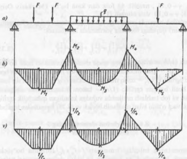
8.7-rasm. Uch oraliqli uzluksiz balkaning solqiligi: a — hisoblash tashqi; b — eguvchi momentlar epyurasi; v — egirliklar epyurasi.
