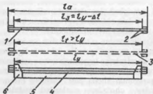
3.2-rasm. Armaturani elektrotermik usulda taranglash: 1 — sovuq sterjen; 2 — ankerlar; 3 — qizigan sterjen; 4 — sovugan (taranglangan) sterjen; 5 — qolip; 6 — tirkaklar.
