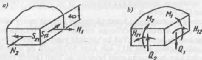
11.11-rasm. Qobiq kesimlarida vujudga keladigan zo'riqishlar.
