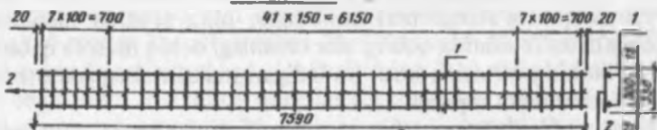
K-1 karkas
