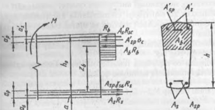
3.8-rasm. Oldindan zo'riqtirilgan elementning mustahkamlikka hisoblashda zo'riqishlar tarhi va kuchlanishlar cpyurasi.
