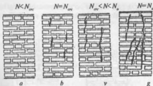
15.2-rasm Terimning siqilishdagi 4-boʻlqichi.
