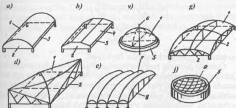
11.10-rasm. Yupqa devorli fazoviy temirbeton yopmalarning turlari:
