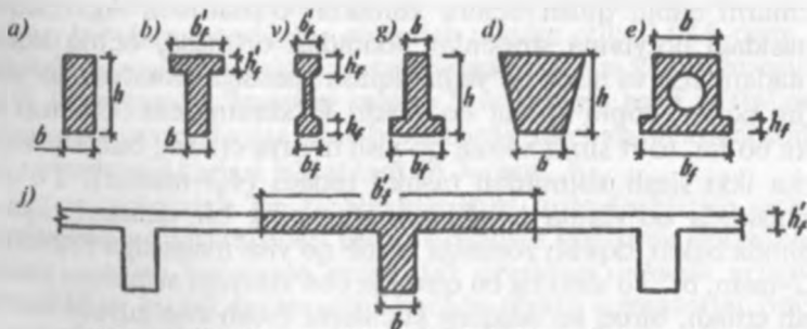
4.1-rasm. Temirbeton to'sinlarning ko'ndalang kesim yuzalari.
