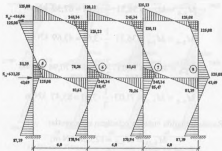
13.13-rasm. Tebranishlarning ikkinchi shakliga oid momentlar epyurasi.
