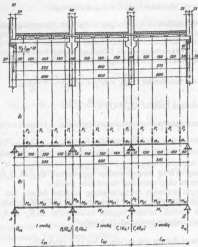
6.4-rasm. Rigelni hisoblashga doir:
