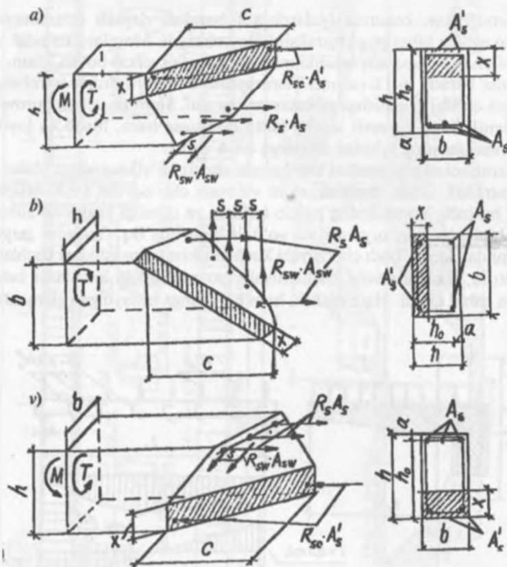
6.13-rasm. Buralib egiluvchi to'sinning kesimdagi zo'riqlari.
