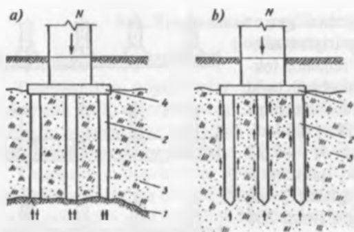
9.6-rasm. Qoziq poydevor tashi: a — ustun - qoziqlar; b — osma qoziqlar; 1 — qattiq grunt; 2 — qoziq; 3 — yumshoq grunt; 4 — rostverk.
