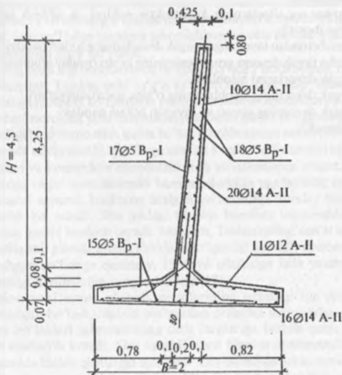
12.11-rasm. Tirkak devor konstruksiyasini armaturalash.
