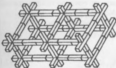
13.3-rasm. Sinchlarni alohida elementlarga ajratish tarhlari.
