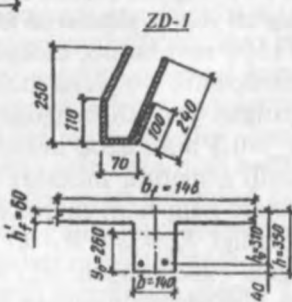
6.3-rasm. Yopma plita.
