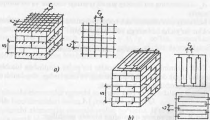
15.9-rasm. Ko'ndalang armaturalangan terim.
