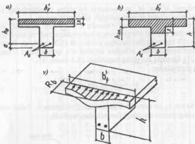
5.3-rasm. Neytral o'q joylashuvining mumkin bo'lgan hollari.
