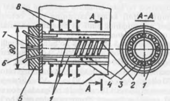
3.3-rasm. 18 ta simdan tashkil topgan armatura tutami:
