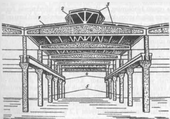
10.2-rasm. Yig'ma temirbeton elementlardan tiklangan bir qavatli sinchli sanoat binosi:
