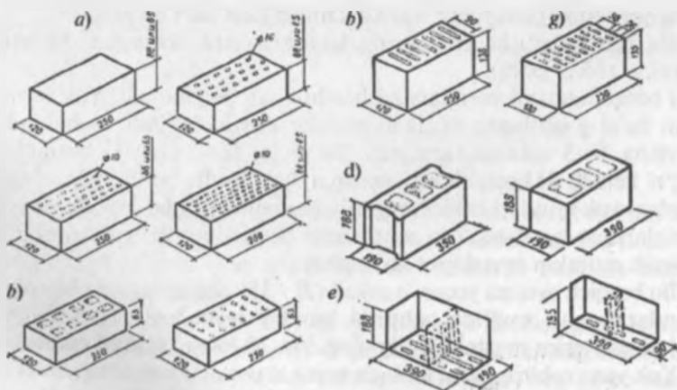
15.1-rasm. Tosh va g'ishtlarning turlari:
