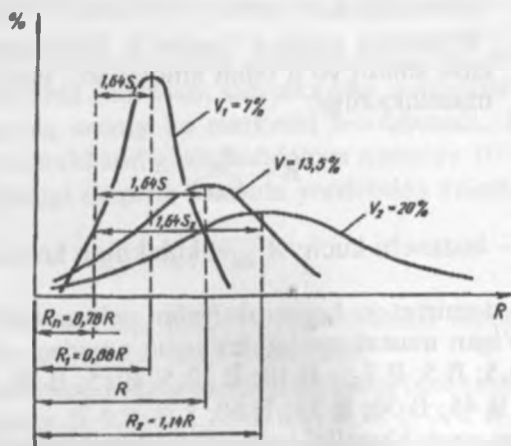
1.3-rasm. O'zgaruvchan koeffitsiyentning turli qiymatlari va betonning kerakli normativ qarshiligi R_n ni olish imkonini beradigan, beton o'rtacha mustahkamligi R_1 ga mos bo'lgan normal taqsimlash egri chiziqlari.
