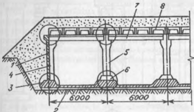
12.4-rasm. Yig'ma to'rtburchak shaklli rezervuarning konstruksiyasi:
