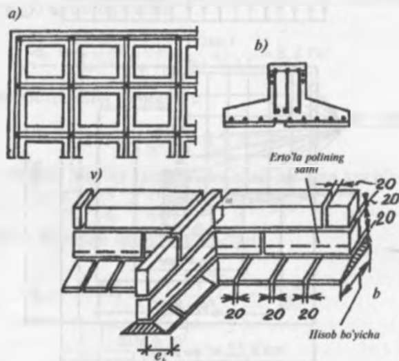
9.4-rasm. Tasmasimon poydevorlar:
