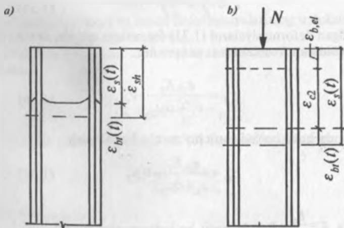
1.14-rasm. Beton cho'kishi va tob tashlashining temirbetonga ta'siri: a — cho'kishda; b — tob tashlashda.
