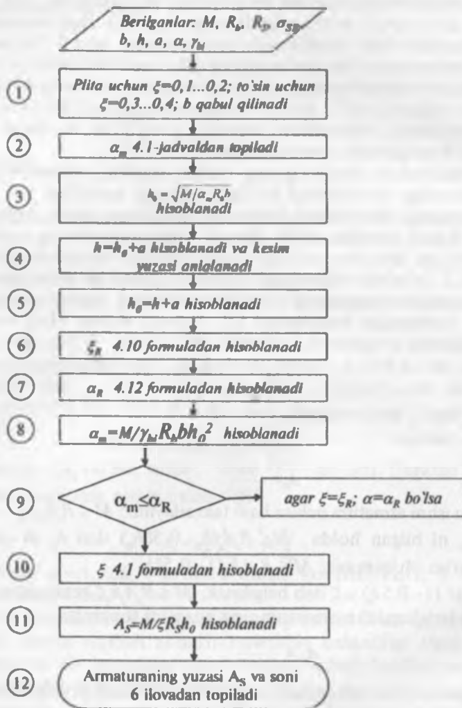
4.7-rasm. Yakká armaturali egiluvchi elementlarda armatura yuzasini topish.
