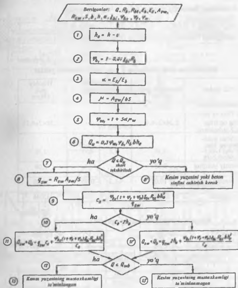
5.5-rasm. Egiluvchi elementni qiya kesim bo'yicha yig'iq kuch ta'sirida mustahkamlikka hisoblash (bukma armatura bo'lmagan hol uchun).
