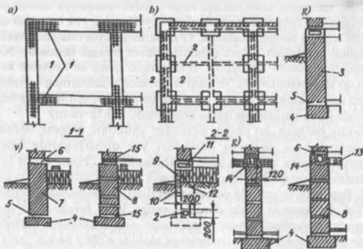
13.19-rasm. Poydevor va erto'la detallari.
