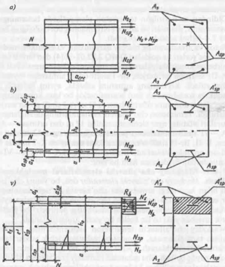
7.8-rasm. Cho'ziluvchi elementlarda kuchlarning joylashishi tarhi:
