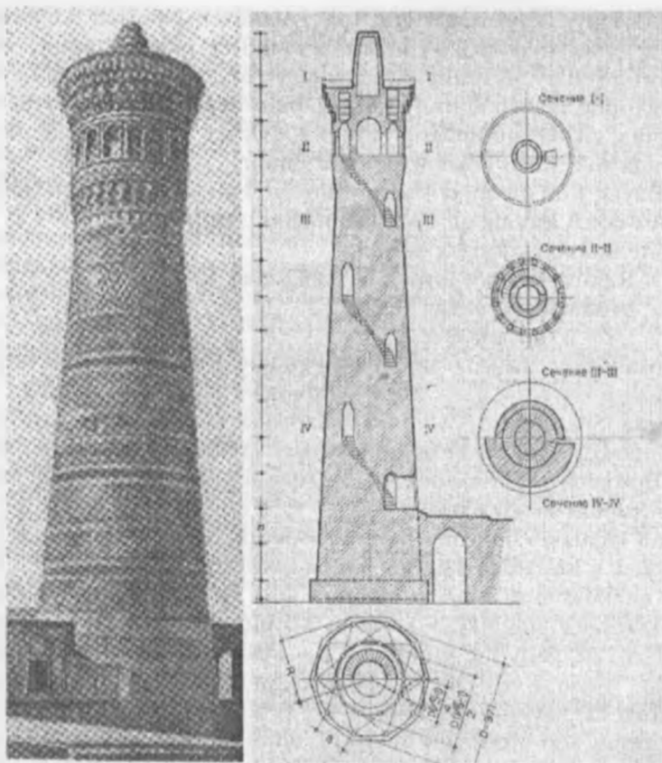
13.20-rasm. Minorai Kalon obidasining umumiy ko'rinishi va uni loyihalashga doir.
