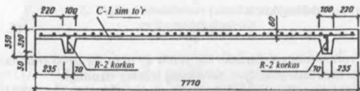
K-1 karkas
