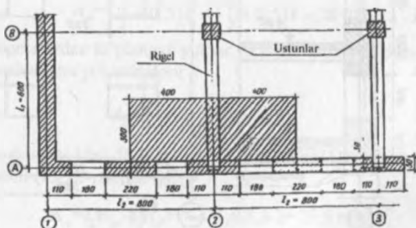
15.12-rasm. Devorning yuk maydonchasini aniqlashga doir.
