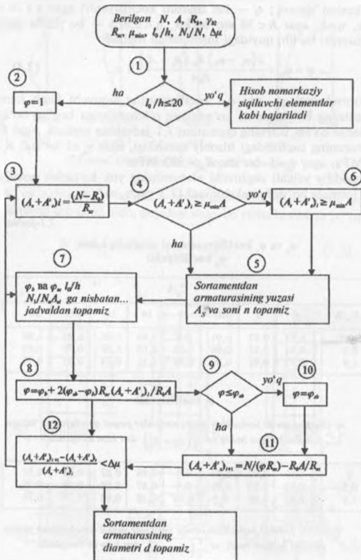
7.4-rasm. Tasodifiy yelkali kesim yuzasi to'g'ri to'rtburchak shaklida bo'lgan siqiluvchi elementlardagi armatura yuzasini aniqlash.
