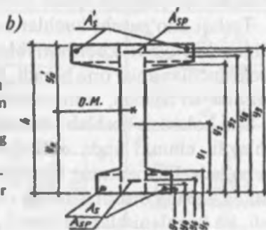
3.7-rasm. Oldindan zo'riqtirilgan element kesimida hosil bo'ladigan kuchlanishlarni aniqlashga doir: a — siqilishdagi kuchlanishlarning joylanishi; b — keltirilgan yuzaning geometrik xarakteristikasini topishga doir sxema.
