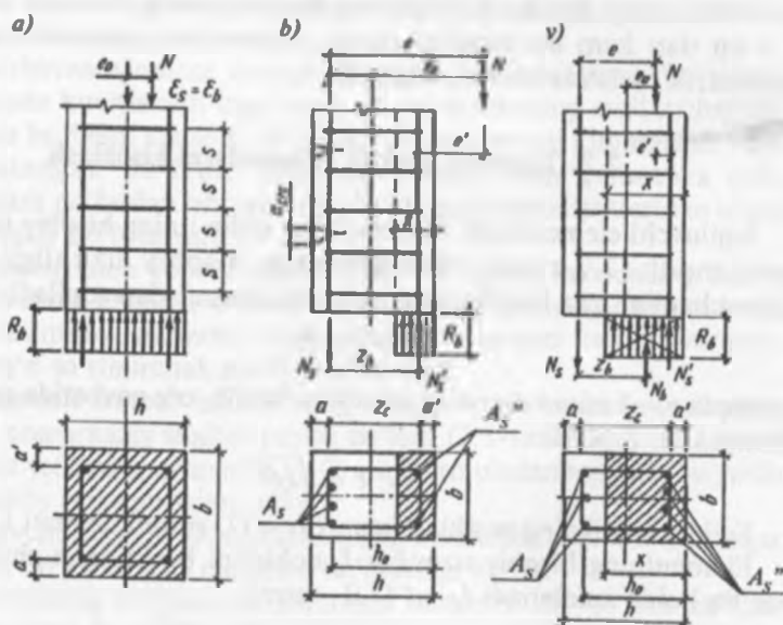
7.3-rasm. Siqiluvchi elementlarning hisoblash turhi:
