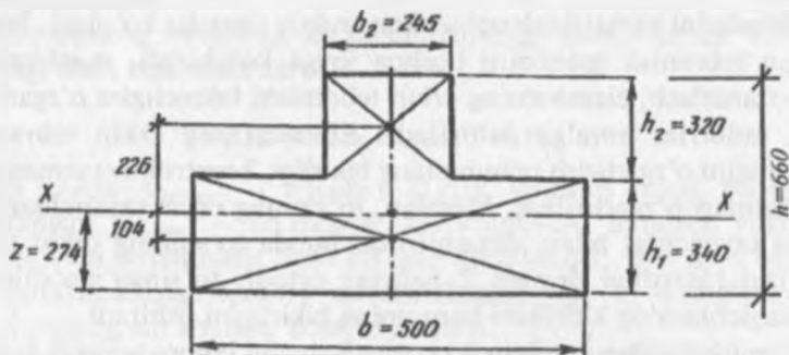
13.6-rasm. Rigelning ko'ndalang kesimi.
