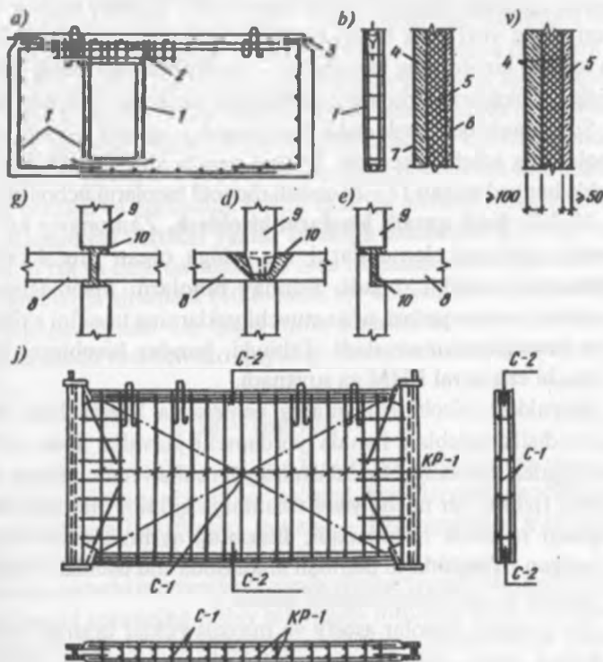
10.7-rasm. Panel binolar konstruksiyalari:
