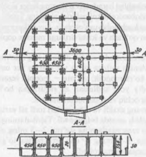
12.1-rasm. To'sinsiz yassi yopmali doiraviy rezervuar.
