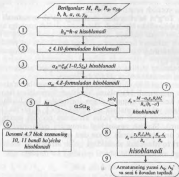
4.10-rasm. Qo'sh armaturali egiluvchi elementlarning armatura yuzasi A_s va A_s' topish.
