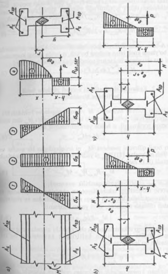
8.1- rasm. Elementlarning yorilishga bardoshligini hisoblashda normal kesimda kuchlarning joylashishi: a — egiluvchi element; b — nomarkaziy siqilish; v — nomarkaziy cho'zilish.
