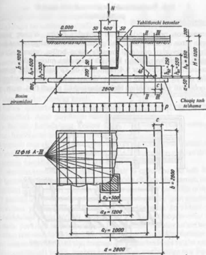
9.3-rasm. Ustun ostiga qo'yiladigan temirbeton poydevor (poyustun).
