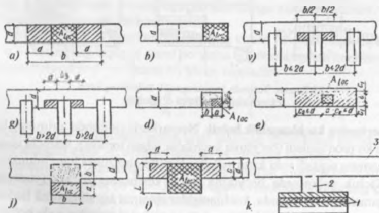
15.6-rasm. Mahalliy siqilishda kesimlarning hisobiy yuzalarini aniqlash.
