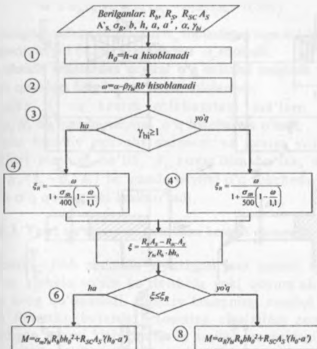
4.11-rasm. Qo'sh armaturali egiluvchi elementlarni mustahkamlikka hisoblash.
