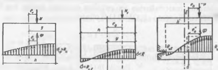
15.7-rasm. Terimda kuchlanganlik holatining kuch ekssentrisitetiga ko'ra o'zgarishi.
