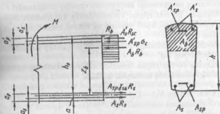
3.8-rasm. Oldindan zo'riqtirilgan elementning mustahkamlikka hisoblashda zo'riqishlar tarhi va kuchlanishlar payurasi.
