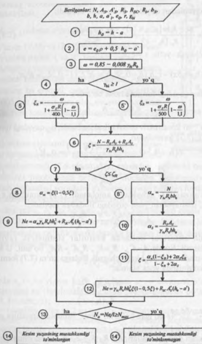
7.5-rasm. Nomsimmetrik armaturalangan nomarkaziy siqiluvchi elementlarni mustahkamlikka hisoblash.
