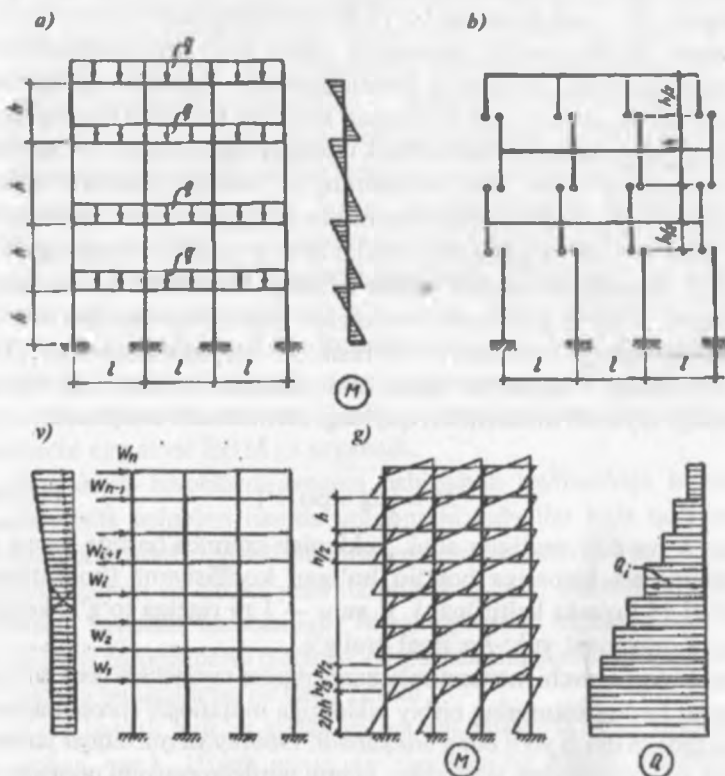
10.8-rasm. Ko'p qavatli ramalarni vertikal (a, b) va gorizontaal (v, g) yuklar ta'siriga hisoblashga doir: Q i — i-qavatdagi ko'ndalang kuch.
