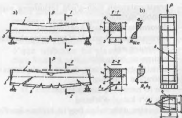
1.1-rasm. Elementlarning kuch ta'sirida ishlashi:
