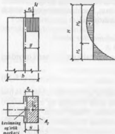
15.8-rasm. Nomarkaziy siqilgan terimning hisobiy tarhi.
