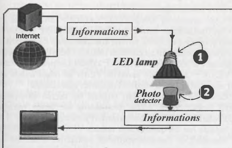
3.10-rasm. Li-Fi ishlash texnologiyasi.
