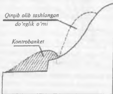
6.4-rasm. Qyaliklarni yassilab va kontrobanket qurib ularning mustahkamligini oshirish chizmasi.
