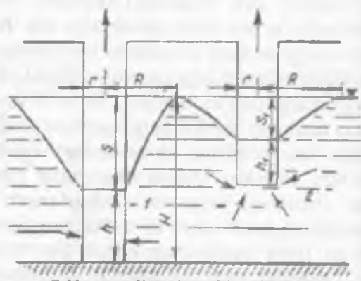
7.16-rasm. Suv yiguvchi quduqlar: 1-tugallangan ko'rinish; 2-tugallanmagan ko'rinish.
