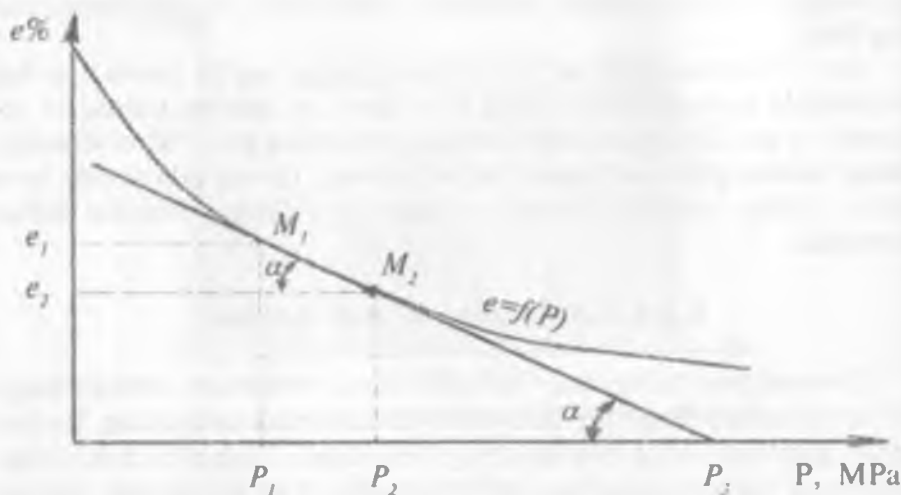
8.3-rasm. Tashqi kuchning g'ovaklilik ko'rsatuvchi grafik.
