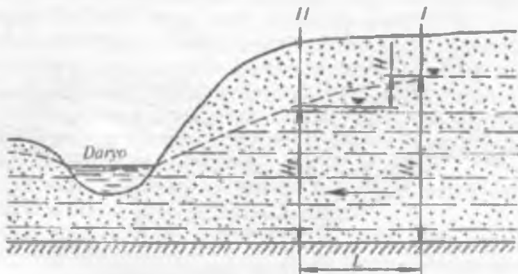
7.11-rasm. Grunt suvlarining sizish chizmasi.
