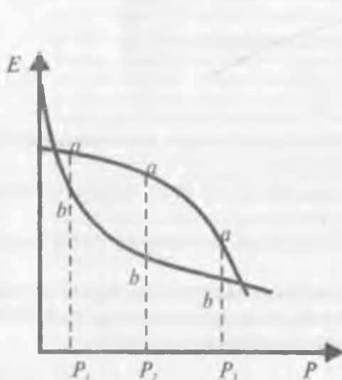
6.12-rasm. Suvga to'la to'yingan va tabiiy namlikdagi lyossimon jinslarning zichlanish grafiqi.
