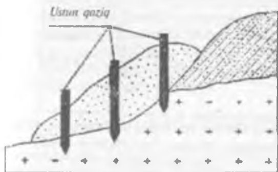
6.3-rasm. Surilishdagi qiyalikni ustun qoziqlar yordamida mustahkamlash. (O.Mavlonov va Zohidov rasmi).
