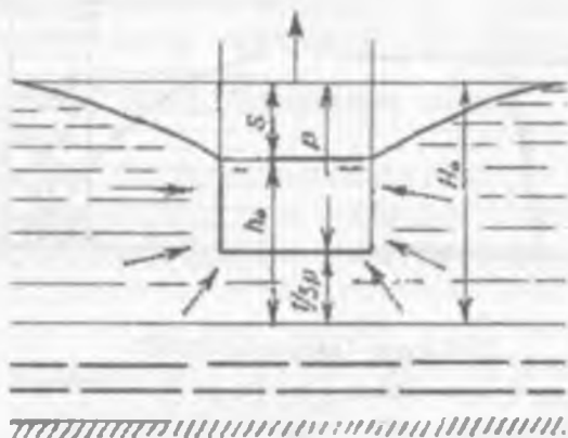
7.17-rasm. Tugallanmagan quduqning ko'rinish chizmasi.
