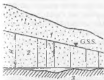
7.4-rasm. Grunt suvi.
