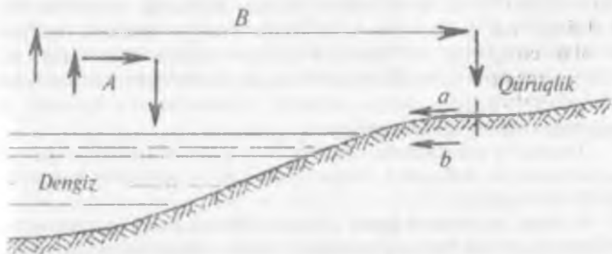
7.1-rasm. Suvning tabiatda aylanishi. A- kichik; B-katta.
