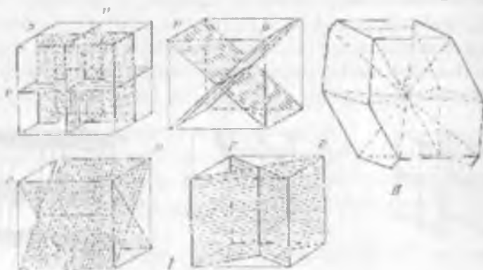
2.3-rasm. Simmetriya teksliklari va markazi
