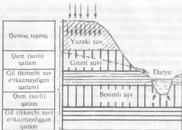
7.2-rasm. Yer osti suvlarining joylanishiga qarab klassifikatsiyasi.
