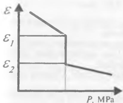
6.14-rasm. Lyossimon tog' jinsining zichlanishini ifodalovchi egri chiziq.
