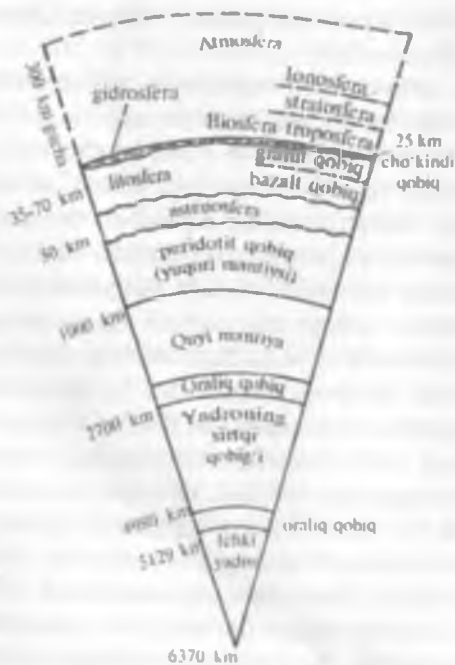
1.1-rasm. Yerning tuzilishi
