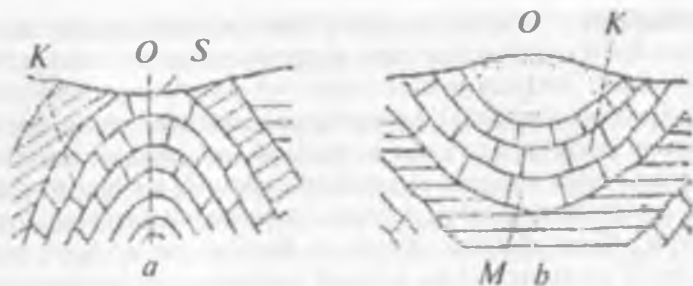
5.1-rasm. Bukilmalar va ularning elementlari: a -antiklinal; b -sinklinap; k -qanoti; o -bukilmalar o'qi; s -egar, M -mulda.
