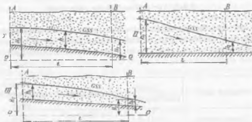
7.12-rasm. Grunt suvlari oqimining sarfini hisoblash chizmasi: I va II suv o'tkazmaydigan qatlamning gorizontaal vaziyati; III qiya vaziyat.
