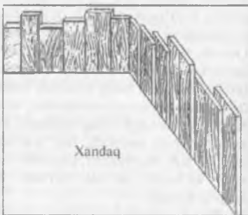
6.10-rasm. Xandaq atrofiga o'rnatilgan shpuntli devorlar.
