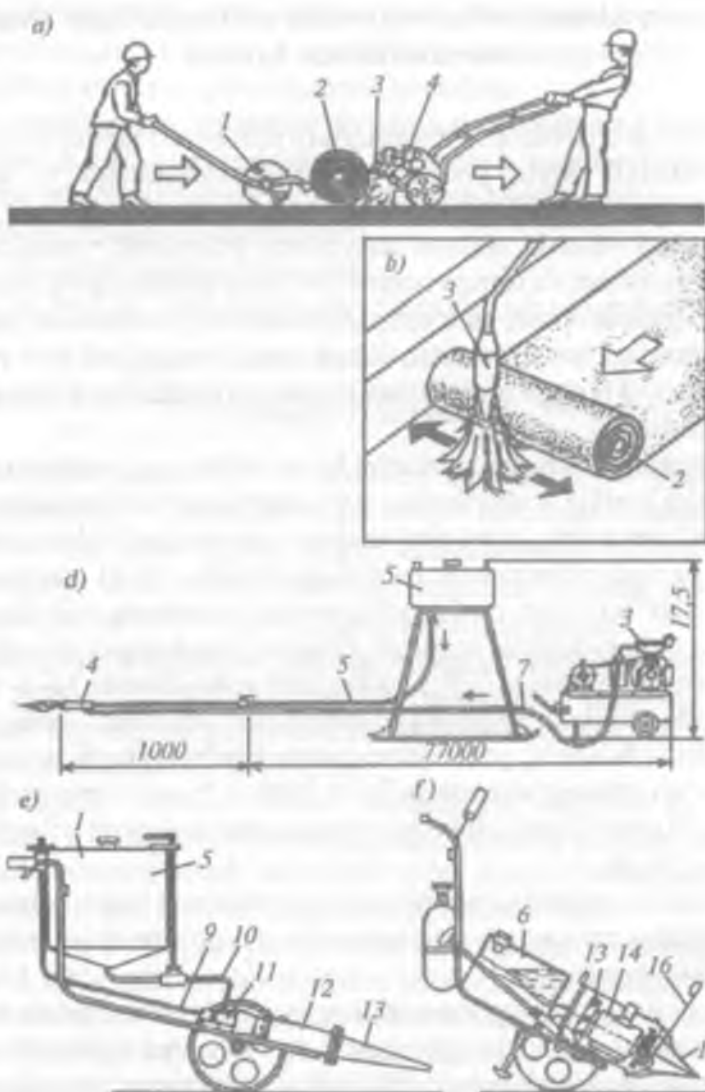
32- rasm. Eriydigan qatlamli ruberoidni qizdirib yelimlash usuli: a—ko'p forsunkali gazli qizdirgich; b—bir forsunkali gazli qizdirgich; d, e, f—suyuq yoqilg'ida ishlaydigan qurilmalar. 1—katok; 2—ruberoid; 3—gazli qizdirgichlar; 4—forsunka; 5, 7—uayt-spirit va havo uzatish uchun shlanglar; 6—bosimsiz bak; 8—kompressor; 9, 10—havo va uayt-spirit uzatish uchun quvurlar; 11—forsunka; 12—yonish kamerasi; 13—kengaygan quvur; 14—parrak; 15—elektryuritkich; 16—yondirgich.
