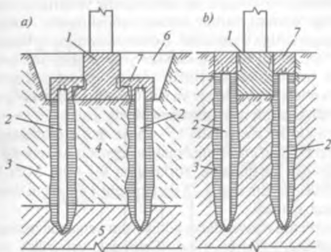
15- rasm. Spirpalsimon snaryadlar bilan quduqlarni botirish sxemasi:
