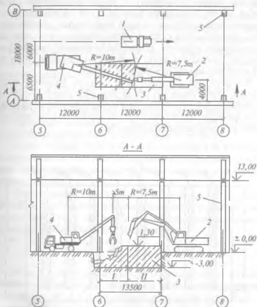
1- rasm. Bino ichida poydevorni bo'laklab olish texnologik sxemasi:
