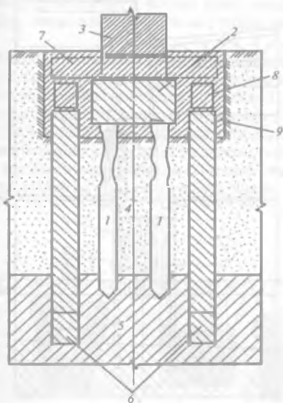
19- rasm. Qoziqli poydevorni qo'shimcha qoziqlar bilan kuchaytirish: 1—eski qoziqlar; 2—rostverk; 3—devor; 4—zamin gruti; 5—mustahkam gruti; 6—qo'shimcha qoziqlar; 7—ko'ndalang to'sin; 8—bo'ylama to'sin; 9—yangi quyilgan beton.
