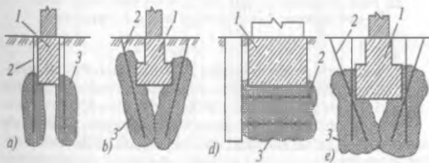
21- rasm. Inyektorlar yordamida poydevorlarni kuchaytirish sxemalari: a—vertikal; b—qiya; d—gorizontal; e—kombinatsiyalashgan. 1—kuchaytiriladigan poydevor; 2—inyektorlar; 3—smola.
