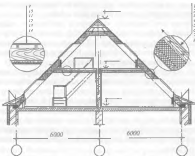
54- rasm. Ikki yarusli mansarda qavatini barpo etish sxemasi: 1—tomqoplama va suvdan himoyalash qatlami; 2—yaxlit reykalari; 3—kontrreyka; 4—reykalar panjarasi; 5—shamoldan himoyalash; 6—mineral paxtali isitkich; 7, 13—bug'dan himoyalash qatlami; 8, 14—koshin qoplama; 9—pol taxtasi; 10—pol osti to'sini(laga); 11—orayopma to'sini; 12—mineral paxtali tovushdan himoyalash qatlami.
