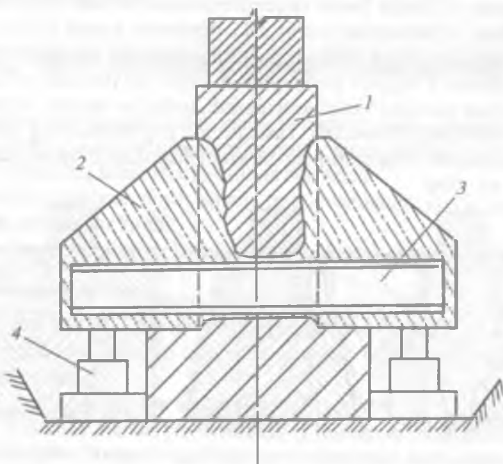
7- rasm. Gidrodomkratlar yordamida poydevorni qisish: 1—eski mavjud poydevor; 2—yangi quyilgan beton; 3—ko'ndalang to'sin; 4—gidrodomkrat.
