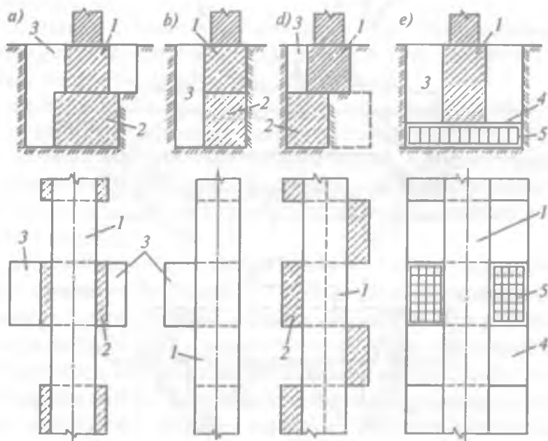
10- rasm. Sayoz joylashgan poydevorlarni kuchaytirish sxemalari: a—bir chiziq bo'ylab alohida bloklar bilan; b—yaxlit devorli bloklar bilan; d—shaxmat tartibida joylashgan bloklar bilan; e—yaxlit temirbeton plita bilan. 1—kuchaytirilayotgan poydevor; 2—kuchaytirish bloki; 3—poydevor yoni chuquri; 4—kuchaytirish plitasi; 5—kuchaytirish plitasini armaturalash.
