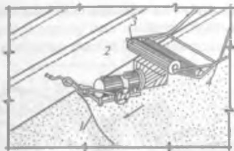
33- rasm. Suyuq yoqilg'ida ishlaydigan qurilma yordamida ruberoidlarni yelimlash:
