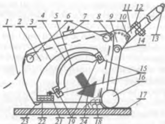
44, b- rasm. Eriyidigan qatlamli ruberoidni infraqizil nuri usulida qizdirib yelimlovchi yangi qurilma («Nur-5U-01») ning sxemasi.
