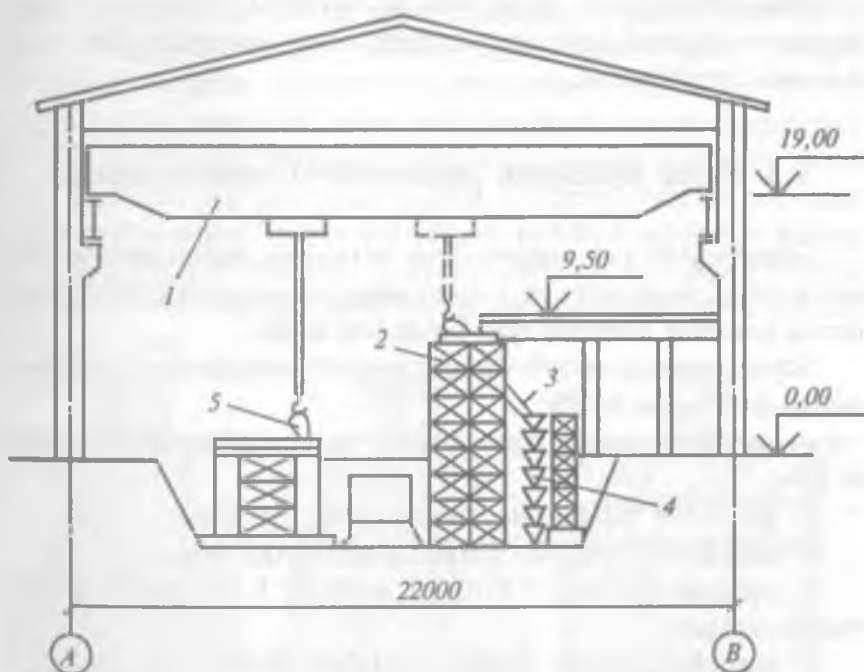
5- rasm. Bino oralig'ida ishlaydigan ko'priqli kranlardan foydalanib poydevorlarni qayta qurish texnologik sxemasi:
