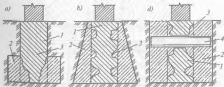
6- rasm. Temir-beton belbog' yordamida poydevorlarni kuchaytirish: a—poydevor tubini kengaytirish; b—poydevorni balandligi bo'yicha kengaytirish; d—poydevorni ko'ndalang to'sin bilan kuchaytirish; 1—kuchaytirilayotgan poydevor; 2—yangi quyilgan beton; 3—ishlov berilgan yuza; 4—ko'ndalang to'sin.
