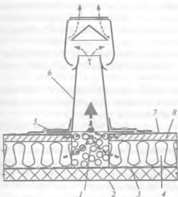
53- rasm. Shamollatgich quvurcha(deflektor)ni o'rnatish sxemasi: 1—almashtiriladigan zichlagich; 2—tom yopma plitasi; 3—bug'dan himoyalash qatlami; 4—issiqdan himoyalash(isitkich) qatlami; 5—tomqoplama ashyosining qo'shimcha qatlami; 6—shamollatish quvurchasi; 7—shamollatiladigan ikki qatlamli tomqoplama(ruberoid); 8—tekislovchi suvoq qatlami.
