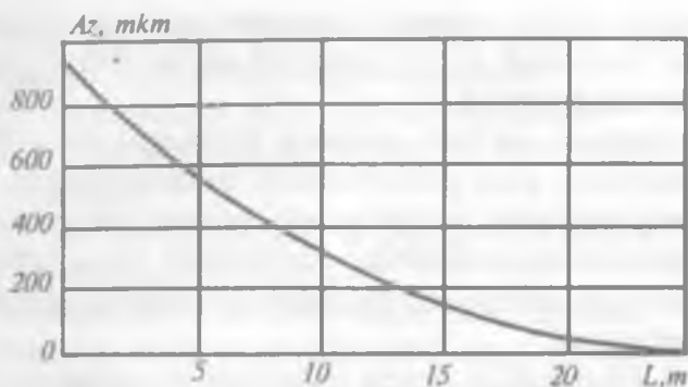
4- rasm. Binoga ta'sir qiluvchi tebranish amplitudasi qiymatini tebranish manbai uzoqligiga bog'liqligi.
