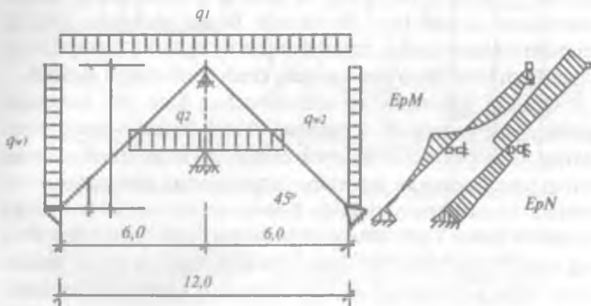
57- rasm. Fermaning statik ishlashi.
