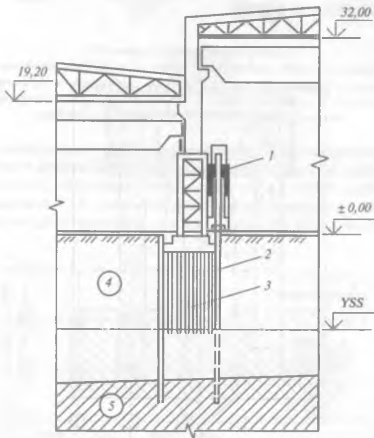
20- rasm. Qoziqni kiritish uchun qurilma: 1—UKS-22 dastgohi; 2—po'lat qobiqda botiriladigan qoziq; 3—eski qoziq; 4—bo'sh grunt; 5—mustahkam grunt. YSS — yer osti suvlar sathi
