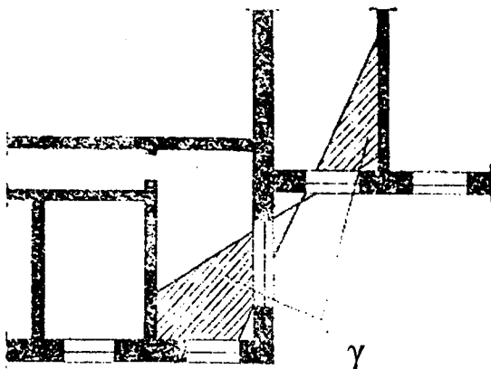
1.18-rasm. Yonma-yon kvartiralarda insolatsiyaning buzilishi ( \gamma – diskomfort zonalar)
