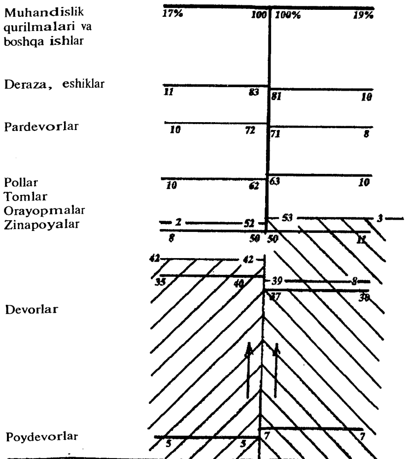
1.20-rasm. Bino konstruktiv unsurlarining solishtirma og'irligi. Almashtirilmaydigan konstruksiyalar shtrix bilan ko'rsatilgan.
