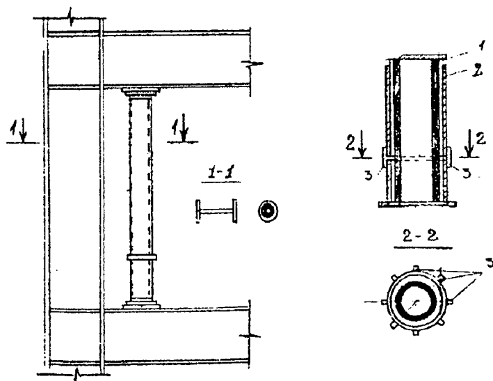
9.8-rasm. Oldindan zo'riqtirilgan tirkak bilan kuchaytirish.
