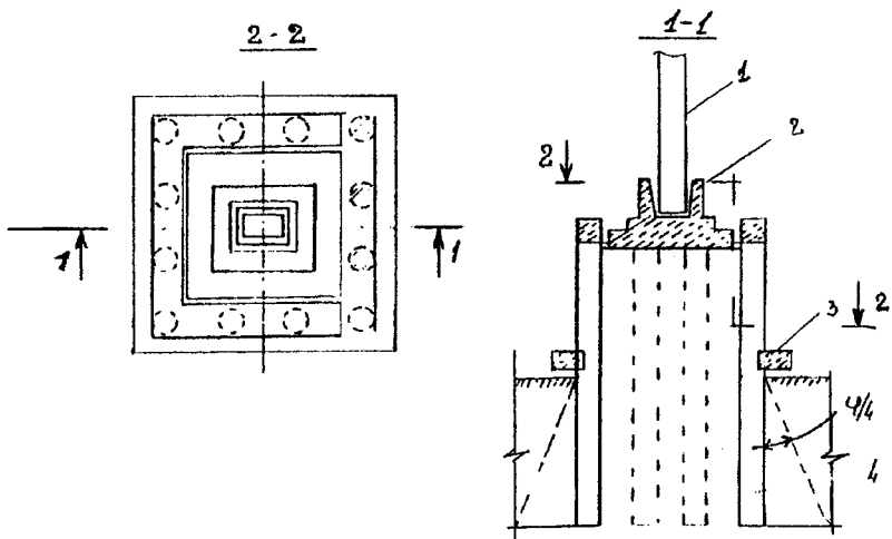
8.1-rasm. Zaminlarni to'siqli svaylar bilan kuchaytirish.
