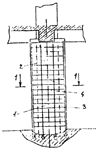
9.5-rasm. Ustunni temirbeton xalqa bilan kuchaytirish.
