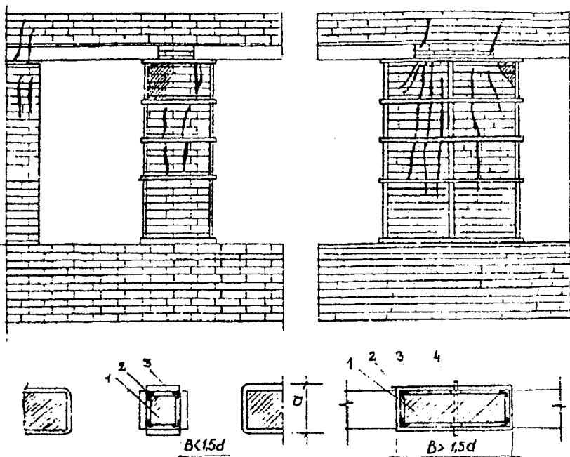
9.4-rasm. Oraliqni po'lat xalqa bilan kuchaytirish:
