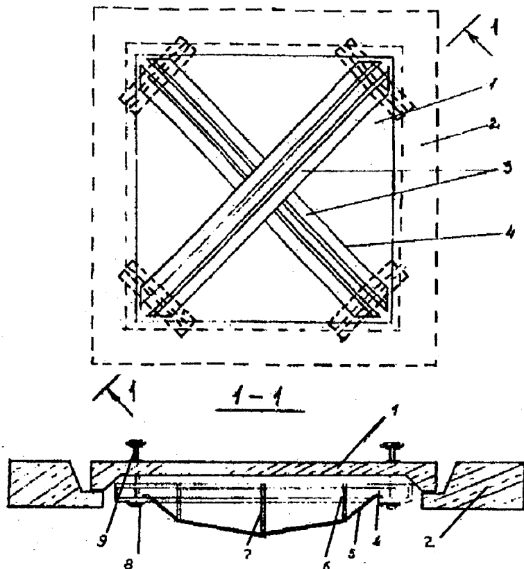
9.7-rasm. Kontur bo'yicha tayanuvchi yig'ma plitani fazoviy shprengel yordamida kuchaytirish.
