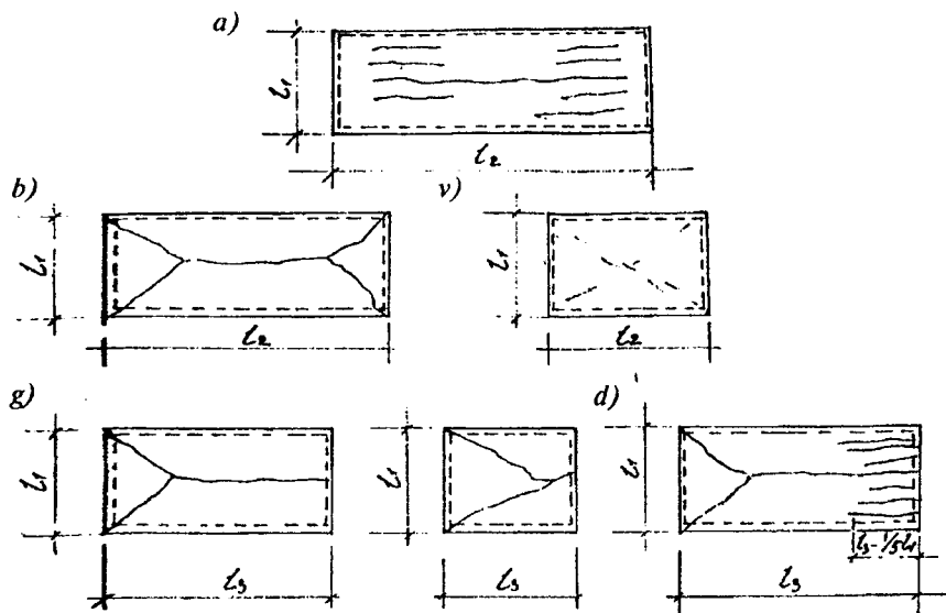
6. 1-rasm. Plitaning pastki yuzasidagi tavsifli darzlar:
