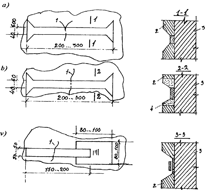
5.2-rasm. Nishonlarning turlari.
