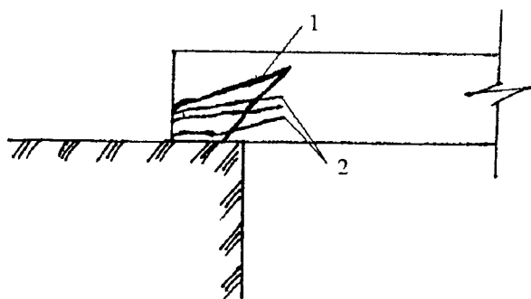
6.2-rasm. Oldindan zo'riqtirilgan elementning tayanch qismidagi darzlar.
