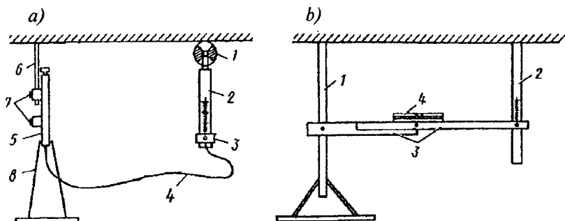
3.7-rasm. Solqilarni o'lchash uchun asboblar.
