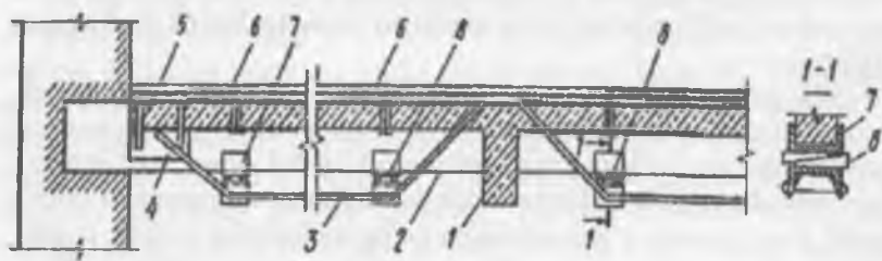
10.4-rasm. Yaxlit quyma temirbeton orayopmani kuchaytirilishi.
