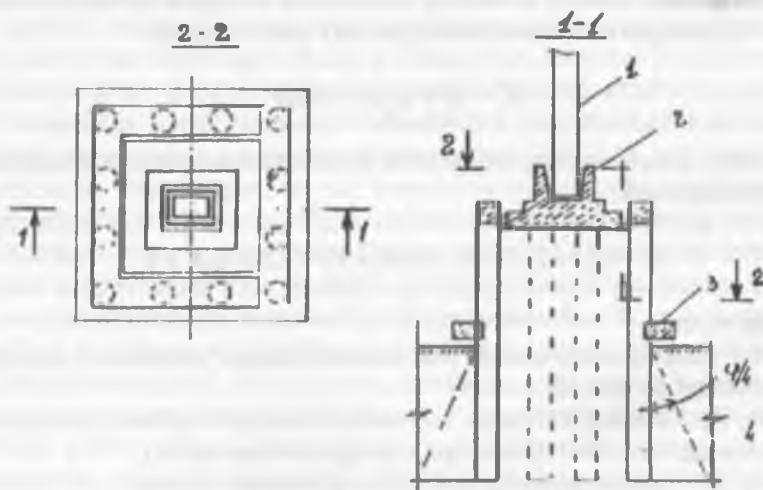
8.1-rasm. Zaminlarni to'siqli svaylar bilan kuchaytirish.
