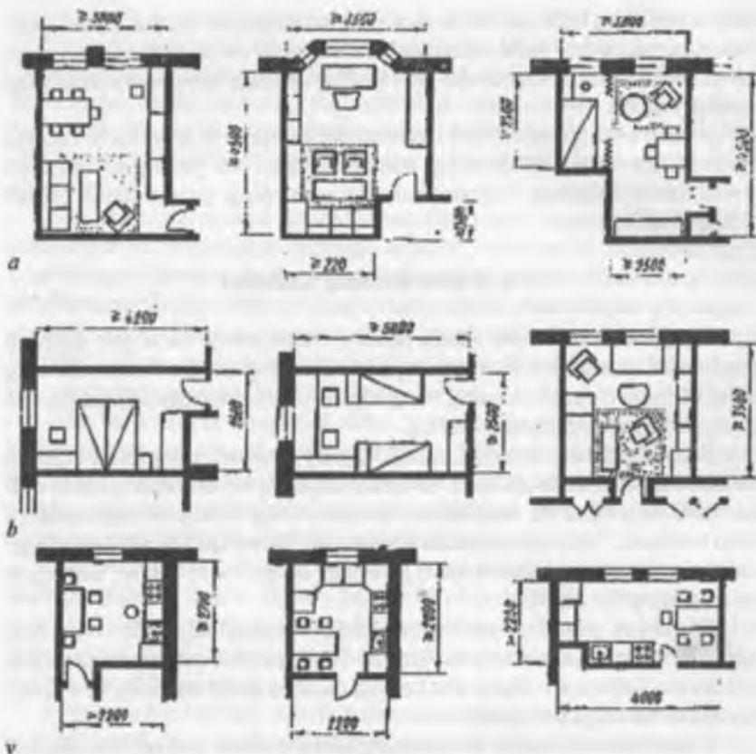
1.19-rasm. Kvartiraning rejayiy unsurlari.
