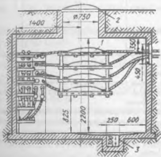
13-rasm. Kabelli quduqning qirgimi.
