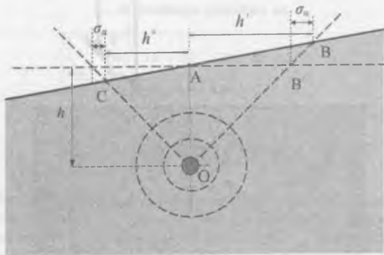
53-rasm. \sigma_v xatosining grafik ko'rinishi.
