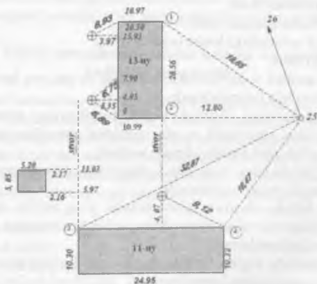
17-rasm. Turli usullarda gorizonta planga olishning abrisi.
