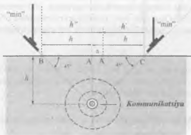
50-rasm. Kommunikatsiya joylashish chuqurligini aniqlash sxemasi
