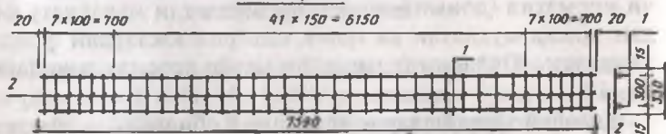
К-1 қарқас
