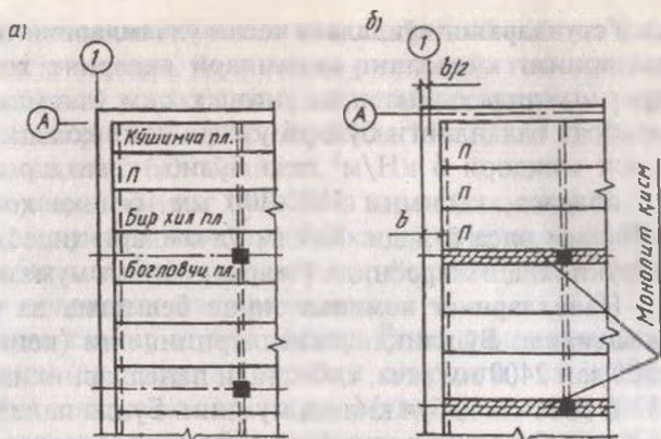
6.1-расм. Ёзма панелларни жойлаштириш намуналари.
