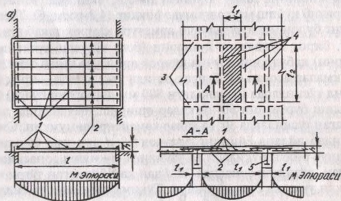
4.4-расм. Тўсинсимон яхлит плиталарни арматуралаш:
