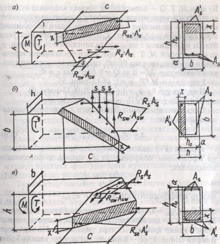
6.13-расм. Буралиб эгилювчи тўсиннинг кесимдаги зуриқишлари.
