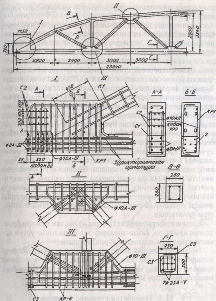
11.7-рasm. Сегмент панжарали ферма.
