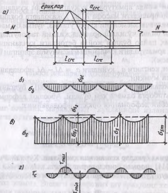
8.3-расм. \psi , \eta ни аниқлашга доир тарх:
