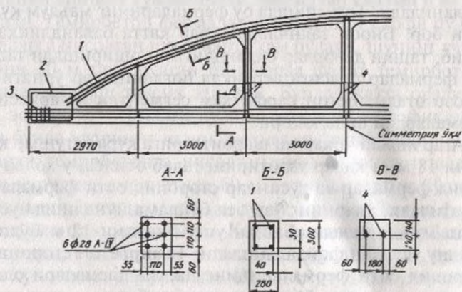
11.6-расм. Пастки тасмаси ва устунилари олдиндан зўриқтирилган ҳовонсиз фермани арматуралаш:
