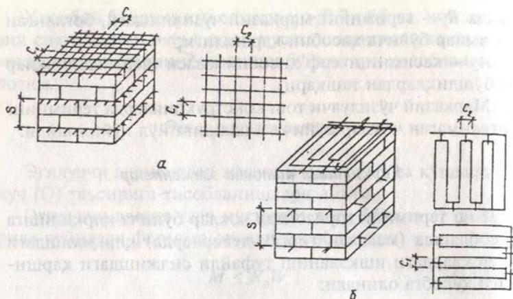
15.9-расм. Кўндаланг арматураланган терим.
