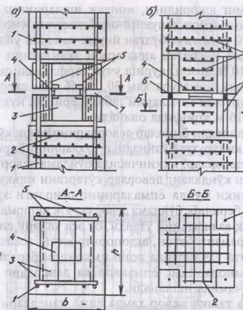
10.6-расм. Устуннинг бикир чоклари:
