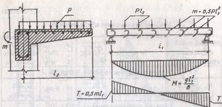
6.12-расм. Тусиннинг бурилиб эгилишини ҳисоблашга доир.
