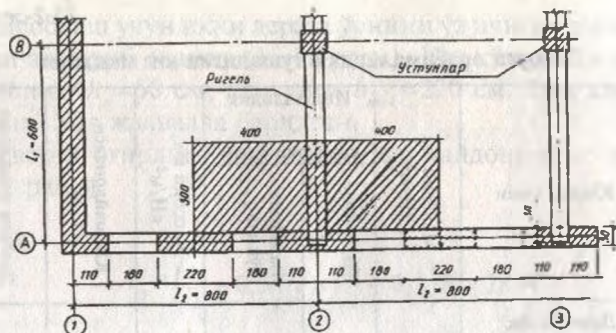
15.12-рasm. Деворнинг юк майдончасини аниқлашга доир.
