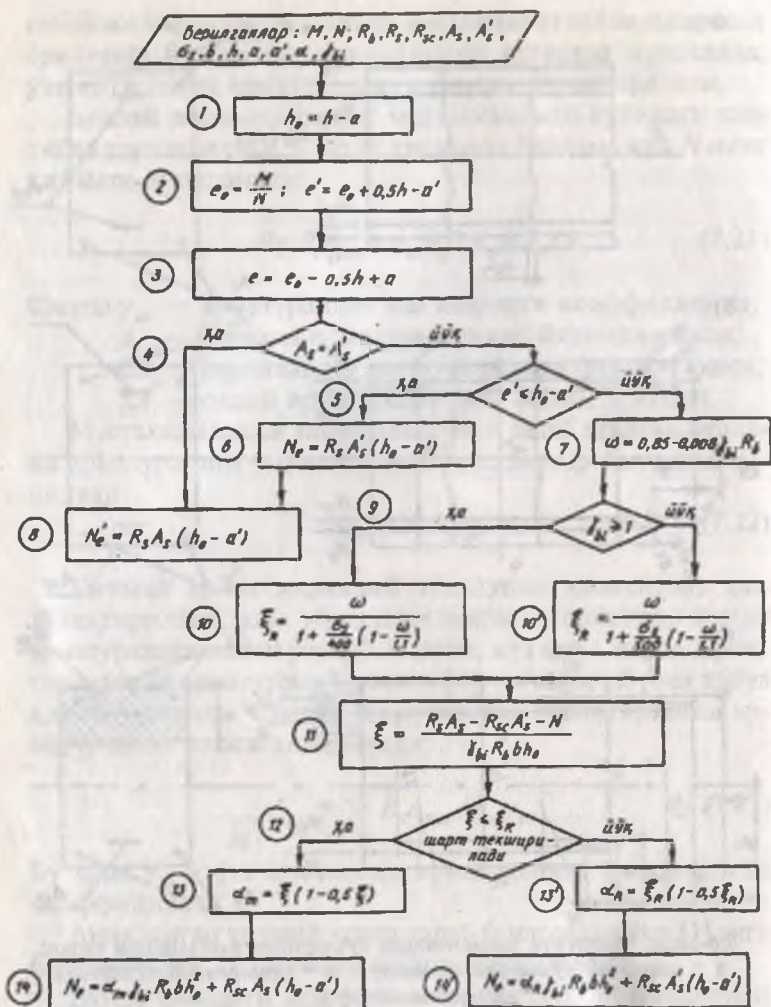
7.9-расм. Номарказий чузилувчи элементлар кесим юзасини мустаҳкамликка ҳисоблаш.
