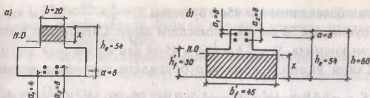
6.10-расм. Ригелнинг характерли ҳисобий кесимлари: а — оралиқда; б — таянчда.
