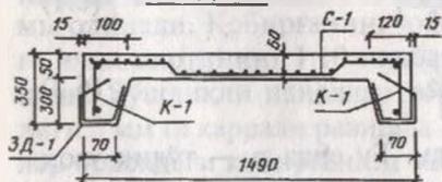
2-2 қирқим
