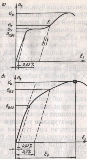
1.11-расм. Арматура пўлатининг характерли диаграммалари.
