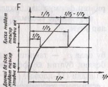
8.6-расм. Олдиндан зуриқтирилган элементларнинг тўлиқ эгрилигини ҳисоблашга доир.
