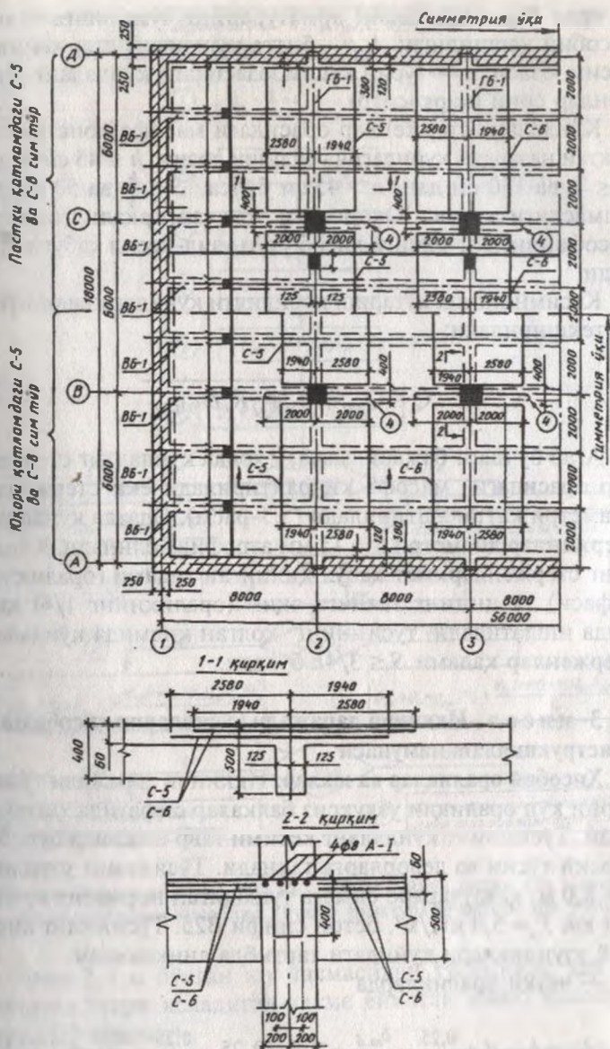
5.4-рasm. Иккинчи даражали түсиннинг таянч қисмини арматуралаш.
