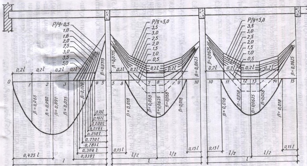
5.1-расм. Тенг оралиқли узлуксиз тўсинлар учун ҳисобий моментлар эпюралари.
