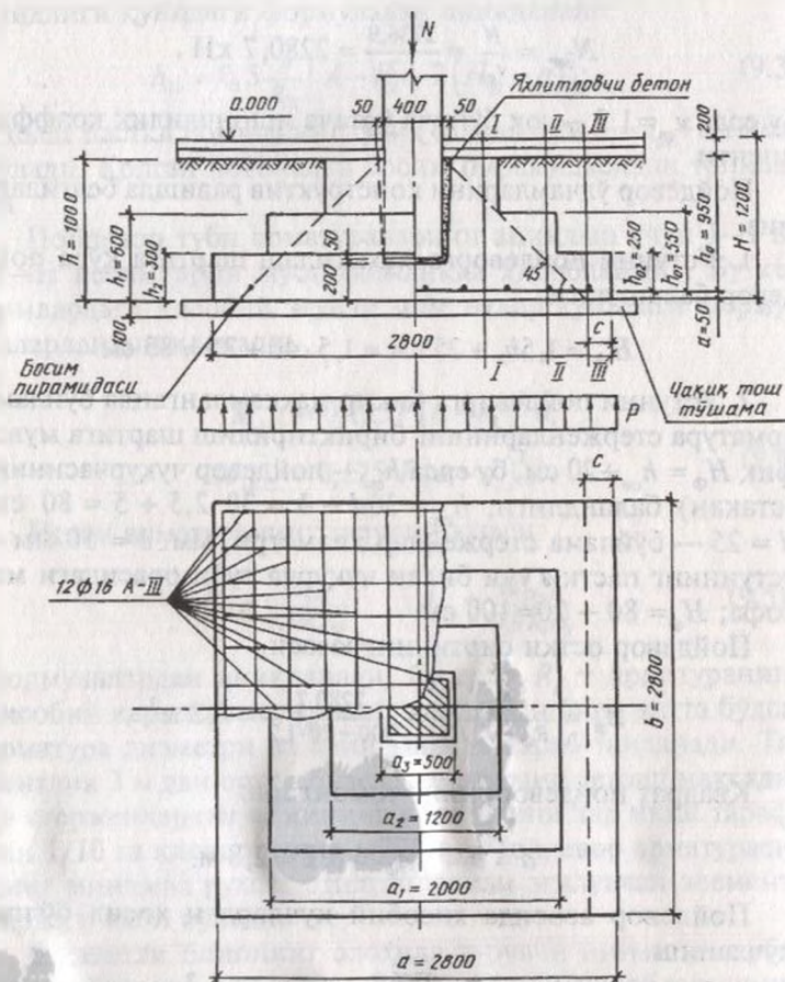
9.3-рasm. Устун остига кўйиладиган темирбетон пойдевор (пойустун).
