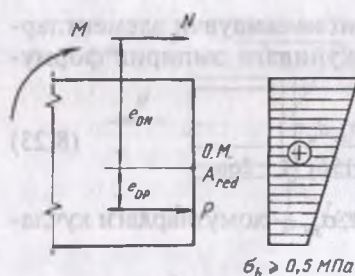
8.4-расм. Нормал ёриқларни ёпилишига доир.
