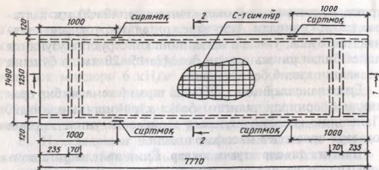
1-1 қирқим
