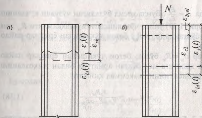
1.14-расм. Бетон ҳўкиши ва тоб ташлашининг темирбетонга таъсири: а — ҳўкишда; б — тоб ташлашда.
