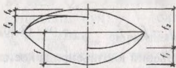
8.8-расм. Чўзилиш зонаси ёрилмаган темирбетон тўсинининг тўлиқ солқилигини аниқлашга доир.
