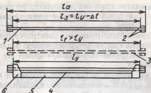
3.2-расм. Арматурани электротермик усулда таранглаш:
