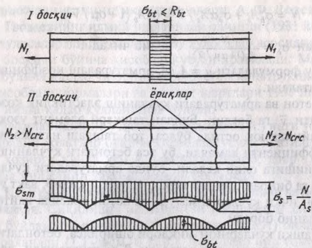
2.1-рasm. Уқ буйлаб чўзилганда кучланиш ҳолати.
