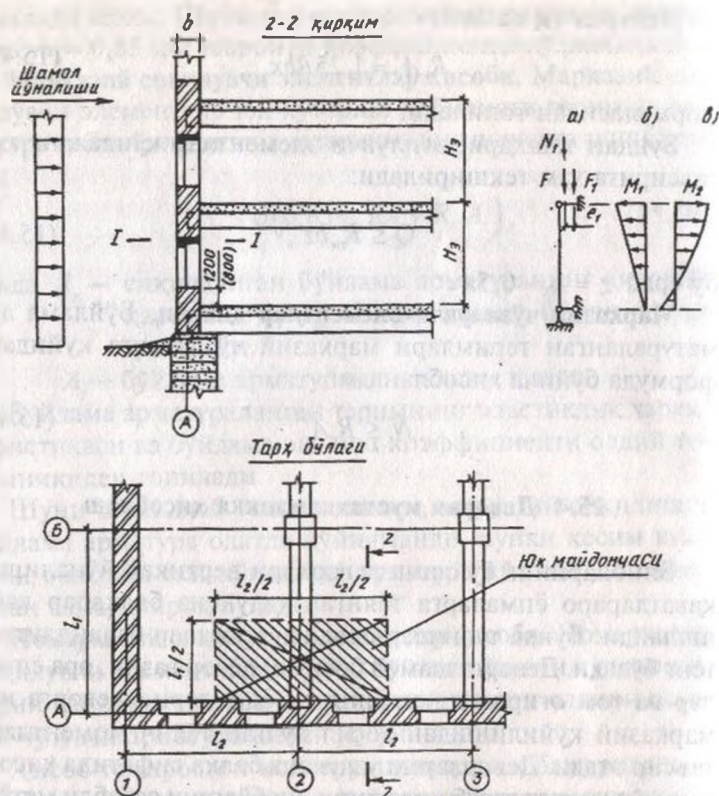
15. 10-расм. Деворлар ҳисобиغا доир тарҳ: а — деворнинг ҳисоблаш тарҳи; б — вертикал юклардан ҳосил бўлган моментлар эпюраси; в — шамол кучидан ҳосил бўлган моментлар эпюраси.
