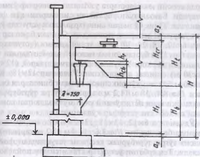
10.1-расм. Устун баланглигини аниқлашга доир.
