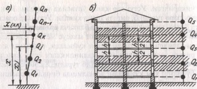
3.4-расм. Қаватлар бўйича вертикал юкларни гуплашга доир тарҳ: а — \eta_k коэффициентини аниқлашга доир схема.
