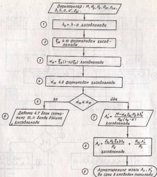
4.10-расм. Қўш арматурили эгиловчи элементларнинг арматура юзаси A_s ва A'_s топиш.
