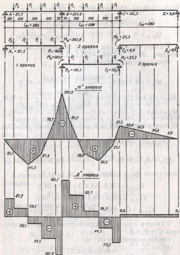
6.7-рasm. Биринчи ва иккинчи оралық муваққат юк билан юкланган- да ригелдаги ҳисобий зўриқишлар элюрасини қуриш.
