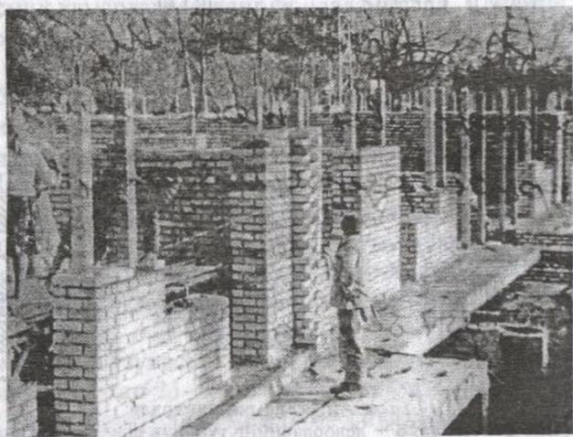
13.18-расм. Темирбетон ўзакли гишт деворнинг қурилиши
