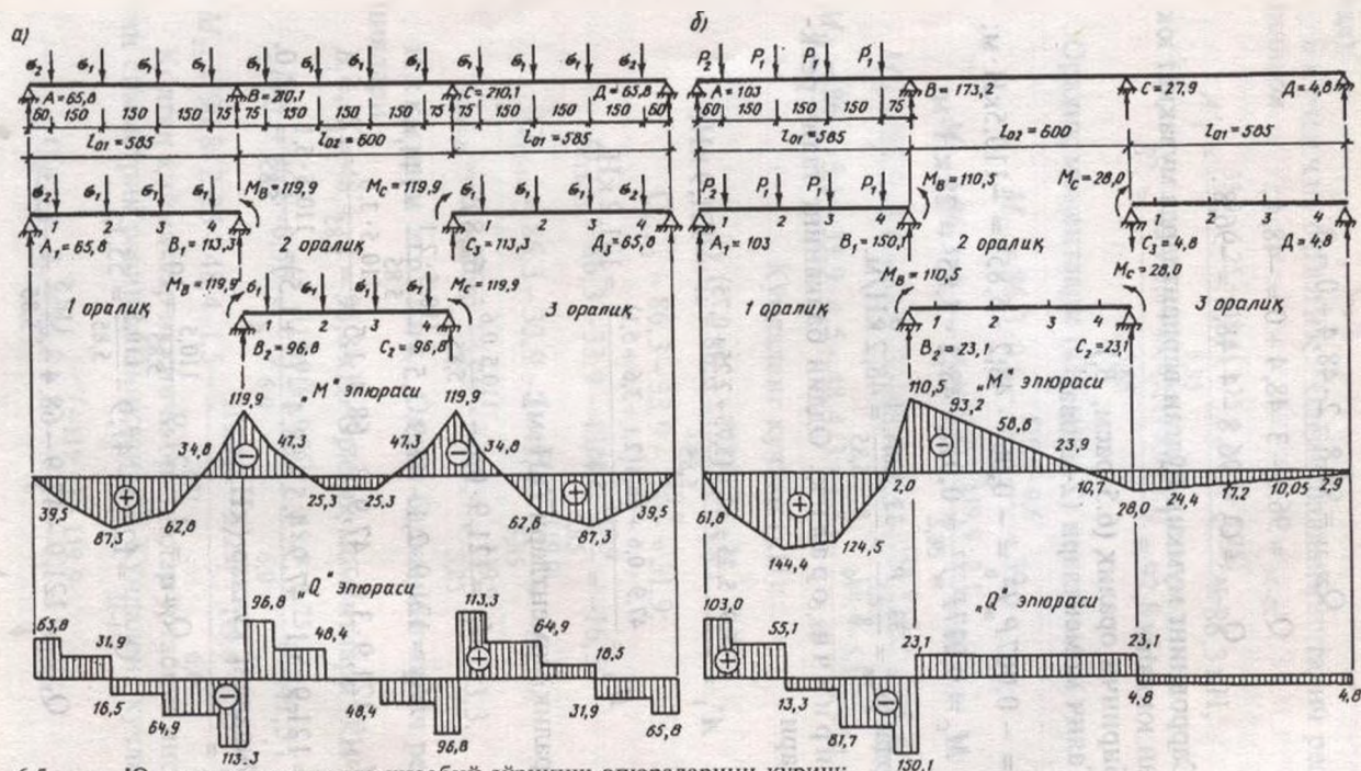
6.5-расм. Юкланган ригелларда ҳисобий зўриқиш эпюраларини қуриш: а – доимий юк ( G_1 = 48,4 кН; G_2 = 33,9 кН) билан юкланганда; б – биринчи оралиқ муваққат юк ( P_1 = 68,4 кН; P_2 = 47,9 кН) билан юкланганда.
