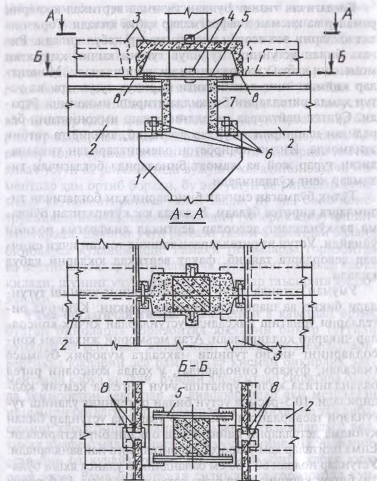
10.5-рasm. Устун ва ригелларнинг бирикуви:
