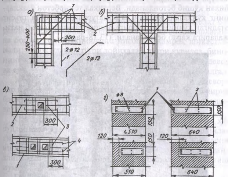
13.17-расм. Антисейсмик камарлар:
