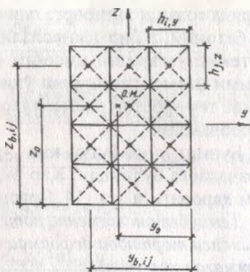
14.3-расм. Элементнинг кесими юзачаларга бўлиш: i, j — кичик юзачаларнинг координаталари: i — 1 дан n у гача j — 1 дан n з гача.
