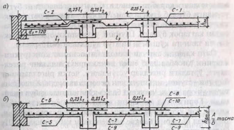
4.15-расм. Плитани арматуралаш: а — пайвандланган урама симтўрлар; б — пайвандланган ясси симтўрлар.
