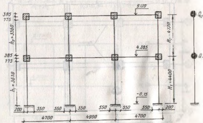
13.9-расм. Кўндаланг рамани ҳисоблаш тарҳи.
