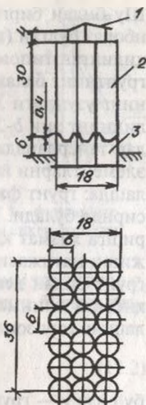
12.7-расм. Доиравий силослар тарҳи:
