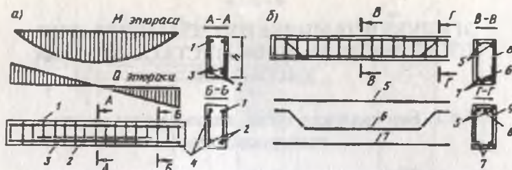
4.2-расм. Бир оралиқли түсинларни арматуралаш: а — пайванд каркаслар; б — туқима каркаслар.
