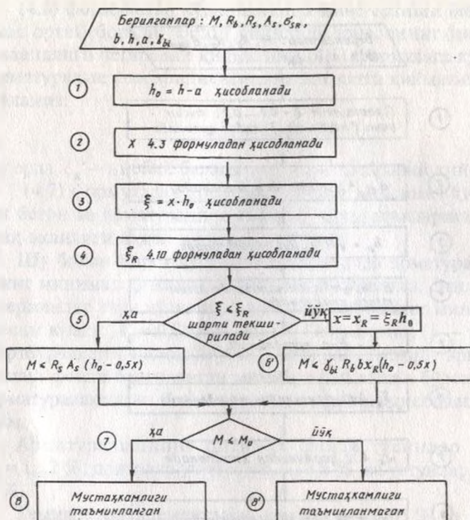
4.8-расм. Эгилувчи элементларни мустақкамликка ҳисоблаш.
