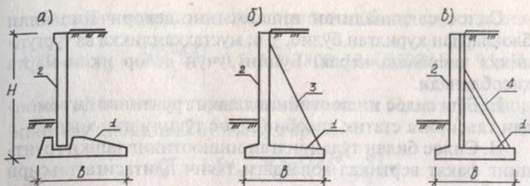
12.9-расм. Юпқа тиргак деворларнинг турлари: 1— фундамент плитаси; 2 — девор плитаси; 3 — контрфос; 4 — анкер тортқич.
