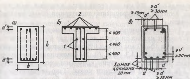
4.3-расм. Пайванд ва тұқима каркас билан арматураланган түсиннинг кўндаланг кесимлари:
