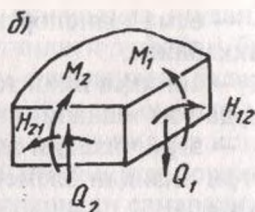
11.11-расм. Қобик кесимларида вужудга келадиган зүриқишлар.
